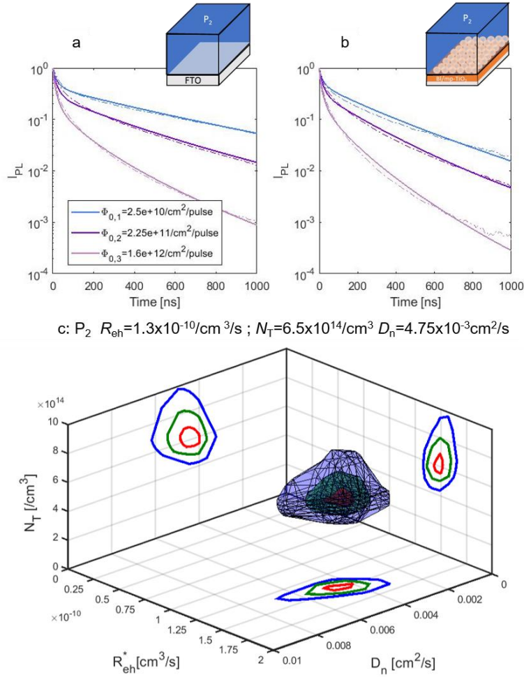
Figure R4 Déclins de I_{PL} expérimentaux (lignes en pointillés) et ajustés numériquement (lignes simples) pour une pérovskite à cations mixtes b). Différents ordres de grandeur du niveau d'illumination ont été testés. (c) Les iso-surfaces montrant un ensemble de paramètres ( R_{eh}^* D_n N_T ) conduisant à une erreur de reconstruction ne dépassant pas 10% (rouge), 20% (vert), 50% (bleu) de l'erreur de reconstruction optimale.
