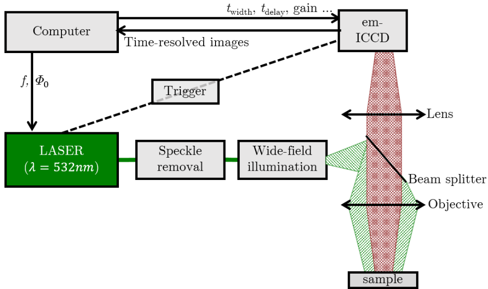
Figure R3 Schéma du set-up TR-FLIM (Computer : ordinateur / Time-resolved images : images résolues en temps / Speckle removal : filtre anti-speckle / Wide-field illumination : illumination grand champ / Lens : objectif / Beam Splitter : lame séparatrice / Objective : objectif / Sample : échantillon)
