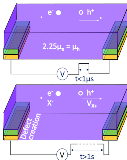
Figure R6 Résumé des 2 expériences à l'étude dans le chapitre 6. La couche mince de pérovskite (violet) est contacté latéralement par des couches d'ITO (vert) et or (jaune). Un biais électrique rapide ( < 1 \mu\text{s} ) ou plus long est appliqué. Le champ résiduel est de 2500 \text{ V/cm} , car on considère un canal de 20 \mu\text{m} avec un potentiel électrique de 5 \text{ V} .
