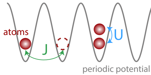
Figure 1: Particules bosoniques piégées dans un potentiel périodique
