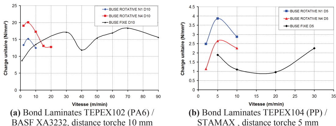
Figure 4-31 Comparaison des types de buse
