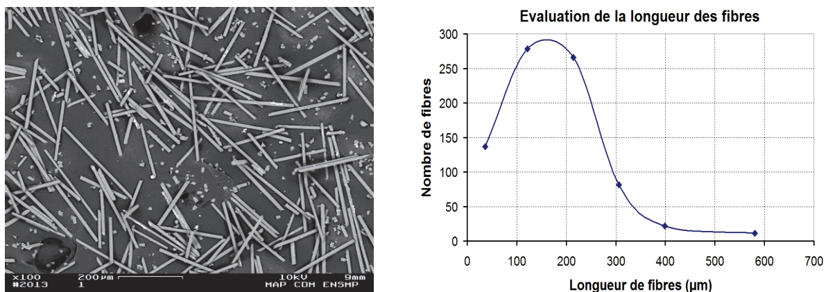
Figure 5-19 Détermination de la longueur moyenne des fibres par observation au MEB
