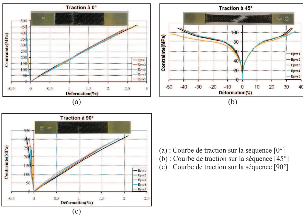
Figure A-2 Contrainde vs déformation pour le TEPEX 104-RG600/47% BOND LAMINATES
