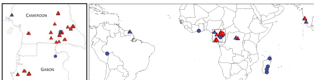
Figure 1. Distribution spatiale des jeux de données utilisés. Les points et les triangles représentent les sites où des arbres ont été coupés/pesés et les sites où des parcelles d'inventaire ont été établies, respectivement. La couleur rouge indique que les données ont été collectées par l'IRD. La couleur bleue indique que les données proviennent de la littérature, d'institutions ou de chercheurs partenaires.
