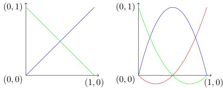
FIGURE 1.12 – Gauche : Fonctions de forme P^1 . Droite : Fonctions de forme P^2 .
