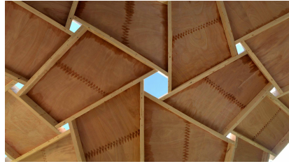
(d) Beam network of a shell-nexorade hybrid at École des Ponts, Champs-sur-Marne, France [Mesnil et al., 2018a] (Photo credits: Romain Mesnil)
