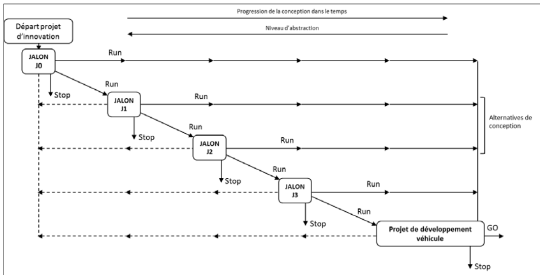
Figure 6. Développement jalonné d'un projet de recherche et d'exploration (inspirée de [139, OZER] et des processus internes à Renault).
