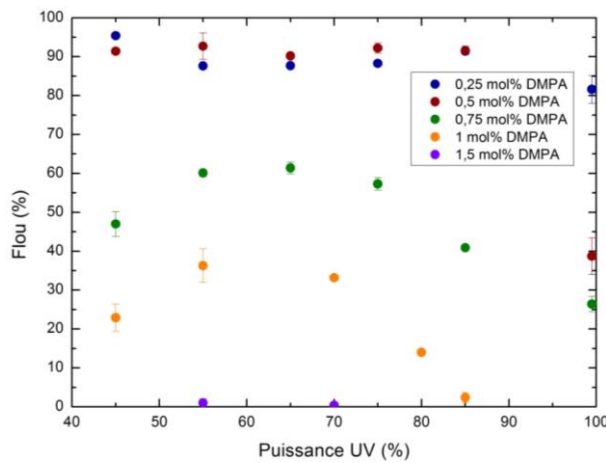
Figure 151. Influence de la puissance UV sur le flou de films de HEA, 2 mol% réticulant, 3 m/min, épaisseur 20 μm pour différentes concentrations en amorceur (100% de puissance correspond à 1,5 W/cm 2 ).
