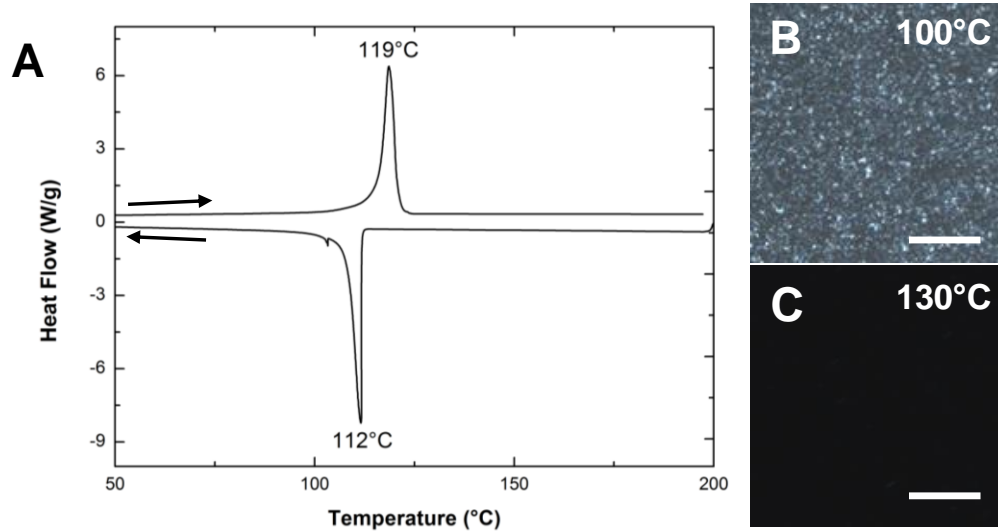
Figure 84. (A) DSC du mélange équimolaire de PE 1700 -Thy/DAT-PE 1700 (exo down, 10°C/min) et microscopie optique polarisée à (B) 100 °C et (C) 130°C (échelle 50 μm).
