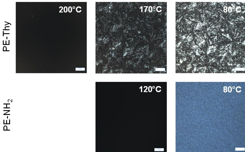
Figure 60. Images en microscopie optique polarisée de PE 1700 -Thy (haut) et PE 1700 -NH 2 (bas) à différentes températures obtenues lors du refroidissement de l'échantillon depuis 200°C à 10°C/min (échelle 100 µm).
