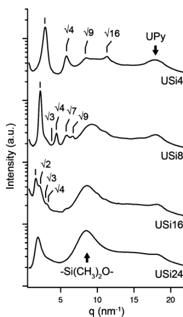
Figure 16. SAXS de UPy-PDMS-UPy monodisperses pour différentes tailles de chaîne (4, 8, 16 et 24 motifs -\text{Me}_2\text{SiO}- ). 37
