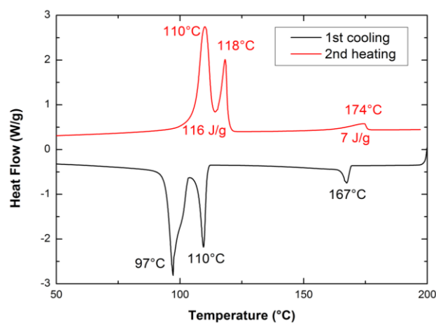
DSC de PE_{1500}\text{-Thy} avec une fonctionnalité de 80% (exo down, vitesse 10^\circ\text{C}/\text{min} ).
