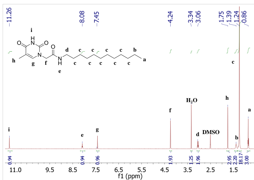
^1\text{H} RMN de \text{C}_{12} -Thy (DMSO- d_6 297 K).
