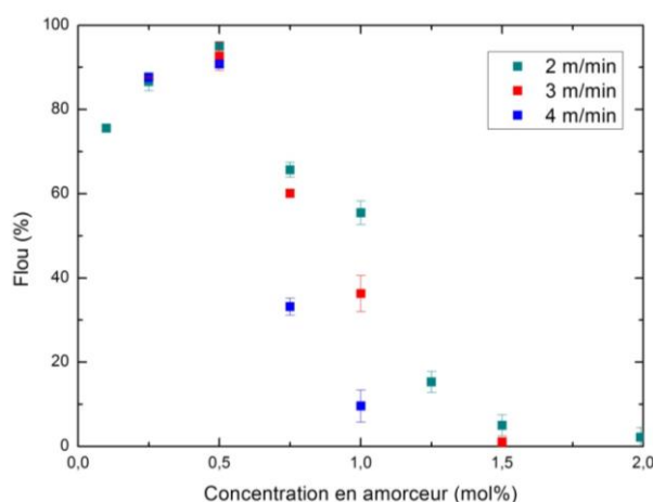
Figure 152. Influence de la concentration en amorceur sur le flou pour des films de HEA, 2 mol% réticulant, 800 mW/cm 2 , épaisseur 20 μm à différentes vitesses du convoyeur.
