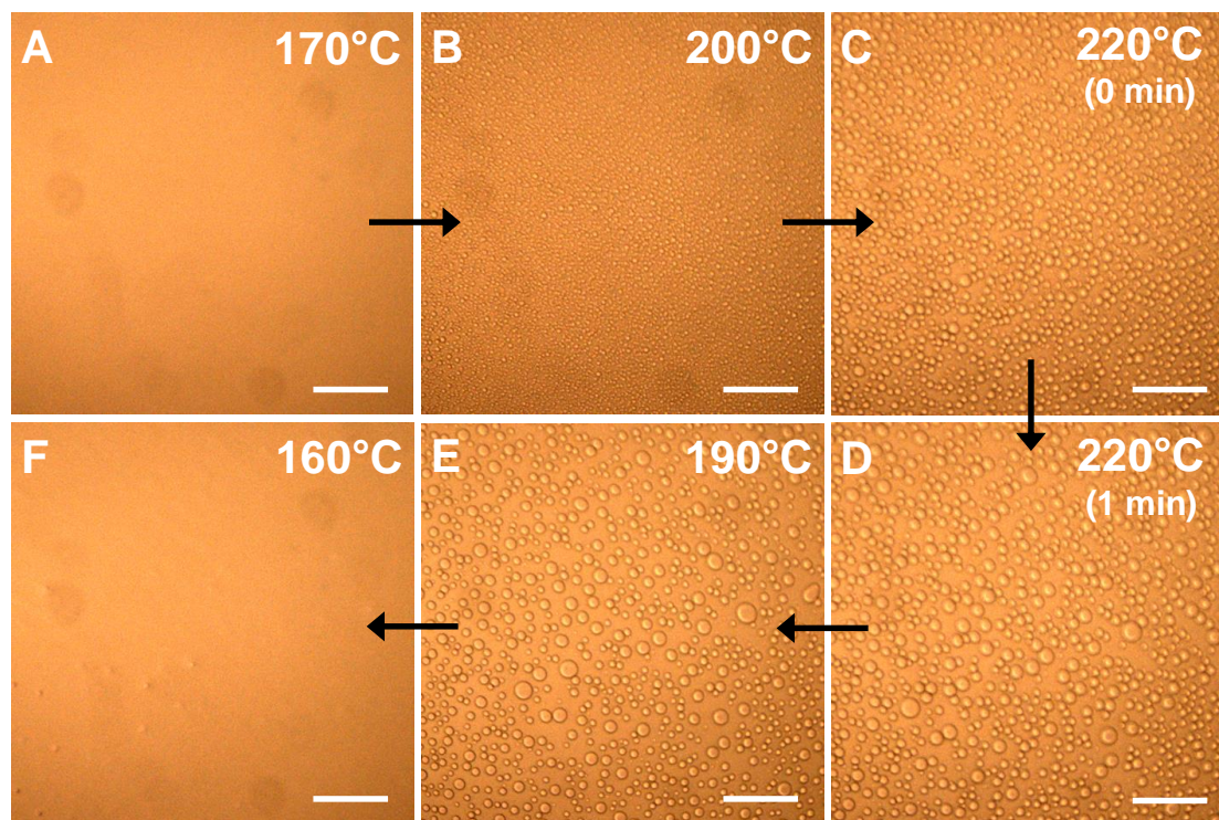
Figure 108. Microscopie optique du mélange PE 1500 -DAT/Thy-PDMS 1660 -Thy à différentes températures en chauffant jusqu'à 220°C (température maintenue 1 minute) puis en refroidissant à 160°C (chauffage et refroidissement à 30°C/min, sans polariseurs). Echelle 100 μm.
