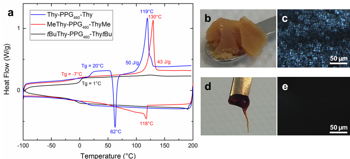
Figure 35. a) DSC de Thy-PPG 460 -Thy, MeThy-PPG 460 -ThyMe et t BuThy-PPG 460 -ThytBu à 10°C/min (exo down). Photos des échantillons b) MeThy-PPG 460 -ThyMe et d) t BuThy-PPG 460 -ThytBu et en microscopie optique polarisée à 20°C de c) MeThy-PPG 460 -ThyMe et e) t BuThy-PPG 460 -ThytBu.
