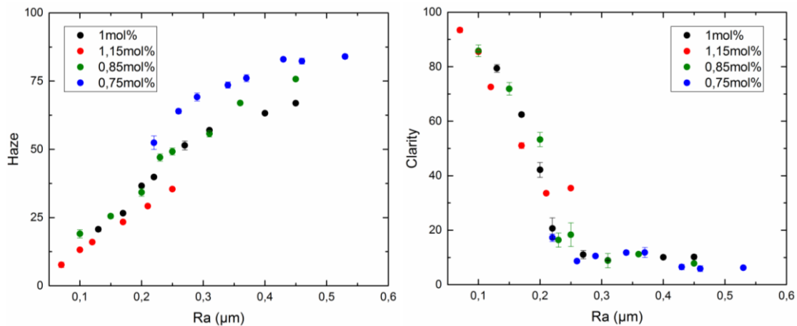
Figure 154. Evolution du flou et de la clarté en fonction du paramètre de rugosité R_a pour des films de HEA (20 \mu\text{m} , 2 mol% réticulant) obtenus avec des concentrations en amorçeur et intensités UV variables.
