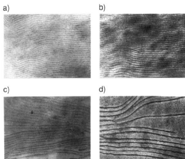
Figure 103. TEM du mélange HO_2C-PEO_{8,6k}-CO_2H/H_2N-PS-NH_2 pour différentes tailles de chaînes PS a) 5,8k, b) 19k, c) 30k et d) 76k. 42
