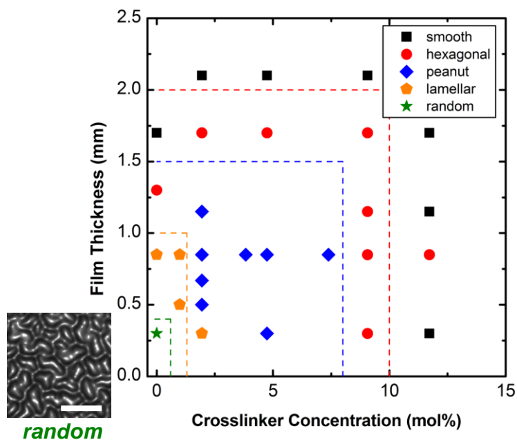
Figure 137. Diagramme de phase d'existence des morphologies en fonction de la concentration en amorceur et de l'épaisseur du film (monomère PEA, amorceur 0,4 mol%, irradiation 30 s). Echelle 50 μm.
