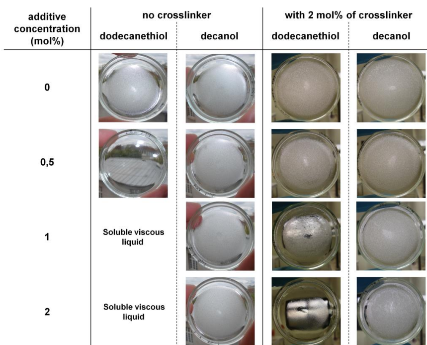
Figure 138. Photos de la surface de films de PEA obtenus en présence de dodécane-thiol (agent de transfert) ou du décanol (référence), avec 2 mol% ou sans réticulant (amorçeur 0,4 mol%, épaisseur 1 mm, irradiation 60 s).
