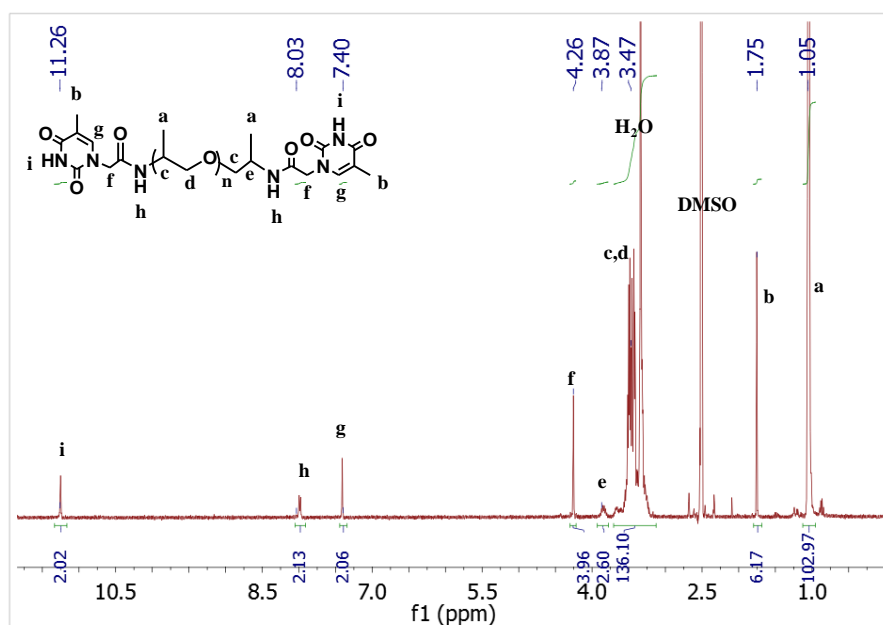
1 H RMN de Thy-PPG 2000 -Thy (DMSO-d 6 297 K).
