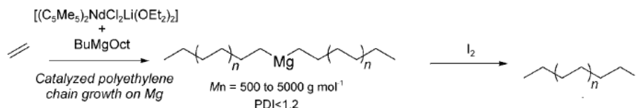
Figure 47. Schéma réactionnel de la synthèse d'un PE-I monofonctionnel. 5
