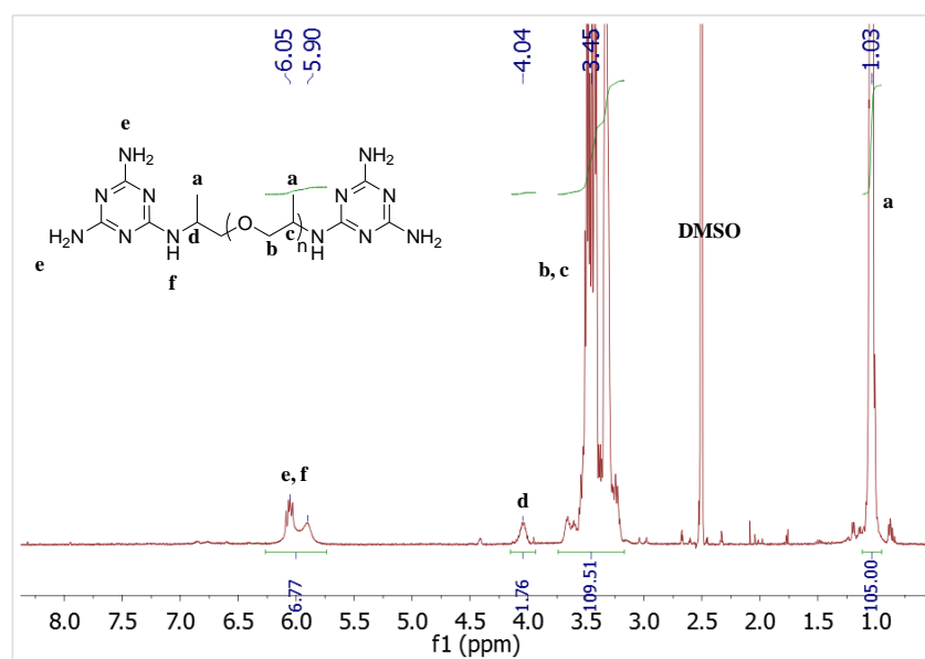
1 H RMN de DAT-PPG 2000 -DAT (DMSO-d 6 297 K).
