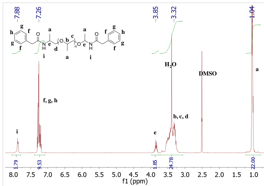
^1\text{H RMN} de Ph-PPG 460 -Ph (DMSO-d 6 297 K).
