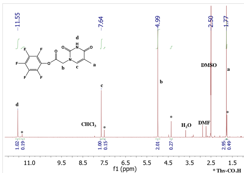
^1\text{H} RMN de Thy-PFP (DMSO- d_6 297 K).
