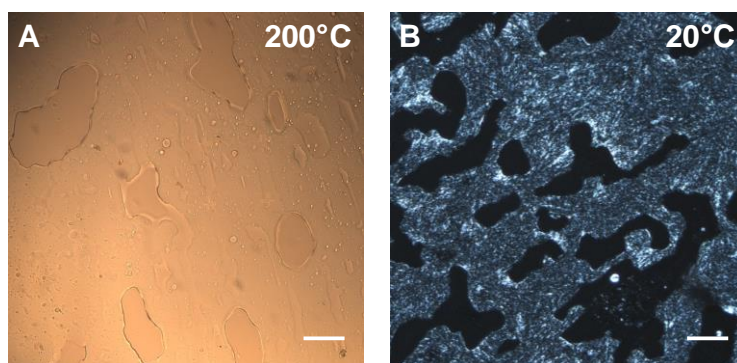
Figure 106. Microscopie optique du mélange PE 1500 -Thy/Thy-PDMS 1660 -Thy A) à 200°C sans polariseurs et B) à 20°C entre polariseurs croisés. Echelle 100 µm.
