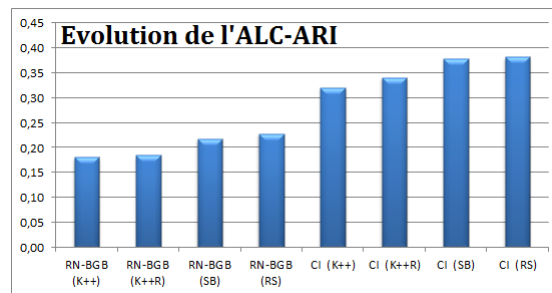
FIGURE 4.17 – Évolution de l'ALC-ARI (en test) suivant le prétraitement et la méthode d'initialisation utilisée
