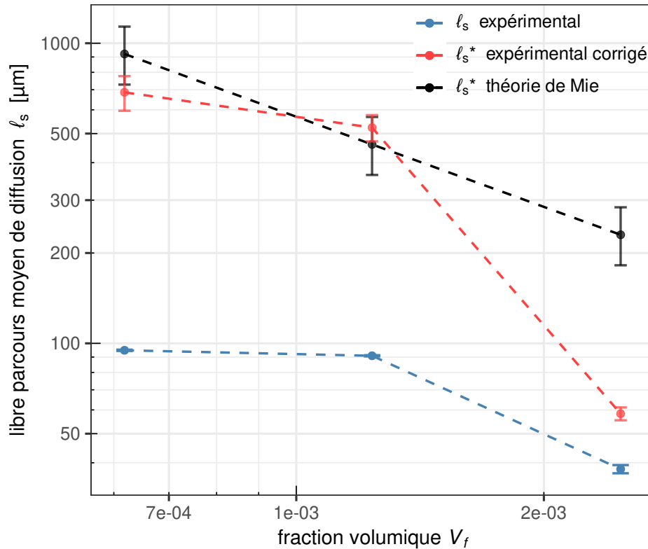
Figure III.23 – Libres parcours moyens de diffusion de gels d'agarose contenant une solution monodisperse de billes de polystyrène de diamètre 0,51\mu\text{m} à différentes concentrations. La courbe noire représente les valeurs calculées par la théorie de Mie (avec en barre d'erreur les valeurs à 650\text{nm} et 800\text{nm} ), la courbe bleue celles mesurées par analyse du signal de l'OCT plein champ et la courbe rouge les valeurs mesurées corrigées en tenant compte de la diffusion du gel d'agarose à 1%. Les deux axes sont en échelle logarithmique pour comparer les deux courbes à des droites.
