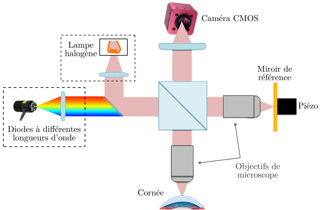
Figure III.5 – Schéma du montage d'OCT plein champ de LLTech modifié pour pouvoir utiliser des sources à différentes longueurs d'ondes.
