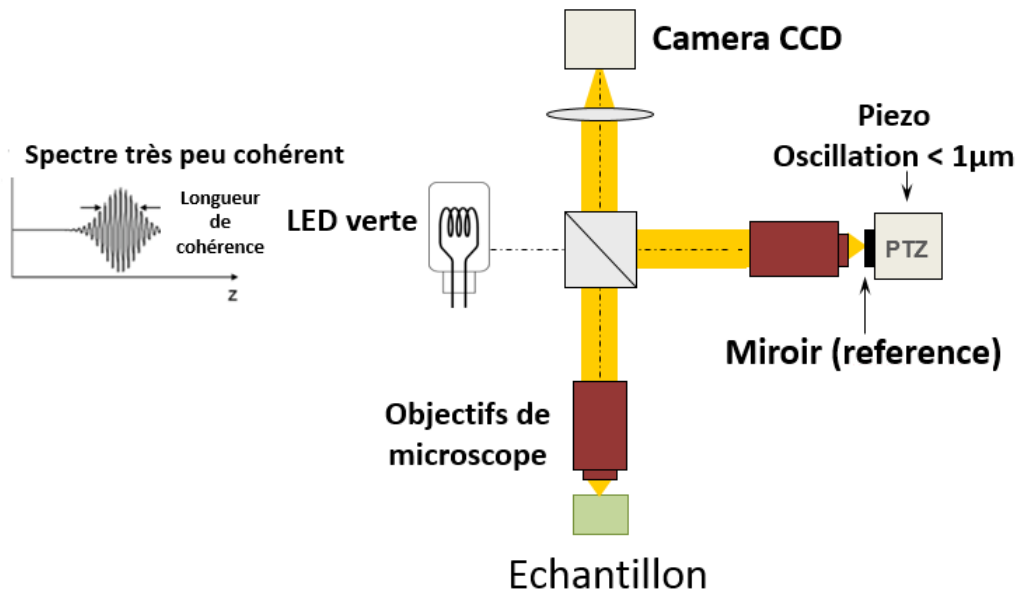
Figure III.3 – Schéma d'un montage d'OCT plein champ - https://upload.wikimedia.org/wikipedia/commons/9/9b/Oct_FF.png
