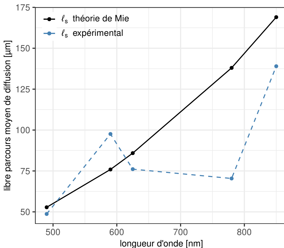
Figure III.25 – Libre parcours moyen de diffusion en fonction de la longueur d'onde pour une solution de billes de polystyrène de 0,51 \mu\text{m} de diamètre concentrée à 0,5 \% . La courbe noire représente les valeurs calculées par la théorie de Mie et la courbe bleue représente les valeurs extraites des données d'OCT plein champ.
