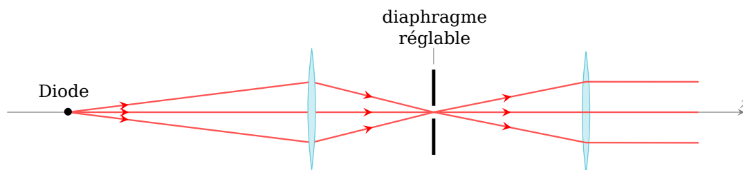
Figure III.26 – Schéma d'un montage permettant de régler la cohérence spatiale de la source en changeant l'ouverture du diaphragme.
