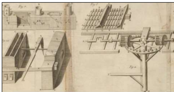
Figure 91 - ventilateur Hales 430 (1744)
