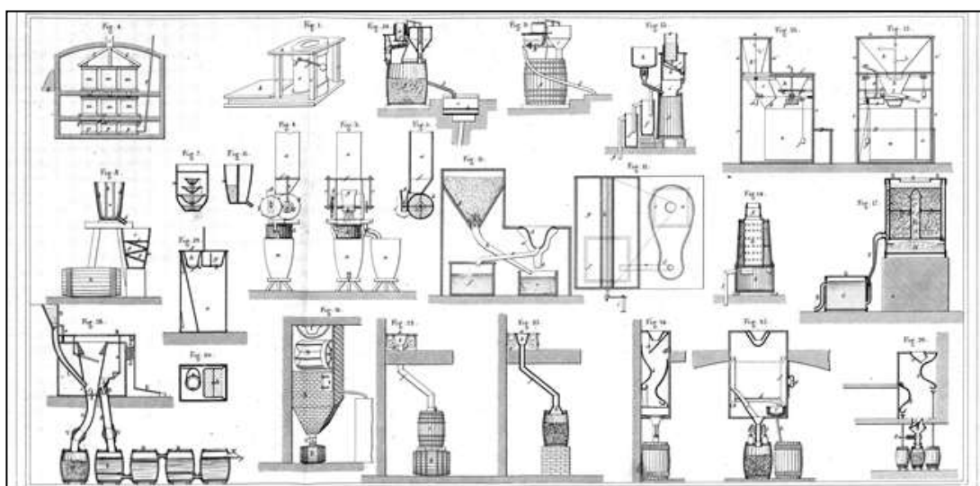
Figure 73 - appareil séparateur désinfecteur Guibout et Sanson 322 (1848)
