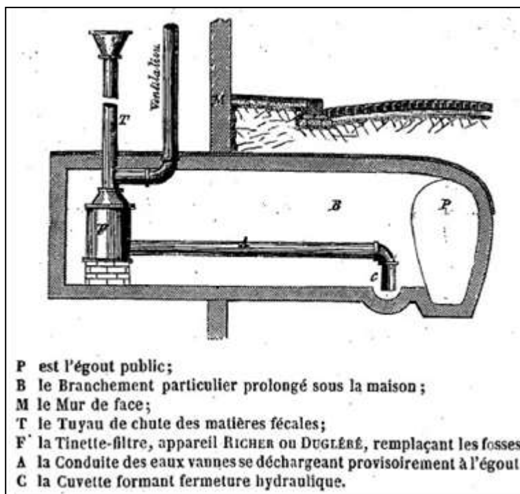
Figure 66 - système Ducléré sans fosse fixe 302 (1864)
