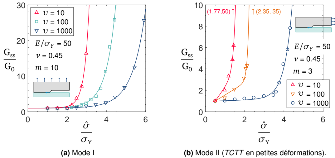
Figure 9 Énergie de fracture en régime stationnaire vs. contrainte cohésive, dans un matériau visco-plastique : effet de la vitesse de propagation \nu .
