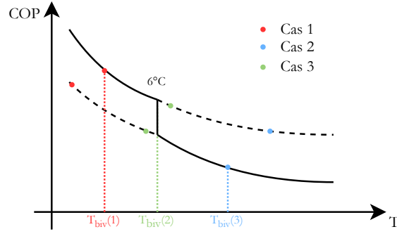
FIGURE F.3 – Représentation des solutions permettant l'identification du point de bivalence PC-CR ou CR-m/a
