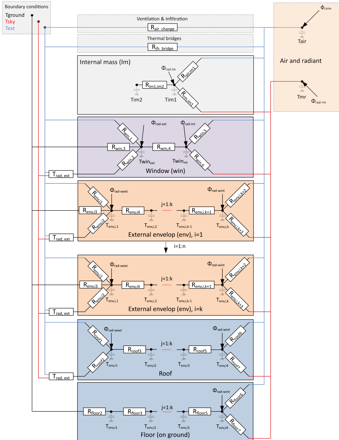
FIGURE 2.5 – Modèle du bâtiment implémenté dans l'outil de simulation urbaine DIMOSIM. Source : Garreau [62]
