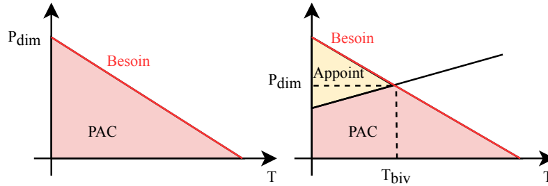
FIGURE 3.16 – Les modes de fonctionnement des pompes à chaleur : monovalent et bivalent
