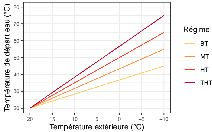
FIGURE 3.15 – Lois de régulation de température de l'eau de chauffage pour une température de base de -10°C.
