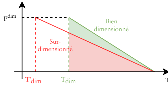
FIGURE 4.3 – Sur-dimensionnement du chauffage suite à une rénovation thermique
