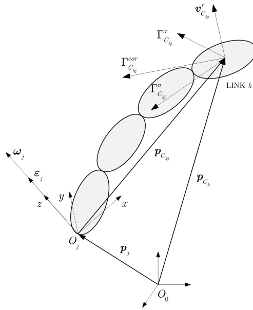
Figure 6.18: Accélérations tangentielles, normales et de Coriolis du centre de masse k .
