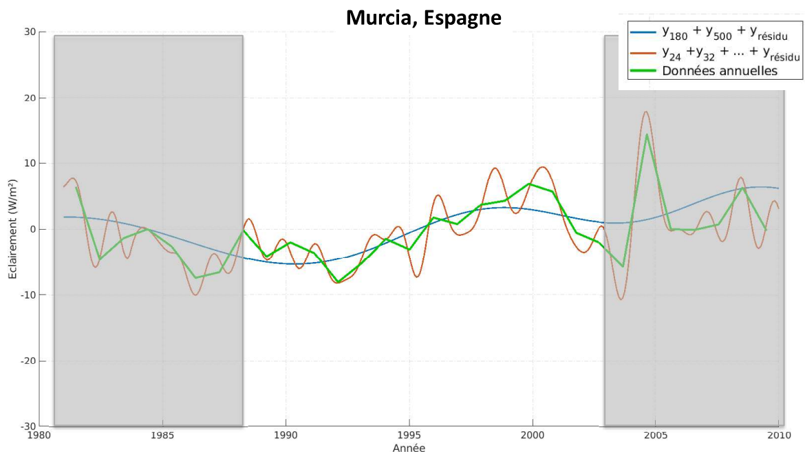
Figure 37 : Equivalent de moyenne annuelle, de moyenne annuelle glissante, et du filtrage par un filtre passe bas gaussien de 13 ans. Ces équivalents sont construits par une somme d'éléments de la décomposition temps-fréquence de la station Murcia.
