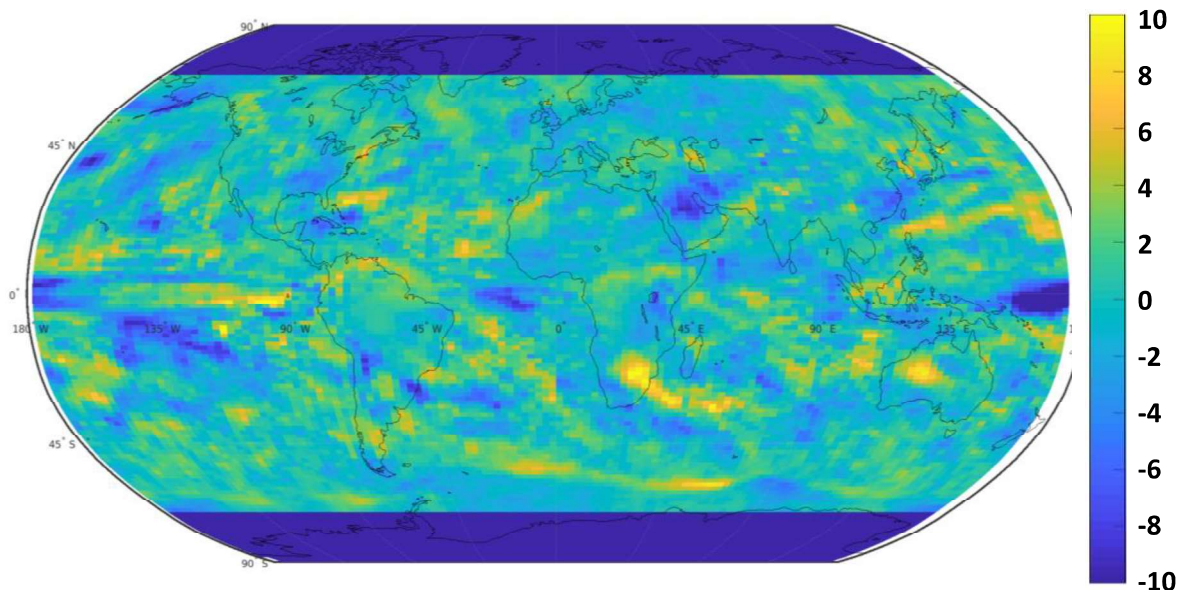
Figure 47 : Ecarts relatifs entre les valeurs de variance de la réalisation du modèle IPSL-CM6A-LR sélectionnée, et la valeur de variance moyenne entre les 31 réalisations. L'écart relatif, calculé pour chaque pixel, est exprimé en pourcentage et représentée en couleurs.
