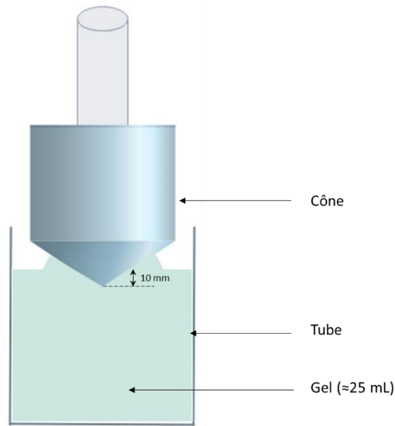
Figure S3 : Schéma du dispositif de mesure de texture des gels formés au bain-marie
