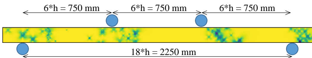
Figure 85 : Variation de la fibre neutre en fonction de la cartographie du module d'élasticité local.
