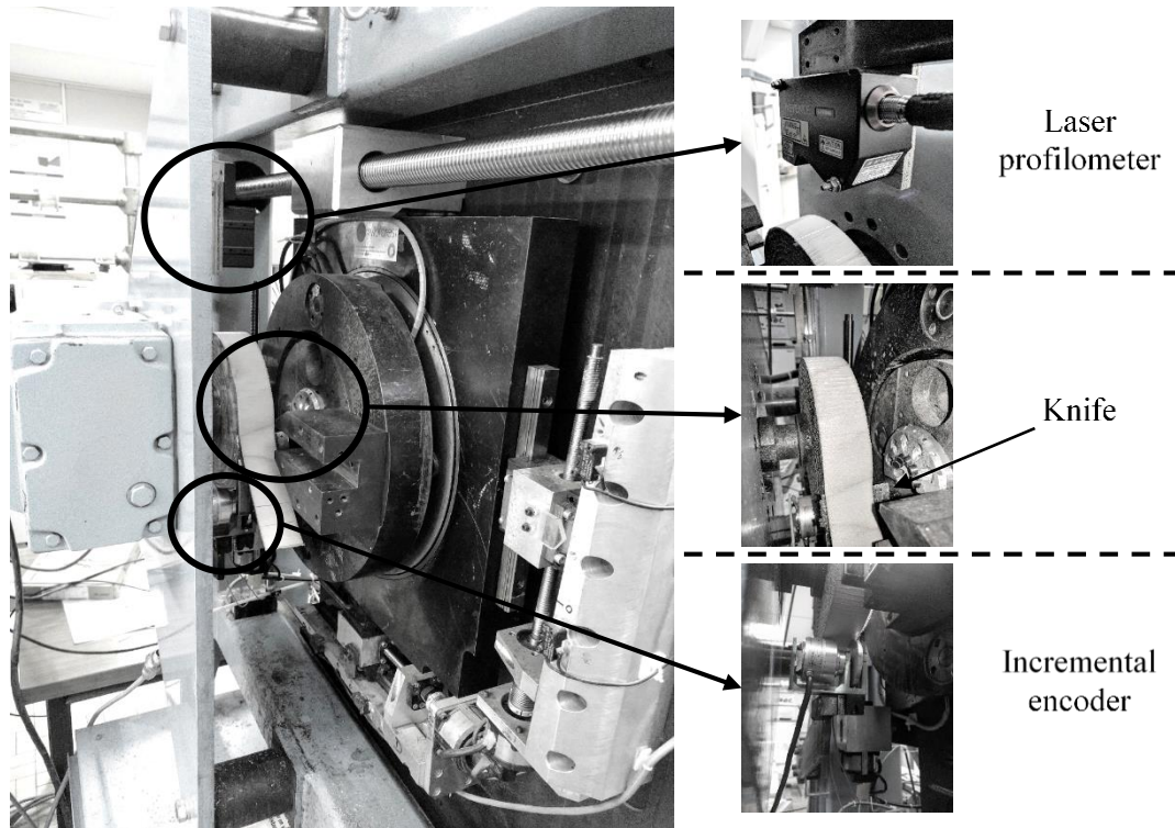
Figure 30 : Microdérouleuse avec profilomètre laser [54]
