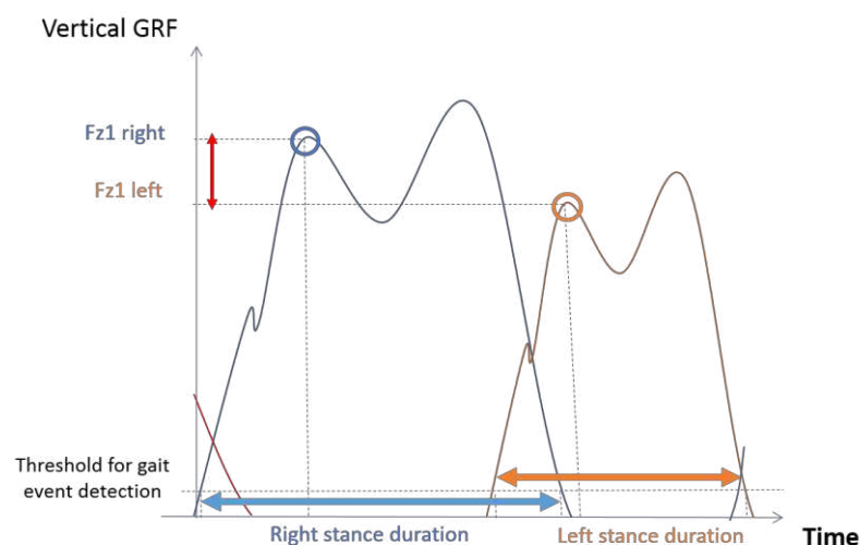
Figure 62 : Durée de phase d'appui (stance duration) et pic d'effort de début d'appui (Fz1) dérivé de la composante normale des efforts de réaction au sol (Vertical GRF) avec des semelles de pression droite (Right – courbe bleue) et gauche (Left – courbe orange)
