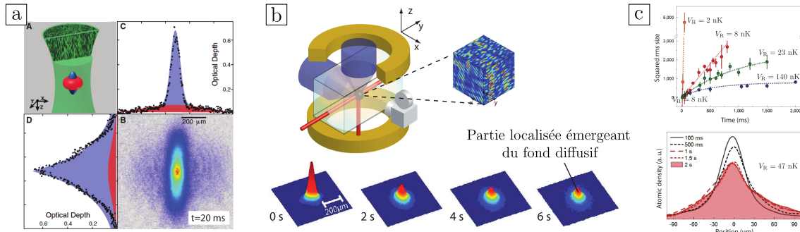
FIGURE 2.6 – Observation de la localisation d’Anderson à trois dimensions avec des atomes ultra-froids. a : Localisation d’une partie du nuage de ^{40}\text{K} à temps très court. Une partie localisée émerge du centre d’un fond balistique. Figure tirée de [54]. b : Observation à temps très long d’une partie localisée du nuage de ^{87}\text{Rb} qui se démarque d’un fond très peu diffusif dans un désordre quasi-isotrope. Figure tirée de [47]. c : Localisation d’un nuage de ^{39}\text{K} complet dont les interactions sont annulées à l’aide d’une résonance de Feshbach. Figure tirée de [107].
