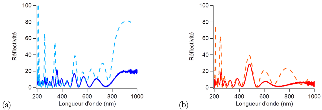
Figure III 34 Comparaison des données issues de la simulation (lignes pointillées) et des expériences (lignes continues) pour un miroir pNIPAM / Au composé de 4 périodes dans les états gonflé (a) et collapsé (b).
