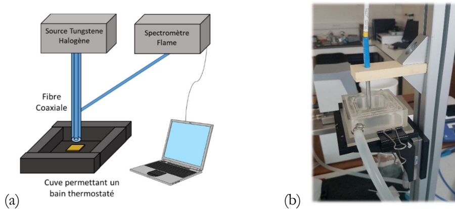
Figure III 13 (a) Schéma du montage expérimental de spectrométrie. (b) Photo du montage expérimentale.
