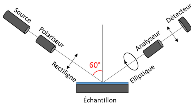
Figure Annexe 1 Montage de fonctionnement d'un ellipsomètre.
