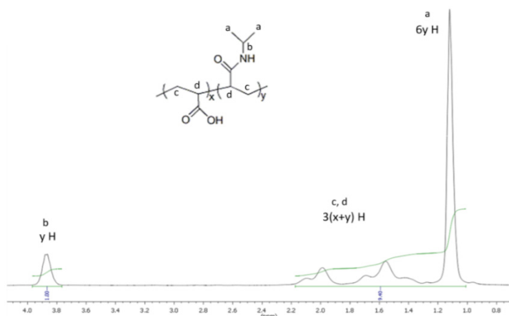
Figure II 4 Spectre RMN ^1\text{H} du poly(NIPAM-co-AA) dans \text{D}_2\text{O} synthétisé par polymérisation radicalaire conventionnelle.
