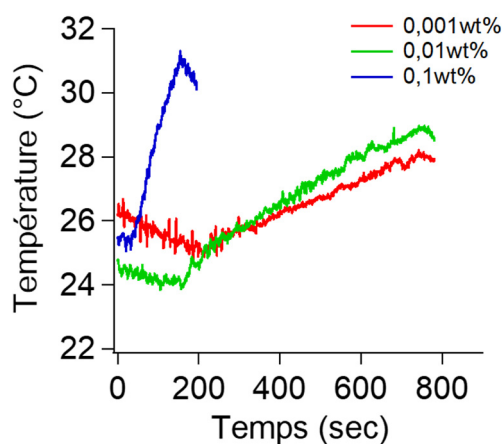
Figure VI 33 Evolution de la température lors de l'application du champ magnétique pour différentes concentrations massiques en nanoparticules en fonction du temps.
