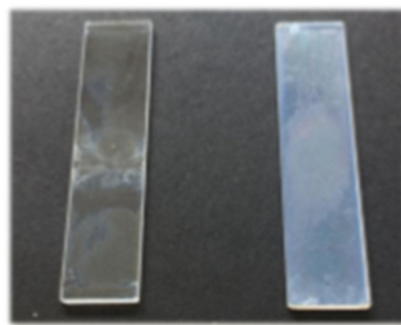
Figure IV 4 Film de TiO 2 -MSMA (à gauche) et film obtenu avec une suspension colloïdale de nanoparticules d'oxyde de titane (à droite). Les deux films ont une épaisseur de l'ordre de 100 nanomètres.
