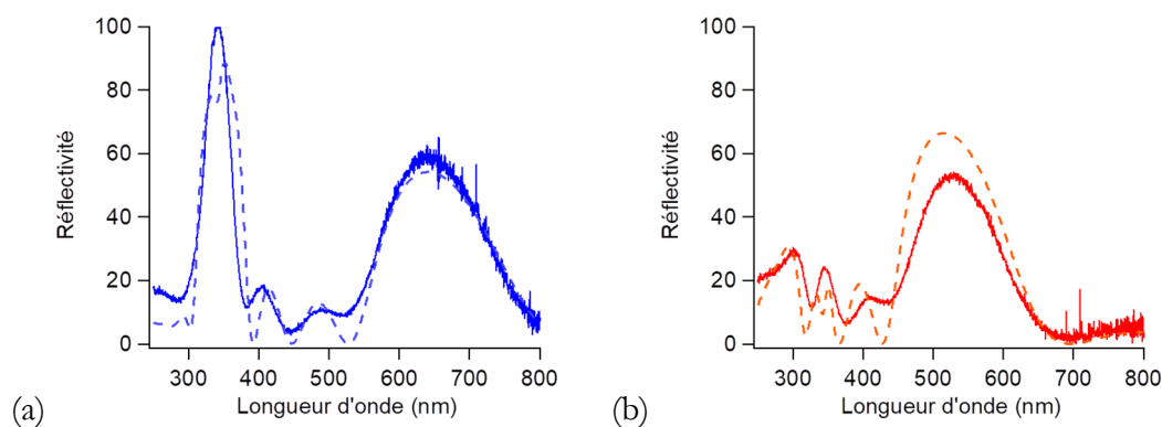
Figure IV 18 Spectres expérimentaux (ligne continue) et spectres simulés (lignes pointillées) pour un miroir de Bragg composé de 4 périodes de pNIPAM et de TiO 2 :MSMA (40:1) déposées sur une lame de verre dans l'eau à 20°C (a) et dans l'eau à 40°C (b). Pour les spectres simulés les valeurs de gonflement sont de 200% dans l'eau à 20°C (a) et de 140% dans l'eau à 40°C (b).
