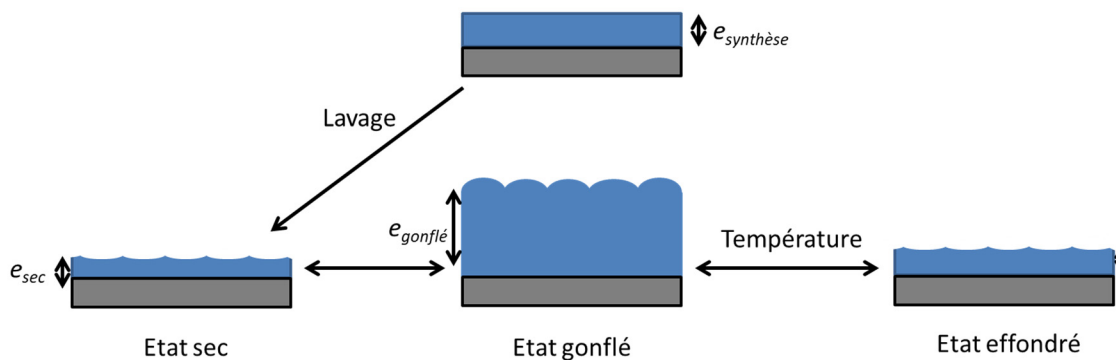
Figure V 14 Représentation schématique des instabilités selon l'état de gonflement du film.
