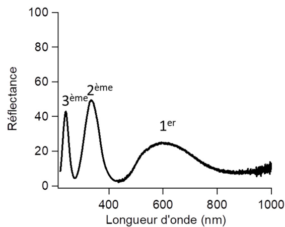
Figure III 14 Spectre de réflectance d'une bicouche pNIPAM 200 nm / Au (6 nm) dans l'air en incidence normale.
