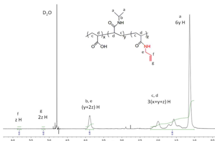
Figure II 6 Spectre RMN ^1\text{H} du poly(NIPAM-co-AA) dans \text{D}_2\text{O} synth tis  par polym risation radicalaire conventionnelle puis post-fonctionnalisation avec de l'allylamine.
