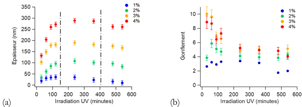
Figure V 1 Epaisseur d'un film d'hydrogel de pNIPAM obtenue en fonction du temps d'irradiation UV pour différentes concentrations de la solution de polymère déposée par spin-coating. Mesures réalisées à l'AFM à sec (a). Gonflement d'une couche de pNIPAM en fonction du temps d'irradiation UV lors de la synthèse pour différentes concentrations déposées. Mesures réalisées à l'AFM dans l'eau à 20°C (b). Les lignes en pointillées sur la figure (a) sont une aide visuelle pour séparer les différents régimes.
