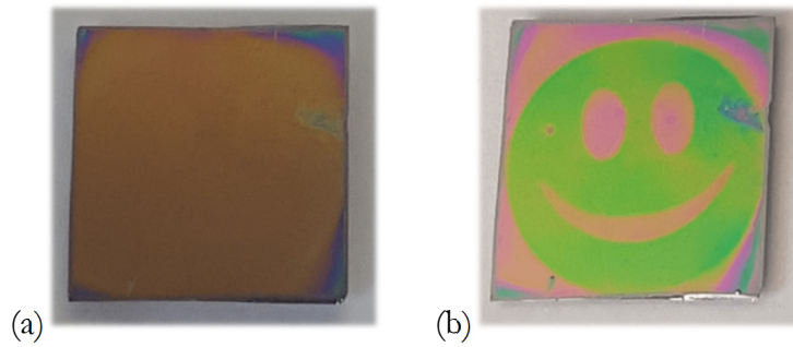
Figure V 3 Photographie dans l'air (a) et dans l'eau à 20°C (b) d'un échantillon de pNIPAM, de deux centimètres de côté, insolé pendant 2 heures avec un masque puis 2 heures sans masque uniformément. Il est ensuite recouvert d'une couche d'or déposée par pulvérisation cathodique.
