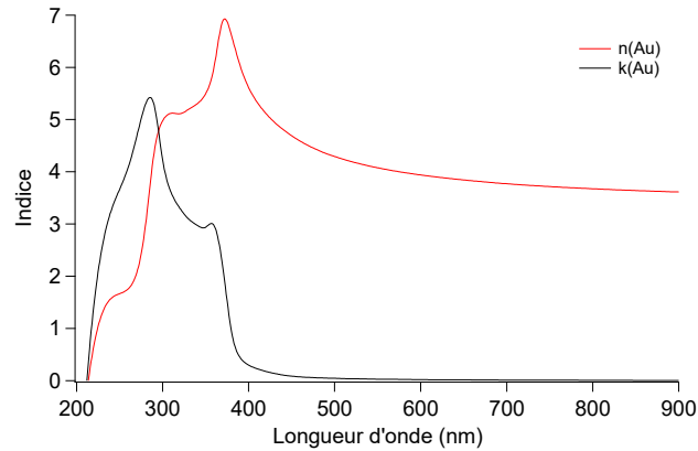
Figure III 30 Courbe de dispersion de l'indice optique d'une couche mince d'or en fonction de la longueur d'onde.
