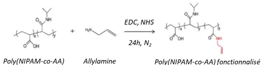
Figure II 5 Repr sentation de la r action de fonctionnalisation de l'acide acrylique par l'allylamine.
