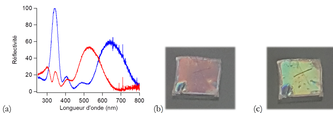
Figure IV 17 (a) Spectre de réflexion d'un miroir de Bragg composé de 4 périodes de pNIPAM et de TiO 2 :MSMA (40:1) déposées sur une lame de verre dans l'eau à 20°C (ligne continue bleue) et dans l'eau à 40°C (ligne continue rouge). Photographie de l'échantillon dans l'eau à 20°C (b) et dans l'eau à 40°C (c).
