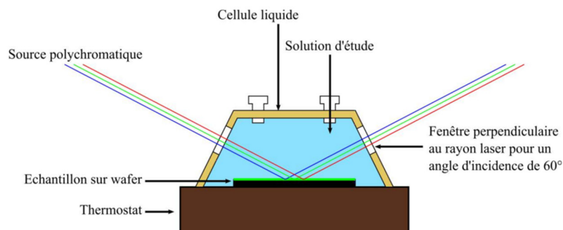
Figure Annexe 4 Représentation schématique de la cellule liquide [119].
