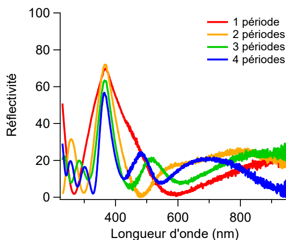
Figure III 24 Spectres de réflexions dans l'air à 20°C de dispositifs pNIPAM (120 nm) / Or (5 nm) présentant différents nombres de période.
