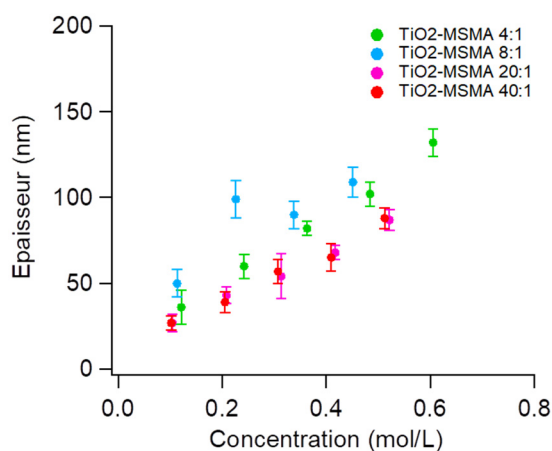
Figure IV 3 Épaisseur de la couche d'oxyde de titane obtenue en fonction de la concentration dans la solution spin-coatée pour différents ratio \text{TiO}_2\text{:MSMA} .
