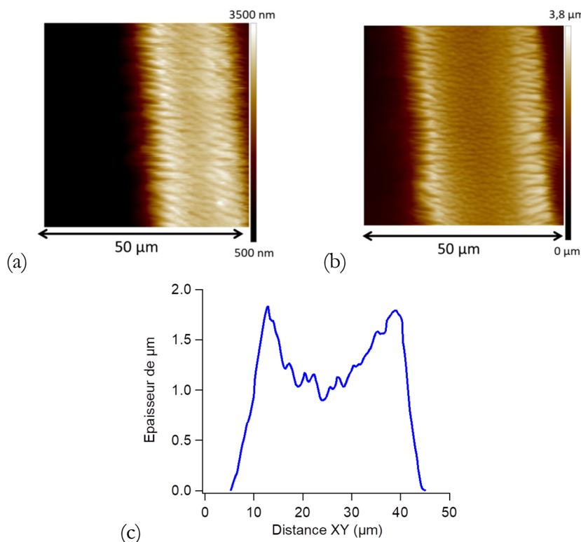
Figure V 18 Images AFM de lignes d'hydrogel de pNIPAM de 10 μm (a) et 20 μm (b) de large dans l'eau à 20°C. Profil d'épaisseur d'une coupe de la ligne de 20 μm.
