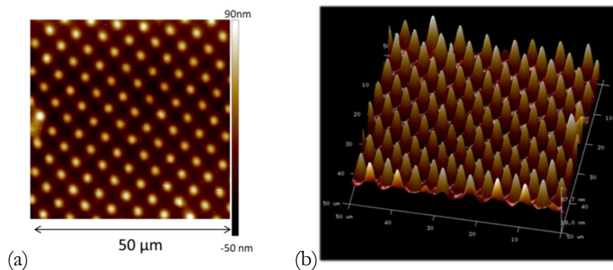
Figure V 9 Image topographique AFM dans l'air d'un réseau de plots de pNIPAM de 2 \mu\text{m} de diamètre (a) et sa représentation en trois dimensions (b).
