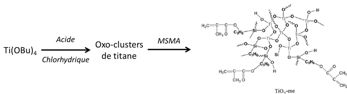
Figure IV 2 Synthèse de la solution de \text{TiO}_2\text{-MSMA} [83].
