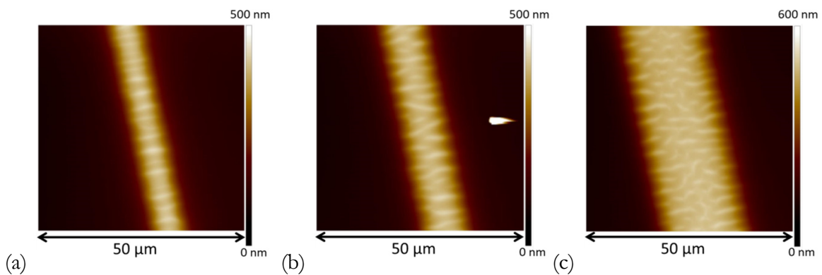
Figure V 15 Images AFM de lignes dans l'air à 20°C de largeur de 5 \mu\text{m} (a), 10 \mu\text{m} (b) et 20 \mu\text{m} (c).
