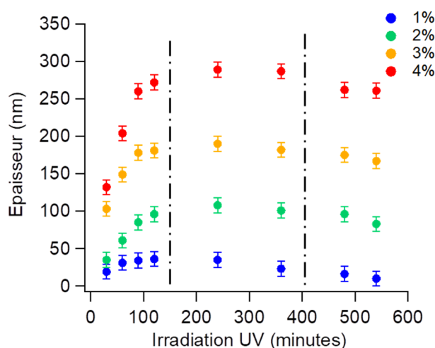
Figure II 12 Epaisseur du film d'hydrogel de pNIPAM obtenu en fonction du temps d'irradiation UV pour différentes concentrations de la solution de polymère déposée par spin-coating.
