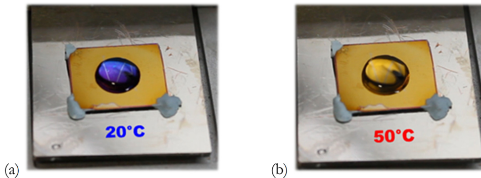
Figure III 5 Schémas des bicouches pNIPAM/Or sous la goutte d'eau (incolore) (a) à 20^{\circ}\text{C} : la goutte d'eau déposée gonfle l'hydrogel polymère dont l'épaisseur correspond alors à la teinte de Newton « bleue », la goutte apparaît bleue (b) à 50^{\circ}\text{C} : l'hydrogel polymère dégonfle et son épaisseur diminue et est inférieure à 200 nm, la goutte d'eau apparaît incolore.
