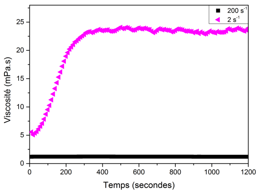
Figure 55 : Viscosité de la formulation AOT 5g/L, NaCl 2.8g/L en fonction du temps. La formulation est pré-cisaillée à 200\text{s}^{-1} durant 1200secondes. Ensuite soumise à un taux de cisaillement de 2\text{s}^{-1}
