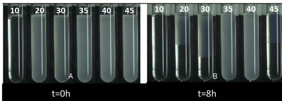
Figure 72 : Diagramme de phases du système SDBS 20g/L Isobutanol 6%v HPAM 3230s 2.5g/L pour différentes concentrations en NaCl (chiffres au-dessus des tubes) à t=0h et à t=8h .
