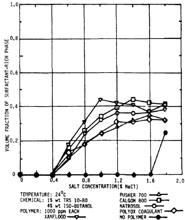
Figure 25 : Influence de la nature du polymère sur la CEC à T=24^{\circ} [5]. Les différentes courbes montrent que le % volumique de la phase démixée ne dépend pas de la nature du polymère mais de la salinité de la solution (Le % volumique de la phase démixée est de presque de 40% peu importe le polymère). Cependant, on remarque une différence en absence du polymère i.e. la démixtion de la formulation ne se produit qu'à partir d'une concentration en sel de 1.6% alors qu'elle est de 0.4% en présence des polymères.
