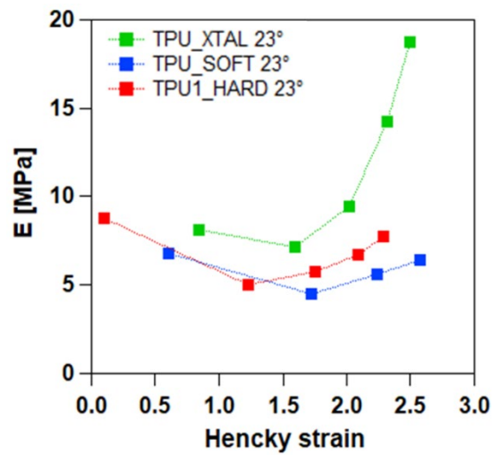
Figure 3 Young Modulus VS Hencky Strain pour les trois TPUs .
