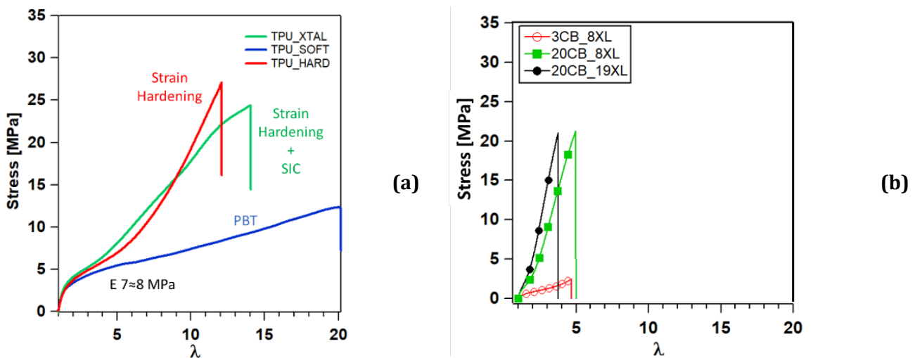
Figure 1 Réponse mécanique des trois TPU (a). Réponse mécanique des trois SBR(Mzabi, 2010)(b)
