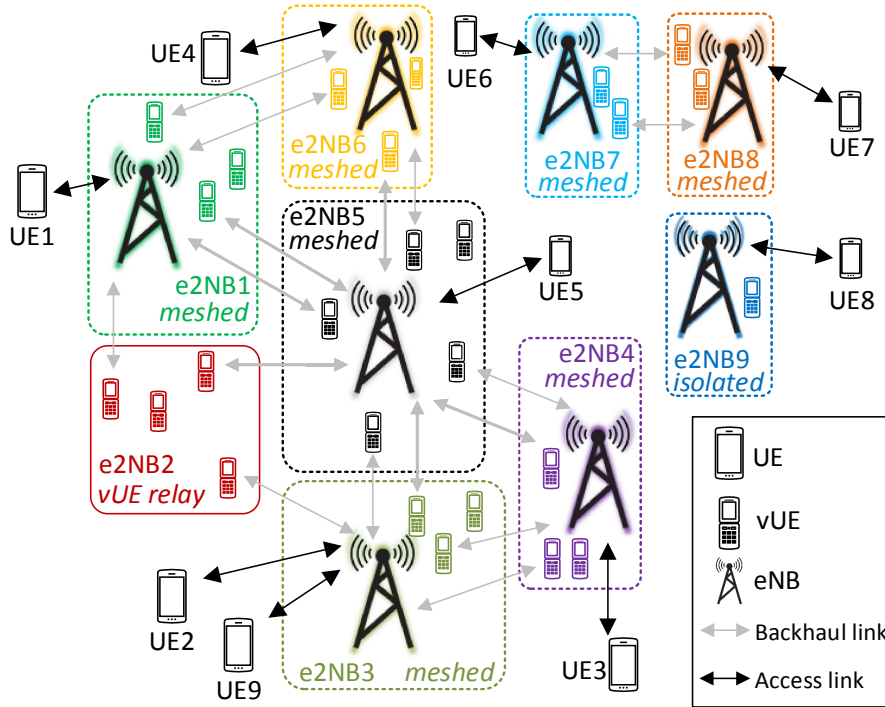
Figure 53 – Exemples de topologies réseaux obtenues grâce aux e2NBs.
