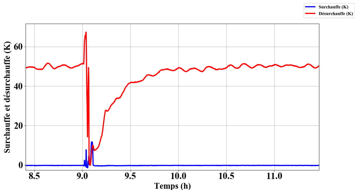
Figure 4.10 : Evolution de la surchauffe au refoulement (Désurchauffe) sur le point d'essai n°31.
