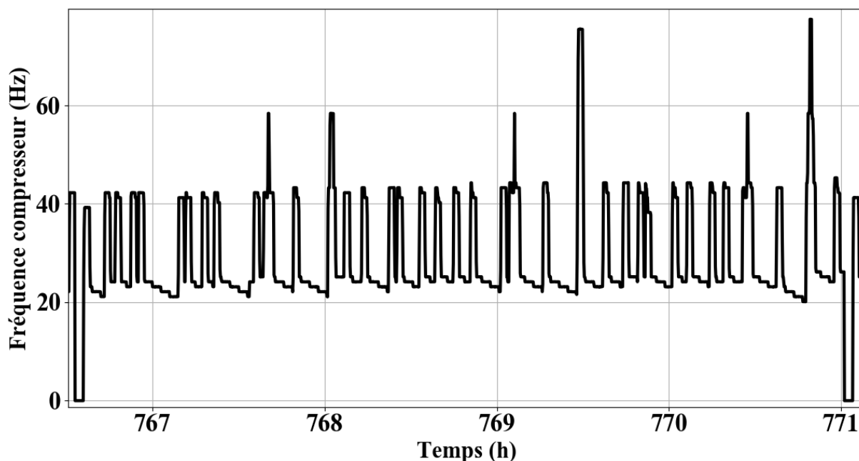
Figure 2.15 : Fréquence compresseur sur une séquence sans arrêt compresseur (MCbc)
