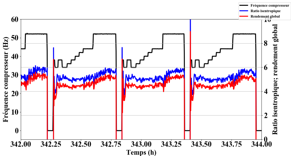
Figure 2.32 : Ratio isentropique, rendement global et puissance compresseur sur une séquence où les arrêts du compresseur sont fréquents (MME)
