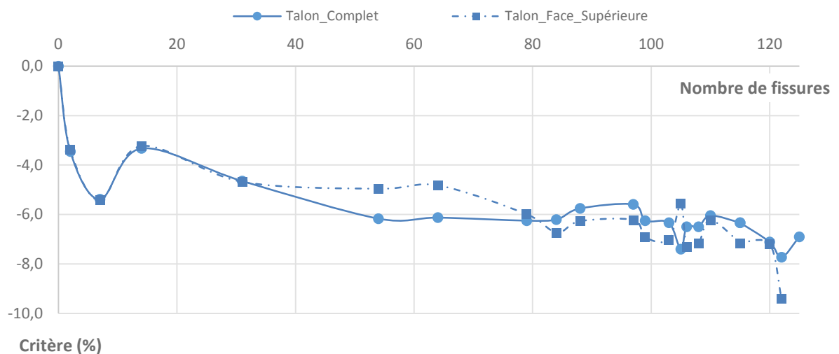
Figure 4.45 – Impact de l'encastrement (a) Talon Complet (b) Talon Face Supérieure, sur l'évolution du critère de santé numérique associé au couple de modes T3F4 de l'éprouvette numérique [0_3,90_3]_S n°2.
