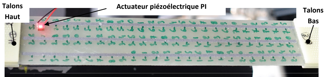
Figure 2.7 – Illustration de l'éprouvette [0_3, 90_3]_S équipée de son actuateur
