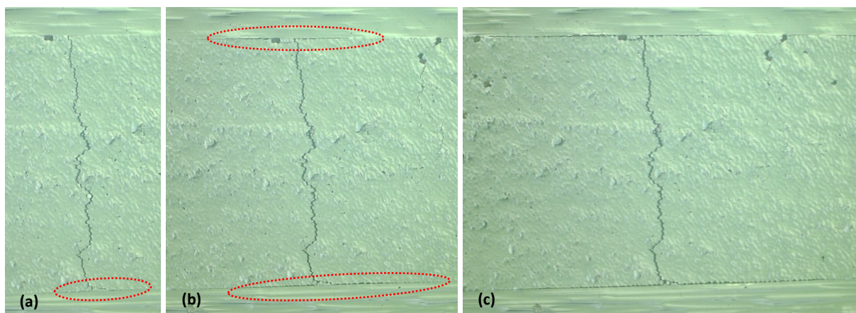
Figure 4.52 – Evolution du délaminage ( 90^\circ, 0^\circ ) en bord d'éprouvette à 0,75% (a), 1,29 % (b) et 1,89% (c) de déformation.
