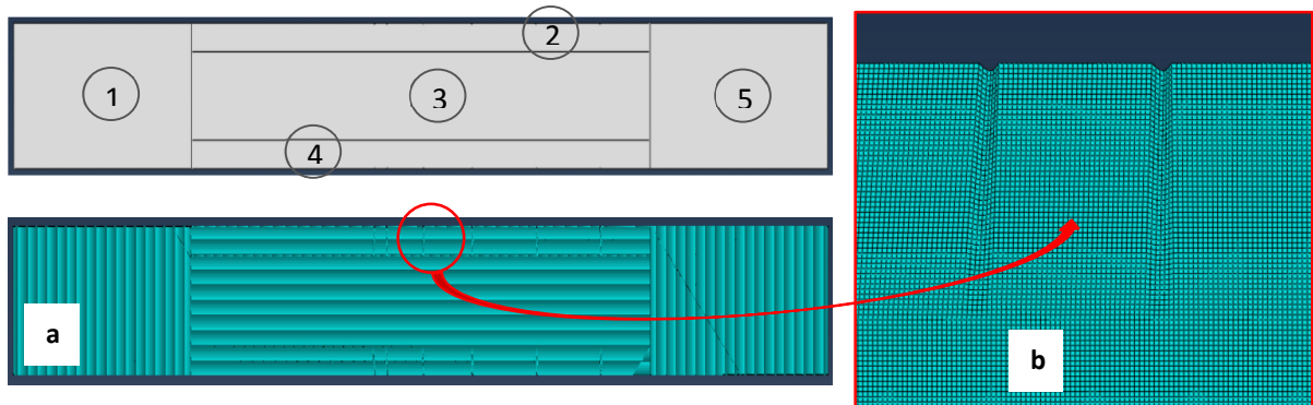
Figure 4.30 – Illustration du maillage progressif d'une interface (a), notamment à l'aplomb de chaque spline (b).
