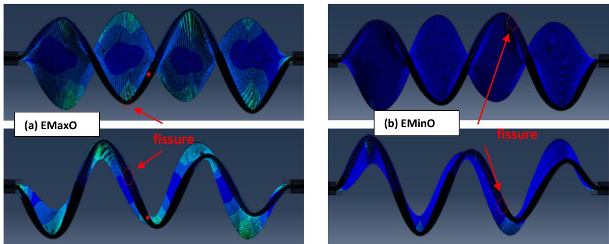
Figure 4.55 – Illustration de la position d'une fissure lorsque l'EMaxO est atteint (a) et lorsque l'EMinO est atteint (b), en fonction du CS_{NUM} représenté par le couple de modes T_4F_5 .
