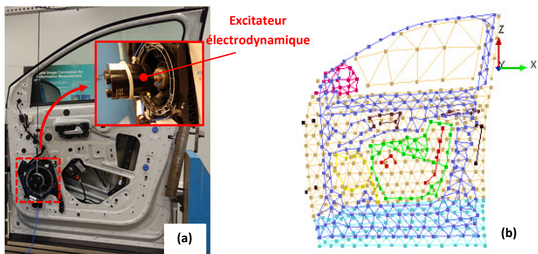
Figure 1.27 – Illustration de la problématique : Structure instrumentée (a) – Maillage expérimental dense associé (b).
