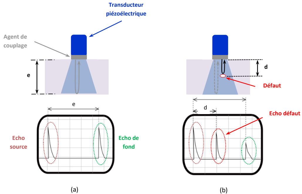
Figure 1.7 – Illustration du principe de détection d'un défaut dans un matériau sain (a) – présentant un défaut à une profondeur « d » (b) [3].
