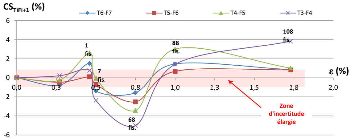
Figure 2.31 – Critère de santé mesuré sur éprouvette [0_3, 90_3]_S , avec fissuration transversale uniquement.
