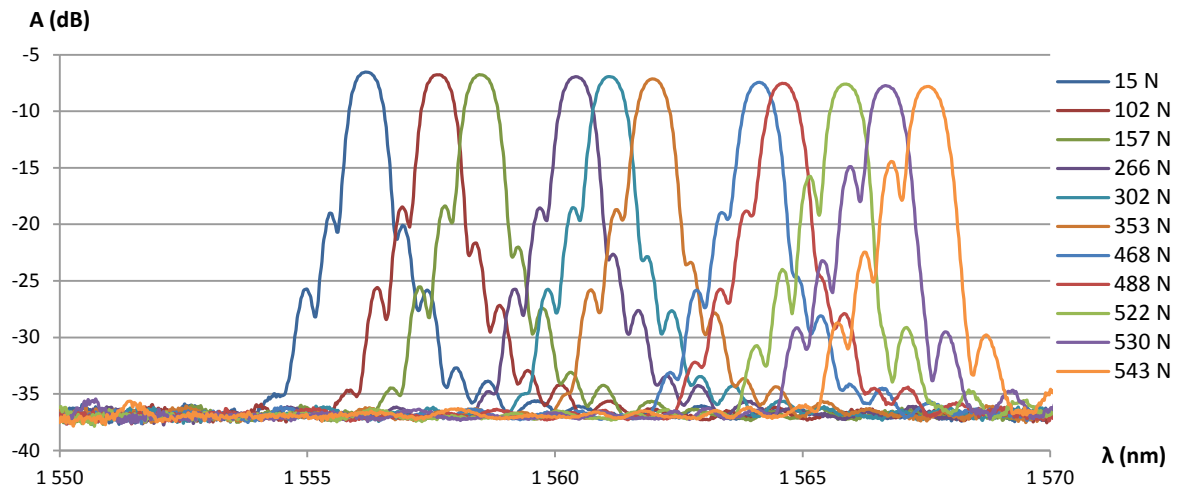
Figure 1.15 – Illustration de l'évolution spectrale d'un FBG uniforme en fonction du chargement appliqué et des dégradations.
