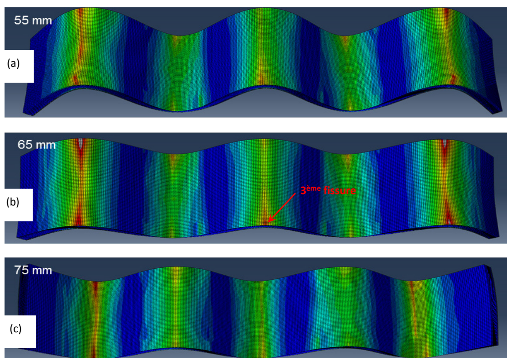
Figure 4.37 – Evolution des champs de contraintes de Von Mises, sur une échelle commune, en fonction des positions extrêmes (a), (c) et initiale (b) de la 3 ème fissure.
