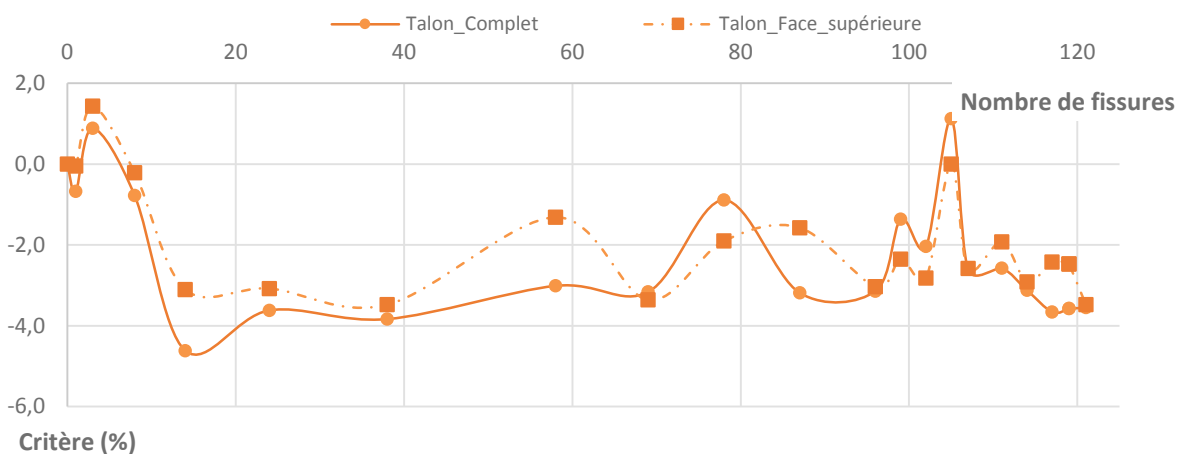
Figure 4.43 – Impact de l'encastrement (a) Talon Complet (b) Talon Face Supérieure, sur l'évolution du critère de santé numérique associé au couple de modes T_4F_5 de l'éprouvette numérique [0_3,90_3]_S n°1.
