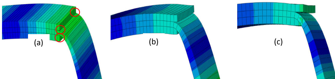
Figure 4.5 – Illustration du décollement des talons (a) aux 4 coins, (b) sur toute leur largeur avec un incrément de profondeur d'une maille, (c) puis de 2 mailles.
