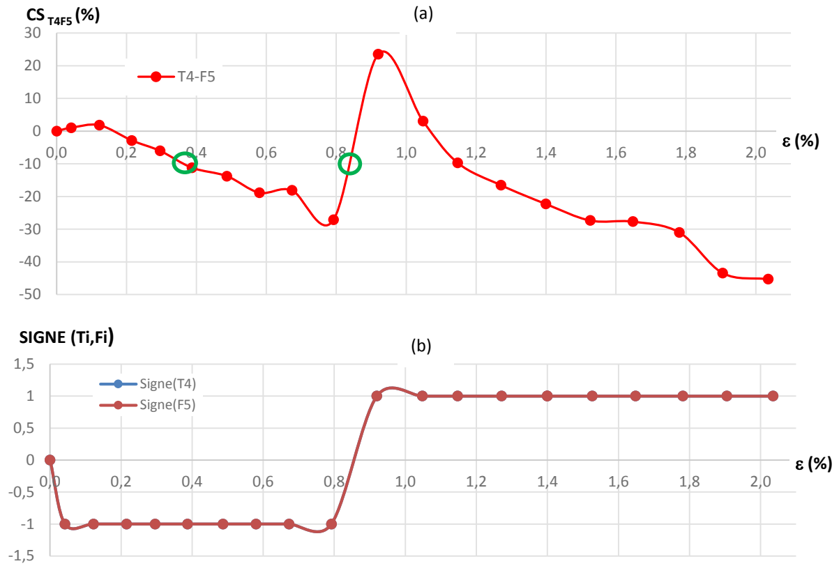
Figure 3.21 – Interprétation du critère de santé (a) à l'aide des fonctions « signe » des modes de torsion T4 et de flexion F5.(b).
