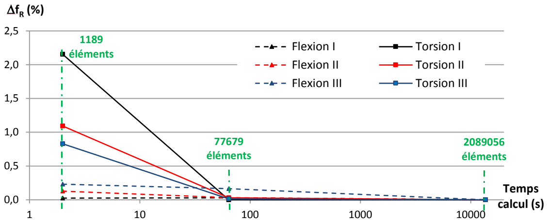
Figure 4.9 – Etude de convergence associée aux 3 premiers modes de flexion et de torsion.
