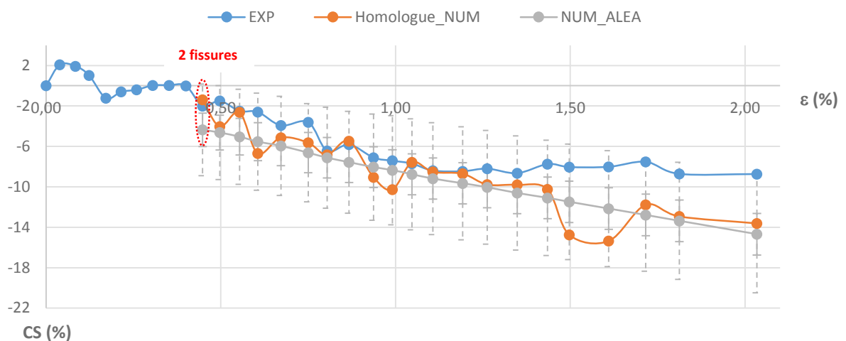
Figure 4.50 – Evolution des critères de santé numérique et physique T_4F_5 associés à l'éprouvette [0_3,90_3]_S n°2.
