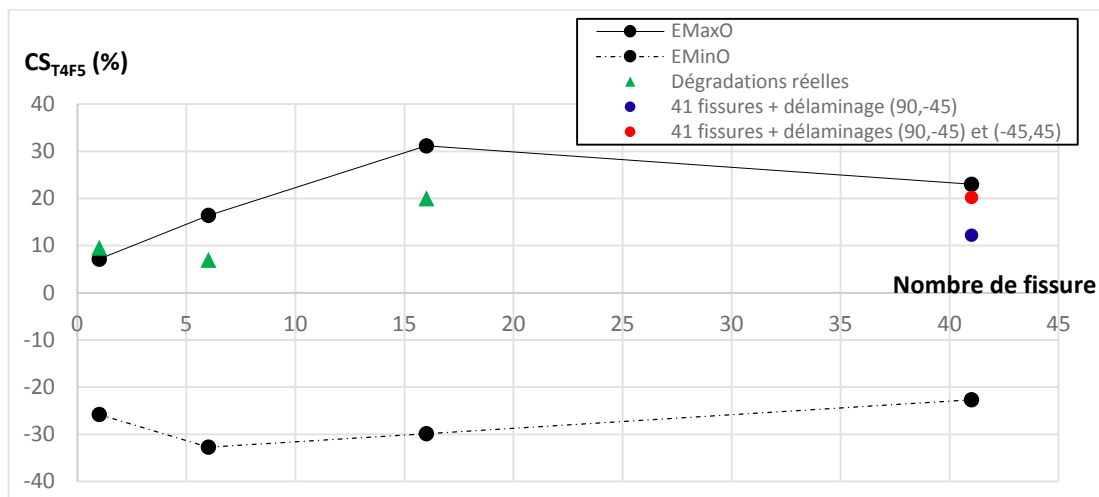
Figure 4.62 – Evolution du critère de santé associé au couple de modes T_4F_5 en fonction des délaminages (90,-45) et (-45,45).
