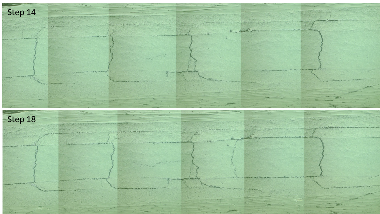
Figure 3.13 – Eprouvette [0_2,+45,-45,90_2]_S n°1 : expansion des mécanismes de dégradations du step 14 à \epsilon=1.47\% (a), jusqu'au step 18 à \epsilon=2.00\% , proche rupture (b).
