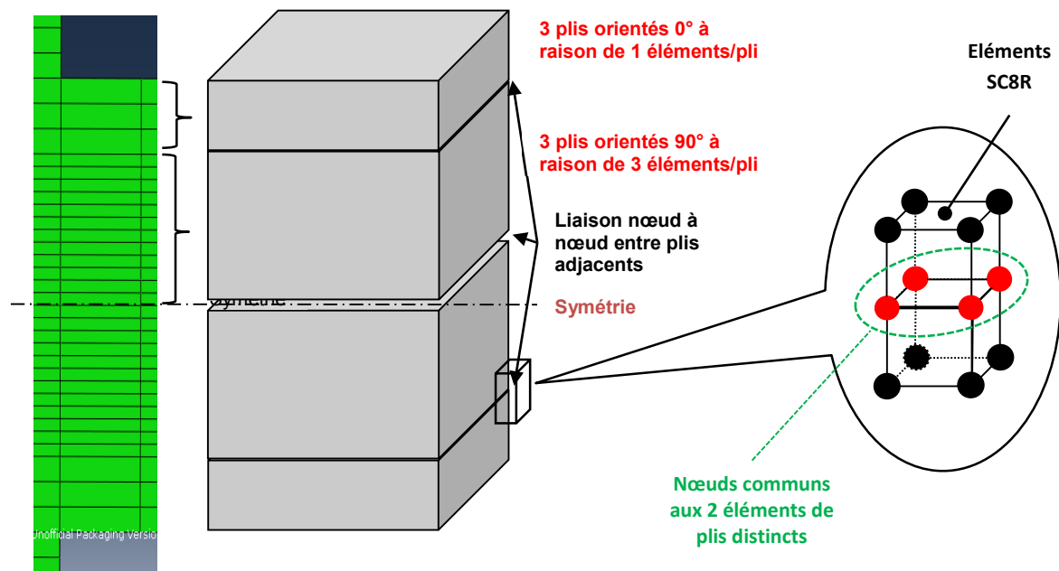
Figure 4.12 – Illustration du maillage associé aux éprouvettes numériques [03,903] S .
