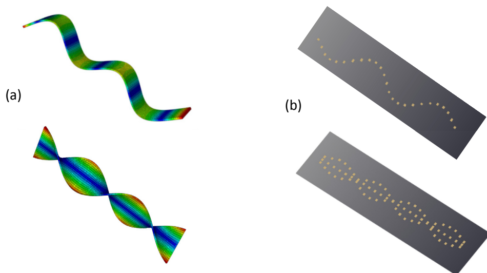
Figure 4.3 – Illustration de quelques déformées modales issues (a) de l'éprouvette numérique et (b) de l'éprouvette physique.
