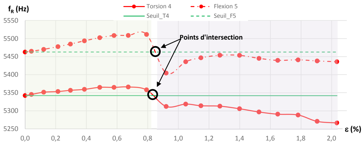
Figure 3.20 – Evolution monomode des modes de torsion T_4 et de flexion F_5 .
