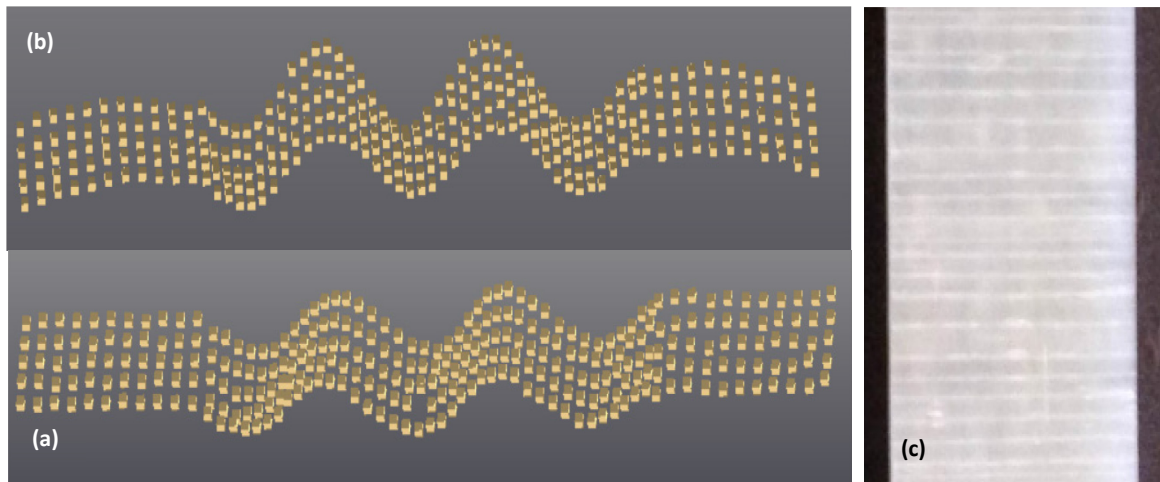
Figure 3.23 – Illustration des déformées modales associées au 5 ème mode de flexion, obtenues aux états (a) sain et (b) dégradée proche rupture (91 fissures transversales), à l'aide d'un maillage expérimental constitué de 300 points de mesure. L'intervalle interfissure est de l'ordre de 1.5 mm (c).
