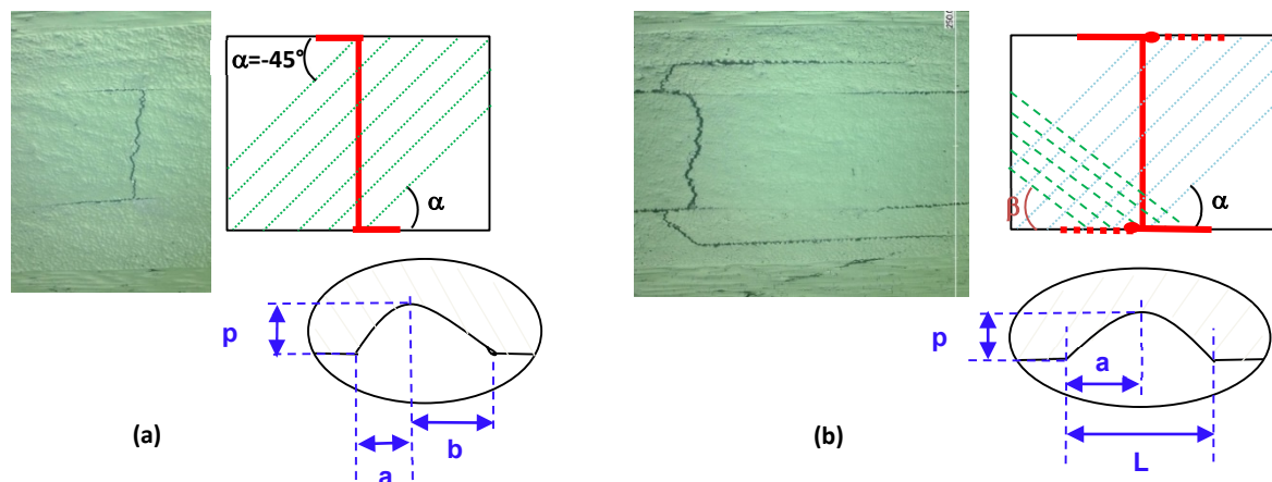
Figure 4.28 – Représentation du délaminage en bord d'éprouvette associé aux interfaces (a) (90, -45) et (b) (-45, 45) .
