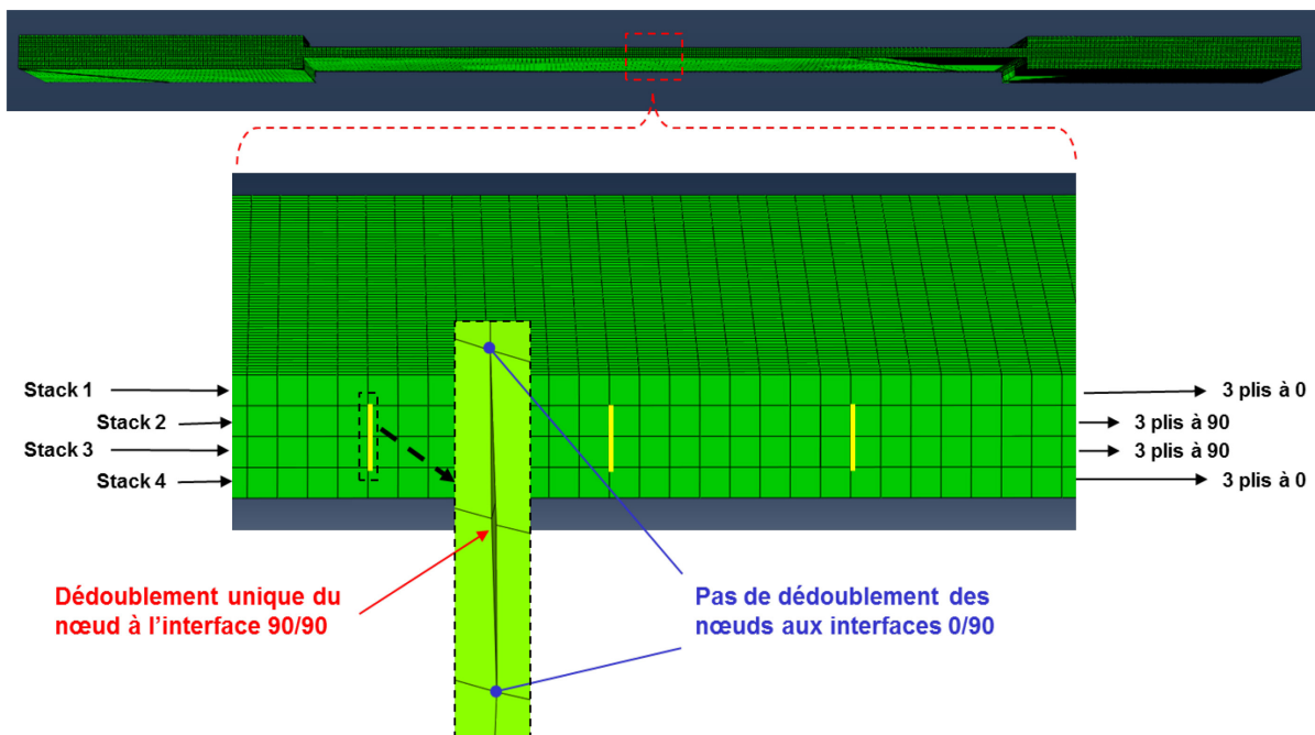
Figure 4.21 – Représentation des fissures transversales dans les plis orientés à 90°.
