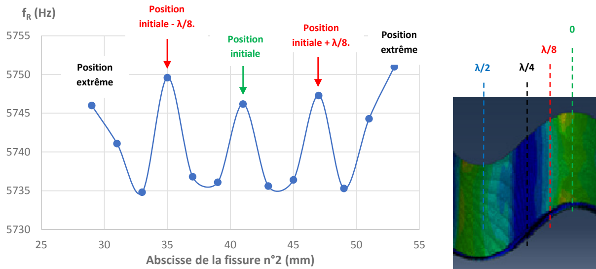
Figure 4.38 – Evolution de la f_R du 5ème mode de flexion en fonction du décalage simultané des 2ème, 3ème et 4ème fissures. Ce décalage est indexé par rapport à la position initiale de la 2ème fissure ( x_{f2}=41\text{mm} ).
