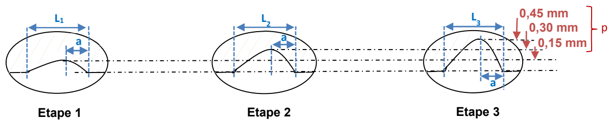
Figure 4.56 – Illustration de la progression du délaminage (90,-45) en bord d'éprouvette au regard des observations effectuées sur l'éprouvette physique [0_2,45,-45,90_2]_S .
