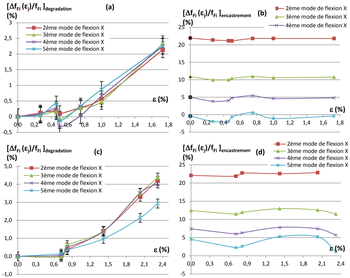
Figure 2.25 – Evolution des modes de flexion F2, F3, F4, F5 des éprouvettes [0, 90]_3S et [0, +45, -45, 90]_2S en fonction des dégradations uniquement (a)(c) et de l'encastrement uniquement (b)(d).
