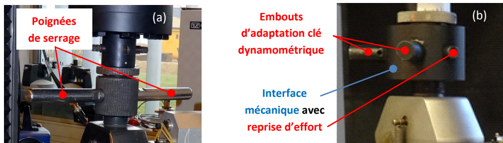
Figure 2.10 – Amélioration du mécanisme de serrage des mors. Systèmes de serrage (a) initial sans contrôle – (b) optimisé avec contrôle.
