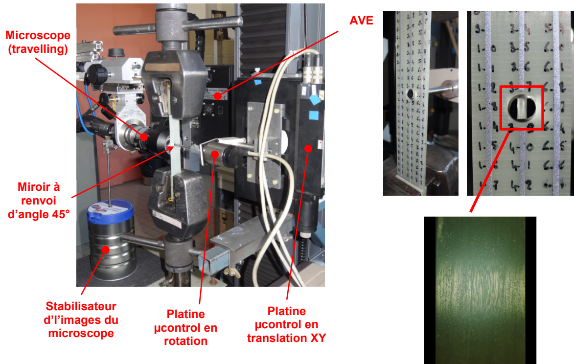
Figure A2-2 - Adaptation du montage expérimental initial pour une observation en rotation.
