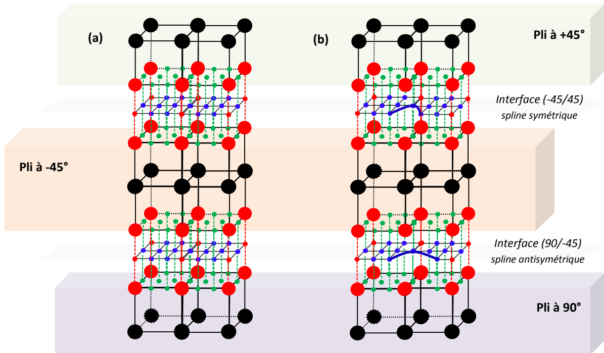
Figure 4.29 – Illustration de la mise en forme du délaminage en bord d'éprouvette [0_2,45,-45,90_2]_s , de l'état sain (a) à l'état fissuré (b).
