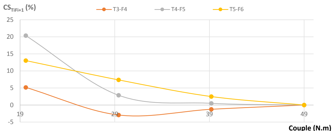
Figure 3.4 – Evolution du critère de santé, associé aux couples de mode T_3F_4 , T_4F_5 , T_5F_6 , en fonction du couple de serrage des mors.
