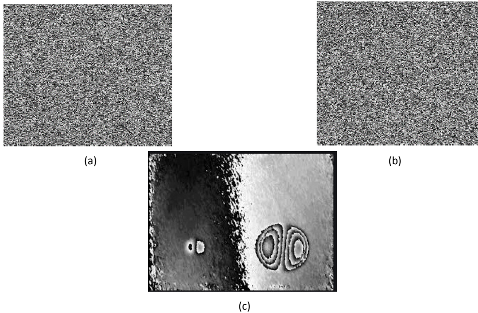
Figure 1.23 – Illustration d'une mesure de dérivée spatiale des déplacements hors plan par shearographie, dont la carte de phase (c) est obtenue en soustrayant l'état déformé (b) à l'état de référence (a) [44].
