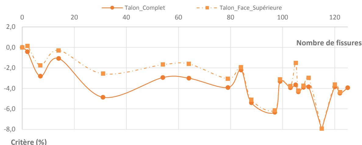
Figure 4.46 – Impact de l'encastrement (a) Talon Complet (b) Talon Face Supérieure, sur l'évolution du critère de santé numérique associé au couple de modes T4F5 de l'éprouvette numérique [0_3,90_3]_S n°2.
