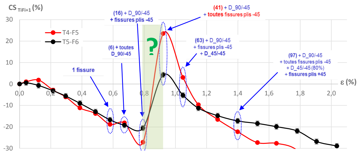
Figure 4.53 – illustration du CSPHYS des couples T_4F_5 et T_5F_6 associés au design d'éprouvette [0_2, 45, -45, 90_2]_s , au regard de multiples dégradations.
