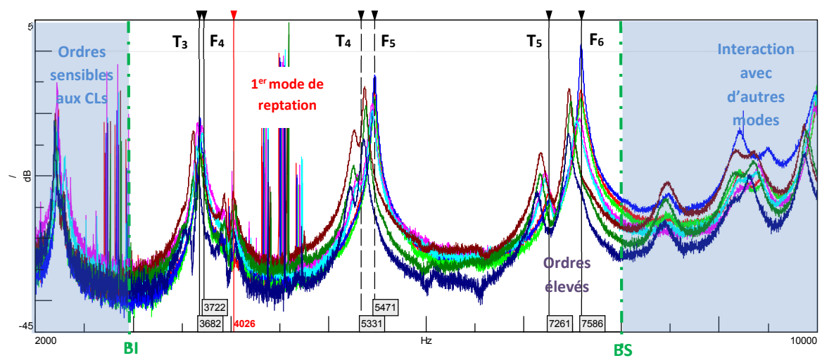
Figure 3.15 – Illustration du protocole de prétraitement des données, à partir des courbes représentatives de la moyenne des FRFs mesurées, à différents stades de dégradations, sur l'éprouvette [0_2,+45,-45,90_2]_s n°1.
