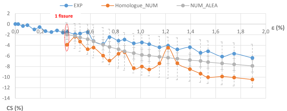
Figure 4.47 – Evolution des critères de santé numérique et physique T_3F_4 , associés à l'éprouvette [0_3, 90_3]_S n°1.
