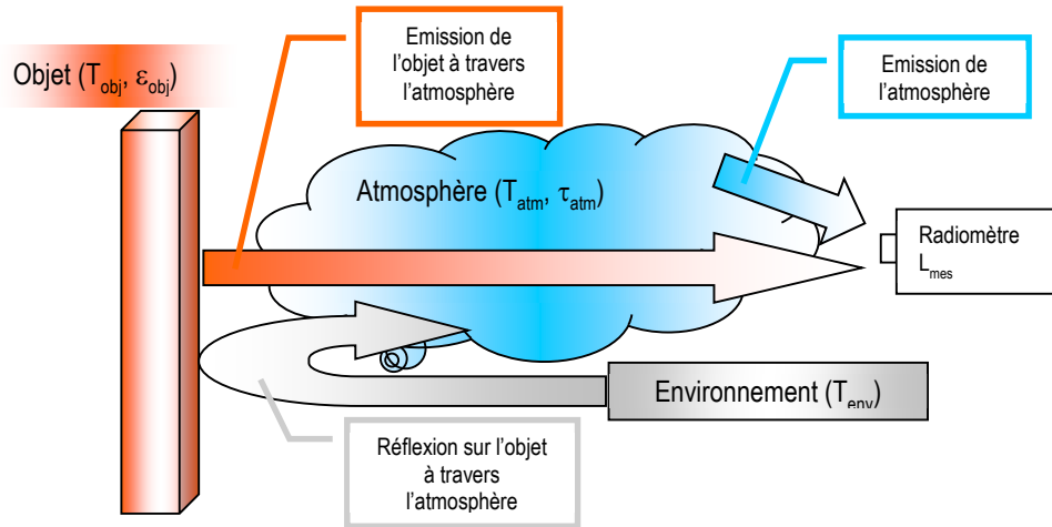
Figure 1.17 – Illustration de la situation de mesure par thermographie [25].
