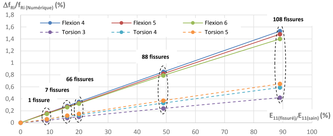
Figure 4.17 – Illustration de la chute du module d'élasticité E_{11} des plis orientés à 90^\circ de l'éprouvette numérique [0_3, 90_3]_s en fonction de la variation fréquentielle numérique de chaque mode aux différents stades de fissuration observés.
