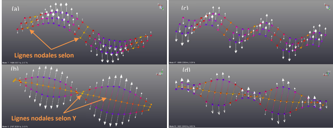
Figure 2.6 – Illustration des déformées modales associées aux (a) 2 ème mode de flexion – (b) 2 ème mode de torsion – (c) 6 ème mode de flexion – (d) 5 ème mode de torsion obtenues sur une éprouvette [0_3, 90_3]_S .
