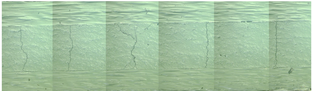
Figure 3.6 – Illustration du délaminage en bord d'éprouvette étendu à toutes les fissures transversales.
