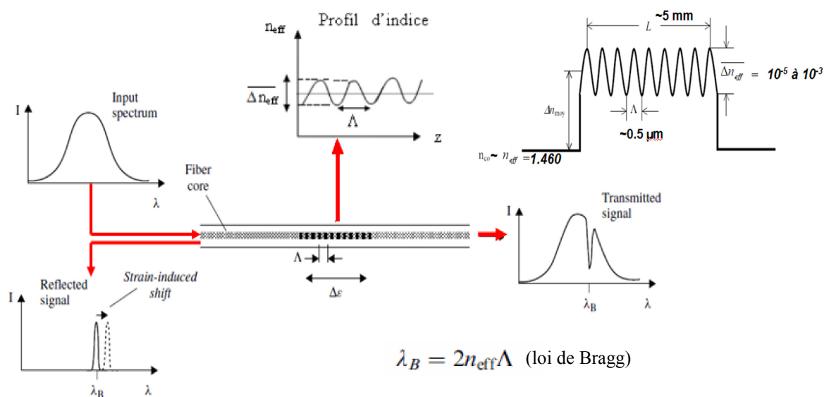
Figure 1.14 – Illustration du principe de mesure par fibre optique à réseau de Bragg.
