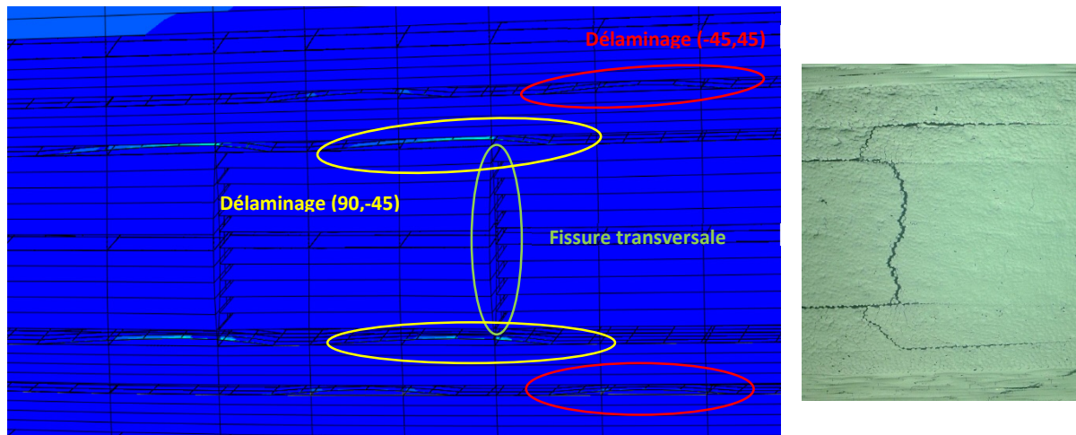
Figure 4.31 – Représentativité et capacité d'ouverture des fissures transversales et du délaminage en bord d'éprouvette [0_2, 45, -45, 90_2]_s aux interfaces (90, -45) et (-45, 45) .
