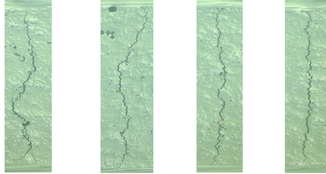
Figure 4.20 – Illustration du profil de quelques fissures transversales observables sur une éprouvette [0_3, 90_3]_S .
