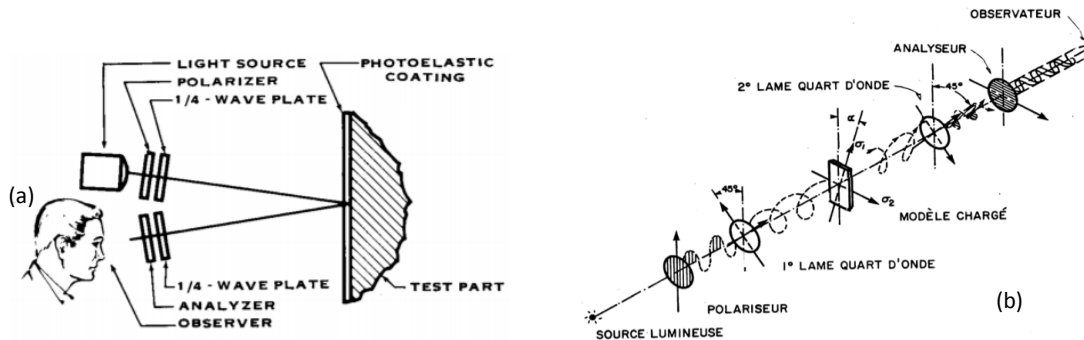
Figure 1.20 – Illustration du contrôle par photoélasticimétrie en réflexion (a), à l'aide d'un polariscope circulaire (principe de fonctionnement) (b) [39].
