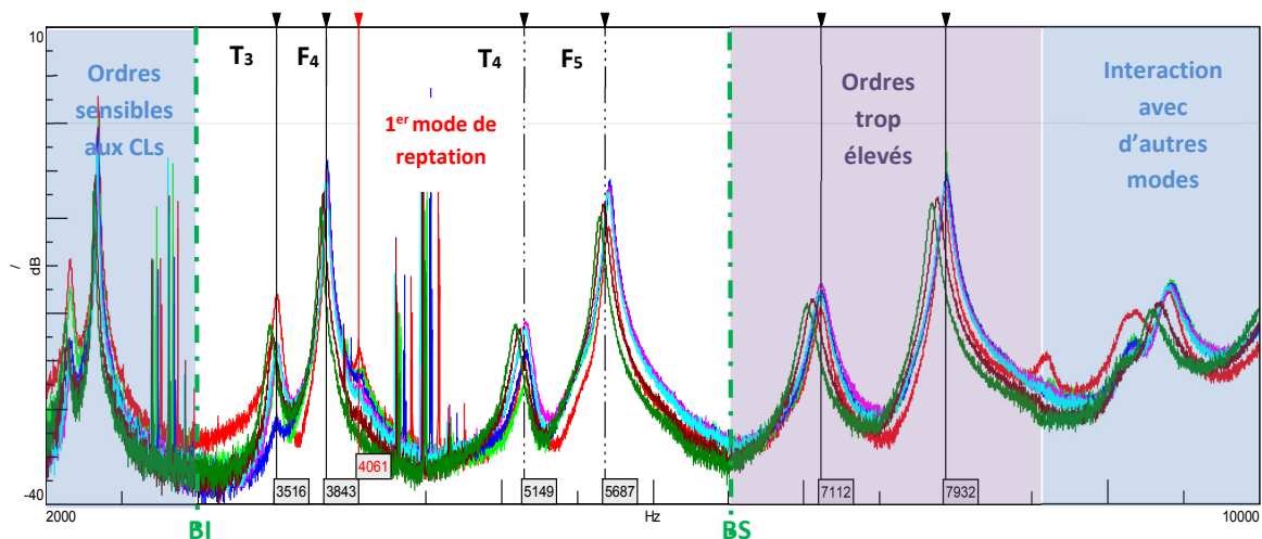
Figure 3.7 – Illustration du protocole de prétraitement des données, à partir des courbes représentatives de la moyenne des FRFs mesurées, à différents stades de dégradations, sur l'éprouvette [0_3, 90_3]_S n°1.
