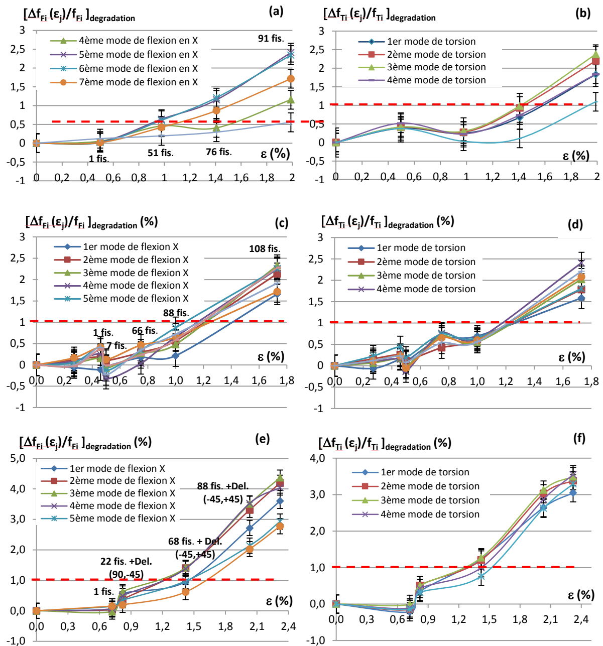
Figure 2.28 – Evolution des modes de flexion (F1 à F6) et de torsion (T1 à T5) pour les éprouvettes [0,90]_s (a), (b), [0,90]_s (c) (d), et [0,45,-45,90]_s (e) (f) en fonction des déformations.
