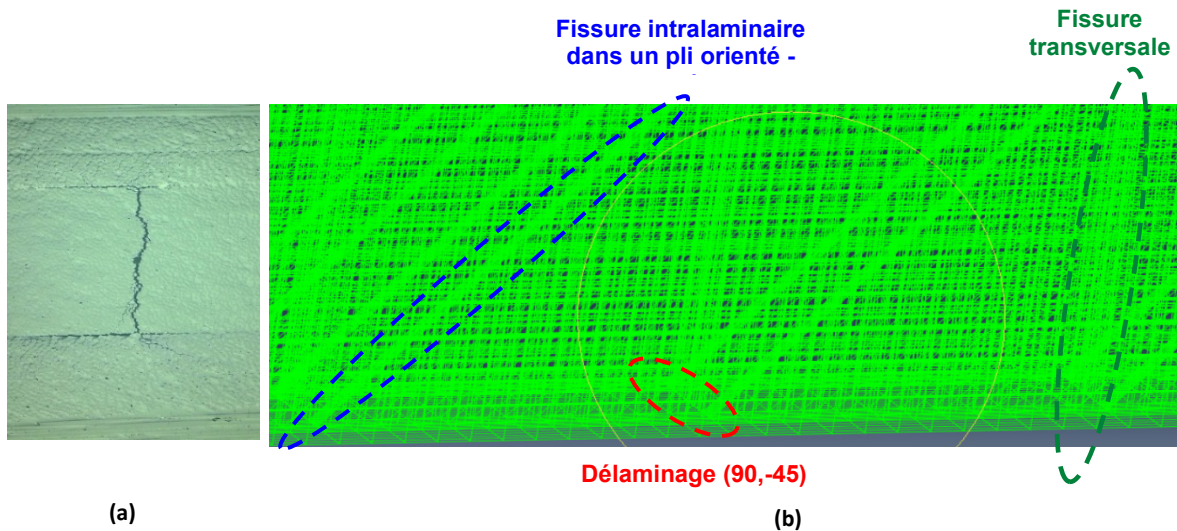
Figure 4.59 – Illustration de l'intégration des fissures intralaminaires dans les plis à -45^\circ (b), au regard des observations (a) faites sur l'éprouvette physique.
