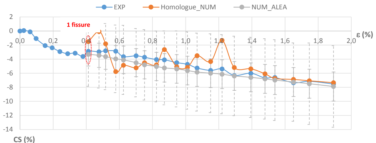
Figure 4.48 – Evolution des critères de santé numérique et physique T_4F_5 , associés à l'éprouvette [0_3,90_3]_S n°1
