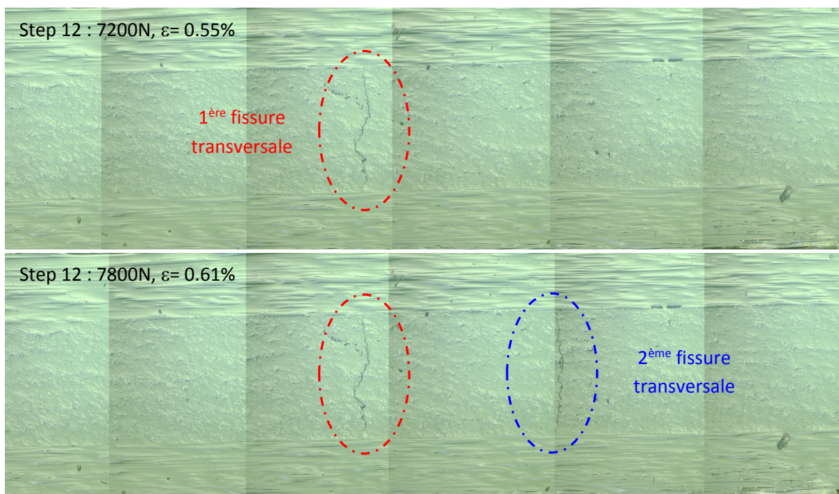
Figure 3.4 – Eprouvettes [0_3, 90_3]_S n°2 : illustration du caractère quasi-instantané lié à l'apparition d'une fissure intralaminare.
