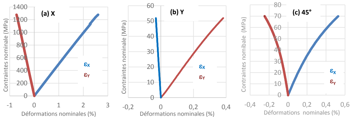
Figure 1.33 – Courbes de réponse macroscopique dans le repère (X, Y, Z) de l'éprouvette. Les renforts sont alignés suivant l'axe X (a), l'axe Y (b) et à 45° de l'axe X de l'éprouvette.
