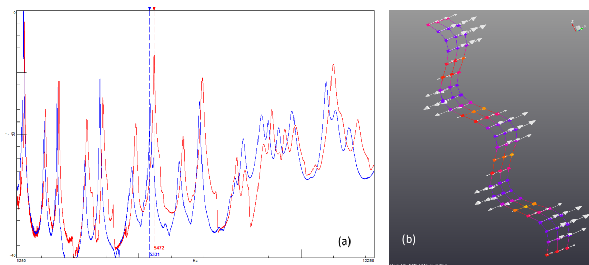
Figure 2.30 – (a) Illustration de l'évolution du comportement modal d'une éprouvette [0_3,90_3]_s de l'état sain (rouge) jusqu'à un stade d'endommagement proche rupture (bleu). (b) illustration de la déformée modale du 5ème mode de flexion.
