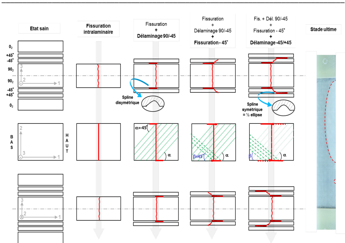
Figure 4.27 – Retranscription de la cinématique de dégradation à partir des observations réalisées simultanément sur les bords d'une éprouvette [0_2, 45, -45, 90_2]_s .
