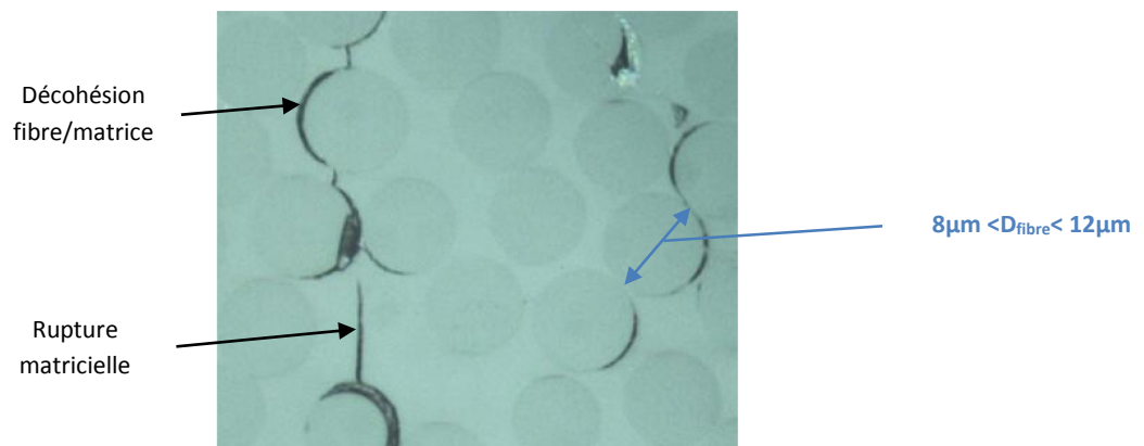
Figure 1.3 – Initiation des mécanismes de rupture élémentaires : décohésion fibre-matrice et rupture matricielle.
