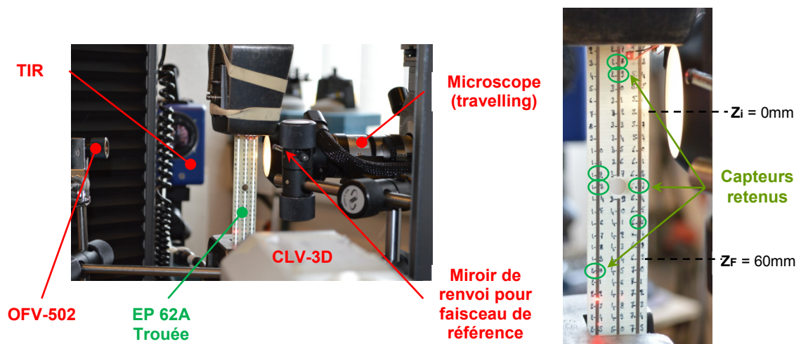
Figure A2-3 - Observation des dégradations sur la tranche de l'éprouvette.
