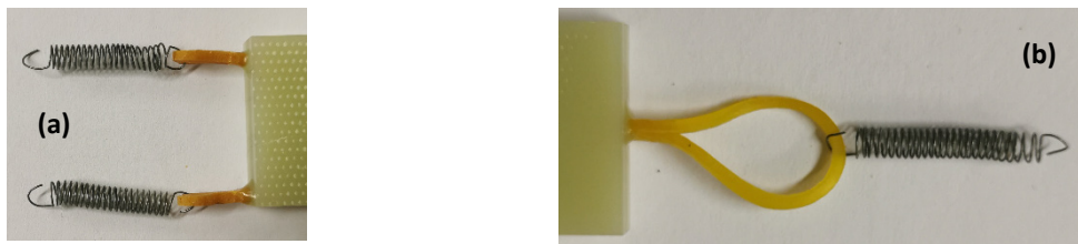
Figure 2.2 – Illustration de la liaison série « ressort – élastique ». Partie haute (a) – Partie basse (b).
