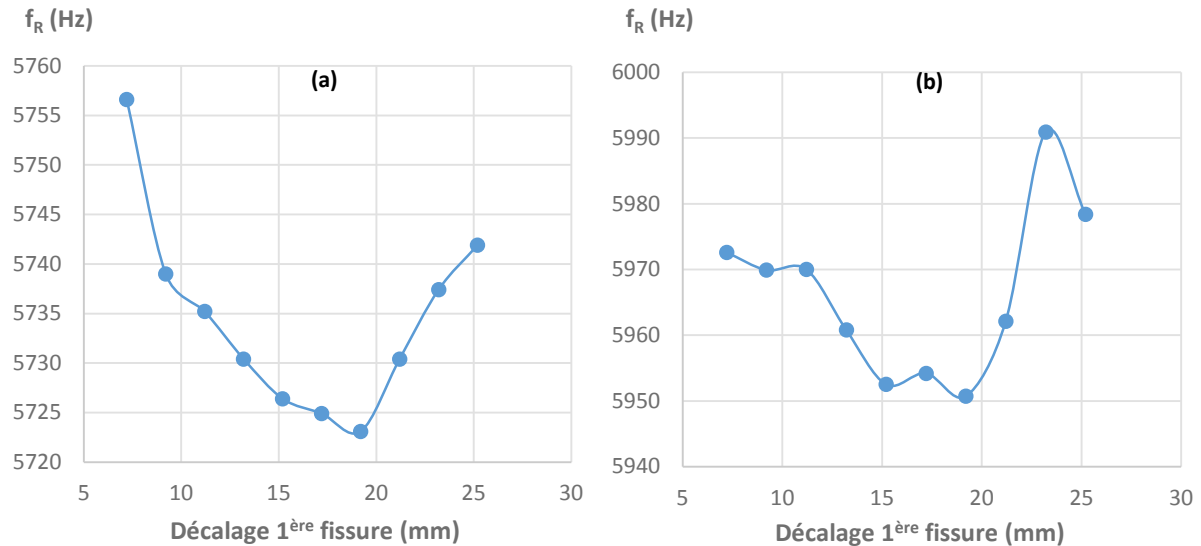
Figure 4.35 – Evolution de la f_R des 5èmes modes de flexion (a) et de torsion (b) en fonction de l'incrément de décalage des 7 fissures.
