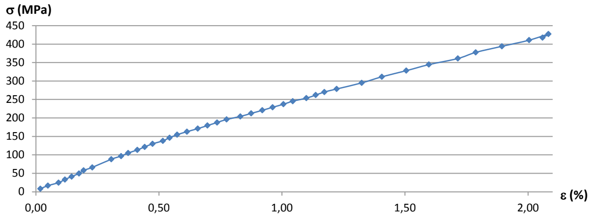
Figure 2.12 – Discrétisation accrue de la courbe contraintes/déformations.
