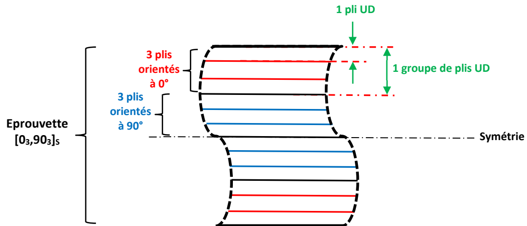
Figure 4.10 – Illustration d'un groupe de plis UD associé au design d'éprouvette [0_3,90_3]_s .
