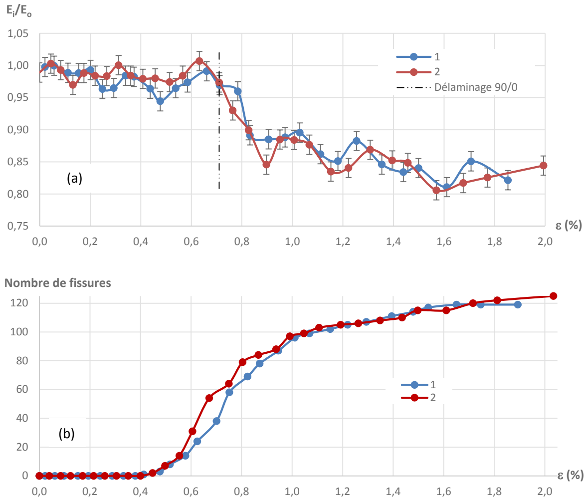
Figure 3.2 – Evolution du module apparent (a) et du nombre de fissures (b) au cours de la sollicitation pour 2 éprouvettes [0_x, 90_x]_s .
