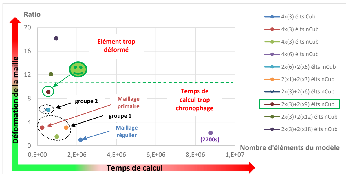
Figure 4.11 – Etude de convergence associée à la fissuration intralaminare.
