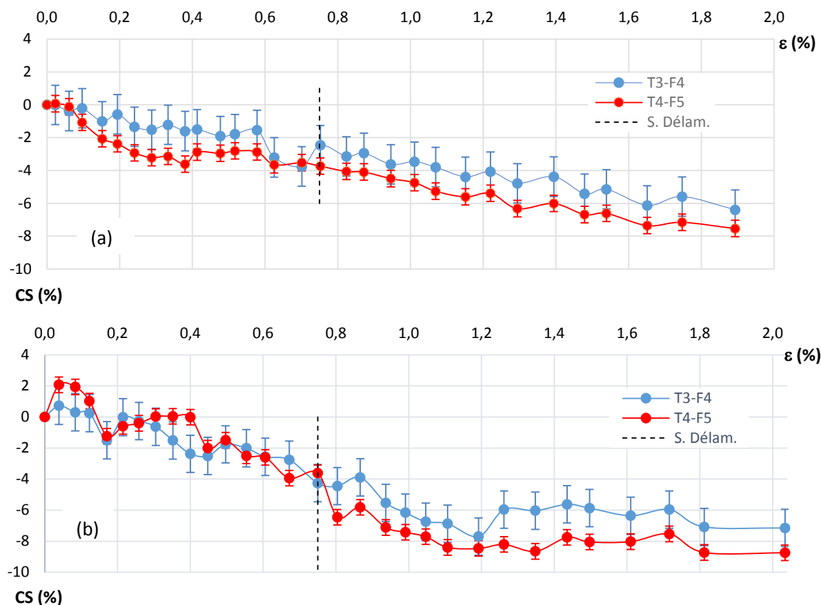
Figure 3.9 – Evolution du critère de santé associé à l'éprouvette 1 (a) et à l'éprouvette 2 (b) : [0_3, 90_3]_s .
