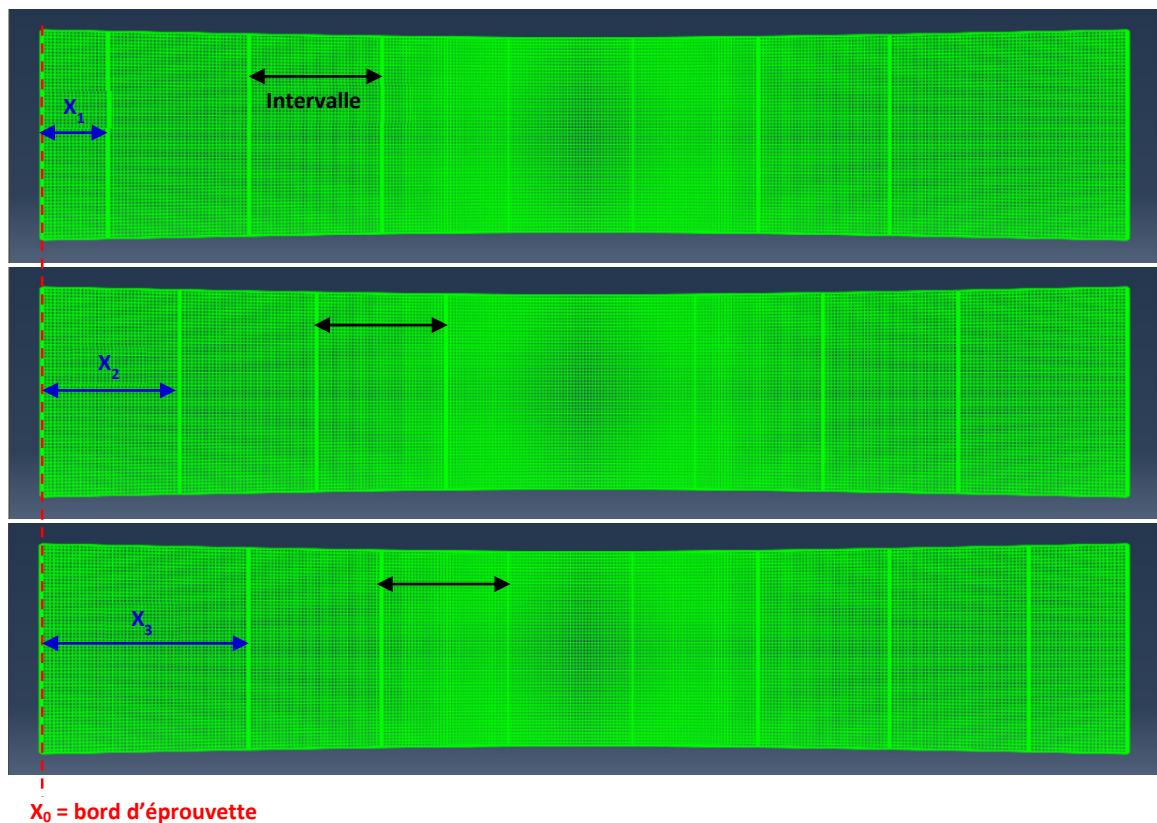
Figure 4.34 – Illustration du principe du décalage simultané des fissures.
