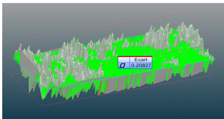
Figure 2.23 – Etat de surface d’une éprouvette réalisé avec une MMT.
