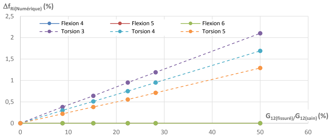
Figure 4.18 – Illustration de la chute du module de cisaillement G_{12} des plis orientés à 90^\circ de l'éprouvette numérique [0_3, 90_3]_s en fonction de la variation fréquentielle de chaque mode aux différents stades de fissuration observés.
