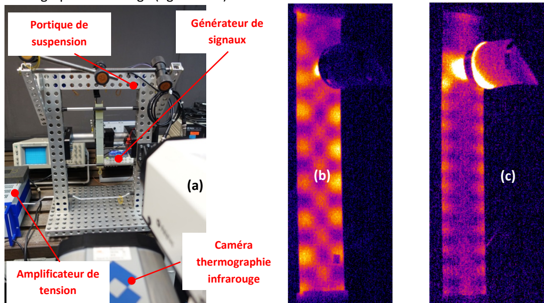
Figure 3.27 – Observation de la déformée modale du mode A_0 au travers de la caméra de TIR (a). Illustration des modes de Lamb antisymétriques A_0 (b) et A_1 (c).
