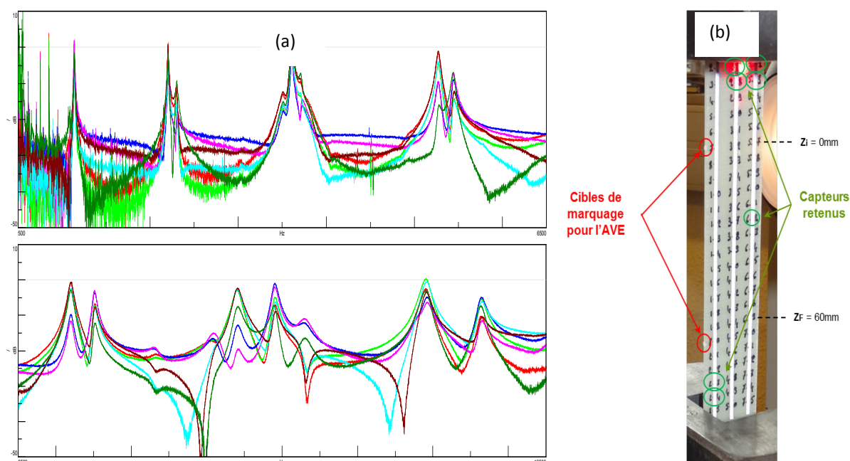
Figure 2.27 – Illustration des FRF (a) associées aux 6 points de mesure retenus (b) selon la direction X (fibres orientées 0^\circ ).
