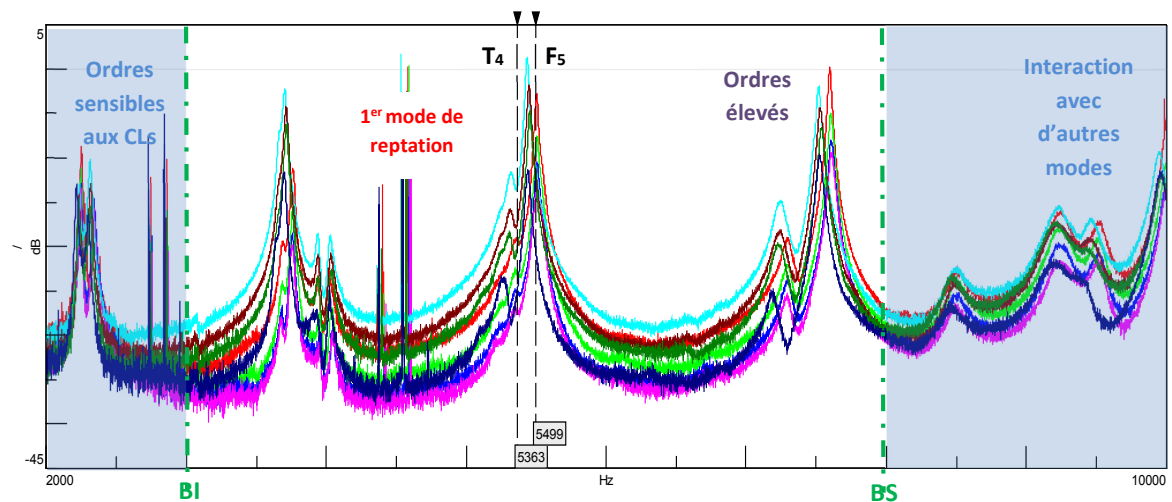
Figure 3.16 – Illustration du protocole de prétraitement des données, à partir des courbes représentatives de la moyenne des FRFs mesurées, à différents stades de dégradations, sur l'éprouvette [0_2,+45,-45,90_2]_s n°2.
