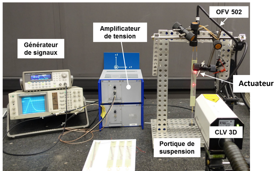
Figure 2.4 – Illustration du banc de caractérisation vibratoire.
