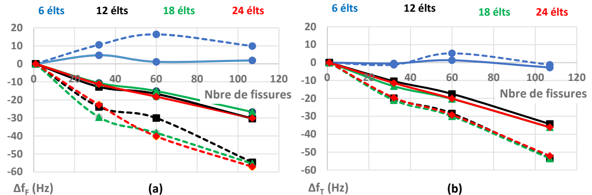
Figure 4.24 – Evolution des fréquences de résonance associées aux modes F_4 (trait plein) et F_5 (trait pointillé) (a) - puis T_3 (trait plein) et T_4 (trait pointillé) (b) selon 4 états fissurés, en fonction du nombre d'éléments présents dans l'épaisseur des plis à 90^\circ .
