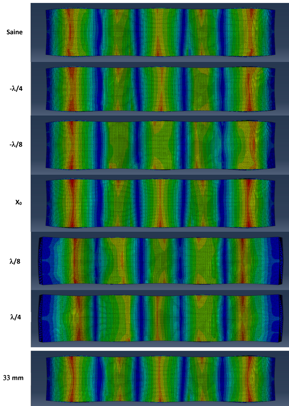
Figure 4.39 – Evolution des champs de contraintes de Von Mises, sur une échelle commune, en fonction du décalage simultané des 2ème, 3ème et 4ème fissures aux positions -\lambda/4 , -\lambda/8 , \lambda/8 , \lambda/4 et x=33 mm.
