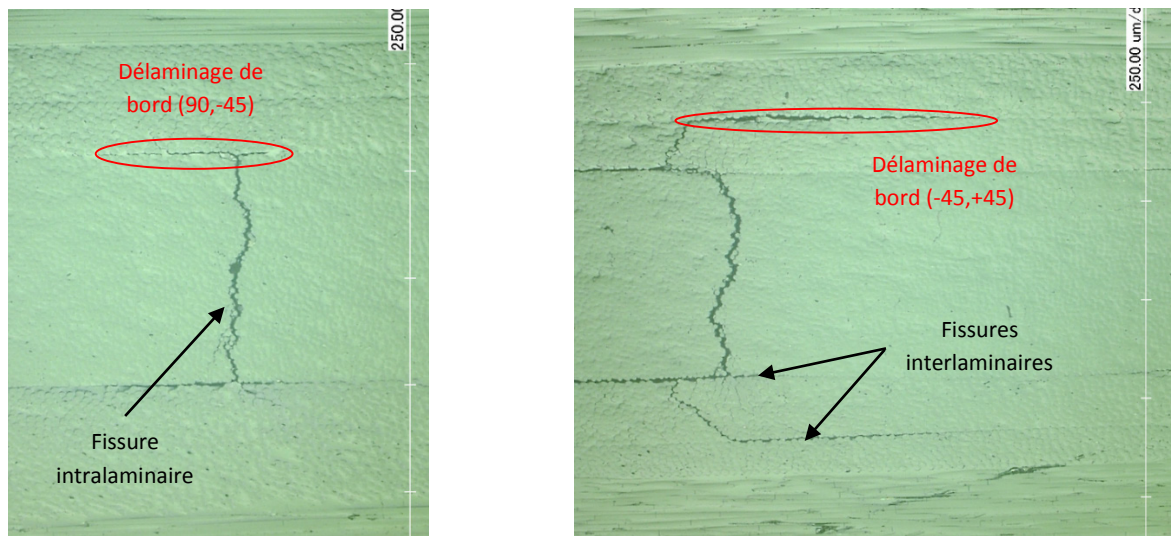
Figure 1.5 – Illustration des mécanismes de rupture macroscopique associés au délaminage entre les interfaces 90^\circ/-45^\circ (a), puis à la fissuration interlaminaire et au délaminage entre les interfaces -45^\circ/+45^\circ (b).
