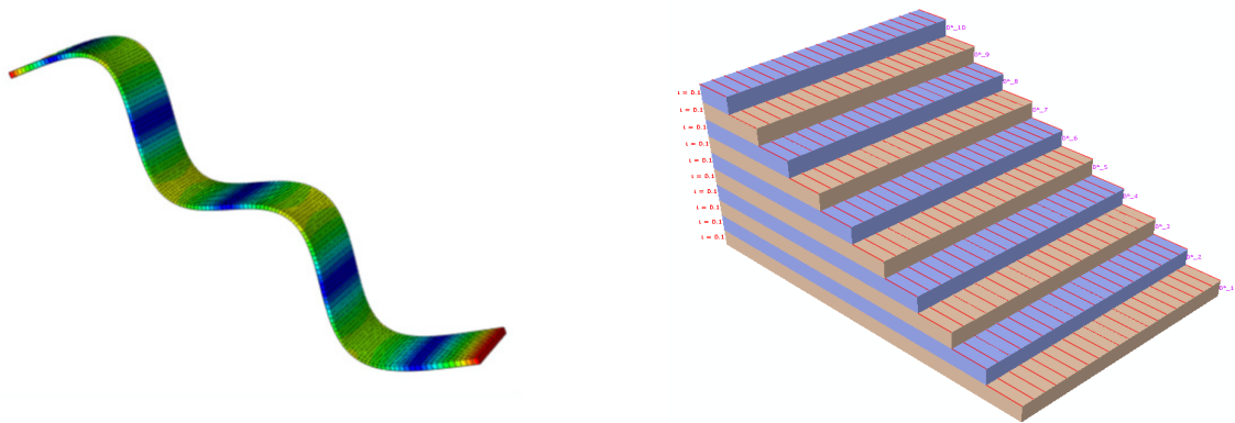
Figure 4.2 – Illustration de l'éprouvette numérique UD10, représentée sous la forme d'un stack de 10 plis (1S).
