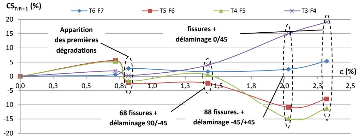
Figure 2.32 – Critère de santé mesuré sur éprouvette [0_2, 45, -45, 90_2]_s , associé à la fissuration transversale et aux délaminages (90,-45) et (-45/+45).
