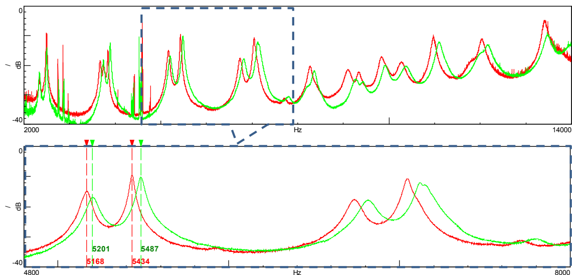
- Figure A2-1 - Comparaison de FRF entre éprouvette trouée (rouge) / non trouée (verte).
