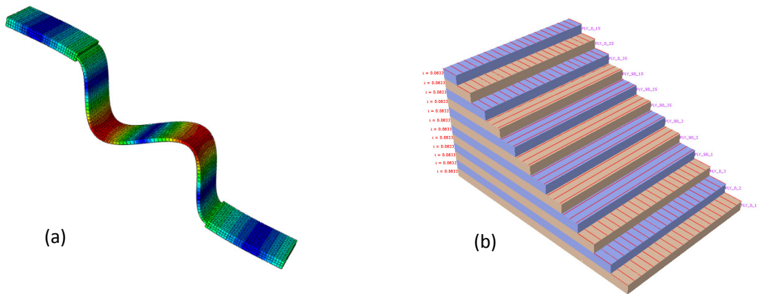
Figure 4.4 – (a) Illustration de l'éprouvette numérique [0_3,90_3]_S « complète » et (b) de sa représentation sous la forme d'un empilement constitué de 12 plis, avec un comportement homogénéisé.
