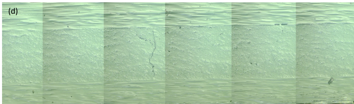
Figure 3.3 – Eprouvettes [0_3, 90_3]_S n°2 : De l'apparition au step 8 à \epsilon=0.35\% (b), jusqu'à la propagation de la première fissure transversale, aux steps de chargement 10 à \epsilon=0.45\% (c) et 11 à \epsilon=0.50\% (d).
