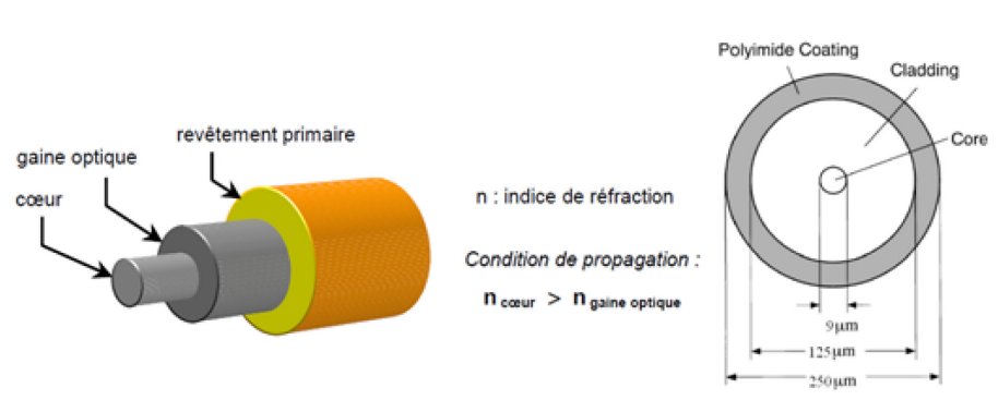
Figure 1.13 – Illustration des constituants d'une fibre optique [17].
