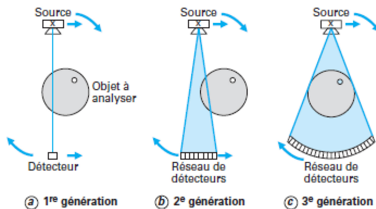
Figure 1.11 – Illustration des capteurs de 1ère, 2ème et 3ème génération [11].
