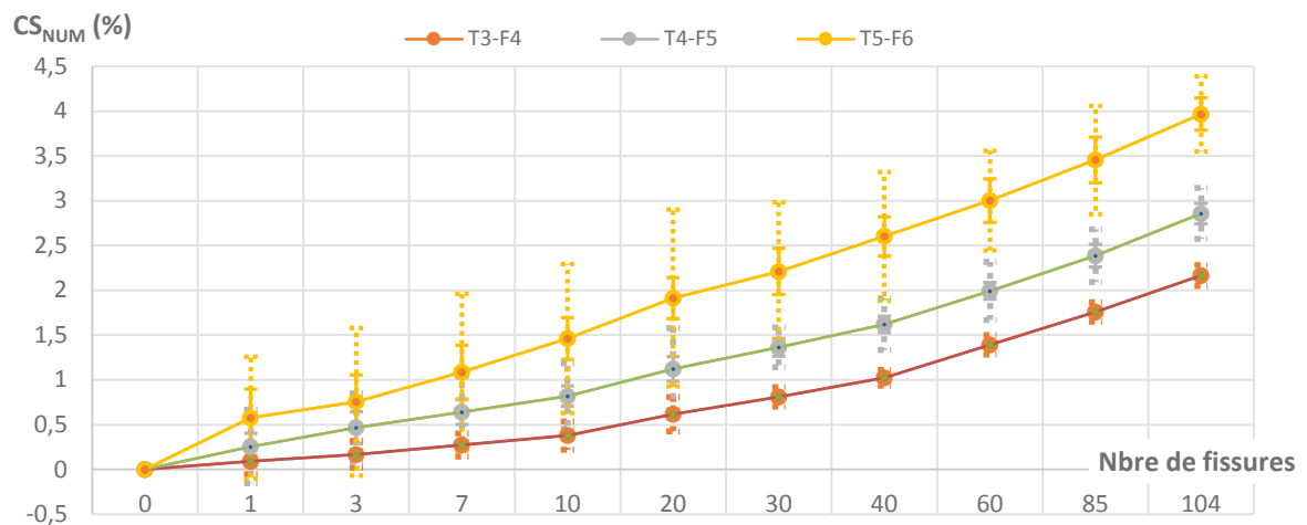
Figure 4.40 – Illustration de la dispersion du critère de santé numérique en fonction du nombre de fissures présentes dans l'éprouvette. L'écart type est représenté par des barres d'erreur en trait plein alors que les valeurs extrêmes sont représentées par des barres d'erreur en trait pointillé.
