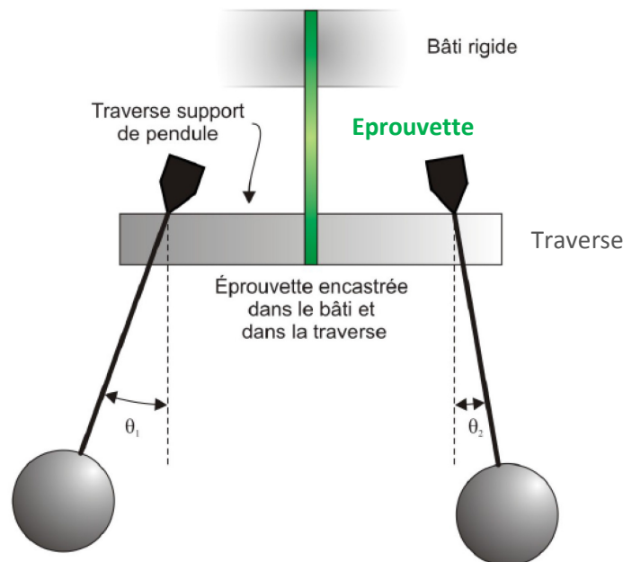
Figure 1.34 – Montage illustrant les « pendules sympathiques » [68].
