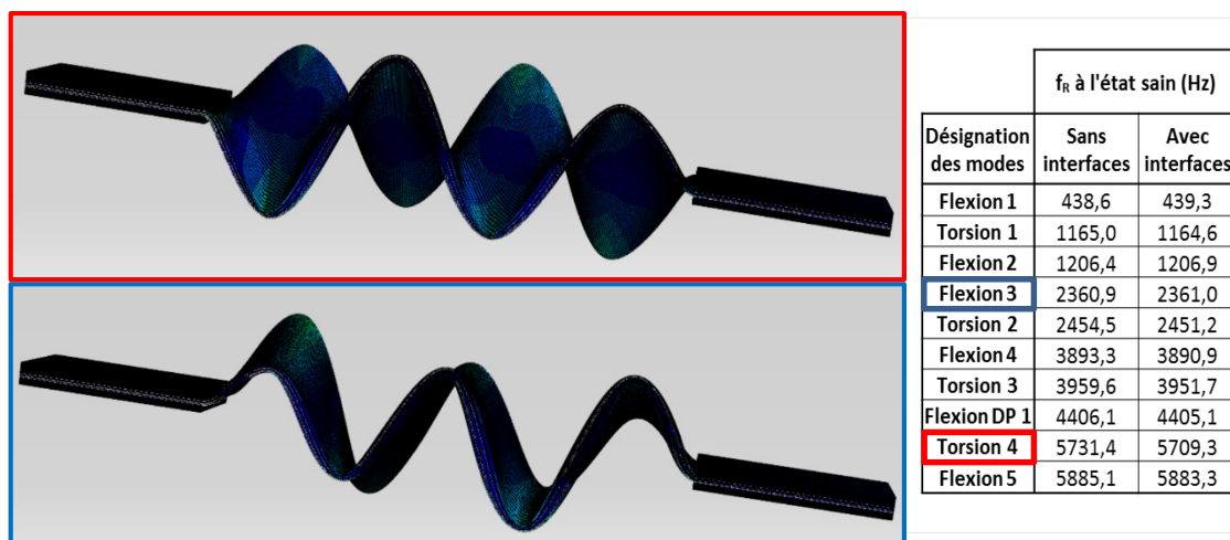
Figure 4.16 – Cohérence du comportement modal de l'éprouvette [0_2,45,-45,90_2]_s . avec et sans interface.
