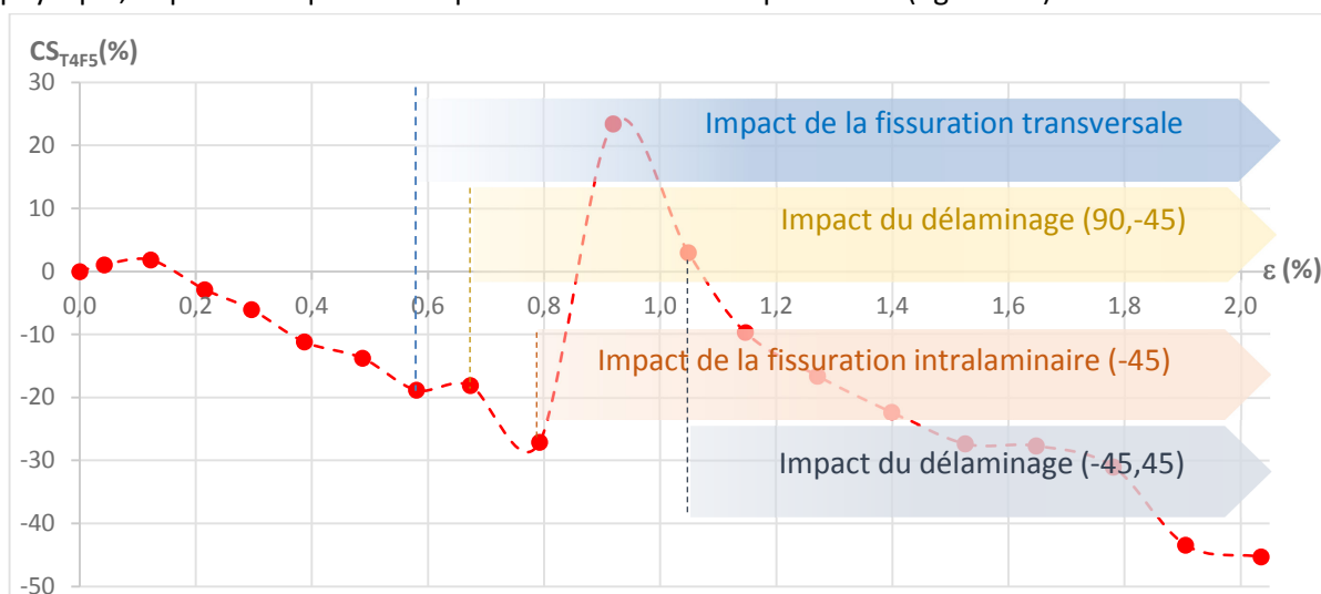
Figure 4.1 – Hypothèses émises à partir d'observations effectuées sur une éprouvette [0_2, 45, -45, 90_2]_S multidégradations.
