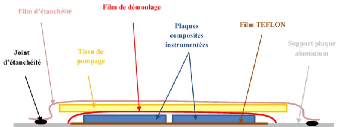
Figure 2.20 – Conditionnement de plaques en composite.
