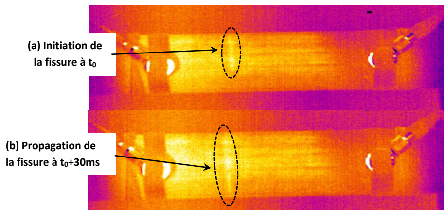
Figure 2.16 – Identification de la nature, de la localisation (a) et de la propagation (b) d'une fissure intralaminare dans les plis à 90^\circ d'une éprouvette [0_2, 90_4]_S .
