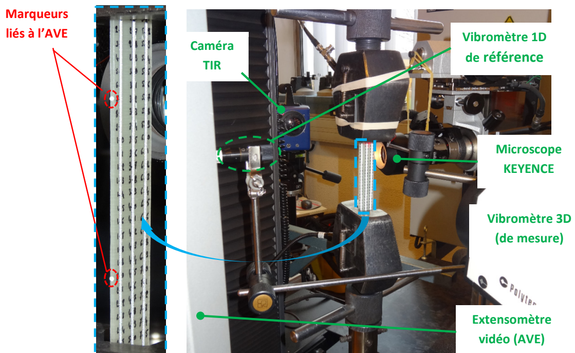
Figure 2.19 – Illustration du montage expérimental.
