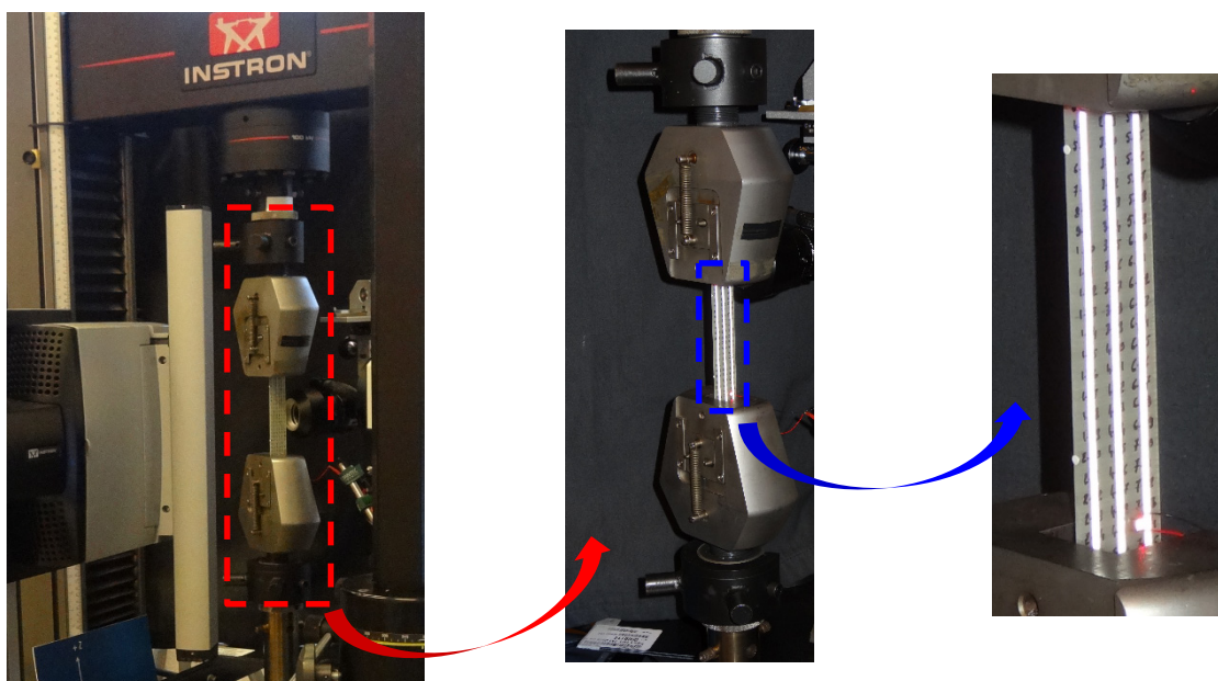
Figure 2.9 – Illustration du système de sollicitation INSTRON.
