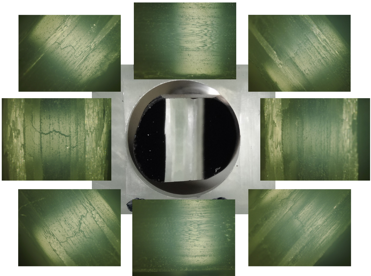
Figure A2-6 - Observation de la paroi du trou à 1,35% de déformation.
