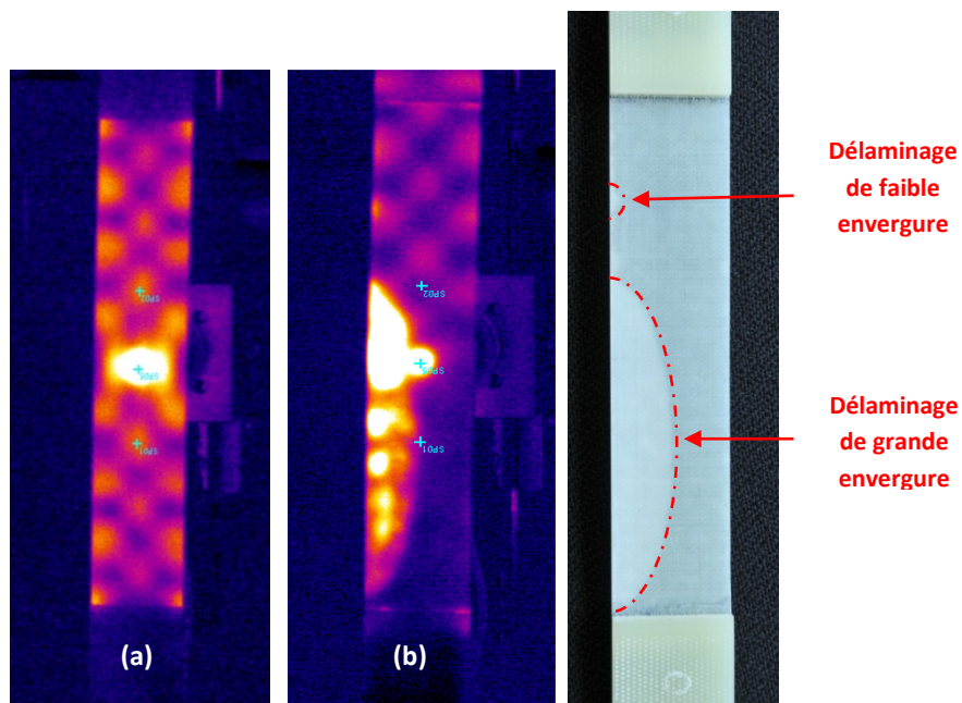
Figure 3.28 – Localisation de délaminages, de faible et grande envergure sur une éprouvette [0_2,+45,-45,90_2]_s . De l'état sain (a) à l'état endommagé (b).
