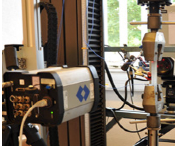
Figure 2.15 – La Thermographie InfraRouge (TIR) en tant que méthode de mesure sans contact sensible à l'apparition d'endommagements.
