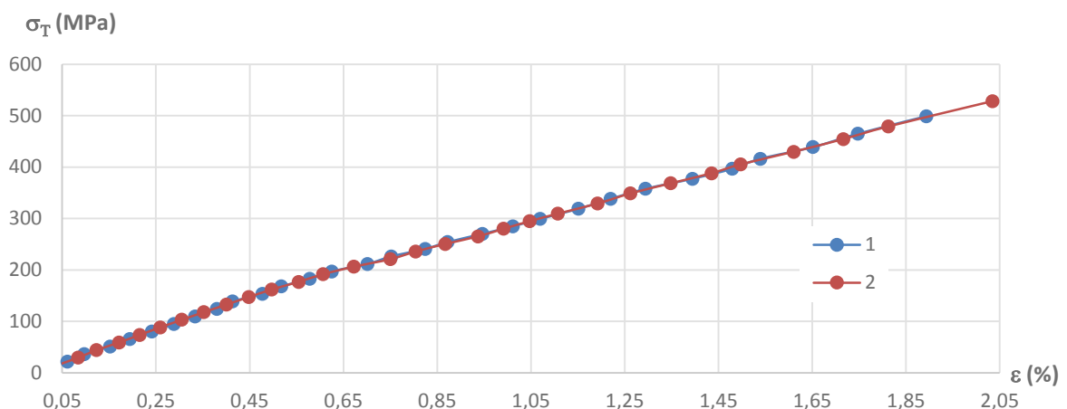
Figure 3.1 – Augmentation artificielle de la discrétisation sous la forme de 60 steps de chargement.
