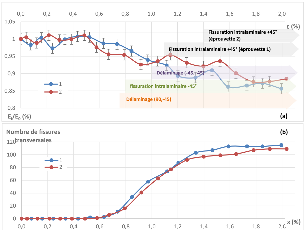
Figure 3.11 – Evolution du module apparent (a) et du nombre de fissures transversales (b) au cours de la sollicitation pour 2 éprouvettes [0_2,+45,-45,90_2]_s .
