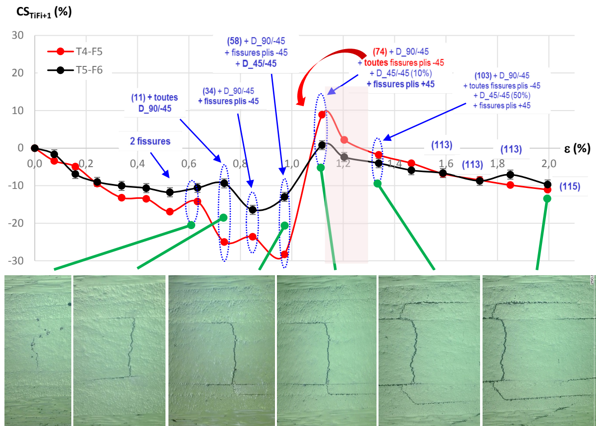
Figure 3.17 – Evolution du critère de santé associé à l'éprouvette [0_z,+45,-45,90_z]_s n°1.
