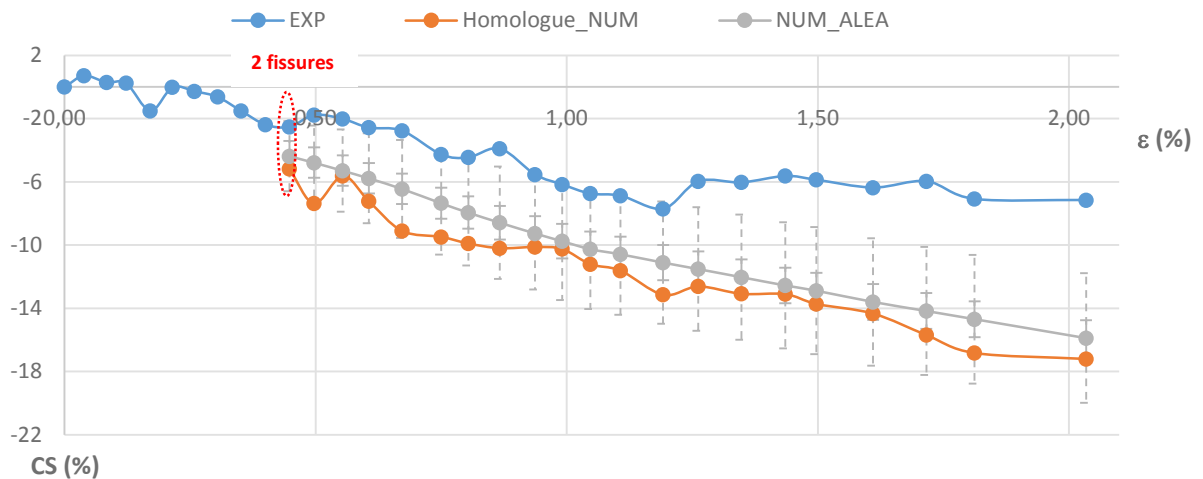
Figure 4.49 – Evolution des critères de santé numérique et physique T_3F_4 associés à l'éprouvette [0_3,90_3]_S n°2.
