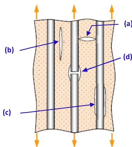
Figure 1.2 – Mécanismes de rupture élémentaires liés à la rupture transversale de la matrice (a), à la rupture longitudinale de la matrice (b), à la décohésion fibre-matrice (c) et à la rupture des fibres (d) dans un UD[2].
