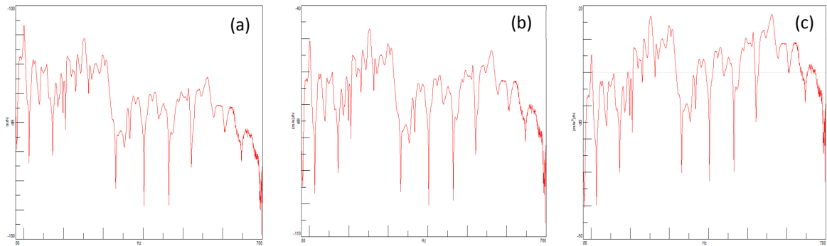
Figure 1.29 – Illustration d'une FRF associée à un réceptance, une mobilité ou une inertance.
