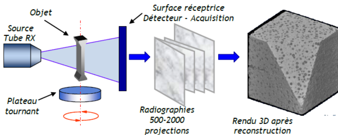
Figure 1.12 – Principe de fonctionnement de l'acquisition des données [13].
