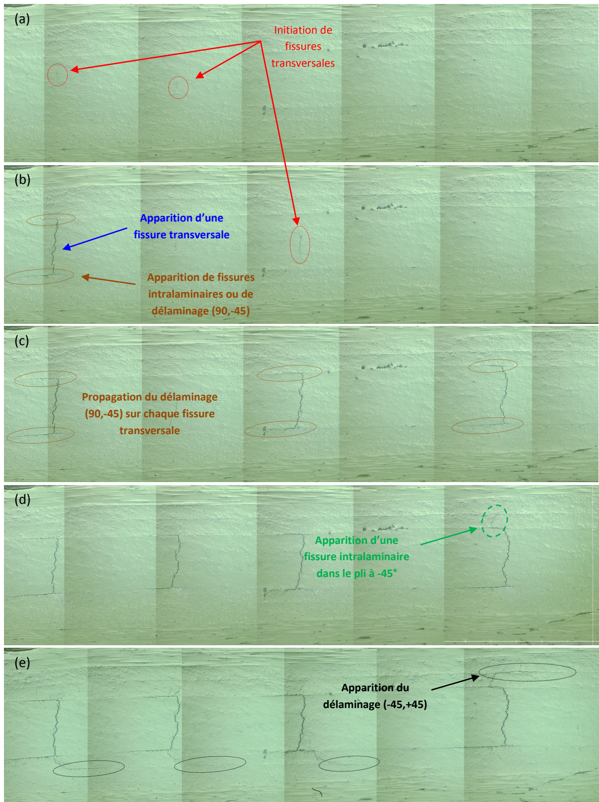
Figure 3.12 – Eprouvette [0_2, +45, -45, 90]_s n°1 : (a) initiation de fissures intralaminaires dans les pli à 90^\circ au step 7 à \varepsilon=0.67\% , (b) apparition d'une fissure transversale et du délaminage (90,-45) au step 8 à \varepsilon=0.79\% , (c) propagation du délaminage (90,-45) au step 9 à \varepsilon=0.85\% , (d) apparition d'un fissure intralaminare dans les plis à -45^\circ au step 10 à \varepsilon=0.97\% , (e) apparition du délaminage (-45,+45) au step 11 à \varepsilon=1.15\% .
