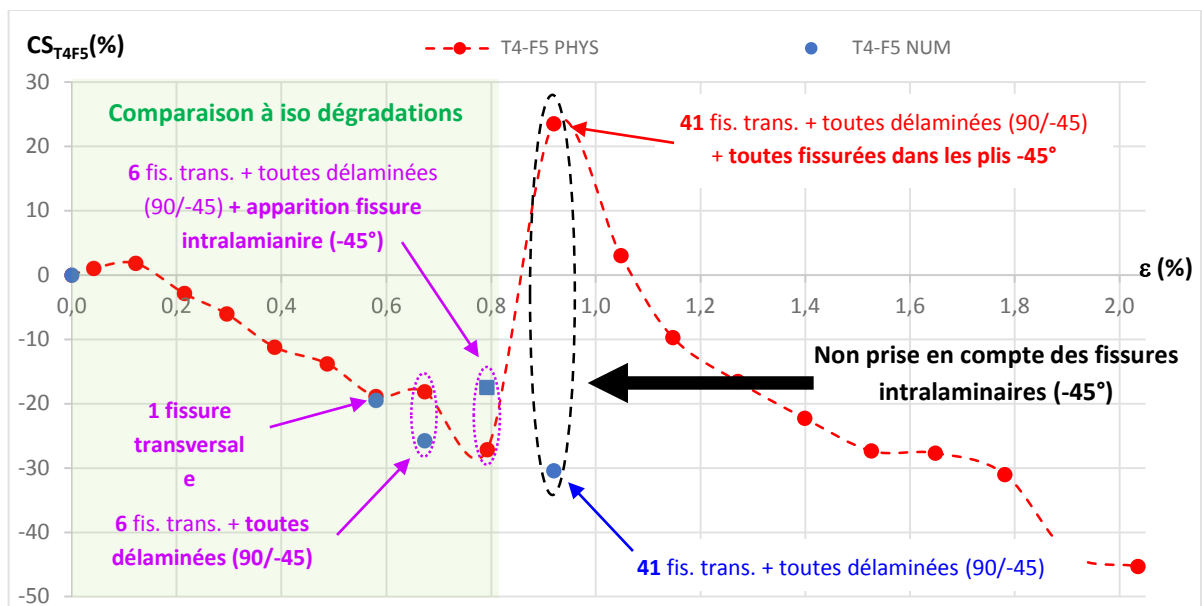
Figure 4.63 – Comparaison des critères de santé physique et numérique, associé au couple de modes T_4F_5 , en fonction de la déformation.
