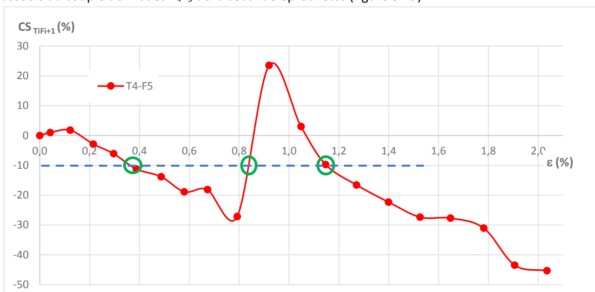
Figure 3.19 – Illustration du dilemme associé à la présence de ce sursaut.
