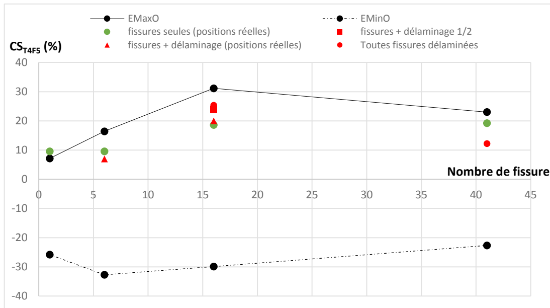
Figure 4.58 – Evolution du CS_{T4F5} en fonction du nombre de fissures transversales et du délaminage (90,-45) associé.
