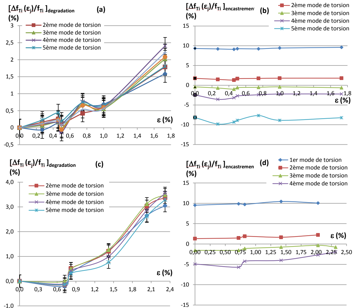
Figure 2.26 – Evolution des modes de torsion T2, T3, T4, T5 des éprouvettes [0_3, 90_3]_S et [0_2, +45, -45, 90_2]_S en fonction des dégradations uniquement (a)(c) et de l'encastrement uniquement (b)(d).
