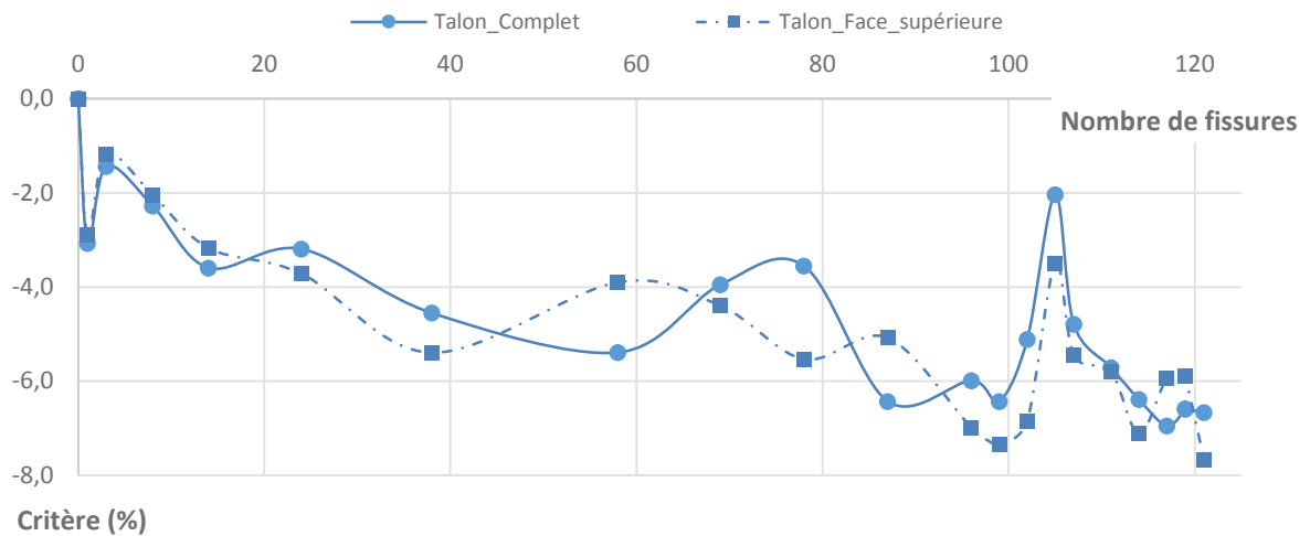
Figure 4.42 – Impact de l'encastrement (a) Talon Complet (b) Talon Face Supérieure, sur l'évolution du critère de santé numérique associé au couple de modes T_3F_4 de l'éprouvette numérique [0_3,90_3]_S n°1.
