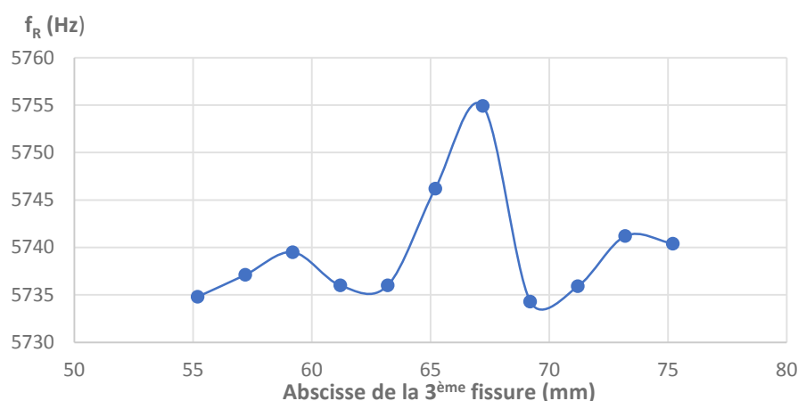
Figure 4.36 – Evolution de la f_R du 5 ème mode de flexion en fonction du décalage de la fissure centrale et en présence de 4 autres fissures positionnées à l’aplomb de chaque lobe.
