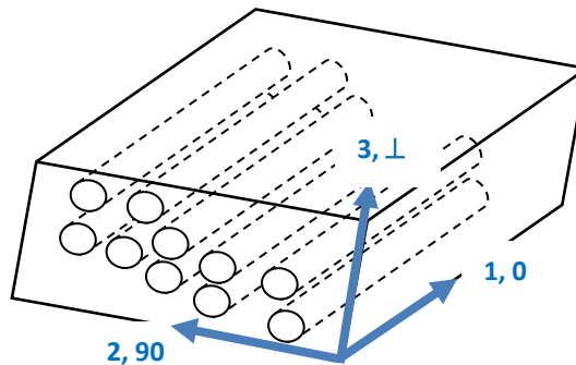
Figure 1.30 – L'axe 1 est orienté selon la direction des fibres de l'UD, l'axe 2 suivant la direction transversale et l'axe 3 selon l'épaisseur de la plaque.
