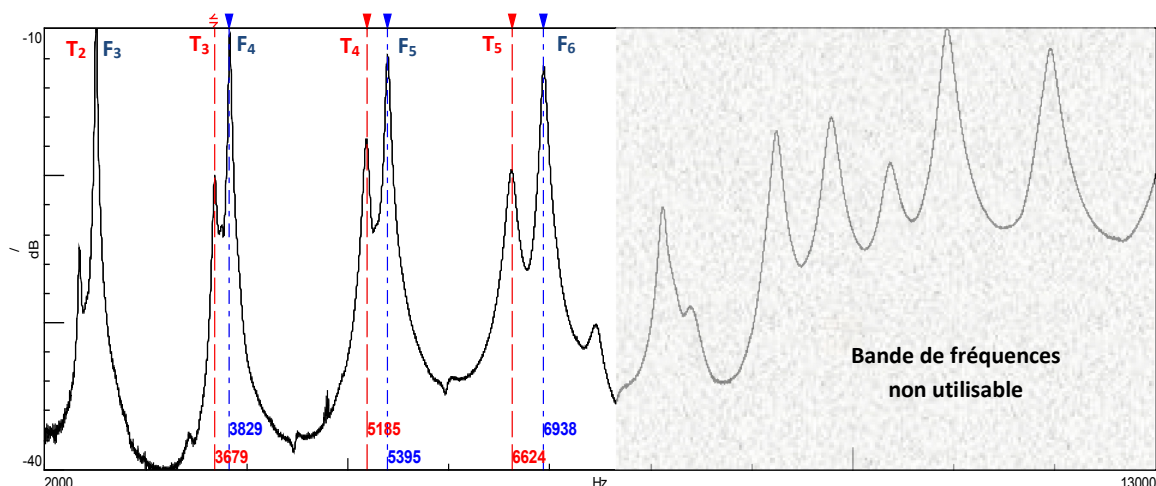
Figure 2.29 – Illustration du phénomène de couplage entre modes de flexion et modes de torsion.
