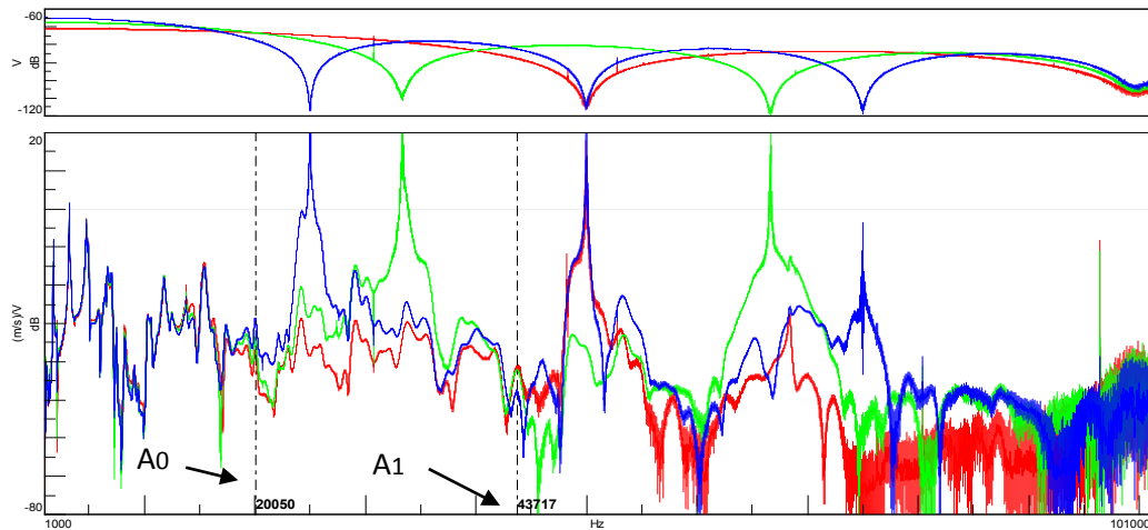
Figure 3.25 – Identification de la f_R du mode de Lamb antisymétrique A_0 .
