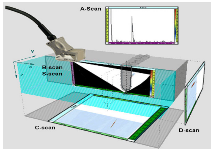
Figure 1.9 – Illustration des méthodes de contrôle A-scan / B-scan / C-scan et D-scan [6].
