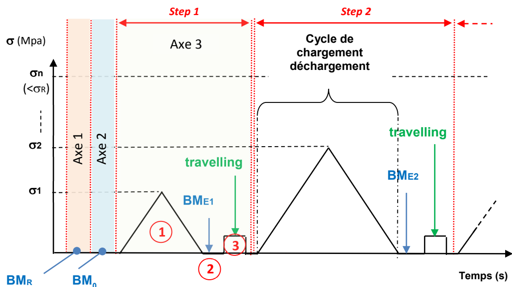
Figure 2.1 – Illustration du protocole expérimental en configuration « encastré – encastré ».
