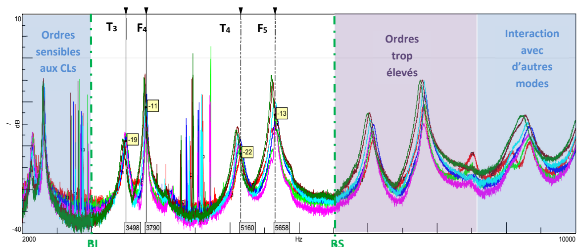
Figure 3.8 – Illustration du protocole de prétraitement des données, à partir des courbes représentatives de la moyenne des FRFs mesurées, à différents stades de dégradation, sur l'éprouvette [0_3, 90_3]_s n°2.
