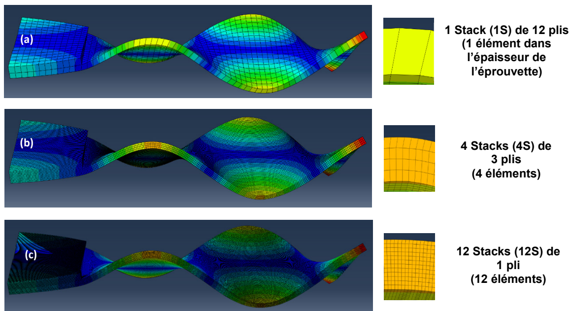
Figure 4.8 – Illustration du composite [0_3, 90_3]_S sous forme de stacks.
