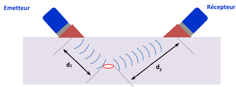
Figure 1.8 – Illustration du principe de détection en réflexion [3].
