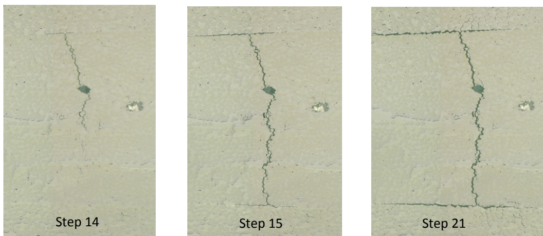
Figure 2.11 – Illustration des phases de transition (steps 14 à 15) ou de propagation (steps 15 à 21) des dégradations.
