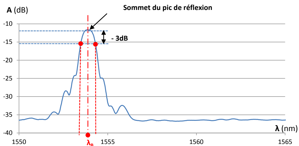
Figure 1.16 – Identification de la longueur d'onde de Bragg.
