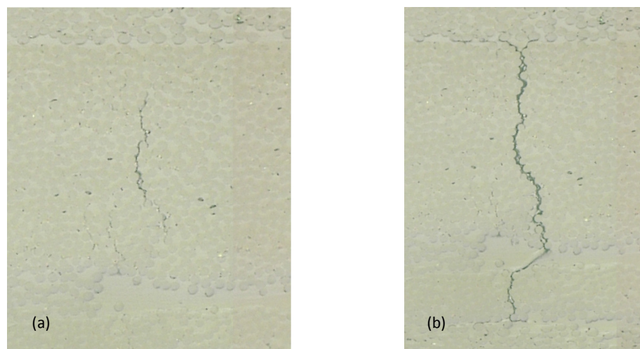
Figure 1.4 – Coalescence des mécanismes de rupture microscopiques liés à la décohésion « fibre/matrice » et à la rupture matricielle (a), puis propagation de la rupture à l'échelle mésoscopique : fissuration intralaminare (b).
