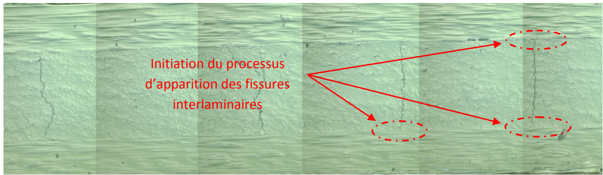
Figure 3.5 – Illustration du processus d'initiation du délaminage en bord d'éprouvette.
