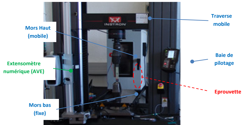
Figure 1.32 – Illustration du banc de caractérisation Matériau (INSTRON).
