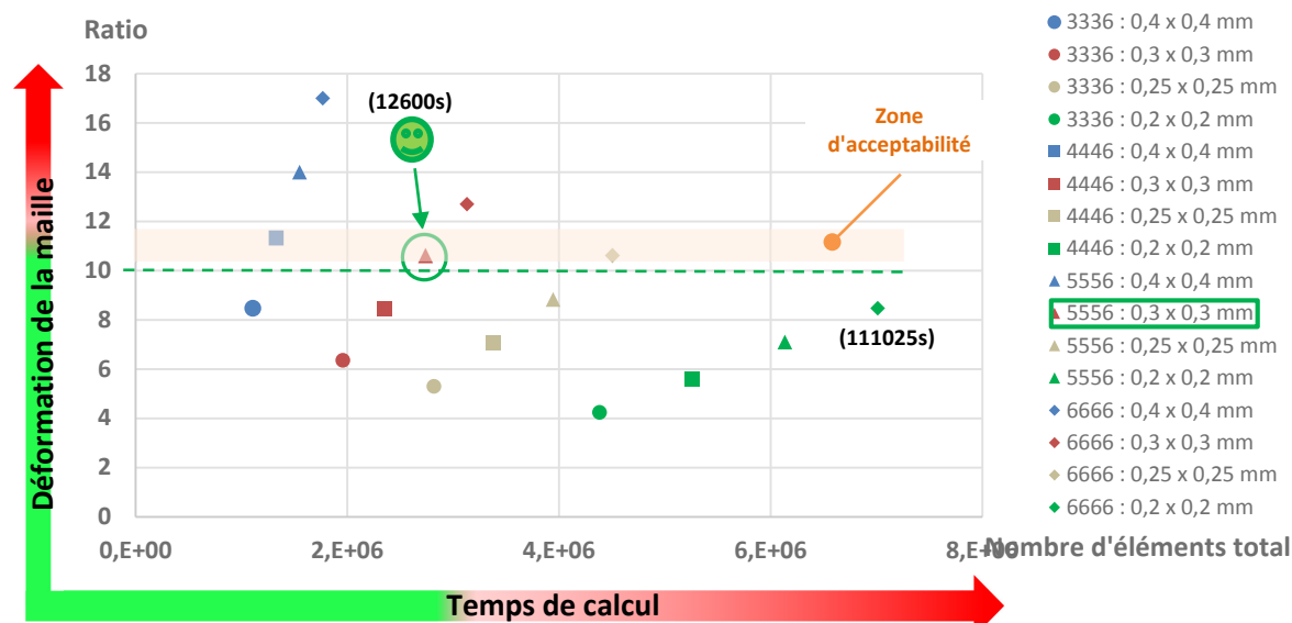
Figure 4.15 - Etude de convergence associée aux différents maillages d'éprouvette [0_2,45,-45,90_2]_s . La zone d'acceptabilité des modèles est fondée sur l'aspect ratio maximal, un nombre maximal (taille du modèle) et minimal (déformée modale) d'éléments.
