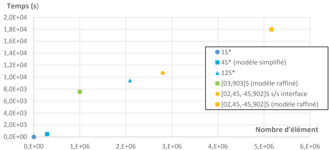
Figure 4.60 – Evolution du temps de calcul en fonction des différents modèles proposés.
