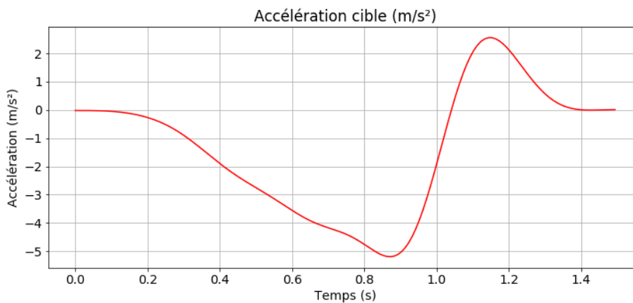
Figure 54 : Accélération cible du profil de commande SAAM (m/s²)
