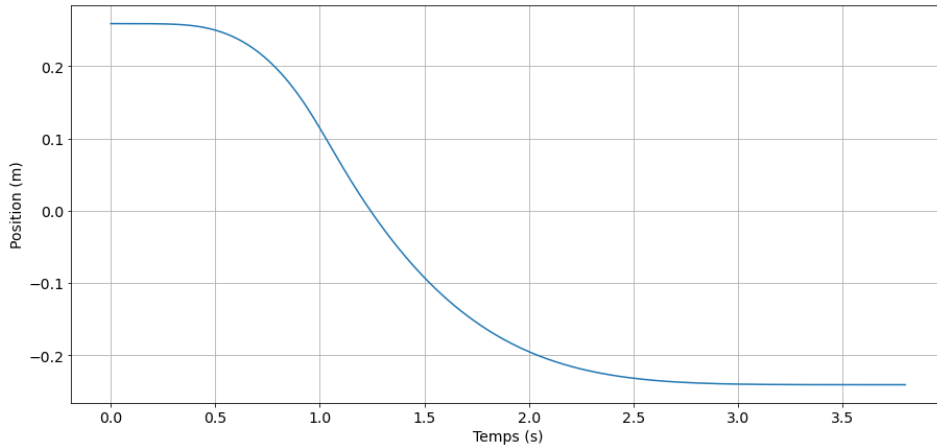
Figure 56 : Commande de position linéaire ( y ) (m)
