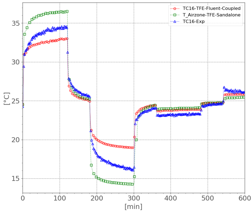
Figure 105: Température entre les deux sièges – supérieur (RMSD Coupled: 1.146 / RMSD Standalone: 1.463)
