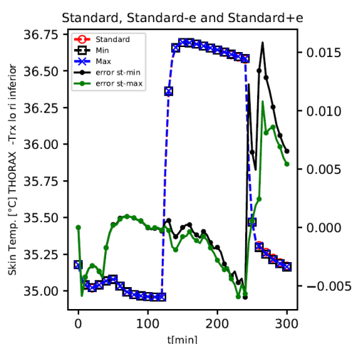
Figure 59 Variation de la température de peau pour le thorax pour les 3 mannequins: standard, avec capacité calorifique maximale (Max), avec capacité calorifique minimale (Min), avec la différence entre le standard et le Max (error st-max) et la différence entre le standard et le Min (error st-min)
