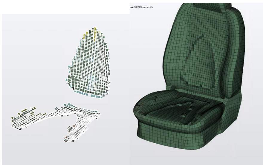
Figure 97 Zone de contact (gauche) et déformation du siège (droite)
