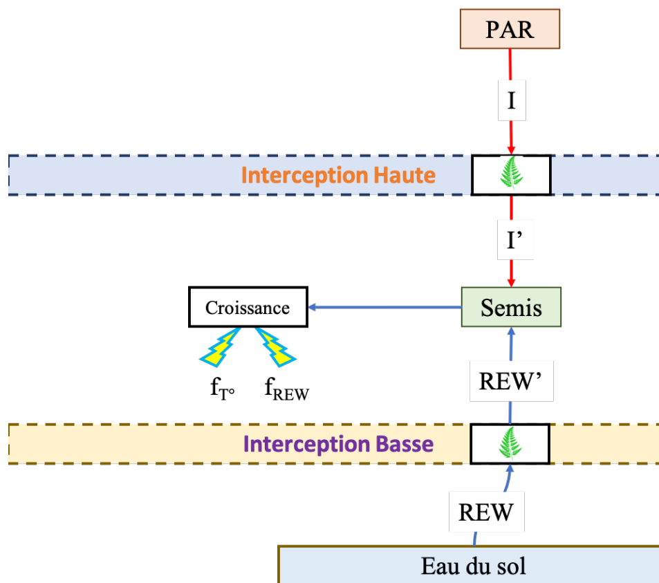
Figure 56. Schéma de la conception pour le modèle de croissance représentant l'interception de la lumière incidente ( I ) et de l'eau du sol ( REW ) par la fougère aigle et l'impact de cette compétition sur la croissance.
