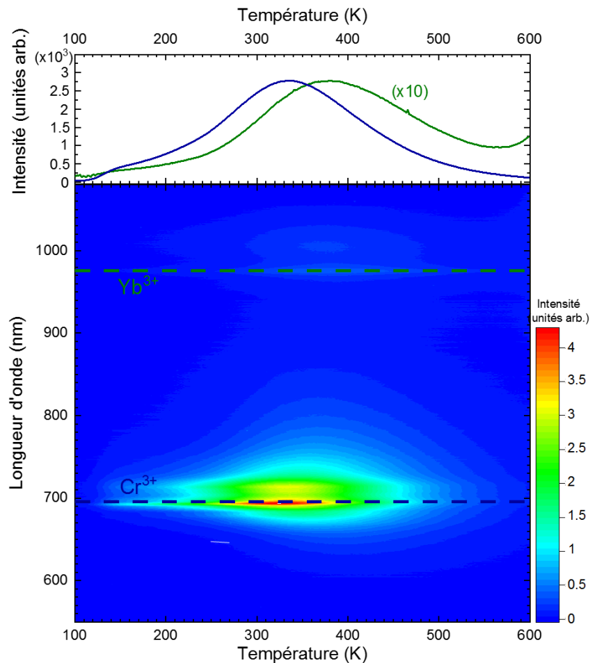
Figure 6.27: Courbe de thermoluminescence 2D de \text{ZnGa}_2\text{O}_4:\text{Cr}^{3+}, \text{Yb}^{3+} nGC après excitation par une lampe Xe (330 nm). Au-dessus, comparaison des profils de thermoluminescence de \text{Cr}^{3+} et \text{Yb}^{3+} .
