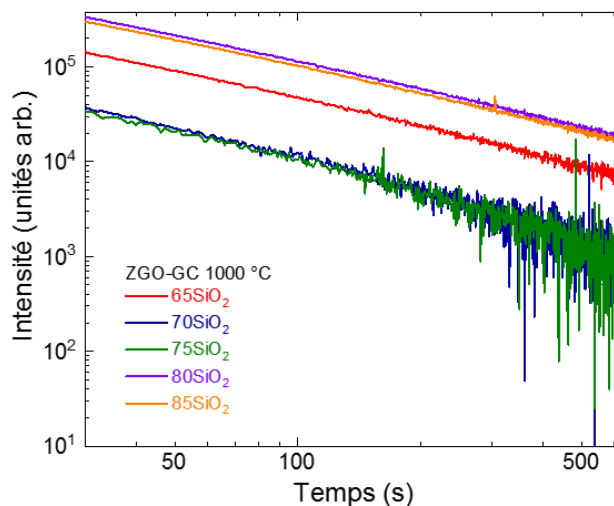
Figure 5.20 : Déclins de luminescence persistante des échantillons nano-vitrocéramiques à différents taux de silice enregistrés après excitation UV ( \lambda_{exc} = 254 nm) pendant 5 minutes.
