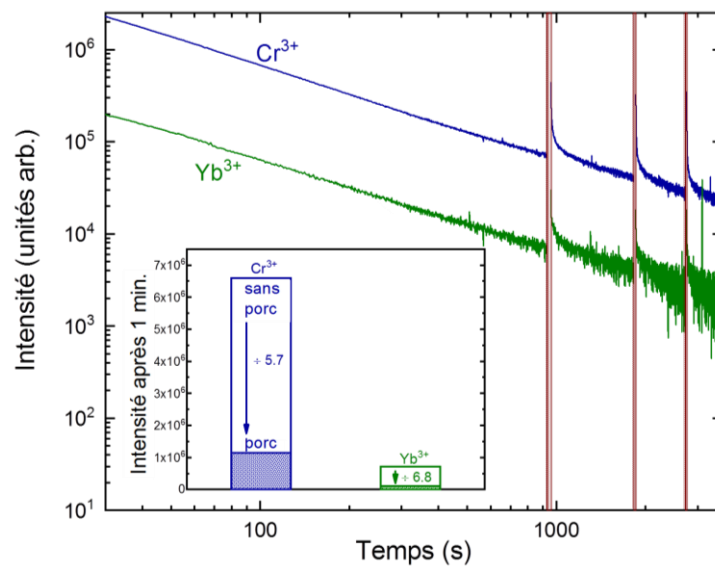
Figure 6.28 : Déclins de luminescence persistante des ions \text{Yb}^{3+} (vert) et \text{Cr}^{3+} (bleu) dans \text{ZnGa}_2\text{O}_4 – GC 1000 °C enregistrés sous une tranche de 4 mm de porc. A la suite de l'excitation ( \lambda_{\text{exc}} = 365 \text{ nm} , 5 min.), des stimulations optiques ( \lambda_{\text{exc}} = 850 \text{ nm} ) de 30 s ont été soumises à l'échantillon 5, 10 et 15 minutes après arrêt de l'excitation. Dans l'insert est représentée la comparaison entre l'intensité de luminescence persistante sans et avec le porc.
