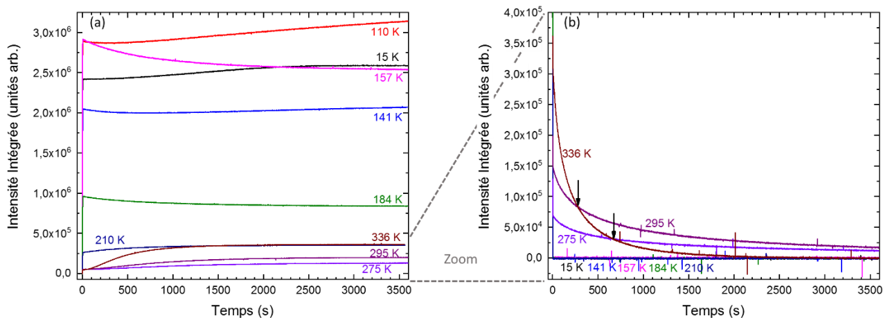
Figure 3.10 : Intensité de luminescence (a) sous excitation et (b) après arrêt de l'excitation (b) de l'aluminate de calcium enregistré à différentes températures. Pour se repérer, les températures utilisées ici sont également indiquées par des flèches sur le profil de thermoluminescence (figure 3.0 (a)).
