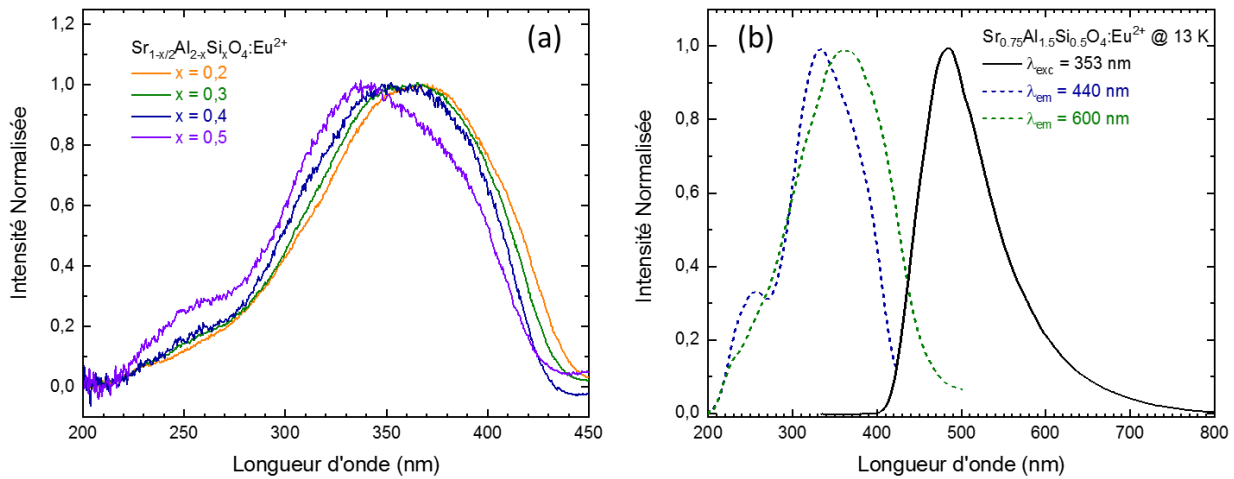
Figure 3.12 : (a) Spectres d'excitation des h-SASO avec \lambda_{em} = 500 nm. (b) Spectres d'excitation de h-SASO 0,5 centrées sur différentes longueurs d'onde d'émission.
