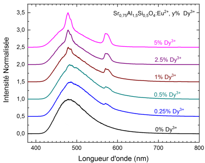
Figure A.3.2 : Spectres de photoluminescence du composé hexagonal \text{Sr}_{0,75}\text{Al}_{1,5}\text{Si}_{0,5}\text{O}_4:\text{Eu}^{2+}, y\% \text{Dy}^{3+} avec y allant de 0 à 5 avec \lambda_{\text{exc}} = 353 \text{ nm} à 10 K.
