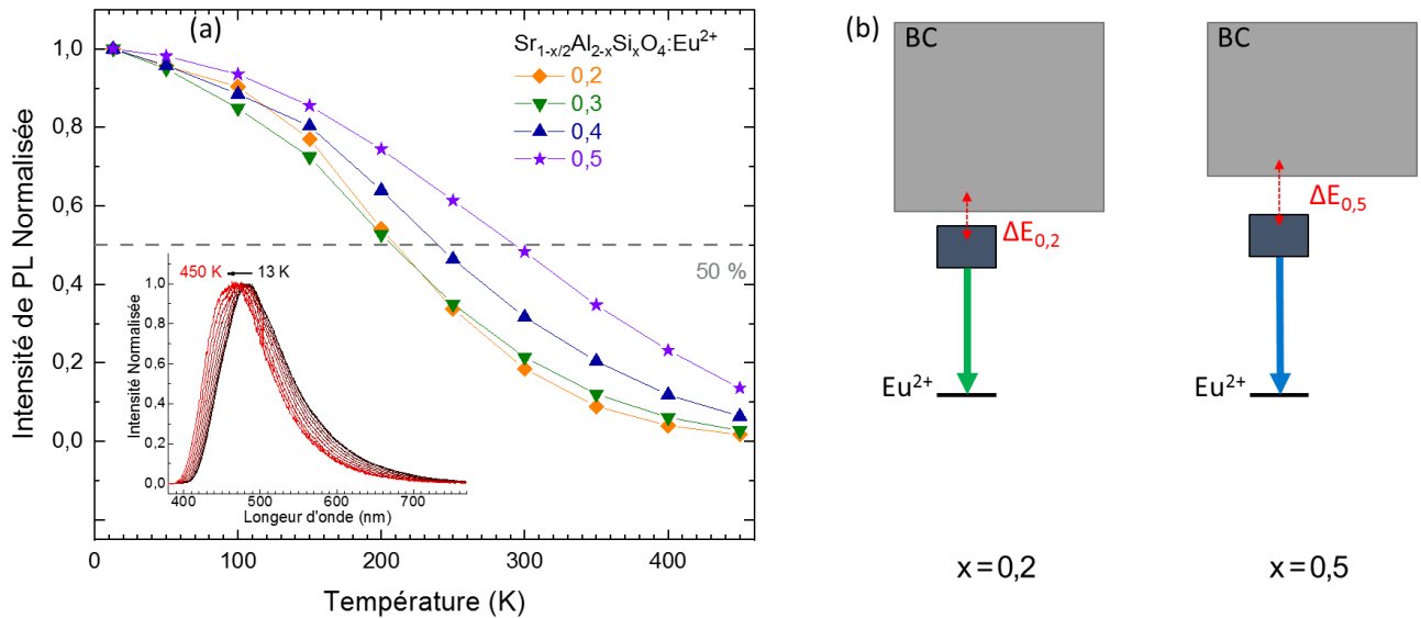
Figure 3.16 : Extinction thermique de l'émission de l'europlum dans les échantillons mono-dopés \text{Eu}^{2+} . En insert est représenté l'évolution des spectres d'émission normalisés de l'échantillon h-SASO 0,5 en fonction de la température de mesure. A droite est représenté un schéma de l'évolution de la position des niveaux d'énergie en tenant compte de l'évolution du « quenching » thermique.
