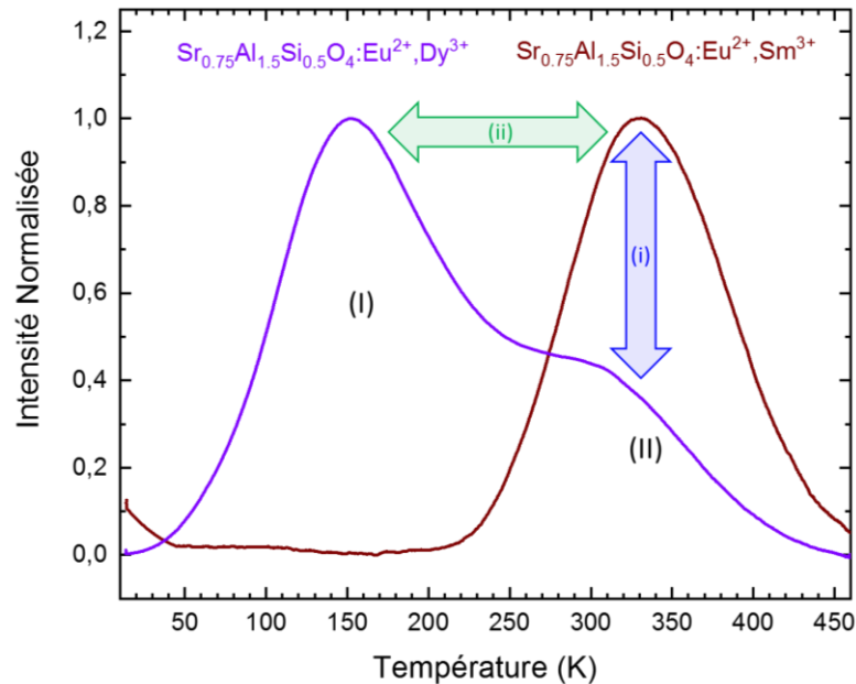
Figure 3.23 : Comparaison des profils de thermoluminescence normalisés des échantillons h-SASO co-dopés Eu^{2+}, Dy^{3+} (violet) et Eu^{2+}, Sm^{3+} (rouge). Le piégeage est effectué sous irradiation UV ( \lambda_{exc} = 365 nm) pendant 5 minutes à 12 K avant la montée en température.
