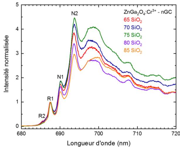
Figure 5.19 : Spectres de photoluminescence normalisés par rapport à la raie R1 des échantillons vitrocéramiques avec différentes compositions de la matrice vitreuse. Les spectres ont été enregistrés à 20 K avec \lambda_{exc} = 420 nm.
