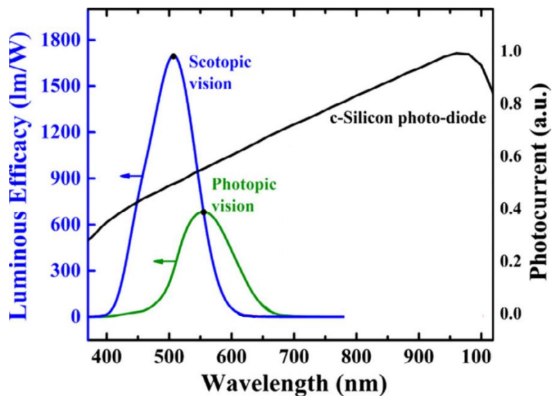
Figure 1.5 : Spectres de détection de l'œil en vision scotopique (bleu) et photopique (vert) comparés avec la détection d'une photodiode silicium utilisée dans les caméras visibles. Cette figure est adaptée de Zhuang et al. 11
