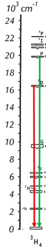
Figure 4.1. Diagramme de Dieke de l'ion \text{Pr}^{3+} .
