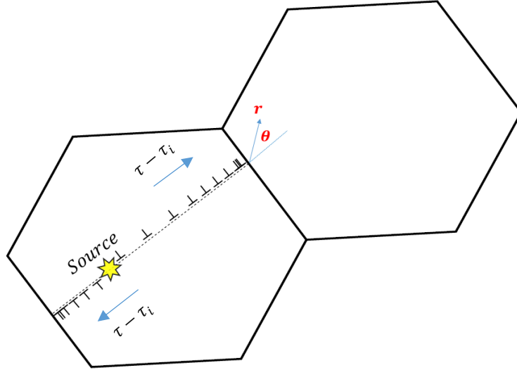
Figure 10 : Empilement de dislocations coins émises par une source de Franck-Read et bloquées au niveau du joint entre deux grains adjacents.
