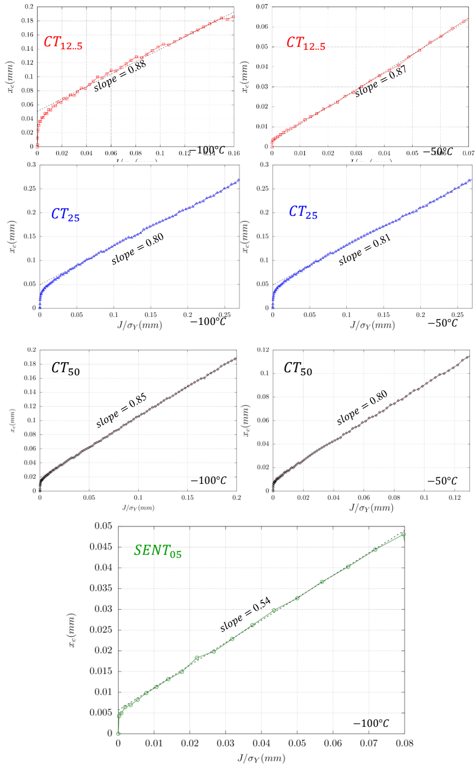
Figure 99 : La distance x_c en fonction de J/\sigma_Y pour les éprouvettes CT_{12.5} – CT_{25} – CT_{50} – SENT_{0.5} à -50^\circ C et à -100^\circ C .
