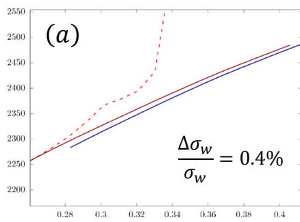
Figure 85 : Comparaison de la contrainte de Weibull à partir des deux méthodes avec m = 20 . (a) Vue de près qui compare la contrainte de Weibull filtrée du rayon R_0 = 0.3\mu\text{m} (courbe rouge) avec le domaine valide du rayon R_0 = 0.9\mu\text{m} (courbe bleue). (b) Vue de près qui compare la contrainte de Weibull filtrée du rayon R_0 = 0.9\mu\text{m} (courbe bleue) avec le domaine valide du rayon R_0 = 3\mu\text{m} (courbe rose).
