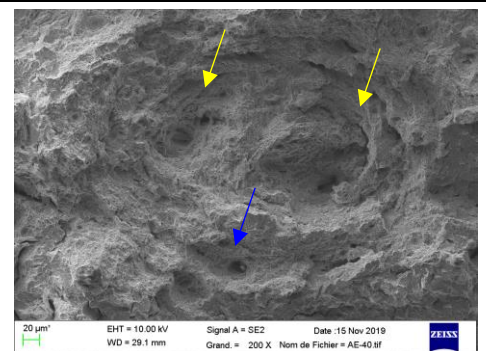
Figure 45 : Image au centre (échelle 20µm) des zones ductiles observées dans la figure précédente. Présence des cupules de grandes tailles initiées sur des inclusions MnS (très allongées) et d'autres relativement de petites tailles)
