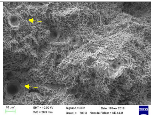
Figure 49 : Images au centre (échelle 10 \mu m) des éprouvettes DP_6 , AE_4 , AE_{10} . Les flèches jaunes désignent la plus grande cupule de l'image.
