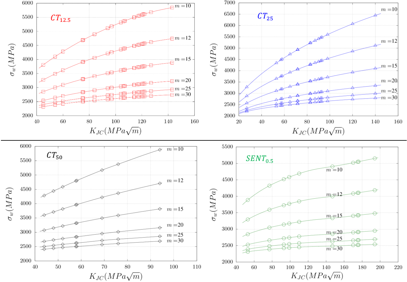
Figure 97 : Effet de m sur la contrainte \sigma_w (corrigée avec l'épaisseur B_e ) pour m = 10; 12; 15; 20; 25; 30 à -100^\circ C
