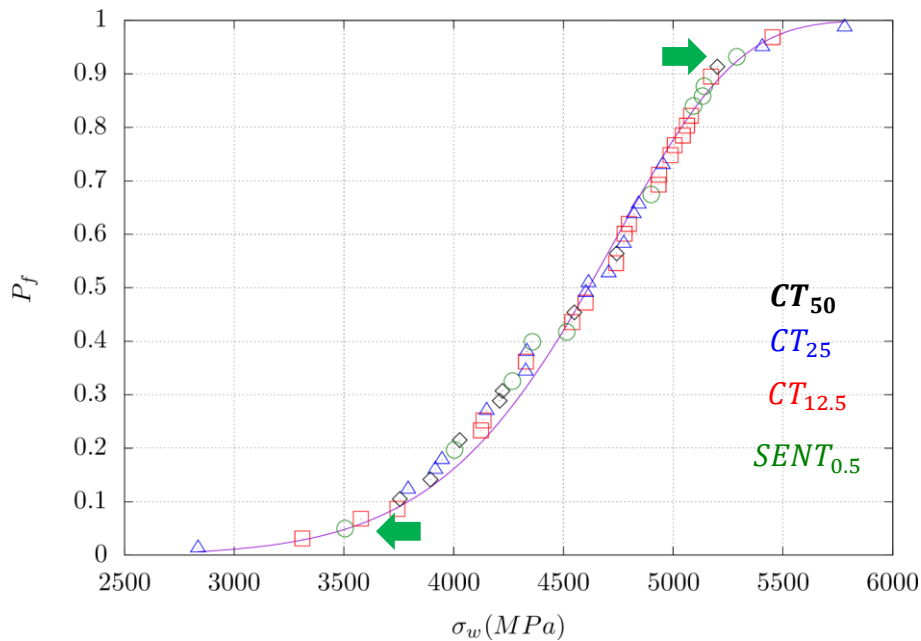
Figure 106 : P_f^{exp} expérimentale (points) et P_f^{weib} numérique (ligne) en fonction de \sigma_w pour m_{1s} = 9.6 ; \lambda_{1s} = 200 ; \sigma_{u_{1s}} = 4793.6 MPa ; Error = 0.2 et T = -100^\circ C
