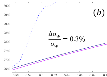
Figure 85 : Comparaison de la contrainte de Weibull à partir des deux méthodes avec m = 20 . (a) Vue de près qui compare la contrainte de Weibull filtrée du rayon R_0 = 0.3\mu\text{m} (courbe rouge) avec le domaine valide du rayon R_0 = 0.9\mu\text{m} (courbe bleue). (b) Vue de près qui compare la contrainte de Weibull filtrée du rayon R_0 = 0.9\mu\text{m} (courbe bleue) avec le domaine valide du rayon R_0 = 3\mu\text{m} (courbe rose).
