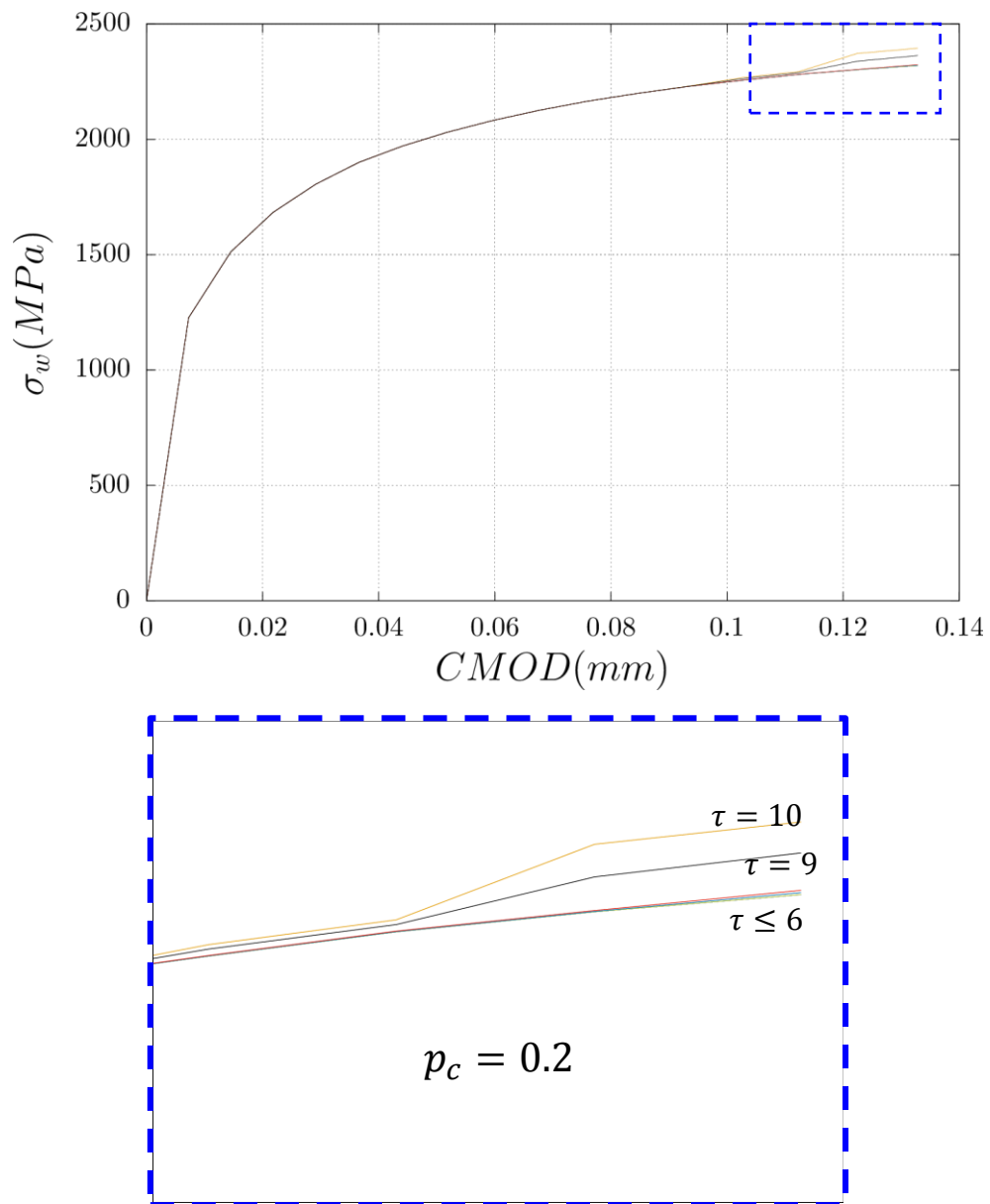
Figure 119 : La contrainte de Weibull \sigma_w en fonction du CMOD pour l'éprouvette CT_{50} à -100^\circ C . Le paramètre \tau a très peu d'effet sur le filtrage lorsque \tau \leq 6 .
