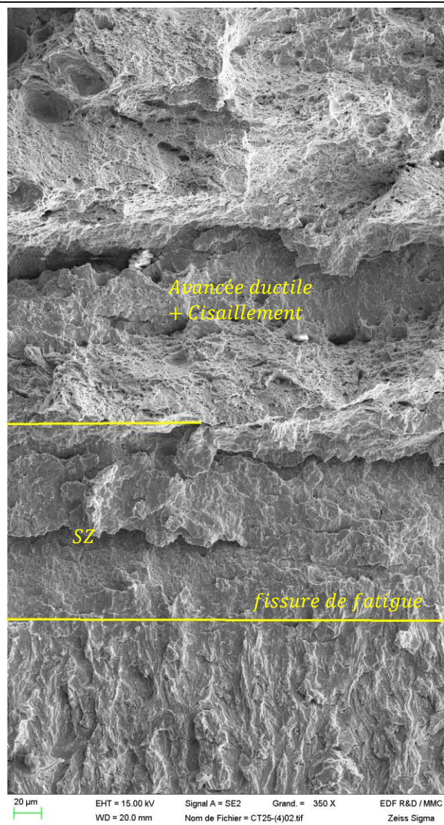
Figure 56 : Faciès des éprouvettes CT_{12.5} et CT_{25} . Existence d'une SZ, d'une zone de déchirure ductile. Ces deux éprouvettes s'amorcent dans le domaine ductile. Echelle est : 20\mu\text{m} .
