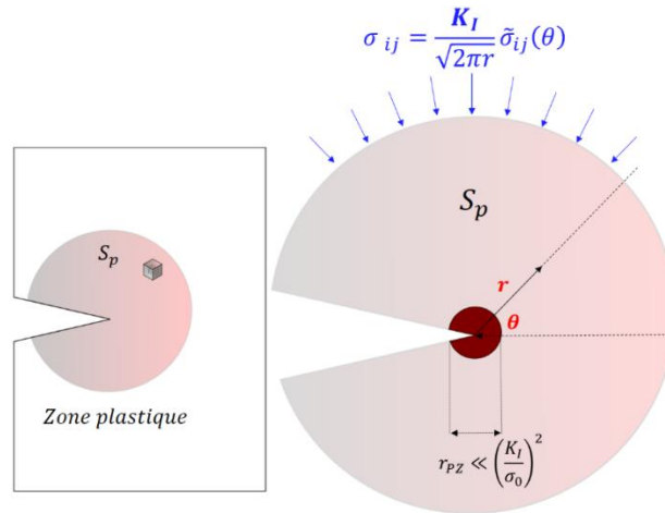
Figure 13 : Epruvette fissurée étudiée sous l'hypothèse de déformations planes dans le domaine de plasticité confinée SSY . La taille de la zone d'élaboration r_{pZ} –zone de couleur foncée– est négligeable devant la taille de zone plastique en SSY .
