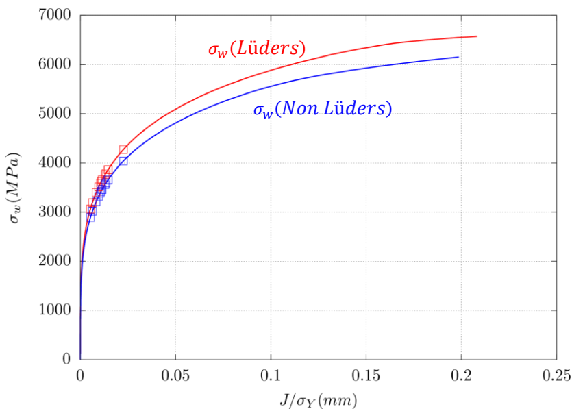
Figure 112 : \sigma_w avec et sans palier de Lüders à -150^\circ C . Eprouvette CT_{12.5} avec R_0 = 5\mu m . Les points représentent les mesures J/\sigma_Y expérimentales.
