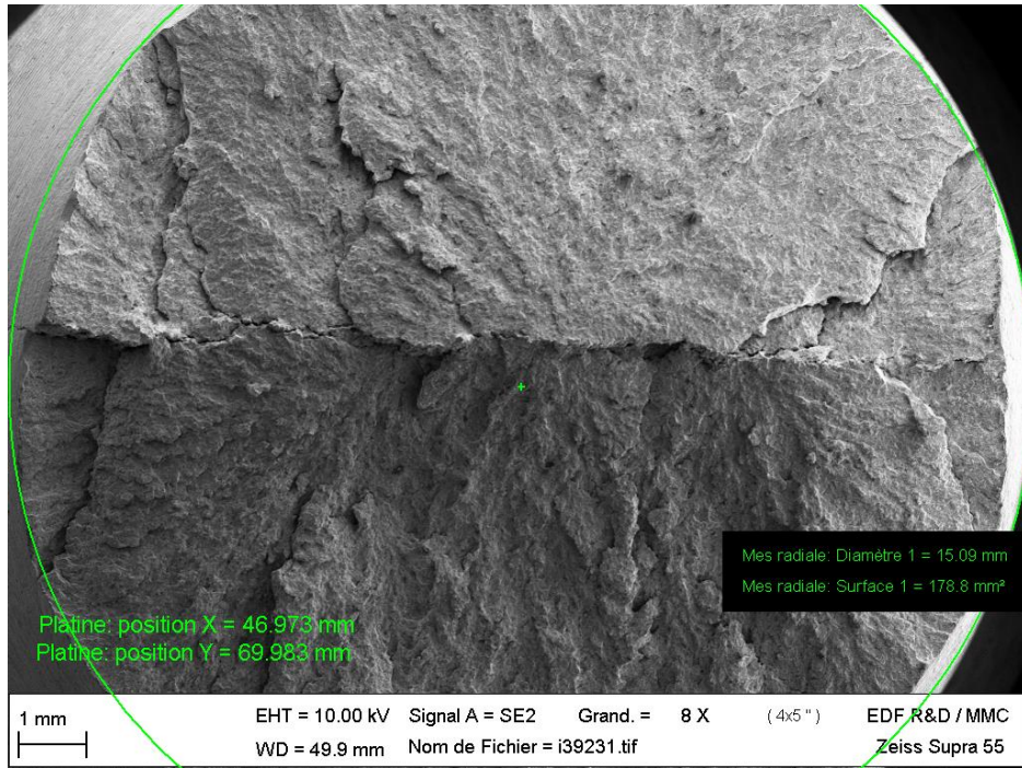
Figure 116 : Faciès du délaminage de l'éprouvette AE_{10} testée à -100^{\circ}C (1987-BT3-AE10-3)
