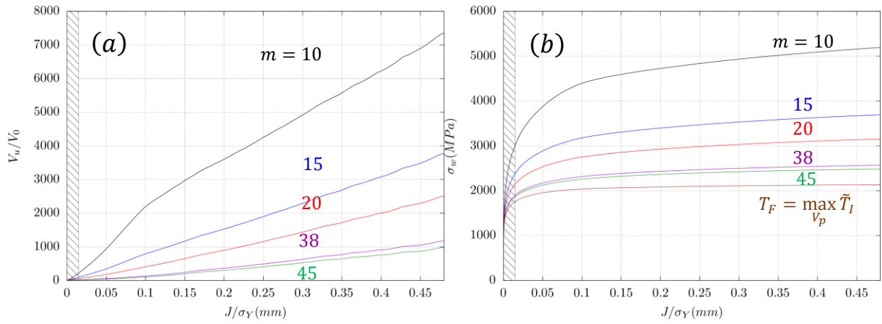
Figure 98 : (a) L'évolution de V_u/V_0 en fonction de m . (b) L'évolution de \sigma_w et de T_F = \max_{V_p} \tilde{T}_I . Sur l'éprouvette CT_{12.5} à -100^\circ\text{C} avec R_0 = 16\mu\text{m} . La zone hachurée correspond au domaine de SSY.
