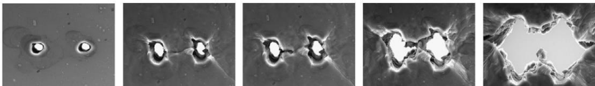
Figure 16 : croissance et coalescence des cavités ( Weck et al., 2008 )
