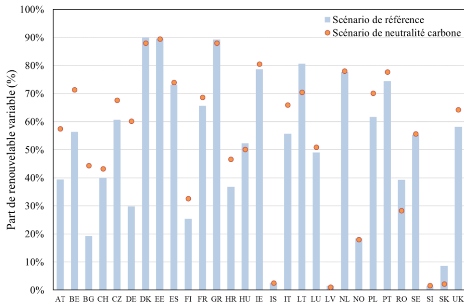
Figure 90- Part de renouvelable variable dans la production électrique totale en 2050 dans les scénarios de référence et de neutralité carbone
