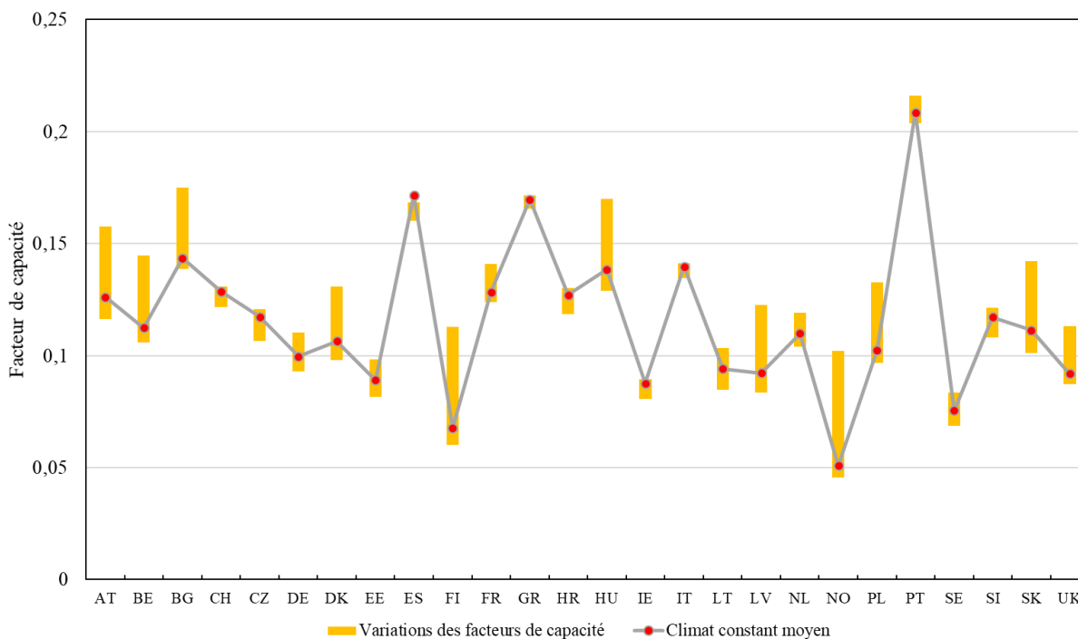
Figure 117- Variations du facteur de capacité du solaire pour l'ensemble des projections sur l'horizon 2030-2050
