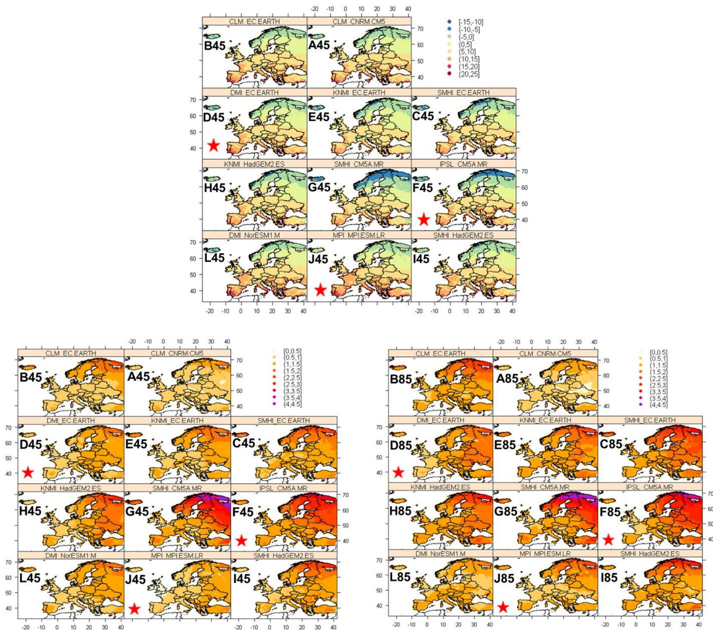
Figure 110- Températures moyennes annuelles (°C) pour la période historique (1976-2005) (figure supérieure) et anomalies (%) pour la période 2016-2045 pour les 11 combinaisons GCM-RCM sélectionnées avec le RCP 4.5 (en bas à gauche) et le RCP 8.5 (en bas à droite)
