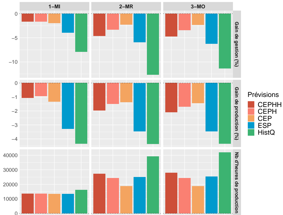
Figure 5.9 – Gains économiques relatifs de gestion, gains relatifs de production et nombre d'heures de production sur l'Ain à Vouglans.
