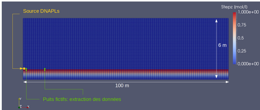
FIGURE 4.7: Modèle 2D du système aquifère-aquitard, représentation de la fonction step(z) dans l'aquitard, emplacement de la zone source ainsi que des zones d'extraction des données. Exagération \times 5 de l'échelle verticale.
