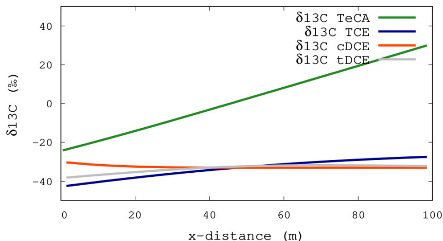
FIGURE 4.13: Profils longitudinaux des \delta^{13}C des concentrations aqueuses
