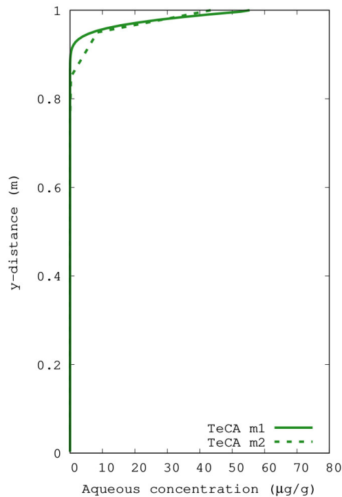
FIGURE 4.18: Profils de concentration (aqueuse) du TeCA dans l'aquitard à 19 ans, résultats des modèles m1 et m2
