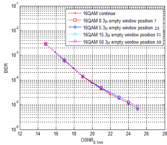
Figure 18 : Les courbes BER en fonction de l'OSNR (0.1 nm) sur différentes signal intervalle configurations en utilisant la méthode fenêtre glissant.
