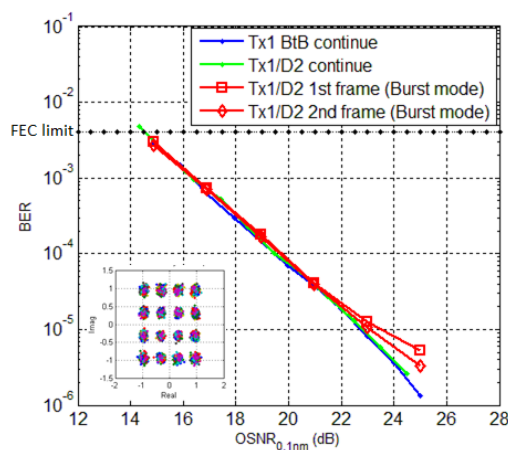
Figure 14 : Les courbes BER-OSNR (0,1 nm) pour Tx-1 / Rx au nœud D-2 en utilisant une modulation format 16QAM.
