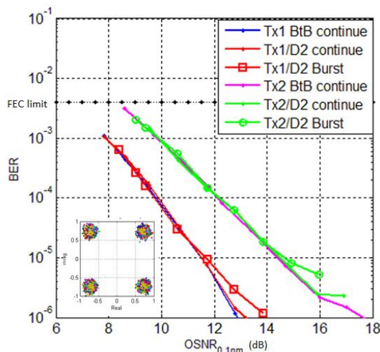
Figure 13 : Les courbes BER-OSNR (0,1 nm) pour Tx-1 et Tx-2 / Rx au nœud D-2 en utilisant une modulation format QPSK.
