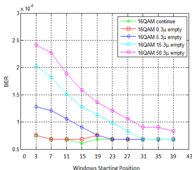
Figure 17 : Les courbes BER en fonction de la position de la fenêtre (le début de la fenêtre) à OSNR fixé (25 dB dans 0.1 nm) pour différentes durées de signal intervalle.
