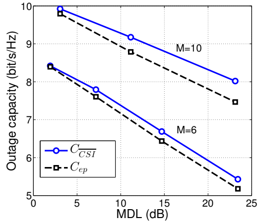
Figure E.7: Capacités de coupure vs MDL pour M = 6, 10 modes, SNR = 10dB.
