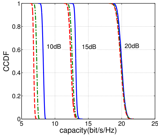
Figure E.4: Capacité CCDF avec CSI (solide), \overline{C_{SI}} (point-tiret) et C_{ep} (tiret) pour SNR=10,15,20 dB et MDL = 15dB
