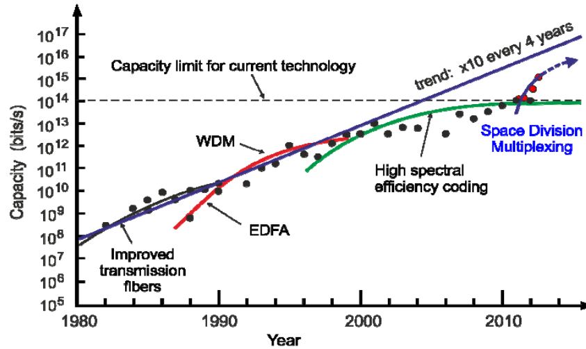
Figure E.3: L'évolution de la capacité des systèmes de transmission par fibre optique au fil des années. Figure tirée de [2].
