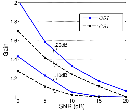
Figure E.5: Gain en C_{SI} (solide), Gain en \overline{C_{SI}} (tiret) en fonction du SNR pour MDL = 10, 20 dB pour la fibre 6-mode.
