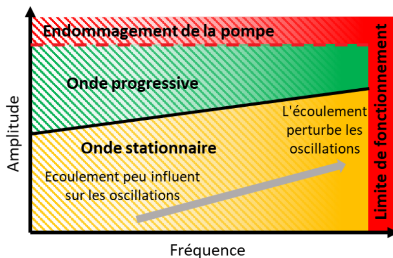
Figure 1.18 : Comportement qualitatif de la membrane en fonction de l'amplitude et de la fréquence d'excitation.
