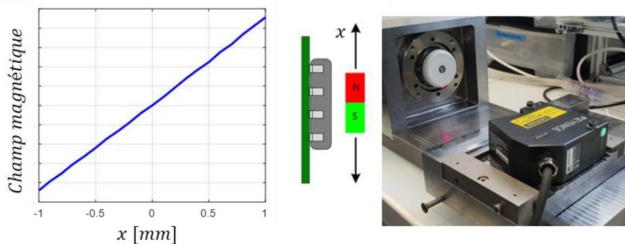
Figure 4.6 : schéma de principe, étalonnage du capteur à effet Hall et mesure laser de position
