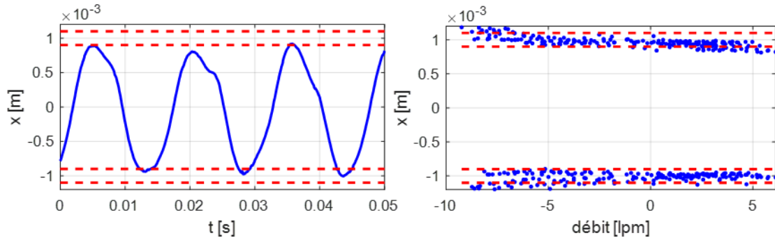
Figure 4.19 : A gauche, La position de la membrane pour Q < 0 lpm et f_d > 60 Hz. La mise en drapeau de la membrane entraine des oscillations instables qui ne sont pas contrôlables par la commande sans capteurs. A droite, Minimum et maximum de la position en fonction du débit. Toutes les fréquences sont confondues.
