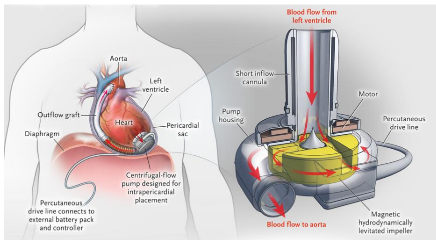
Figure 1.6 : Eléments de la pompe HVAD [14].
