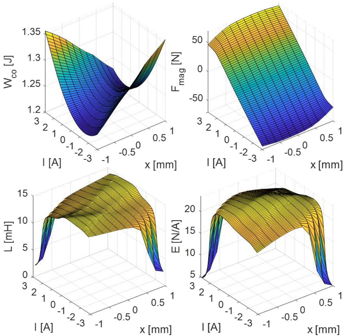
Figure 2.7 : Résultat de la modélisation de l'actionneur. En haut, la co-énergie et la force calculée par le logiciel EF. En bas, l'inductance et la force contre électromotrice.
