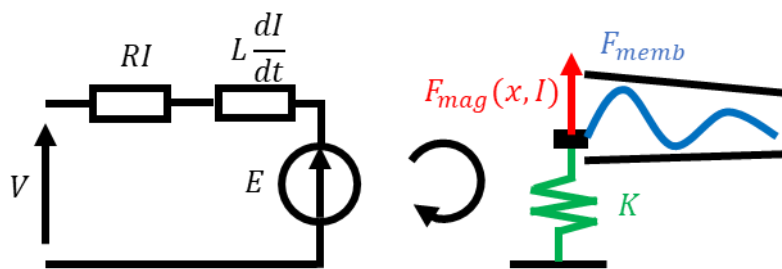
Figure 2.8 : système actionneur et membrane
