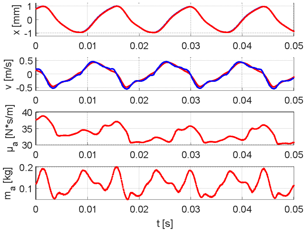
Figure 3.2 : estimation de la force de la membrane par l'EKF sur une co-simulation de la pompe. En bleu les signaux réels. En rouge les signaux estimés pour q_3 = 10^5 et q_4 = 10
