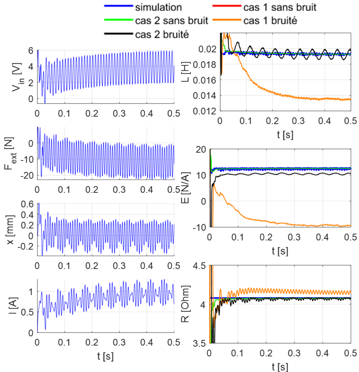
Figure 2.11 : résultat de simulation des cas 1 et 2. Signaux de l'actionneur (gauche) et estimation des paramètres (droite)
