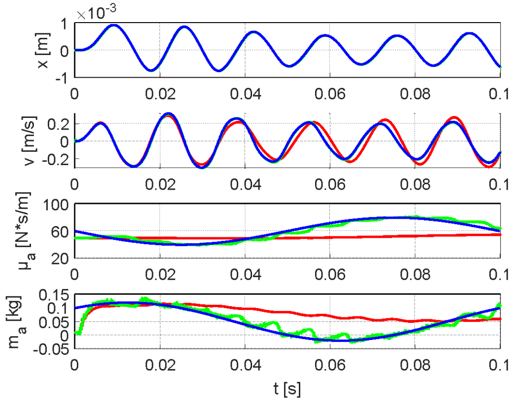
Figure 3.1 : Résultats de réglage de l'EKF. En bleu les signaux réels, en rouge les signaux estimés pour q_3 = 10 et q_4 = 10^{-3} , en vert les signaux estimés pour q_3 = 10^5 et q_4 = 10
