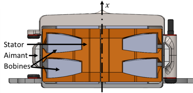
Figure 2.2 : CAD de l'actionneur
