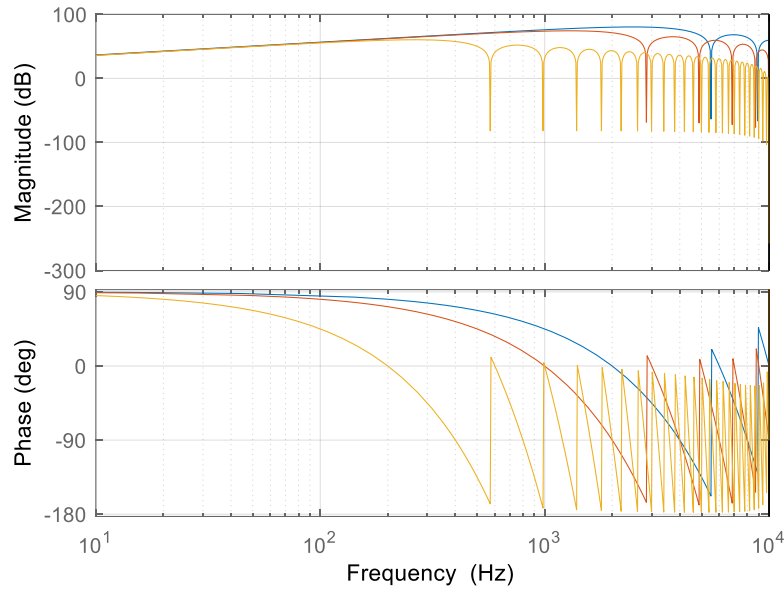
Figure 3.8 : réponse fréquentielle du dérivateur algébrique pour N=5 (bleu), N=10 (rouge), N=50 (jaune)
