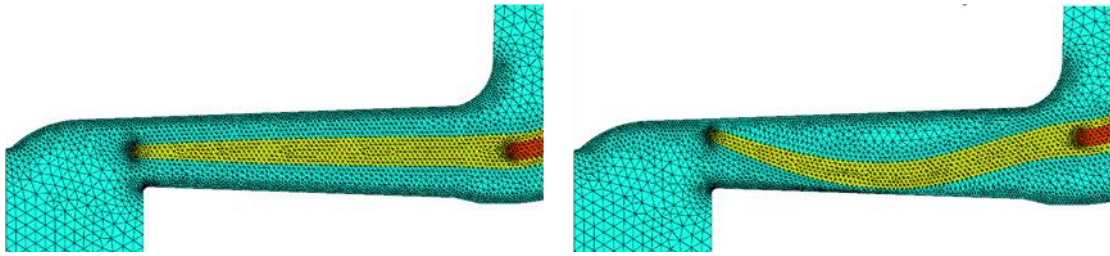
Figure 2.17 : déformation du maillage fluide (droite) par rapport au maillage initial (gauche). Jaune et rouge : maillage du solide ; Vert : maillage fluide
