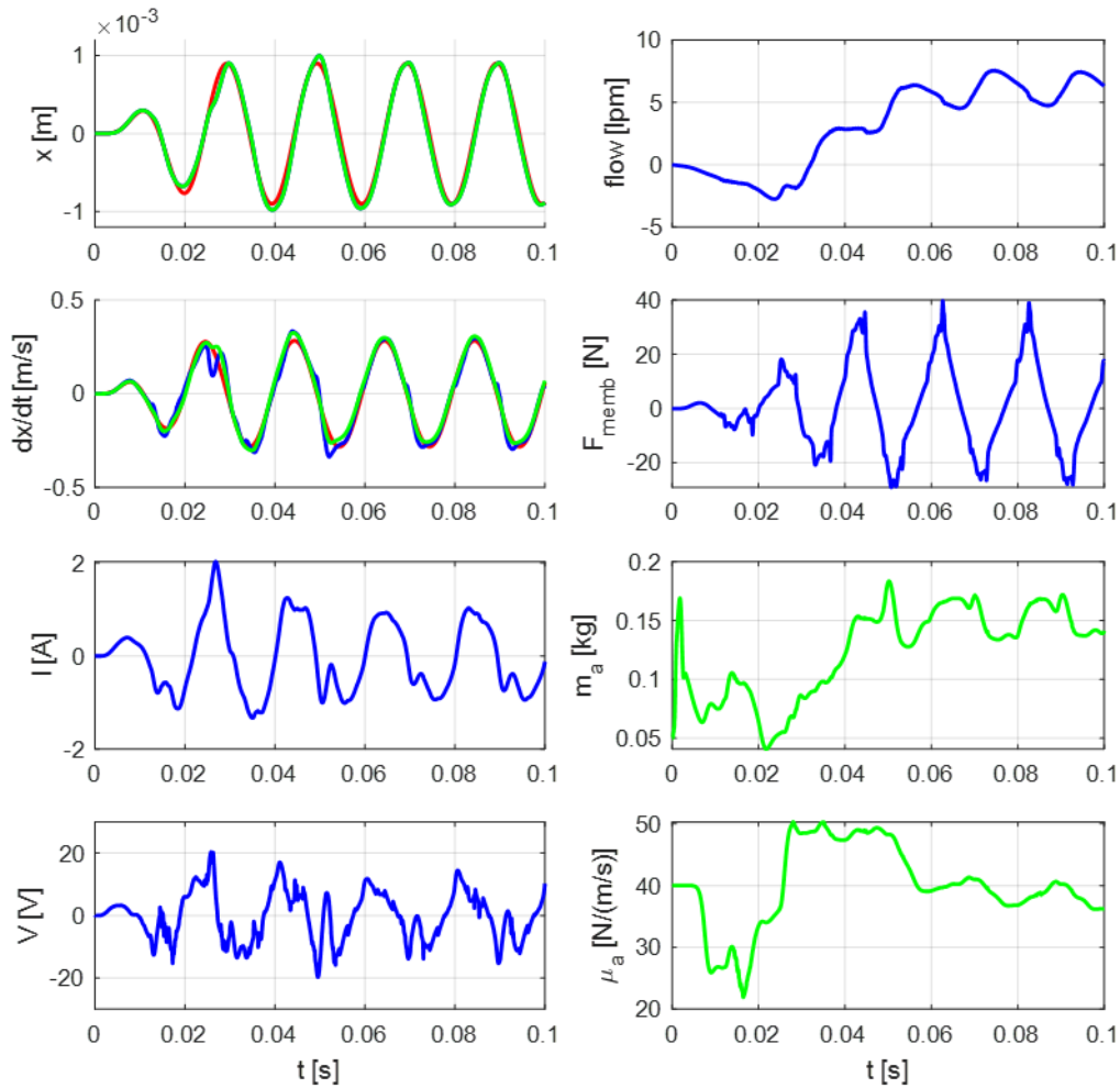
Figure 3.5 : Résultats de simulation de la commande LQ pour S_d = 0.9 \text{ mm} , f_d = 50 \text{ Hz} . En rouge : la trajectoire de référence ; en bleu : les signaux réels ; en vert : les signaux estimés
