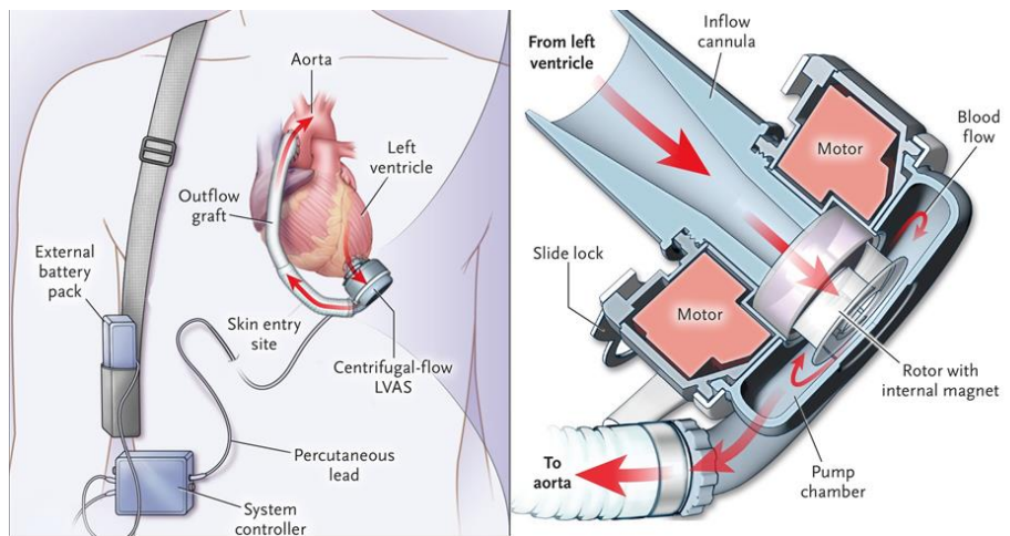
Figure 1.7 : Eléments de l'Heartmate 3 [27].
