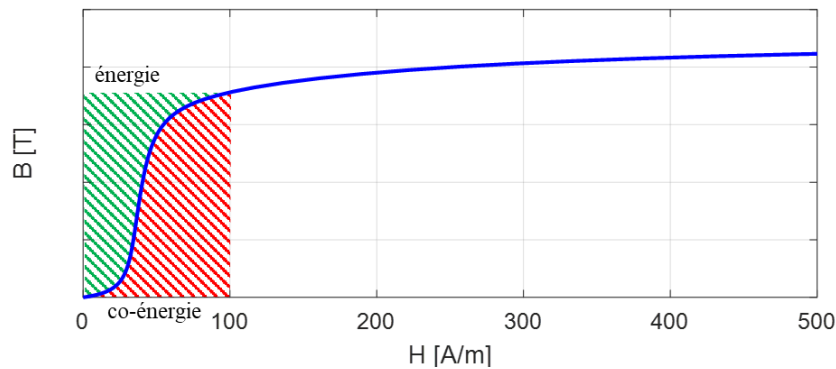
Figure 2.4 : courbe de magnétisation du cœur de l'actionneur 1 . La co-énergie correspond à la surface sous la courbe (hachures rouges) et l'énergie à la surface au-dessus de la courbe (hachures vertes)
