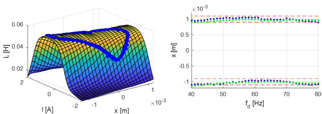
Figure 4.18 : Gauche : variation de l'inductance en fonction de la position et du courant, avec la trajectoire suivie par l'actionneur (bleu). Droite : Min et max de la position mesurée (bleu) et estimée (vert).
