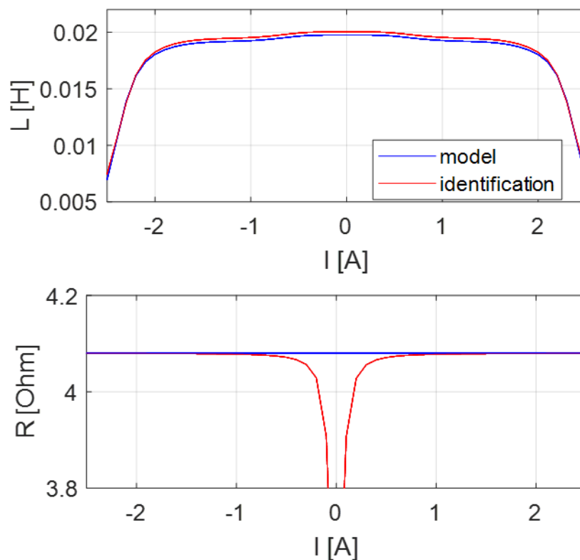
Figure 2.13 : estimation de l'inductance et de la résistance en fonction du courant pour x = 0
