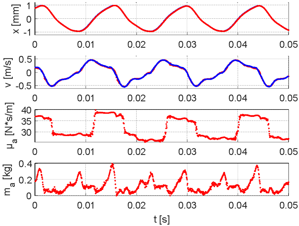
Figure 3.3 : estimation de la force de la membrane par l'EKF sur une co-simulation de la pompe. En bleu les signaux réels. En rouge les signaux estimés pour q_3 = 10^5 et q_4 = 100
