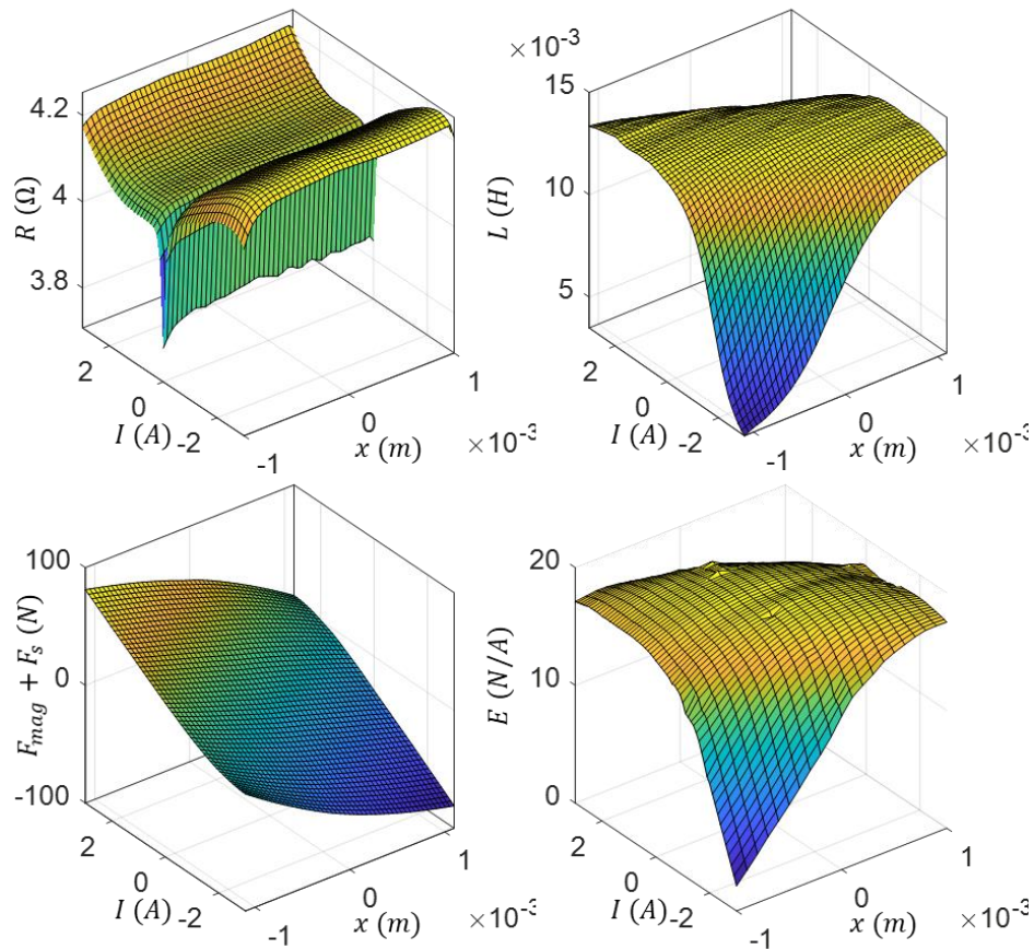
Figure 4.2 : résultats expérimentaux du test API
