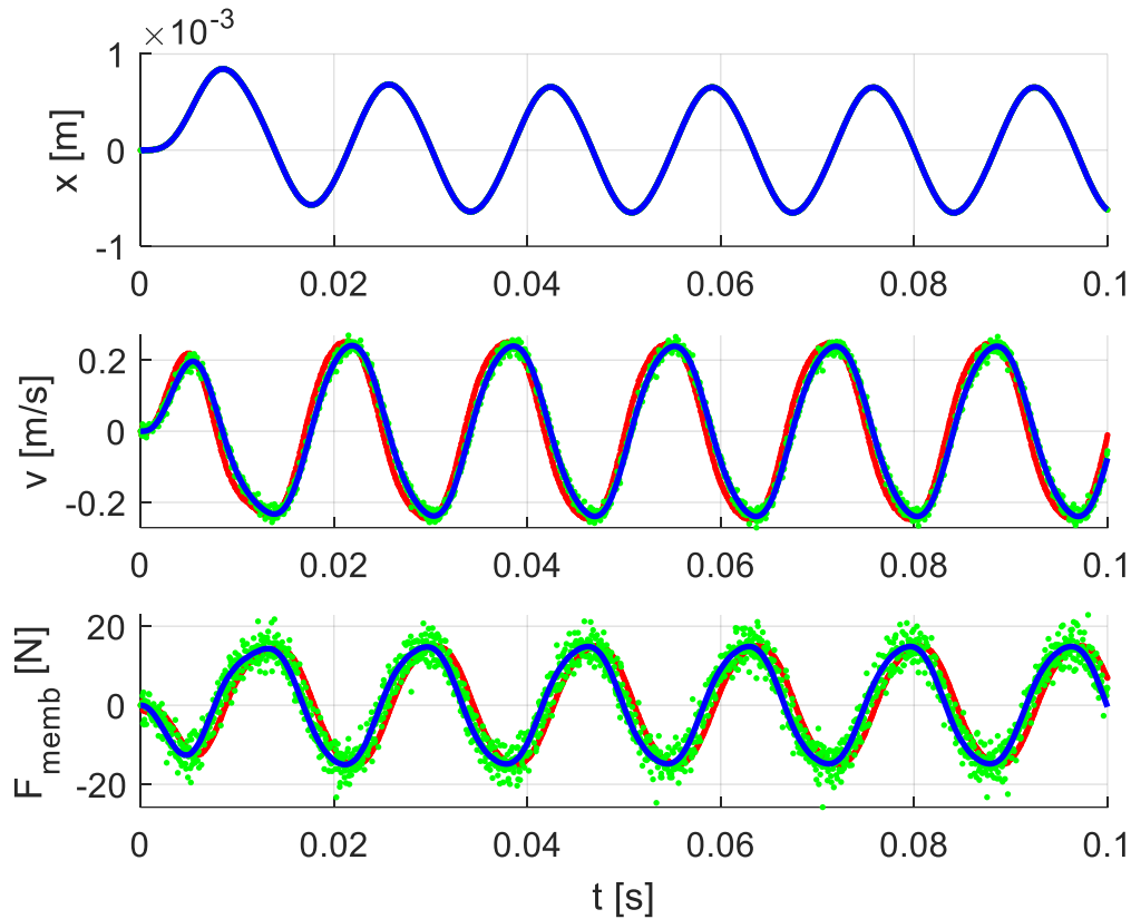
Figure 2.21: Résultats de réglage de l'estimateur de force. En bleu le signal réel, en rouge le signal estimé pour q_3 = 1 , en vert le signal estimé pour q_3 = 1000
