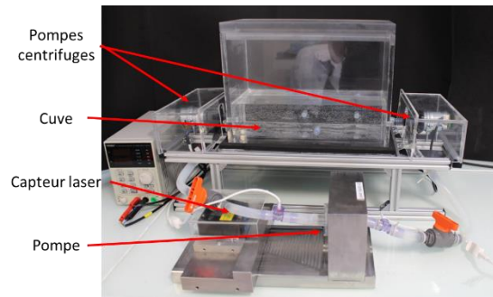
Figure 4.5 : Photographie du banc de test hydraulique
