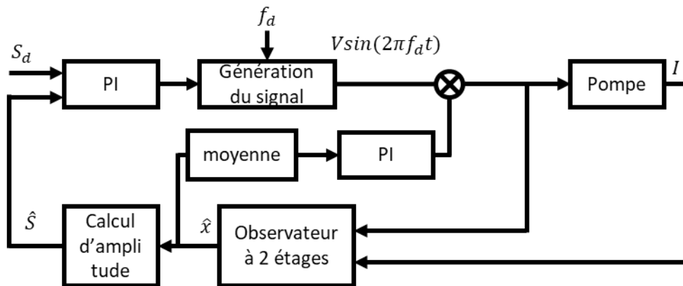
Figure 3.10 : schéma de la commande sans capteur
