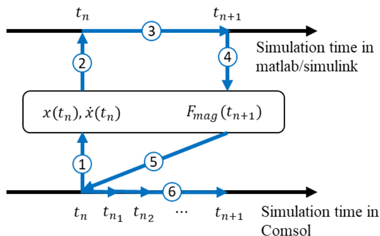
Figure 2.19: Gestion des pas de temps lors de la co-simulation.
