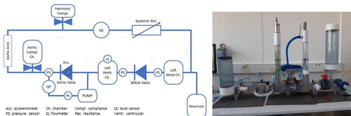
Figure 4.20 : Schéma et photographie du simulateur cardiovasculaire
