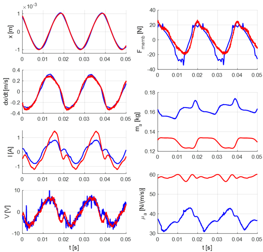
Figure 4.9 : Comparaison entre les résultats de simulation et les résultats expérimentaux sur un point de fonctionnement. Rouge : expérimental ; bleu : simulation. Pour la même pression, la différence de débit est de 25%
