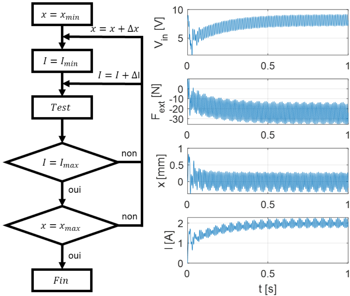
Figure 2.10 : procédure d'identification, et exemple des signaux d'entrées/sorties où les valeurs moyennes de position sont respectivement 0 mm et 2 A
