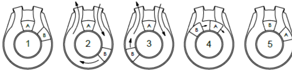
Figure 1.12 : principe de fonctionnement de la pompe TORVAD. Deux vérins (A,B) se déplacent dans la chambre de la pompe. Depuis la position de repos (1), un des vérins (B) se déplace dans la chambre en poussant le fluide vers la sortie pendant que le second empêche la recirculation du fluide (2-3). À la fin de la rotation, les deux vérins échangent leur rôle (4) avant le début d'un nouveau cycle (5) [49]
