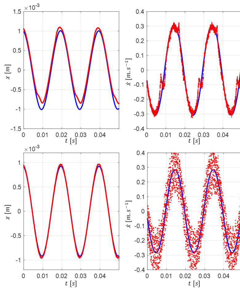
Figure 3.14 : Position et vitesse estimées avec la commande sans capteur en simulation pour un point d'opération haut. En haut, implémentation avec le dérivateur algébrique ; en bas, implémentation avec l'observateur de Levant. Bleu : signaux réels ; rouge : signaux estimés
