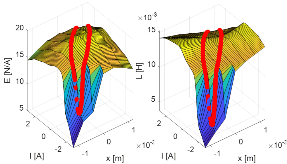
Figure 3.13 : Position et courant de l'actionneur superposés aux paramètres du modèle. Résultat de simulation
