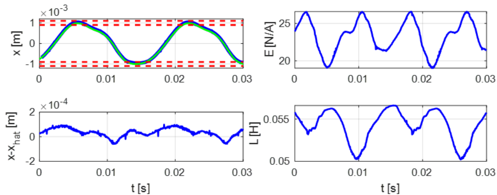
Figure 4.17 : A gauche : oscillations de la membrane ( f_d = 60 Hz). Bleu : mesure ; vert : estimation ; rouge : tolérances d'erreur sur l'amplitude. A droite : variation dans le temps des paramètres de l'actionneur
