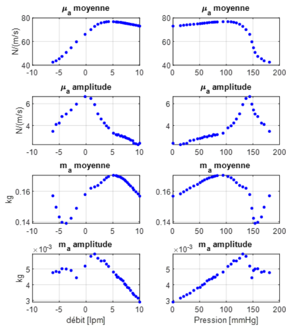
Figure 4.15 : Masse ajoutée et amortissement visqueux (moyennés, et amplitude des variations sur une oscillation) tracés en fonction de la pression et du débit.
