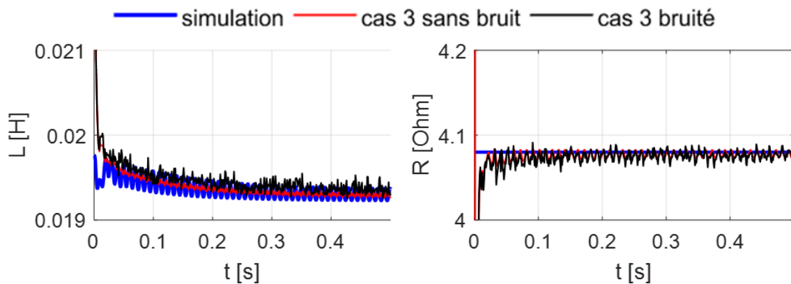
Figure 2.12 : Résultats de simulation du cas 3
