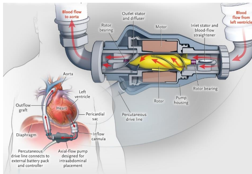
Figure 1.5: Éléments de l'Heartmate II [14].
