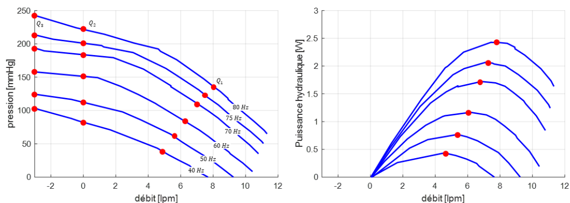
Figure 4.8 : courbes HQ et de puissance de la pompe évaluée. Les points rouges localisent les débits naturels, nuls et négatifs
