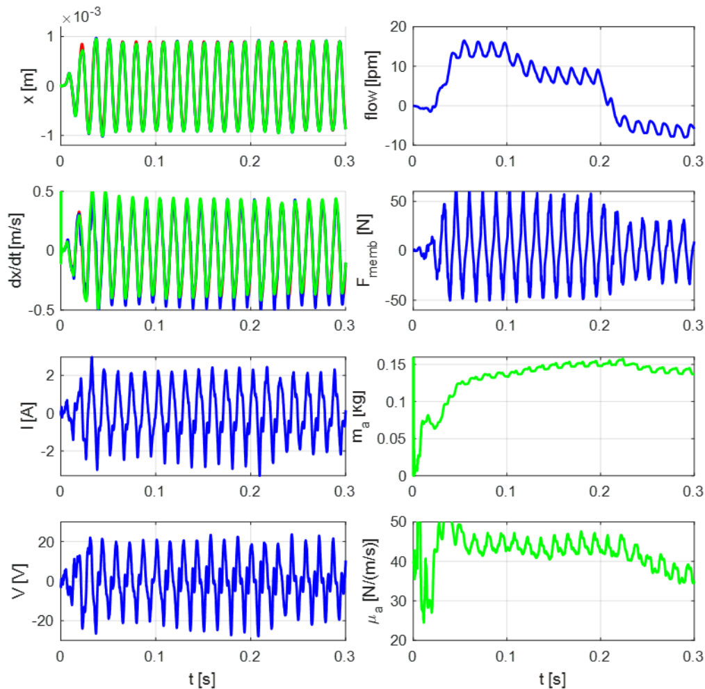
Figure 3.7 : Résultats de simulation de la commande LQ Lors de changements de pression (à 0.1s et 0.2s). En rouge : la trajectoire de référence ; en bleu : les signaux réels ; en vert : les signaux estimés
