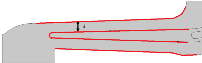
Figure 2.15: zone de la tête de pompe où le contact est implémenté
