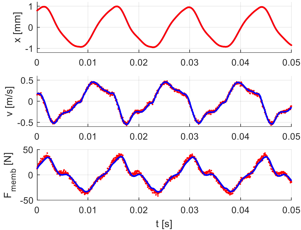
Figure 2.22: estimation de la force de la membrane par l'estimateur de force sur une co-simulation de la pompe. En bleu, les signaux réels. En rouge les signaux estimés. q_3 = 100
