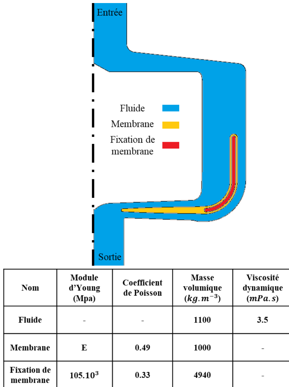
Figure 2.14: géométrie simplifiée de la pompe et données matériaux 1
