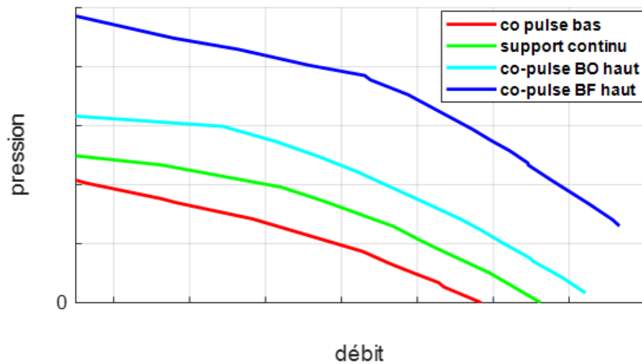
Figure 4.21 : courbes HQ des points d'opération utilisés pour les 3 modes d'assistances
