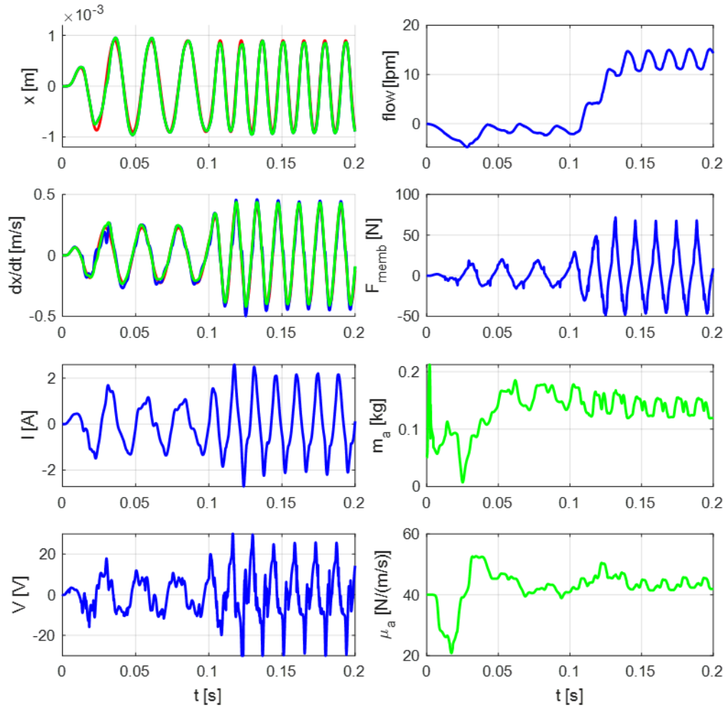
Figure 3.6 : Résultats de simulation de la commande LQ Lors d'une transition entre f_d = 40 Hz et f_d = 70 Hz.. En rouge : la trajectoire de référence ; en bleu : les signaux réels ; en vert : les signaux estimés
