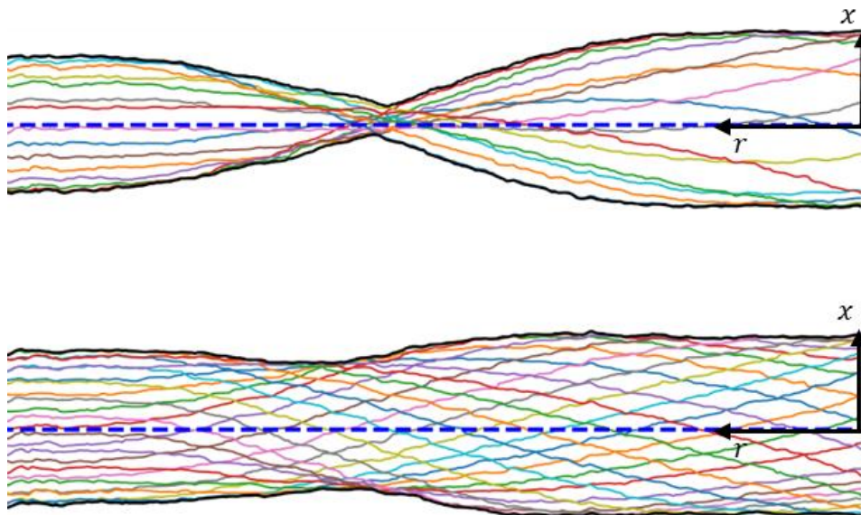
Figure 4.14 : mesures de la déformation de la membrane dans un mode stationnaire (haut) et dans un mode progressif (bas). La ligne pointillée bleue est la position de repos de la membrane. Les lignes noires sont les enveloppes hautes et basses des déformations
