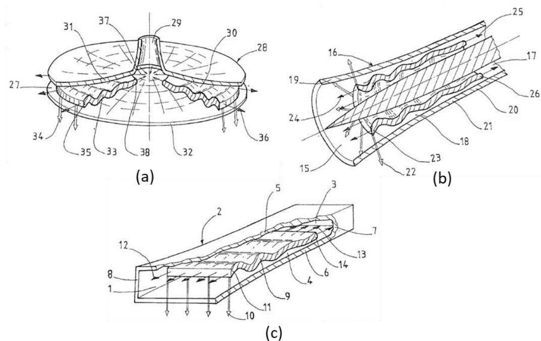
Figure 1.13: schémas de principe des pompes à membranes [51]. (a) : pompe discoïdale ; (b) pompe tubulaire ; (c) pompe rectangulaire
