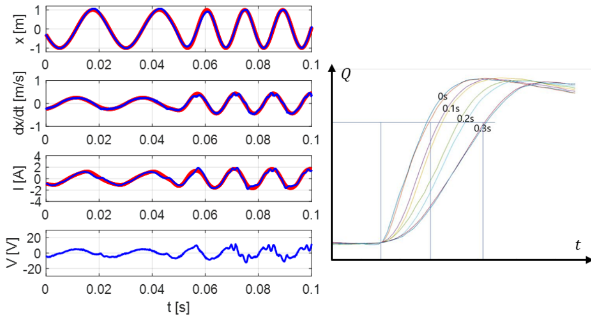
Figure 4.16 : transition entre la fréquence minimale et la fréquence maximale de la pompe en 0.01\text{ s} (gauche) et mesure du débit pour des temps de transition variables ( 0\text{s} , 0.1\text{s} , 0.2\text{s} , 0.3\text{s} ) (droite)
