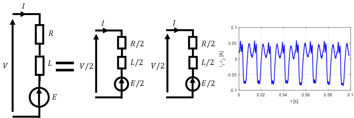
Figure 4.7 : Division de la tension en séparant les bobines (gauche), différence de courant entre les deux bobines lorsque la pompe fonctionne à puissance maximale (droite)
