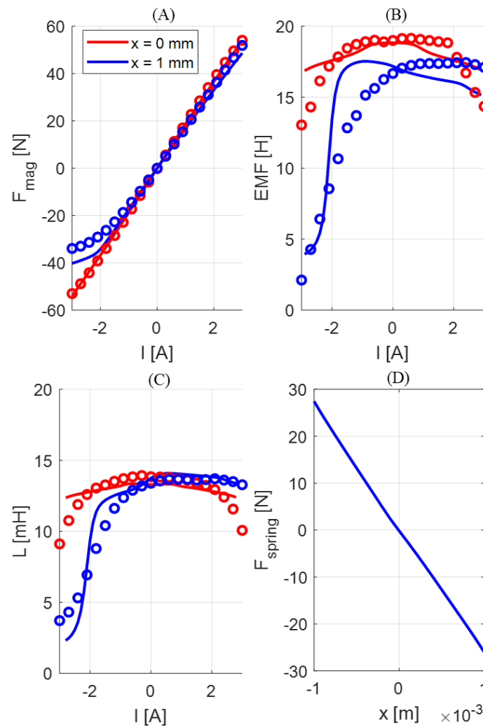
Figure 4.4: (A), (B) et (C) : comparaison entre le modèle construit par simulations EF (-) dont les paramètres sont corrigés par un coefficient (0.85) et les résultats du test API (o) pour deux positions de l'aimant. (C) : force de rappel des ressorts
