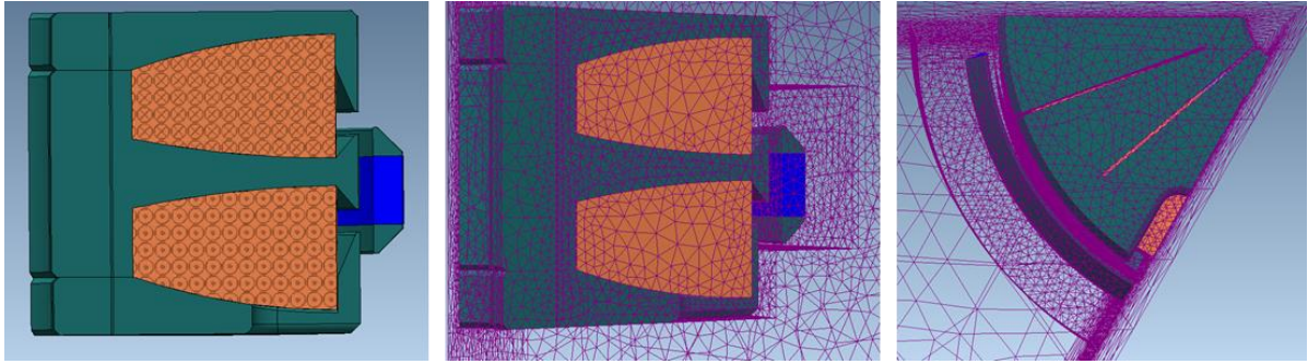
Figure 2.3 : géométrie de l'actionneur sous Magnet. Vue de profil, sans et avec maillage, vue du dessus avec maillage
