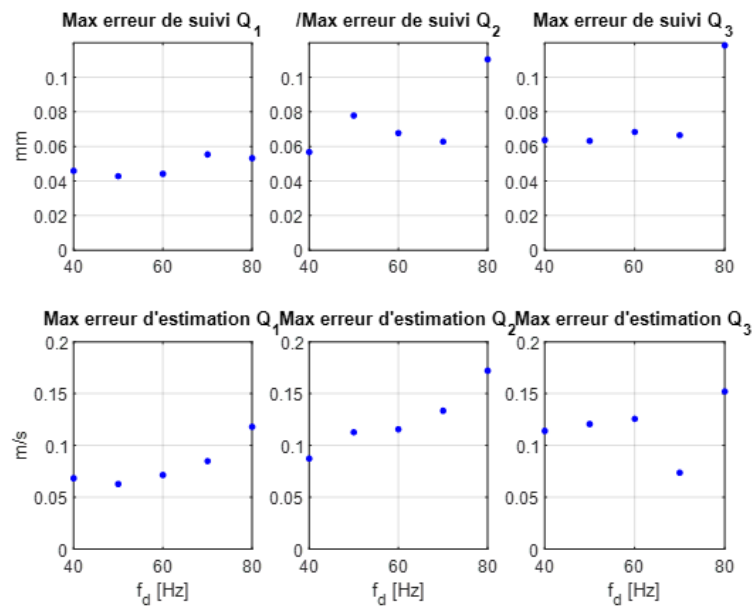
Figure 4.12 : Résumé des résultats du test de la commande. La limite d'utilisation de la pompe est de 80 Hz. Au-delà, le cahier des charges n'est plus respecté.
