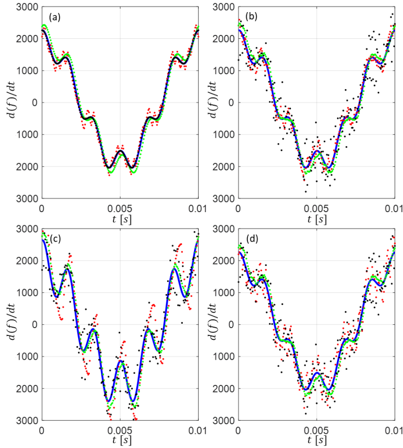
Figure 3.9 : comparaison des dérivateur de Levant (rouge), de Fliess (vert), de la différence finie (noir) par rapport au signal réel (bleu), dans le cas où (a) : le signal est non bruité ; (b) le signal est bruité ; (c) l'amplitude est légèrement augmentée ; (d) la valeur de C est doublée lors de l'élaboration de l'observateur de Levant.
