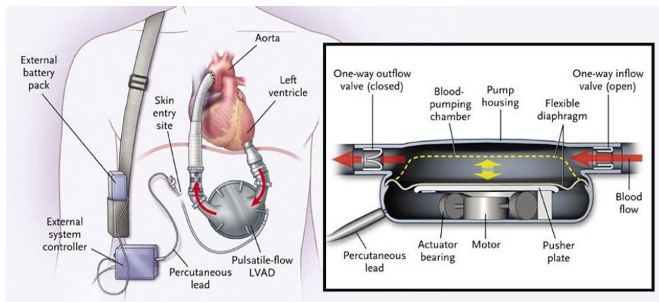
Figure 1.4: Eléments de l'Heartmate 1 [6].
