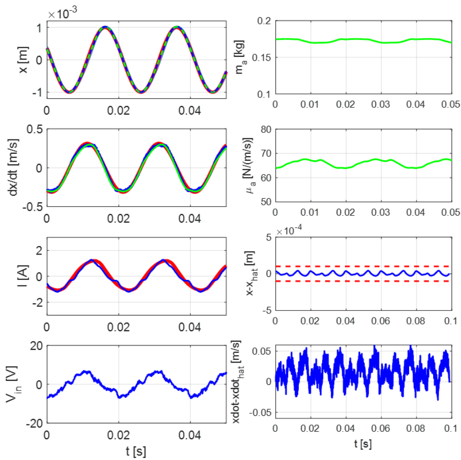
Figure 4.11 : Résultats expérimentaux pour un point de fonctionnement de la pompe. Rouge : trajectoire de référence ; vert : estimation ; bleu : mesure
