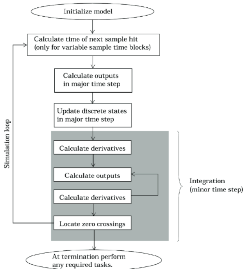
Figure 2.20: schéma de fonctionnement d'une fonction S sous Simulink [84]
