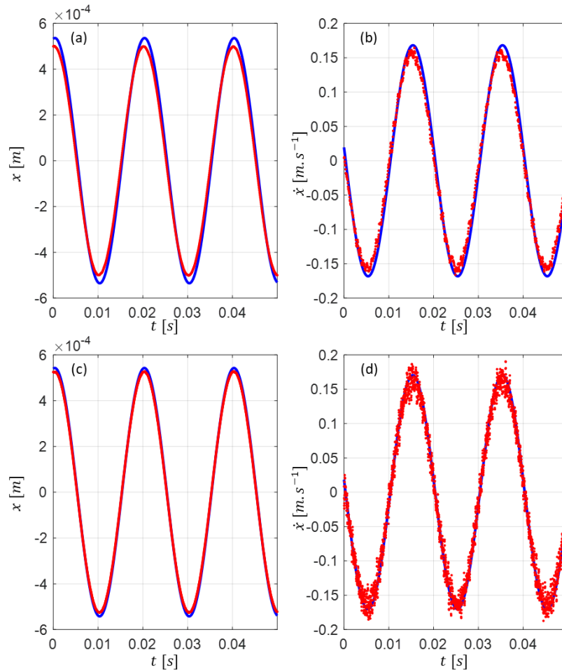
Figure 3.12 : Position et vitesse estimées avec la commande sans capteur en simulation, dans le cas où le 1 er étage est implémenté avec le dérivateur algébrique. (a) et (b) sont effectuées avec T_e = 50 \mu s , (c) et (d) avec T_e = 20 \mu s . Bleu : signaux réels ; rouge : signaux estimés.
