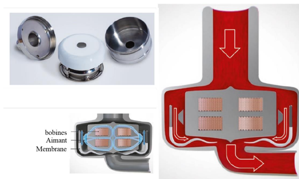
Figure 1.15: photographie et schémas de principe de la pompe cardiaque à membrane ondulante
