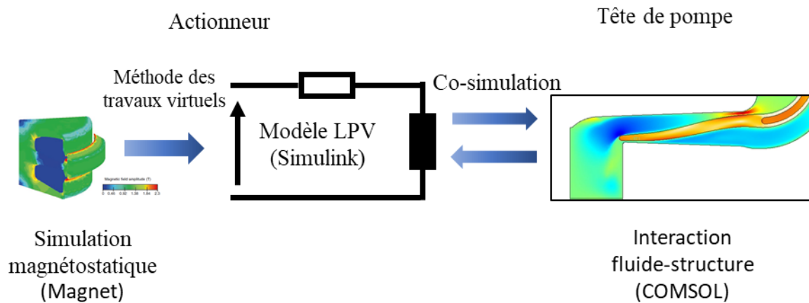
Figure 2.1 : Simulation complète de la pompe
