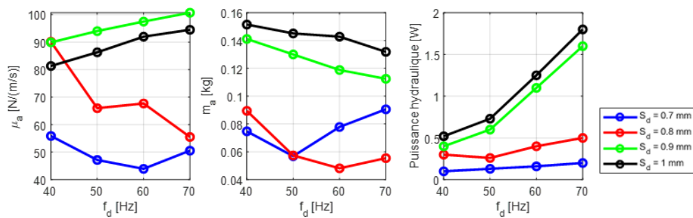
Figure 4.13 : Mesures de m_a , \mu_a et de la puissance hydraulique suivant la fréquence d'oscillation. A S_d = 0.7 mm, la déformation est non propulsive sur toute la plage de fréquence. Pour S_d = 0.8 mm la déformation est propulsive à 40 Hz et devient non propulsive à partir de 50 Hz. Pour des amplitudes supérieures à 0.9 mm la déformation est uniquement propulsive sur la plage de fréquence.
