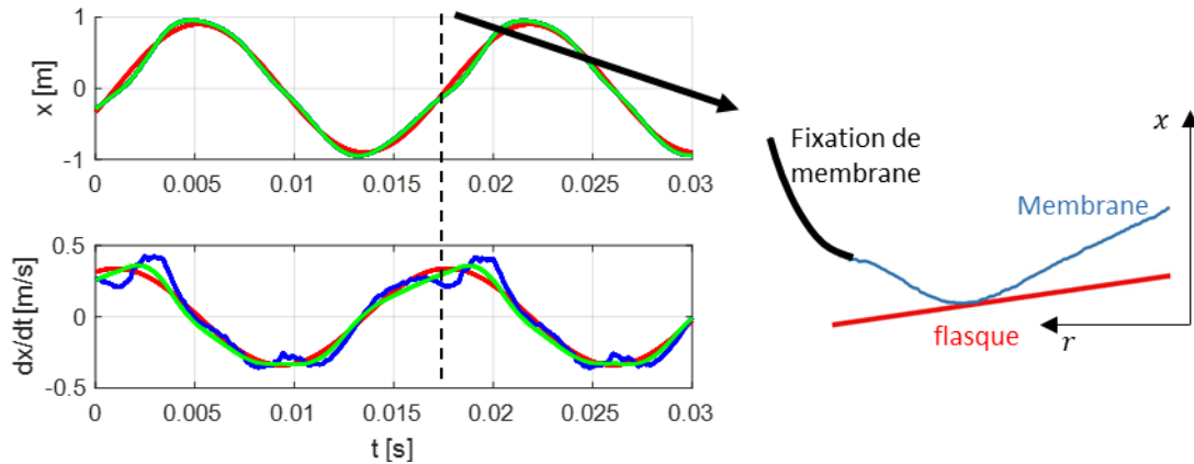
Figure 4.10 : Gauche : position et vitesse de la membrane. Rouge : trajectoire de référence ; Bleu : mesure ; Vert : estimation. Droite : mesure de la déformation de la membrane au moment où celle-ci entre en contact avec la flasque. Un contact brusque entraîne une chute rapide de la vitesse qui n'est pas estimée par l'EKF.
