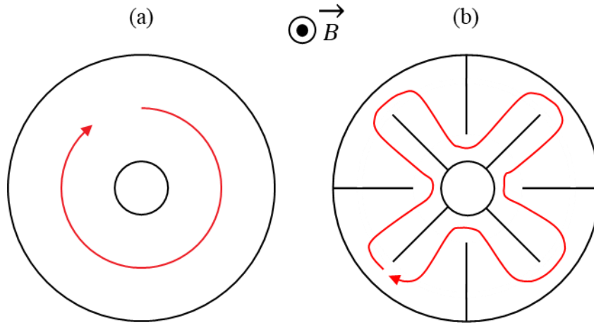
Figure 2.9 : circulation des courants de Foucault. (a) le noyau ferromagnétique est plein. (b) le noyau est entrecoupé de fentes.
