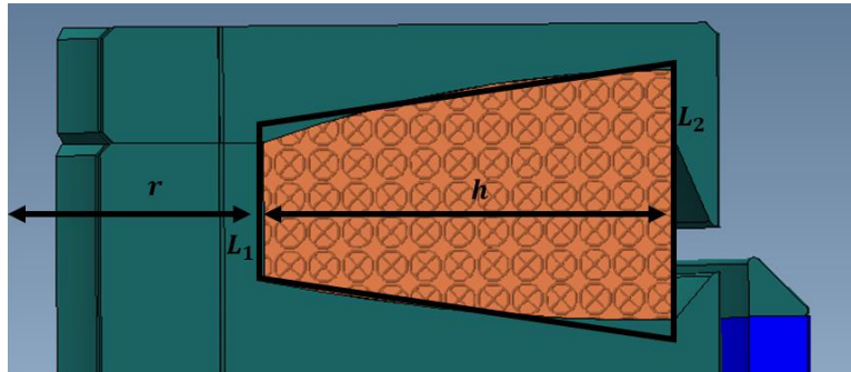
Figure 2.6 : Simplification de la géométrie des bobines
