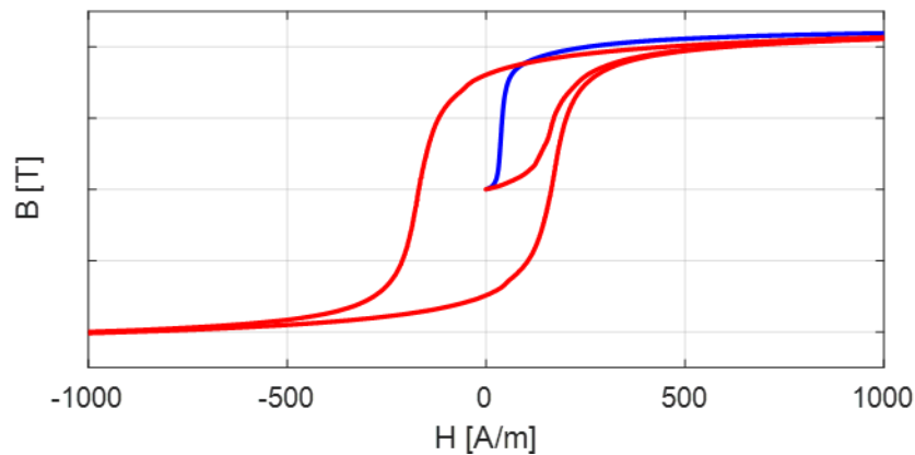
Figure 4.3 : courbe B-H du modèle (bleu) et courbe expérimentale (rouge).
