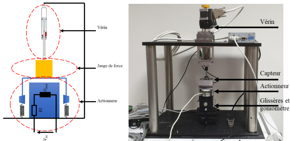
Figure 4.1: Schéma de principe et photographie du banc de test API
