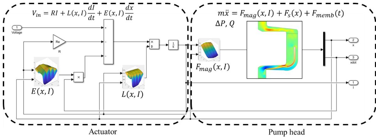
Figure 2.18: schéma de la co-simulation. La partie électromécanique est modélisée via Matlab/Simulink. La tête de pompe est modélisée par le logiciel de simulation EF COMSOL.
