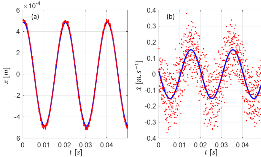
Figure 3.11 : position (a) et vitesse (b) estimées avec la commande sans capteur en simulation dans le cas où le 1 er étage est implémenté avec l'observateur de Levant. Bleu : signaux réels ; rouge : signaux estimés.
