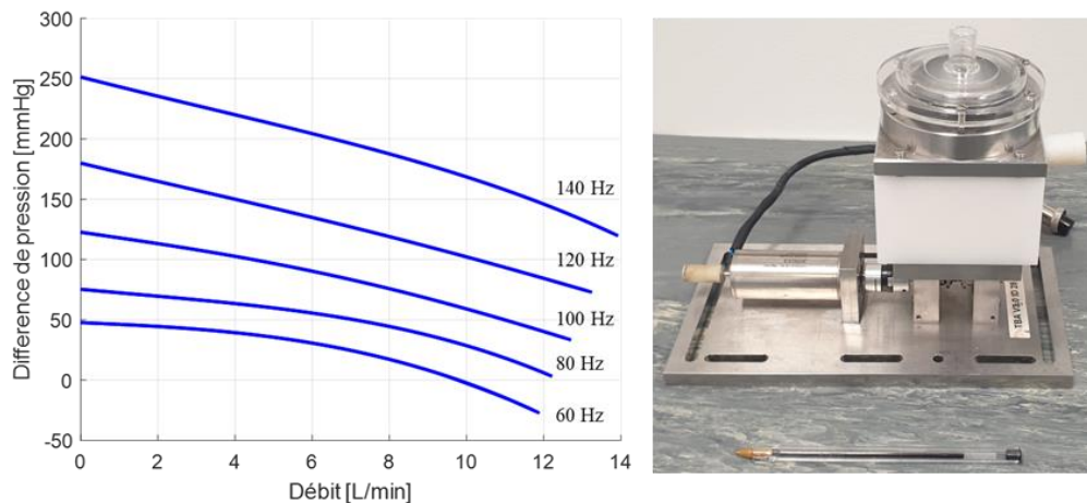
Figure 1.16: Courbes caractéristiques d'une pompe actionnée 1 par un moteur électrique, et photographie de la pompe.
