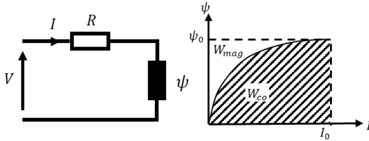
Figure 2.5 : circuit magnétique simple (à gauche) et courbe caractéristique \psi - I du circuit magnétique (droite) [65]
