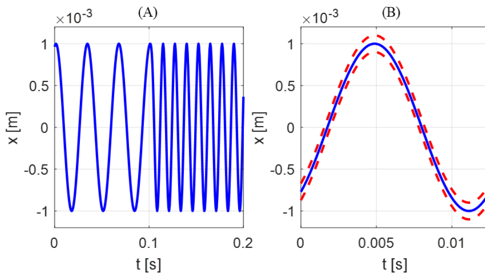
Figure 1.19 : Exemple de trajectoire de référence désirée. (A) : changement de fréquence à 0.1 \text{ s} ; (B) : trajectoire désirée (bleu) et limite maximale pour l'erreur de suivi (rouge) de 0.1 \text{ mm}
