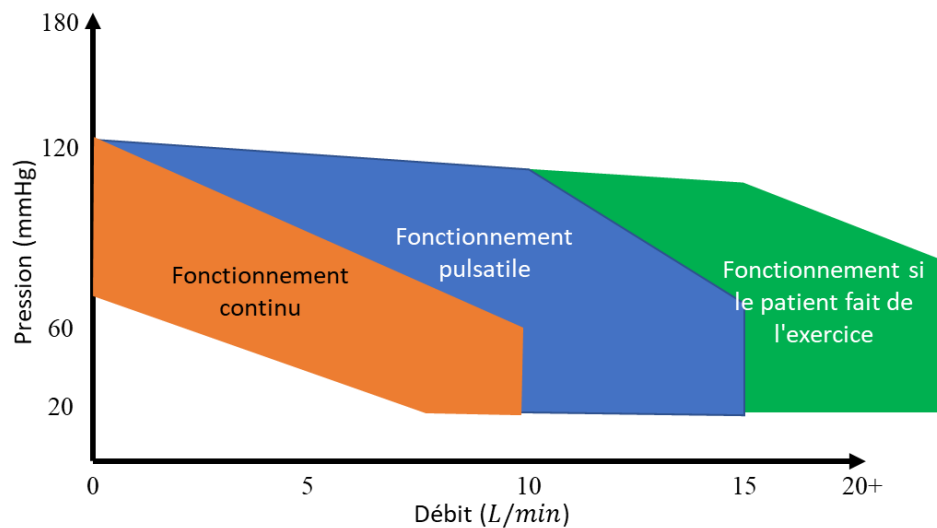
Figure 1.17 : zones de fonctionnement de la pompe suivant le mode de fonctionnement (continu, pulsatile, si le patient doit réaliser un exercice physique).
