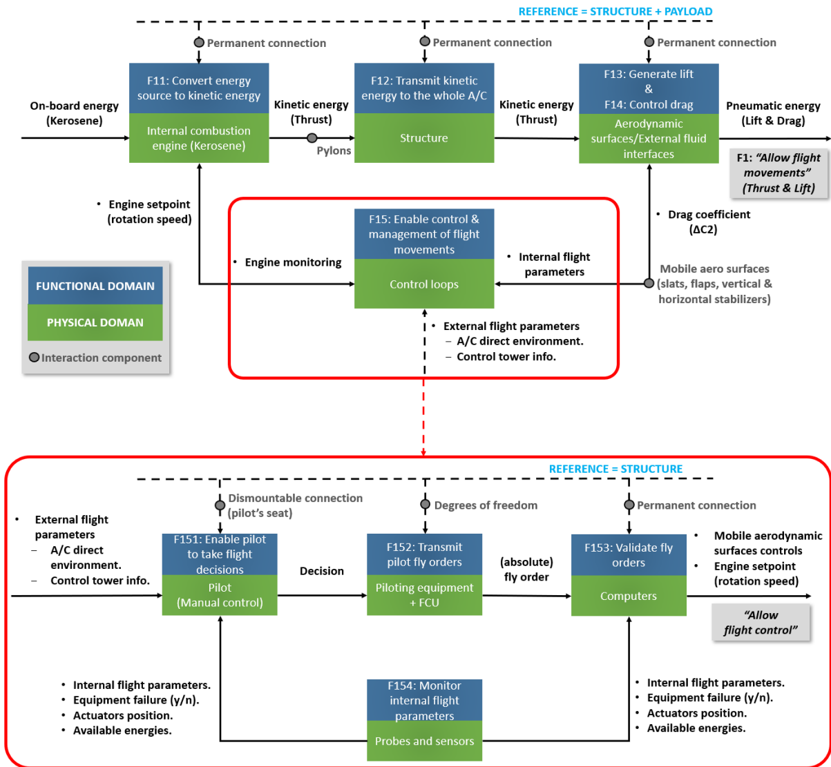
Fig. 44 Illustration du mécanisme de description de l'entité « Contrôle » d'un modèle CTOC.
