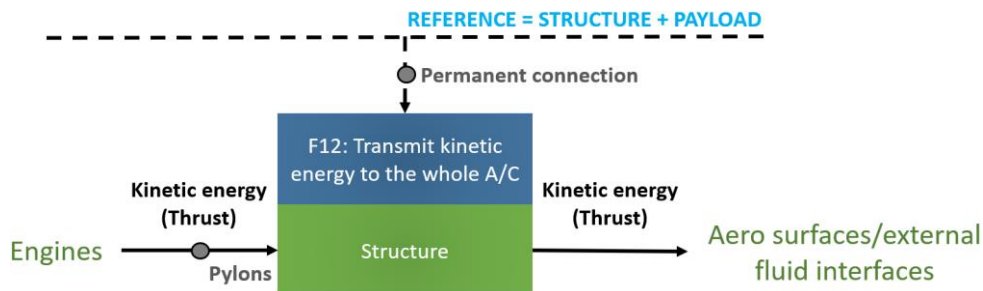
Fig. 45 Modèle boîte noire du composant « Structure » isolé du modèle CTOC de tête.
