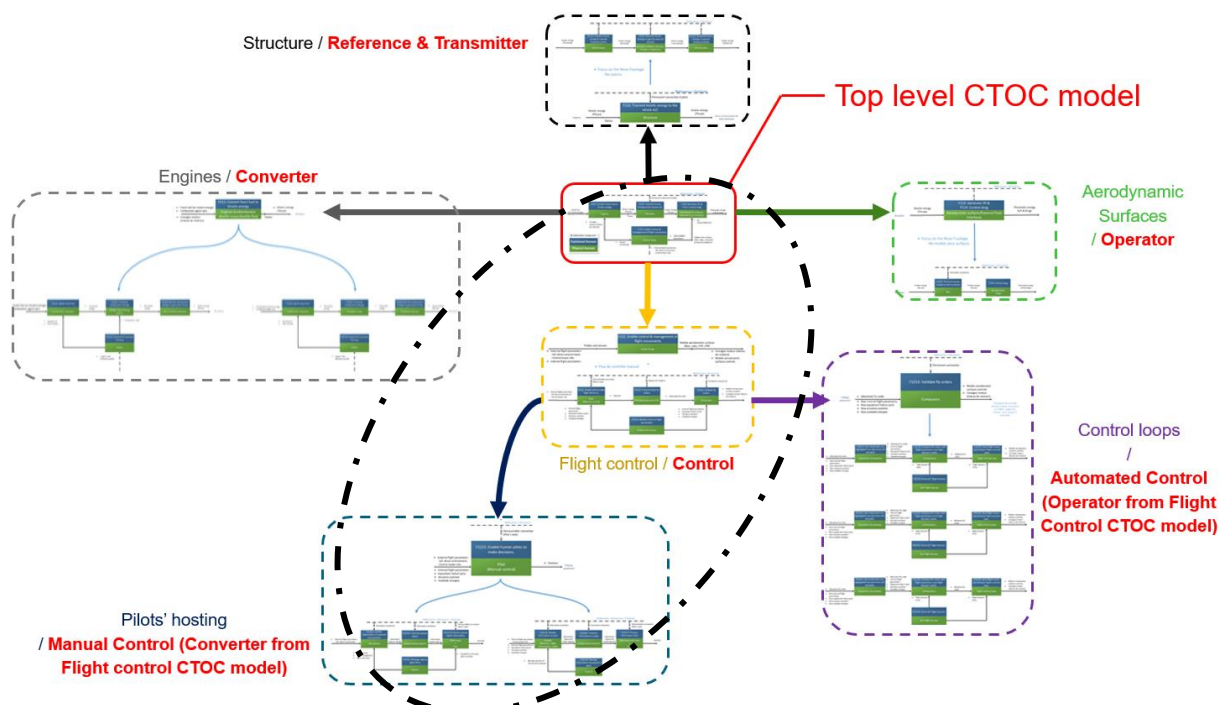
Fig. 74 Vue globale de la représentation CTOC appliquée au produit avion.
