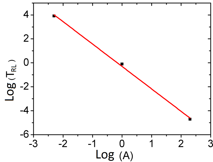
FIGURE 3.9. Courbe représentant la variation du temps de rupture linéaire T_{RL} en fonction de la constante d'Hamaker adimensionnée A .
