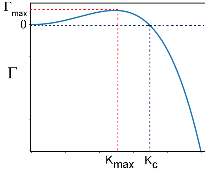
FIGURE 2.6. Courbe théorique du taux d'accroissement \Gamma en fonction de la pulsation spatiale K . Il est possible de distinguer le mode le plus rapide K_{\max} qui correspond à \Gamma_{\max} et le mode critique K_c pour lequel \Gamma = 0 .
