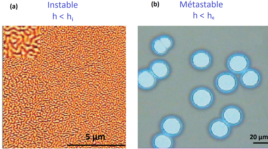
FIGURE 2.3. (a) Image AFM du démoillage spinodal d'un film de PS (b) Micrographie optique montrant la formation de trous dans un film de PS. Figure adaptée de Damman et al. [23] .
