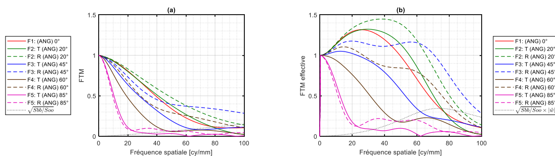
Figure 4.7 (a) FTM et (b) FTM effective (pour un RSB à 34 dB) du fish-eye conventionnel.
