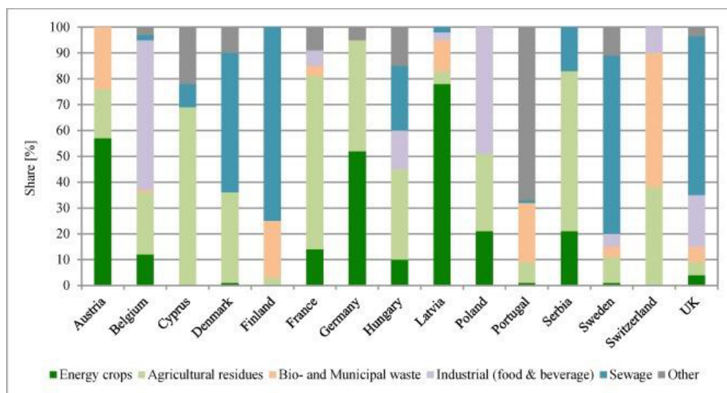
Figure I.1 – Intrants utilisés pour la méthanisation dans différents pays européens, en 2015. La figure est issue de Scarlat et al. (2018).
