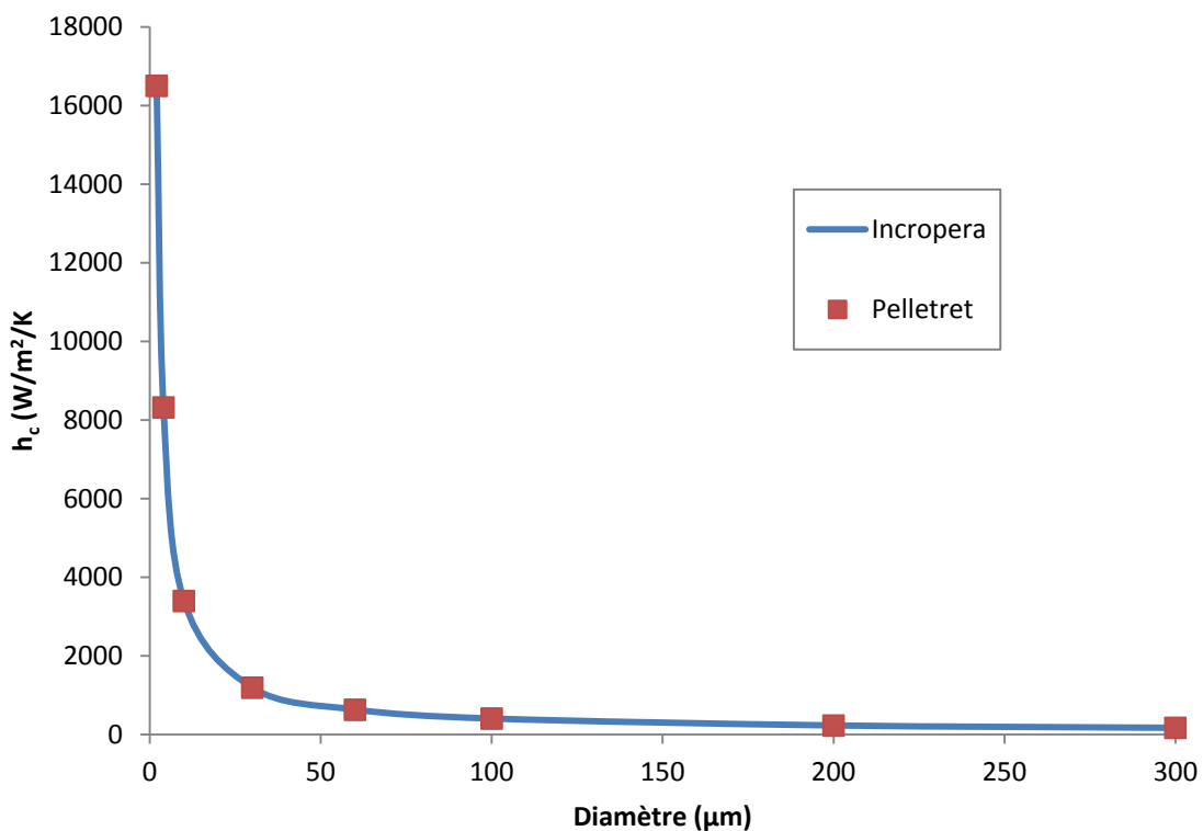
Figure 20: Coefficient d'échange de chaleur par convection entre une gouttelette d'huile et le gaz en fonction du diamètre de la gouttelette d'huile.
