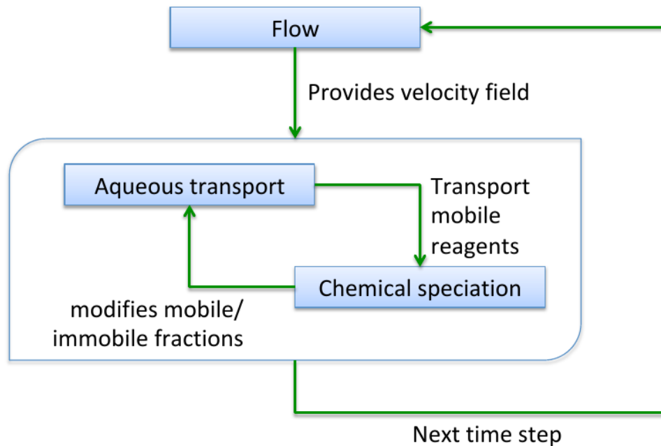
FIGURE 3.1 – Schéma de résolution du modèle de transport réactif par le logiciel Hytec, extrait de Lagneau et al. [2018]. Il illustre la résolution séquentielle selon le temps du modèle avec un certain nombre d'itérations pour faire converger les résultats du transport et de la chimie
