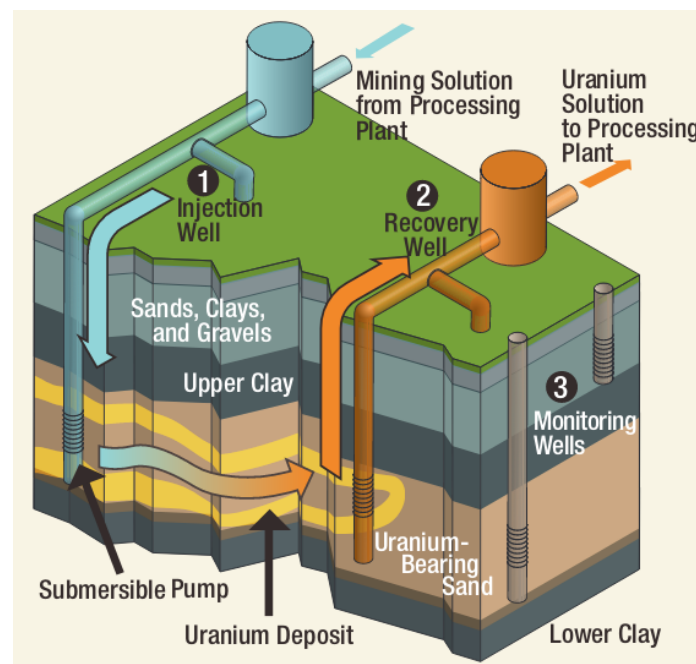
FIGURE 1 – Schéma d'une exploitation par ISR, d'après Ivonne Couret [2013]
