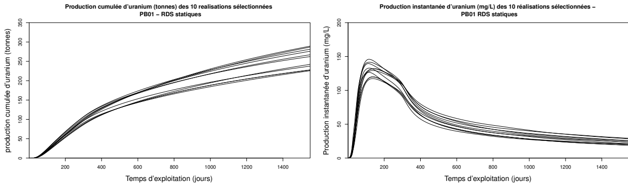
FIGURE 6.4 – Productions d'uranium cumulées et instantanées des 10 réalisations sélectionnées pour le bloc PB01 avec les descripteurs statiques
