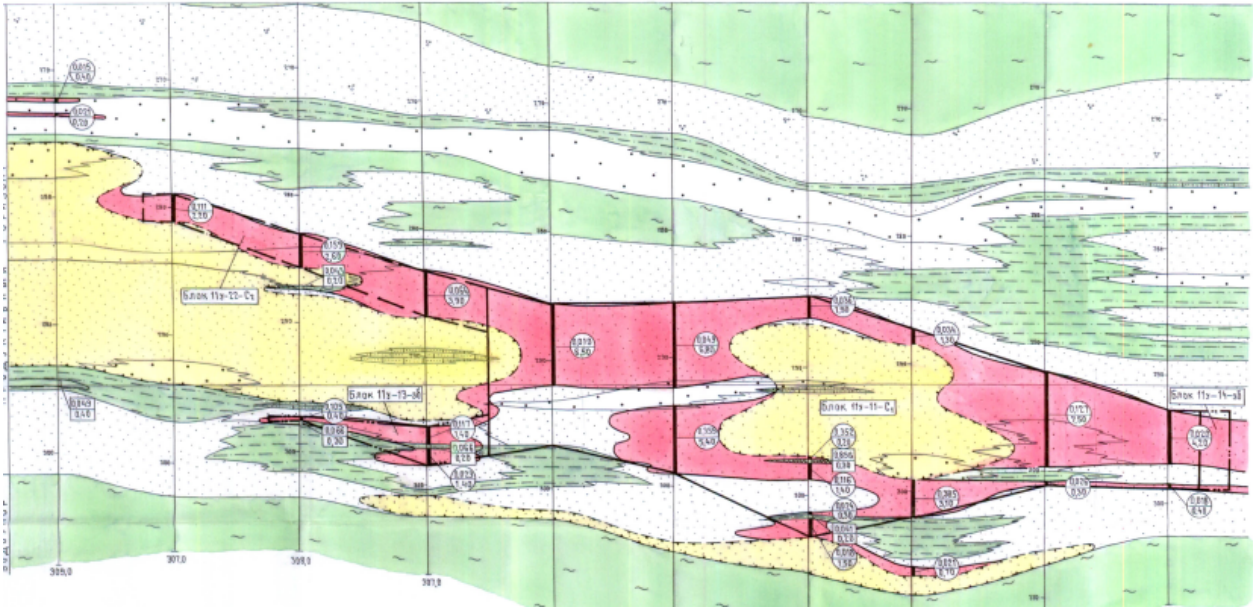
FIGURE 2.2 – Exemple de coupe géologique d'un roll-front [Langlais et al., 2013]. La zone rouge correspond aux sables perméables contenant de l'uranium minéralisé. Celle en jaune correspond aux sables oxydés du réservoir, la roche réduite blanche correspond aux sables stériles, et en vert sont représentées les argiles (dans tous les cas stériles)
