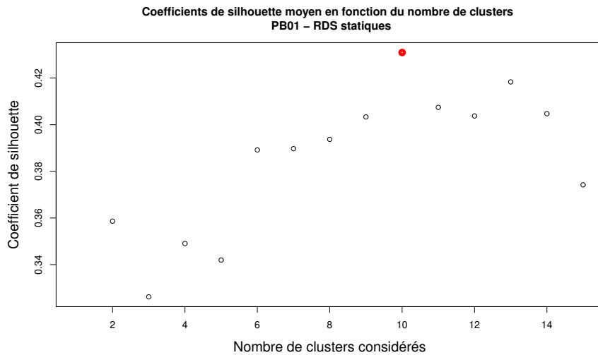
FIGURE 6.2 – Silhouettes moyennes des réalisations en fonction du nombre de clusters après le partitionnement des réalisations de PB01 avec les descripteurs statiques. Dans ce cas ci, on choisira de sélectionner 10 réalisations représentatives
