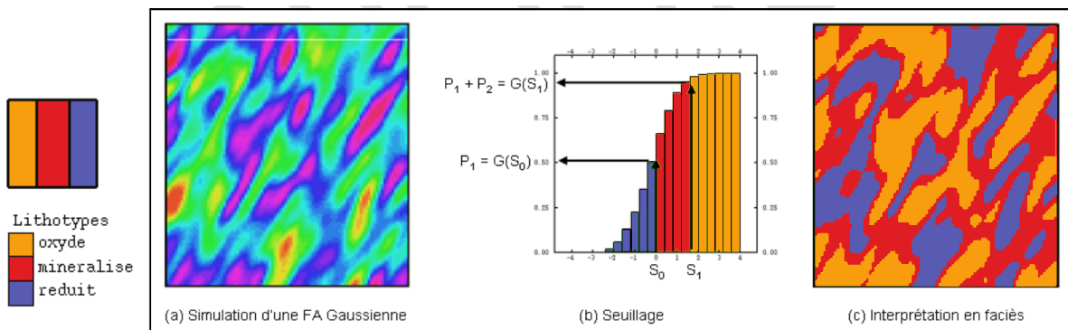
FIGURE 2.5 – Présentation du principe des simulations gaussiennes tronquées sur le faciès OMR, d'après [Garnier, 2014]. La règle de troncature du faciès oxydé-minéralisé-réduit est présentée à gauche. La figure (a) présente le résultat d'une simulation de la fonction aléatoire gaussienne sous-jacente de la propriété, (b) montre les deux seuils de la gaussienne pour respecter les proportions de faciès et la règle de troncature, et enfin, (c) montre le résultat de l'application de ce seuil à la simulation de la gaussienne.
