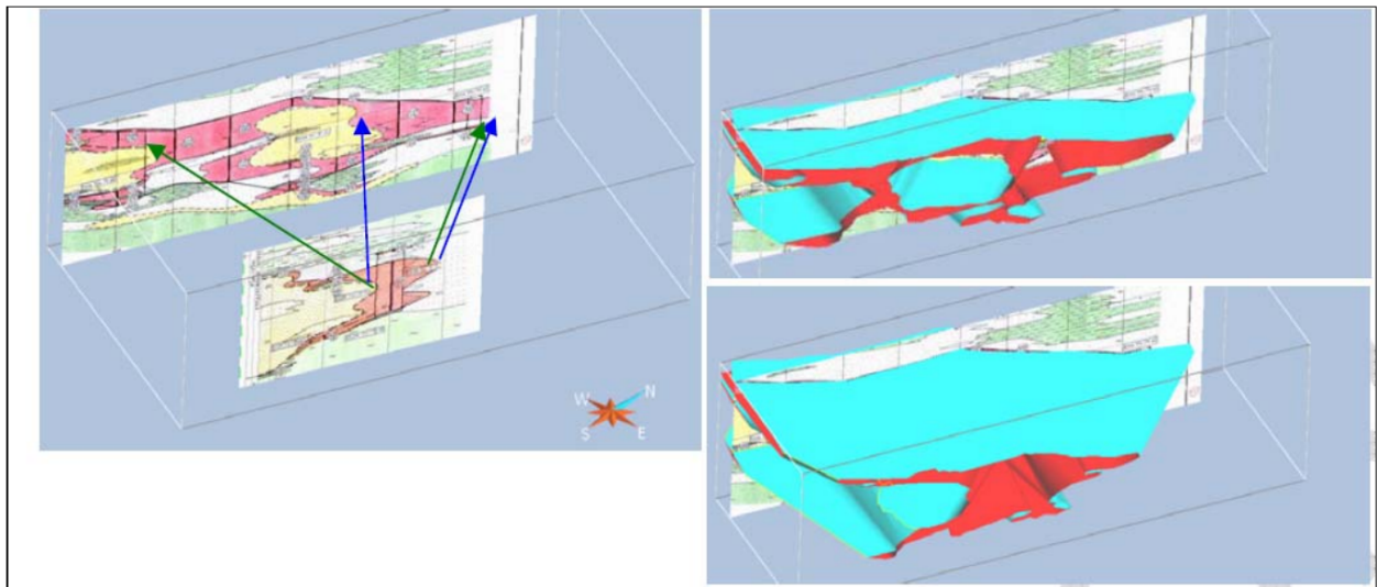
FIGURE 2.3 – Interpolation d'enveloppe minéralisée à partir de coupes géologiques interprétées, d'après Langlais et al. [2013]
