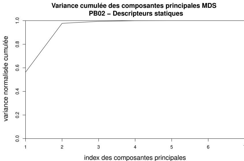
FIGURE 6.6 – Variance cumulée portée par les composantes principales du MDS sur les descripteurs statiques des réalisations du bloc PB02. Les deux premières composantes expliquent 97.7% de la variance des réalisations
