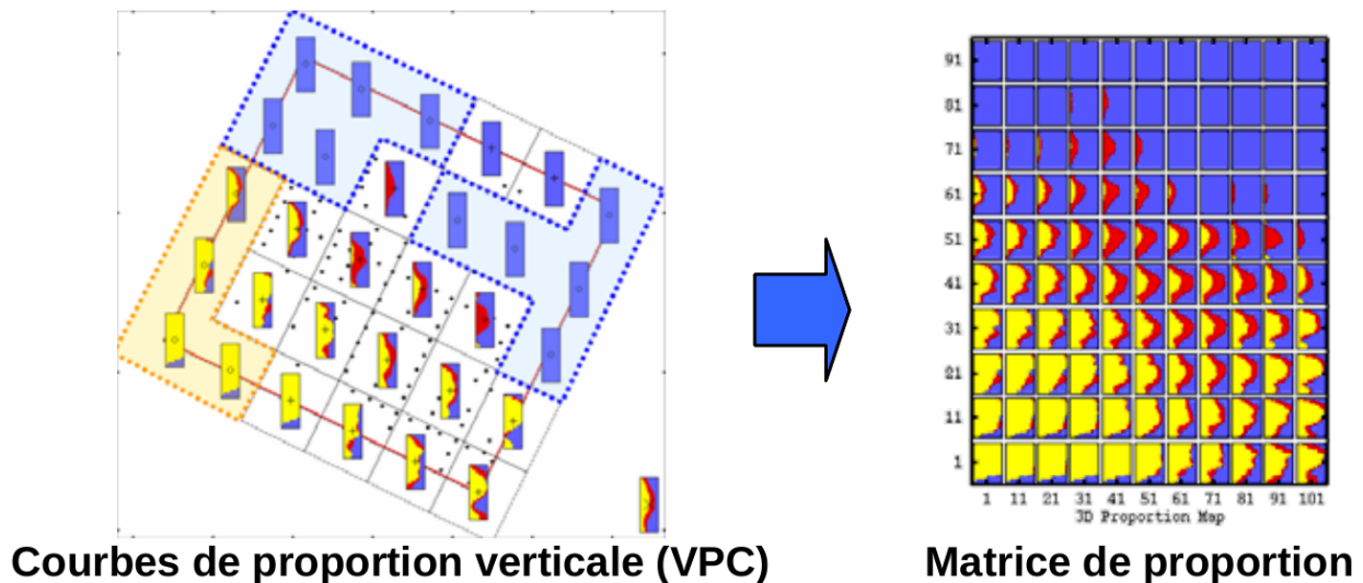
FIGURE 2.6 – Passage des courbes de proportions verticales à la matrice de proportions, d'après [Garnier, 2014]. Les courbes de proportions verticales dans les mailles entourées en pointillés correspondent à des zones où aucun forage n'a été effectué. Ces courbes de proportions verticales sont rajoutées par l'utilisateur en fonction de l'interprétation géologique des données
