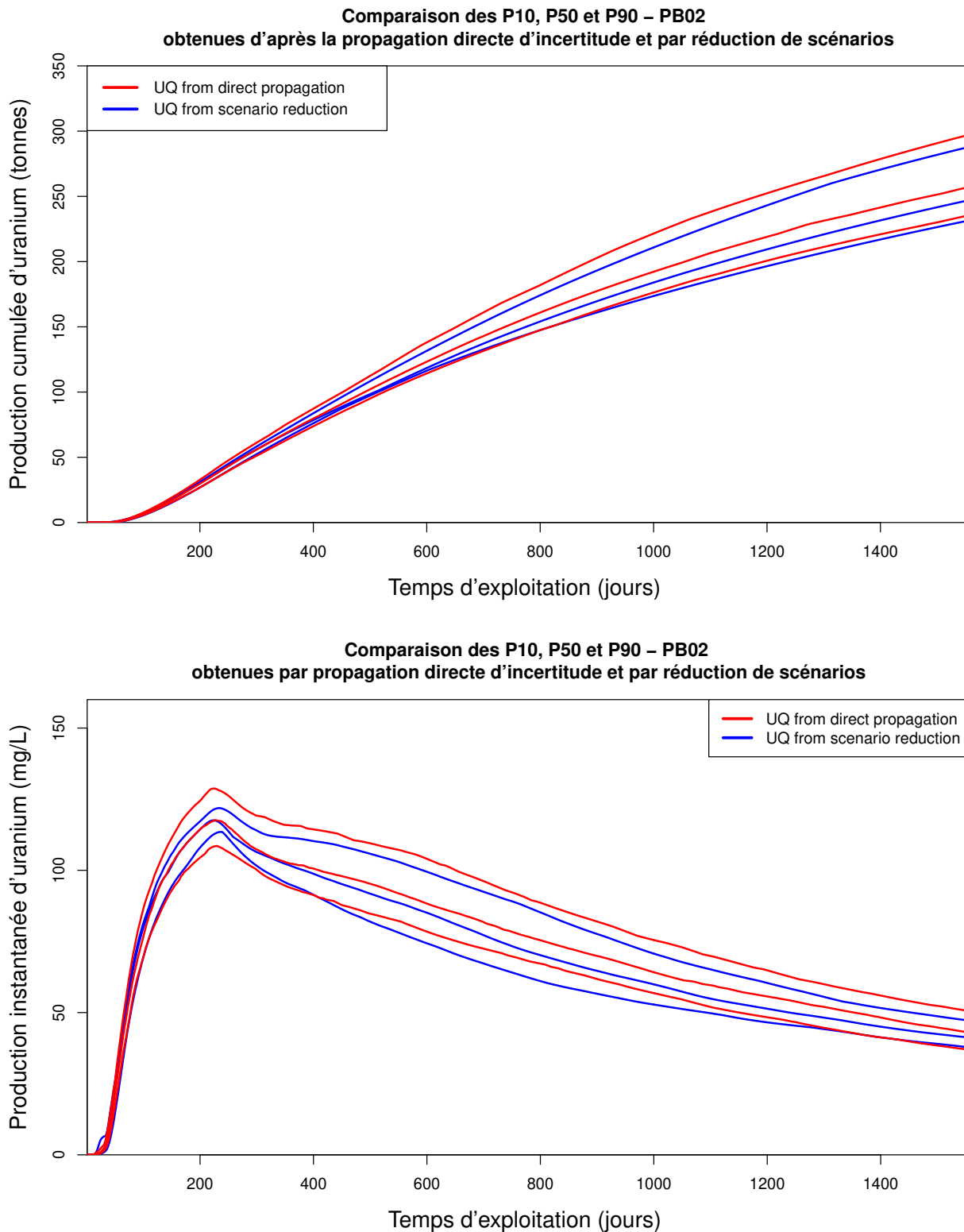
FIGURE 7.7 – Comparaison de la quantification d'incertitude de référence et celle approchée par la réduction de scénarios utilisant les descripteurs statiques et de récupération de traçeurs sur PB02. On observe sur le premier graphe, que les courbes P 50 et P 90 approchées ne s'ajustent pas du tout aux courbes de références. Sur le deuxième graphe, l'enveloppe approchée par les courbes obtenues par réduction de scénarios sous-estime l'enveloppe des courbes de référence
