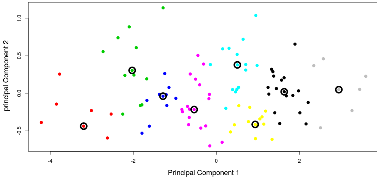
FIGURE 4.3 – Exemple de résultat de l’algorithme des k -médoides pour k = 8 . Les axes sont définis par les deux premières composantes principales de l’espace réduit des descripteurs. Chaque point correspond à une réalisation, chaque couleur à une famille de la classification, et chaque réalisation entourée, à la réalisation représentative de sa famille (le médoides)
