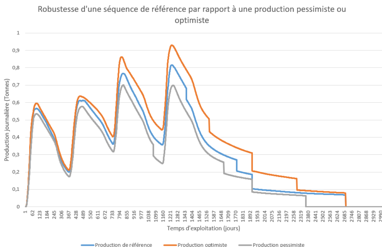
FIGURE 9.4 – Comparaison des productions de la zone dans les cas pessimiste, optimiste et de référence avec les mêmes dates d'ouverture imposées
