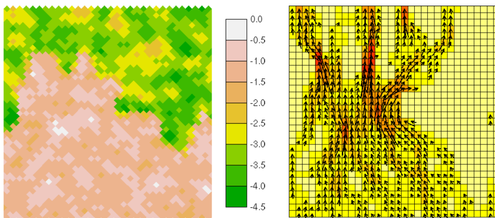
FIGURE 2 – La répartition spatiale hétérogène des propriétés impacte les résultats des simulations de transport réactif. Exemple d'un champ de perméabilité contrôlant les écoulements dans le réservoir, et donc l'apport en réactif au cours de la simulation, [De Lucia et al., 2011]. Le champ de perméabilité est présenté à gauche avec l'échelle logarithmique au centre. À droite sont représentés les vecteurs tangent à l'écoulement dans le milieu
