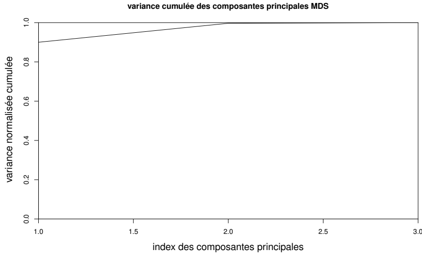
FIGURE 8.6 – Variance cumulée portée par les composantes principales des descripteurs du minéral traceur cinétique sur PB02. Les deux premières composantes expliquent plus de 99% de la variance des données
