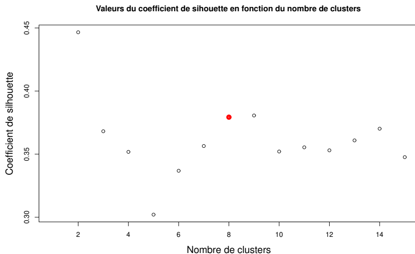
FIGURE 7.6 – Silhouettes moyennes des réalisations en fonction du nombre de clusters après le partitionnement des réalisations de PB02 avec les descripteurs statiques et traceurs. Dans ce cas ci, on choisira de sélectionner 8 réalisations représentatives
