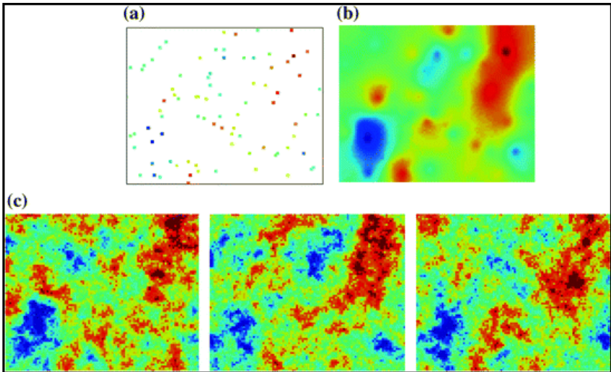
FIGURE 2.4 – Comparaison entre le résultat d'un krigeage (b), qui est déterministe, avec le résultat de trois simulations stochastiques (c). Le krigeage comme le modèle de simulation stochastique sont conditionnés et inférés à partir des mêmes données présentées en (a), d'après [Tahmasebi, 2018]
