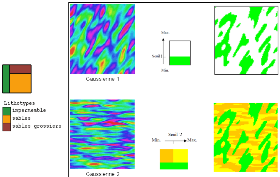
FIGURE 2.7 – Présentation du principe de la modélisation par pluri-gaussiennes du lithotype, d'après [Garnier, 2014]. La règle de troncature utilisée est celle du lithotype, présentée à gauche. Les trois faciès peuvent être en contact.
