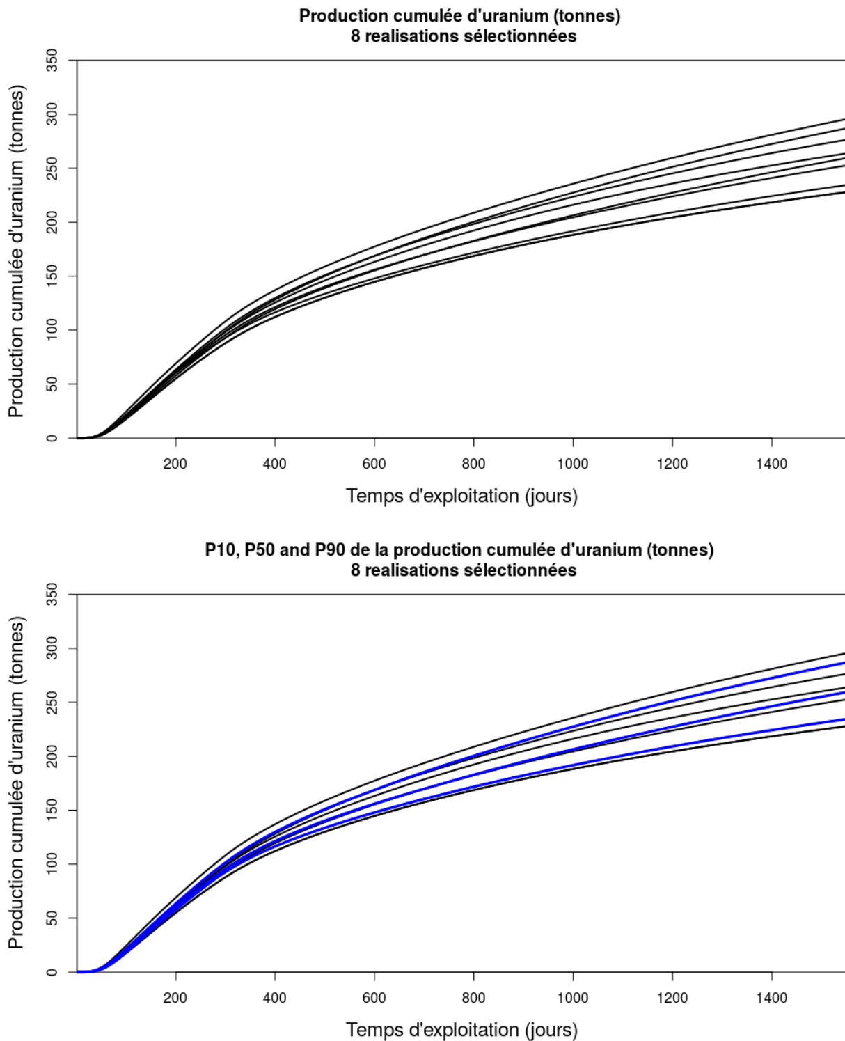
FIGURE 4.4 – Exemple de variabilité des résultats de simulation d'ISR pour un petit nombre de réalisations et quantification de l'incertitude des courbes. La simulation de l'ISR de l'uranium par transport réactif est effectuée uniquement dans les k réalisations sélectionnées. Il est possible de quantifier l'incertitude grâce à ces k réalisations en utilisant les valeurs de production à chaque pas de temps et la pondération des réalisations.
