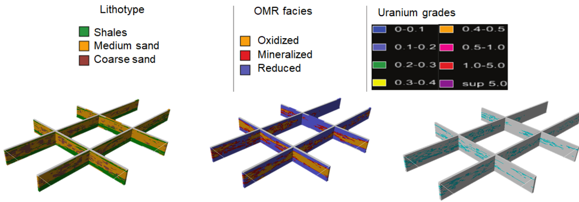
FIGURE 5.3 – Coupes verticales d’une réalisation du bloc de production PB01. La répartition spatiale des propriétés est différente pour chacune des réalisations. Elles sont cependant toutes conditionnées aux puits d’exploration et de développement
