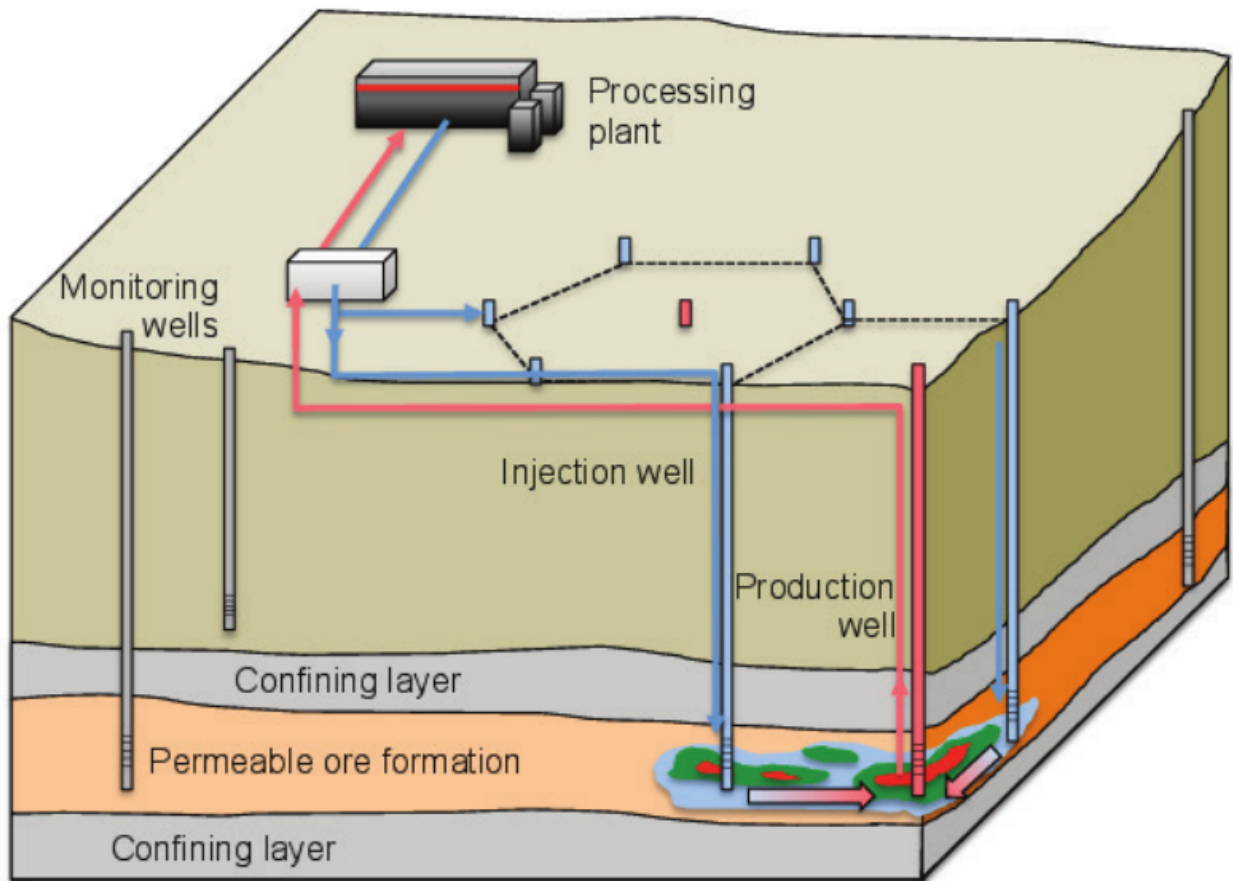
FIGURE 1.1 – Schéma de l'exploitation d'un dépôt d'uranium par ISR, d'après [Lagneau et al., 2019]
