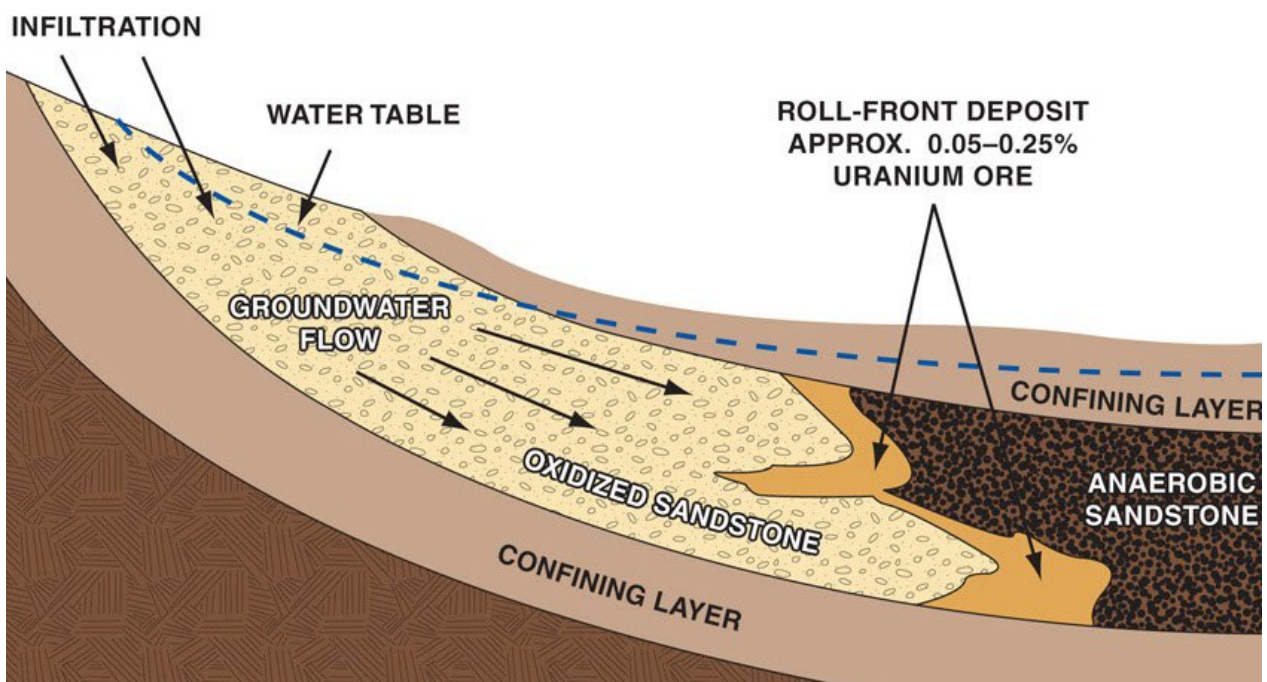
FIGURE 1.2 – Schéma d'un gisement typique de roll-front, d'après [CauldronEnergy, 2015]
