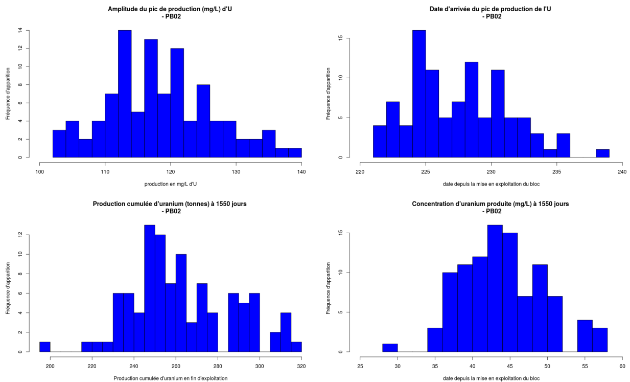
FIGURE 5.9 – Histogrammes des quatre variables résumant la variabilité de la production d'uranium de PB02
