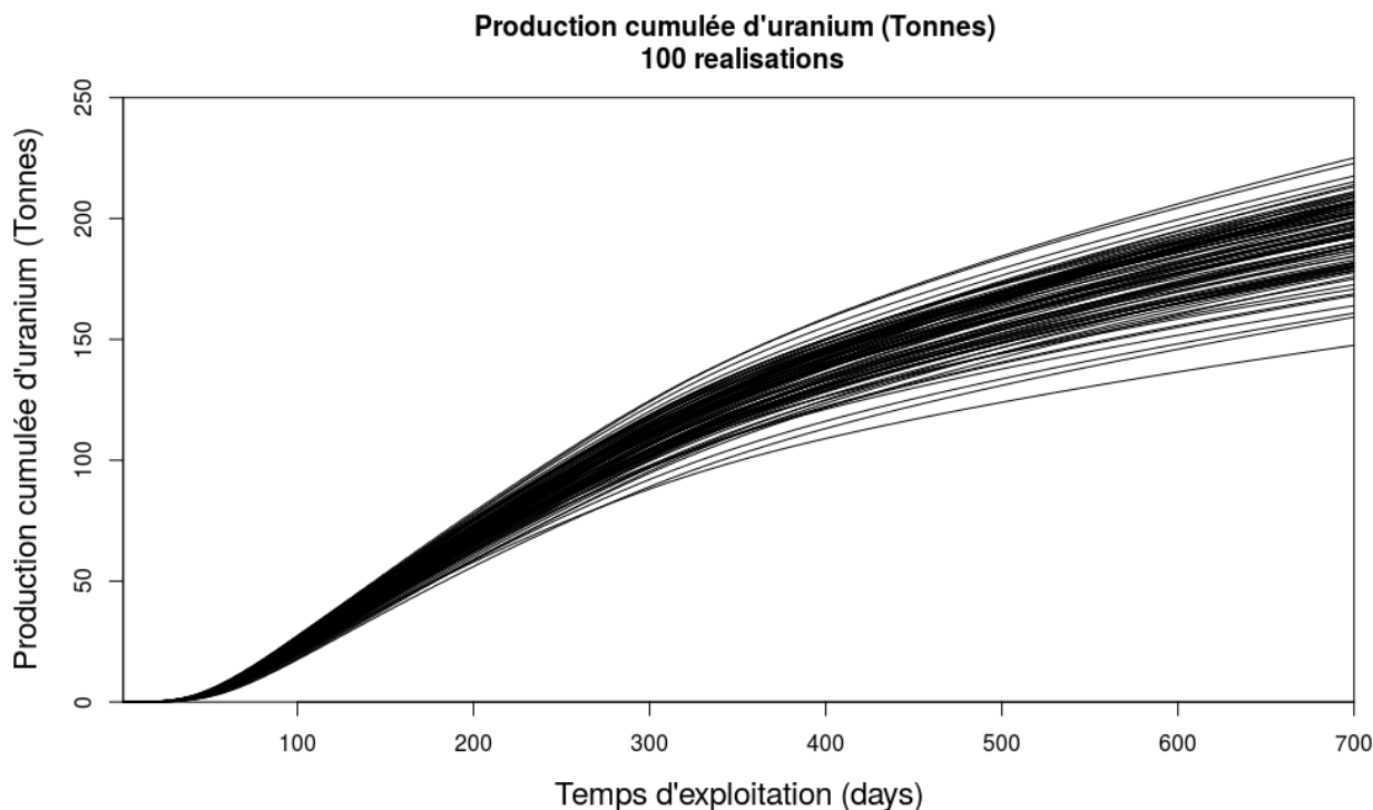
FIGURE 4.2 – Variabilité des résultats de simulation d'ISR pour cent réalisations. L'incertitude représentée par ces résultats pourra être représentée et quantifiée afin d'évaluer l'impact de la propagation de l'incertitude sur les propriétés géologiques.
