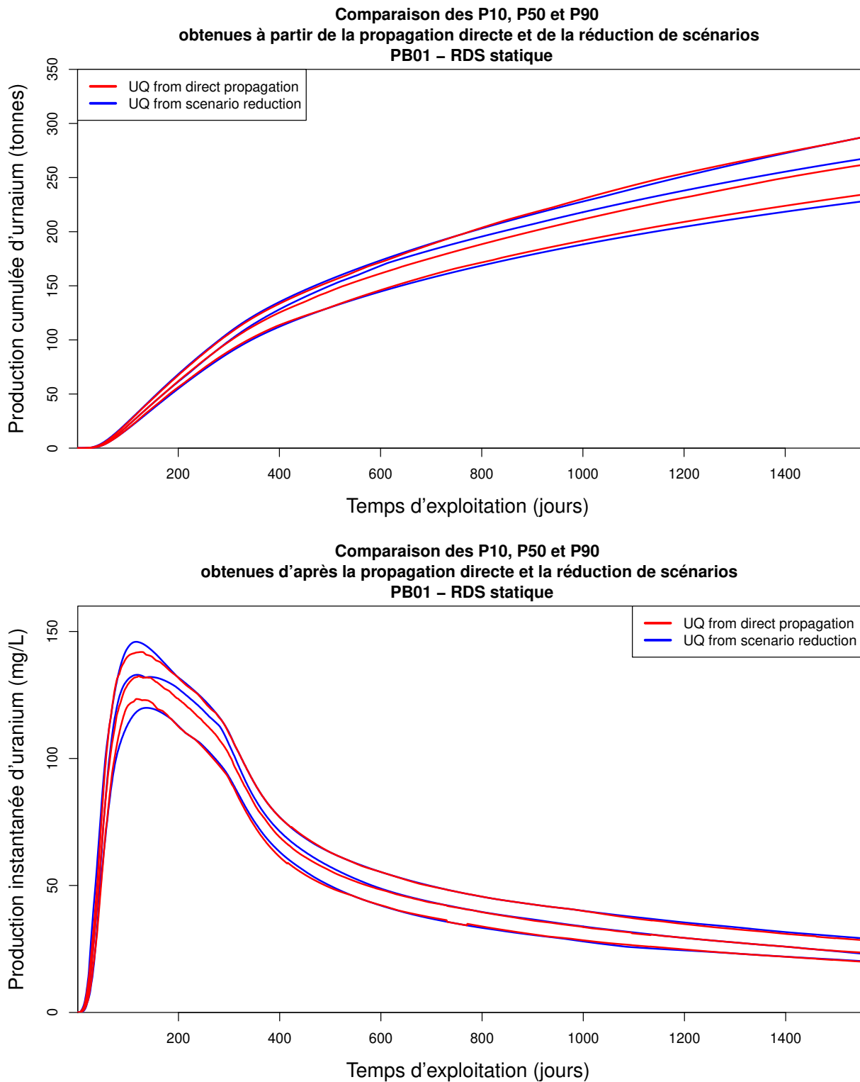
FIGURE 6.5 – Comparaison de la quantification d'incertitude sur la productions d'uranium cumulées et instantanées des dix réalisations sélectionnées pour le bloc PB01 avec les descripteurs statiques. On observe que les courbes P_{10} , P_{50} et P_{90} de référence sont globalement bien approchées, avec cependant un léger biais pour les P_{10} et P_{50} cumulée en fin de simulation, une légère sur-estimation de P_{90} au niveau du pic, et une légère sous-estimation de P_{10} au niveau du pic.
