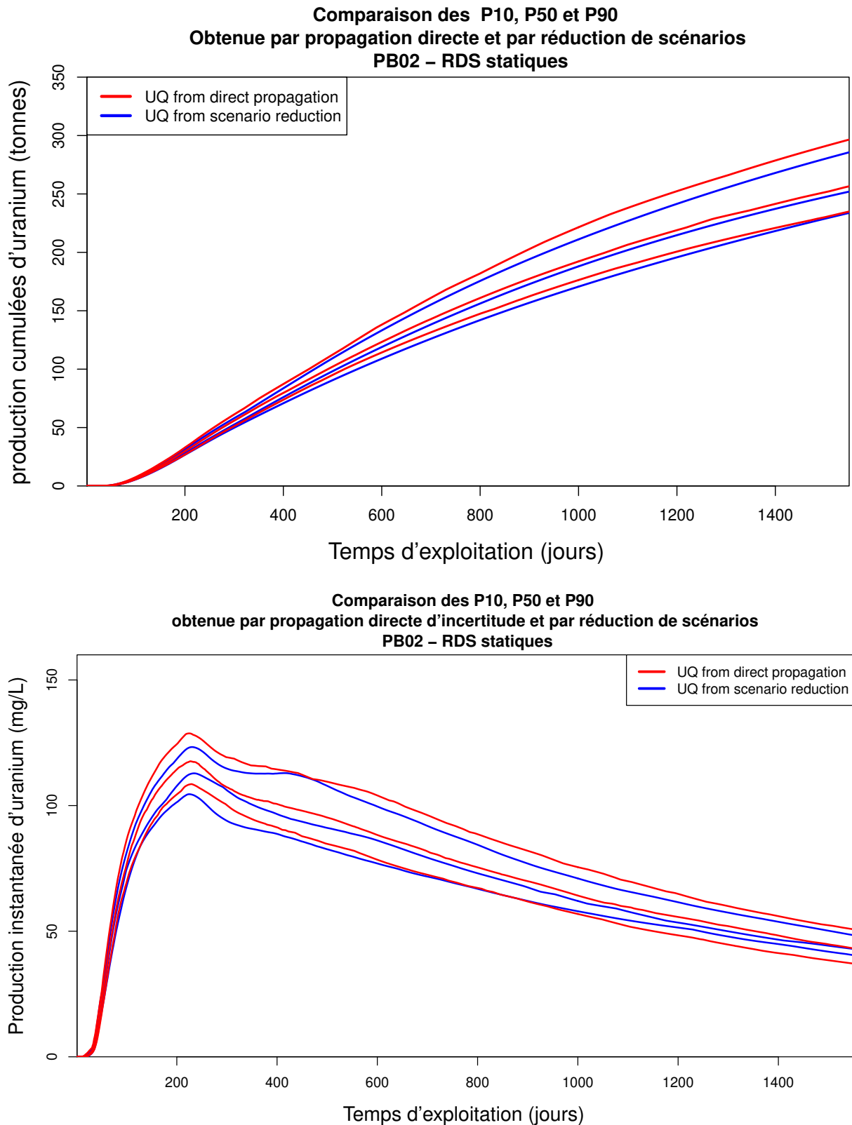
FIGURE 6.9 – Comparaison de la quantification d'incertitude sur la production d'uranium cumulée et instantanée des neuf réalisations sélectionnées pour le bloc PB02 avec les descripteurs statiques. La courbe P_{90} en production cumulée et les courbes P_{10} , P_{50} et P_{90} en production instantanée approchées par réduction de scénarios s'ajustent mal avec les courbes de référence. L'incertitude est plus particulièrement mal évaluée au niveau du pic de production
