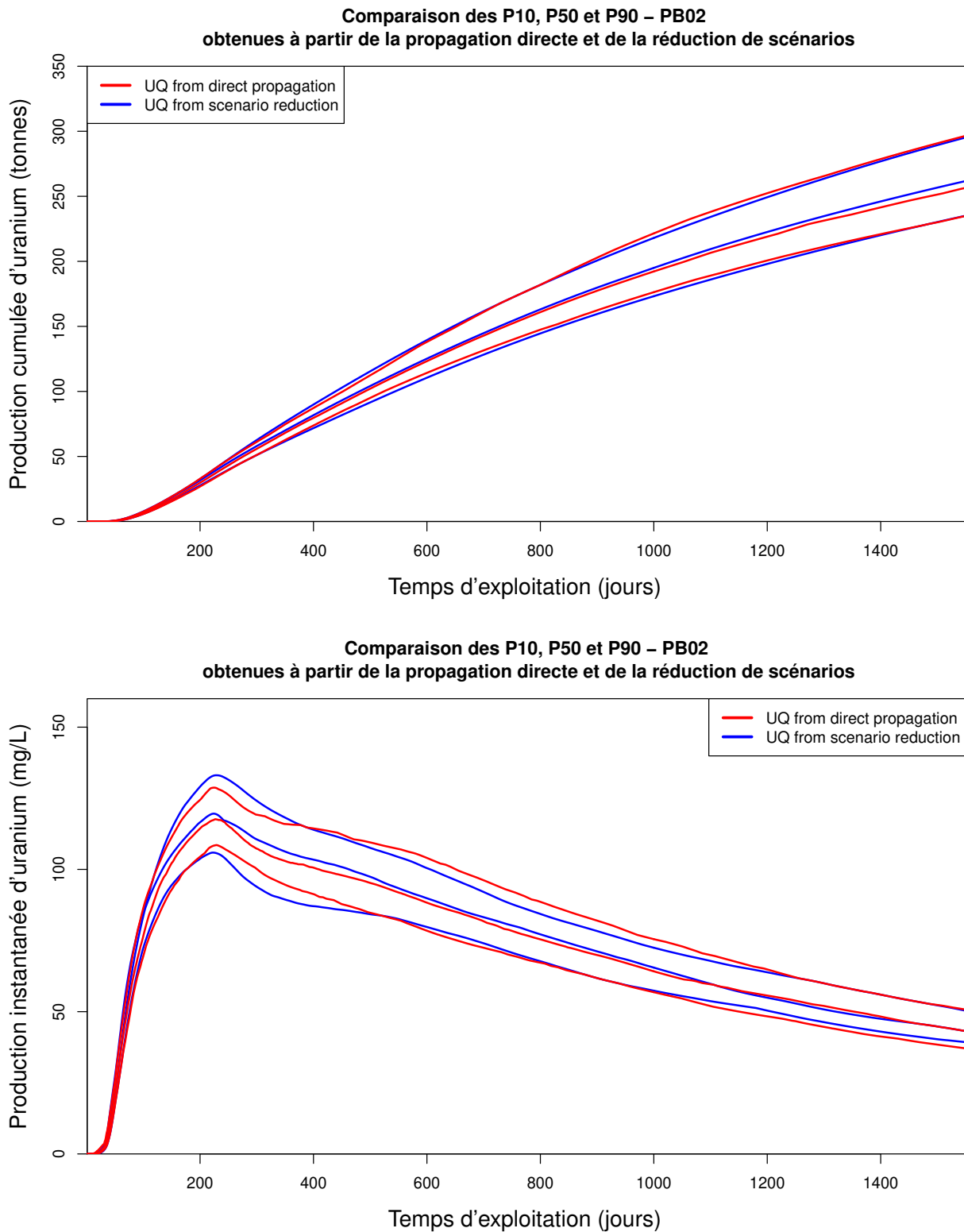
FIGURE 8.8 – Comparaison de la quantification d'incertitude de référence et celle approchée par la réduction de scénarios utilisant les descripteurs obtenues sur la récupération du minéral traceur cinétique sur PB02. On observe une très bonne approximation entre les P_{10} , p_{50} et P_{90} de référence et les déciles approchés par réduction de scénarios. On remarque tout de même une très légère sur-estimation de l'enveloppe d'incertitude au niveau du pic de production
