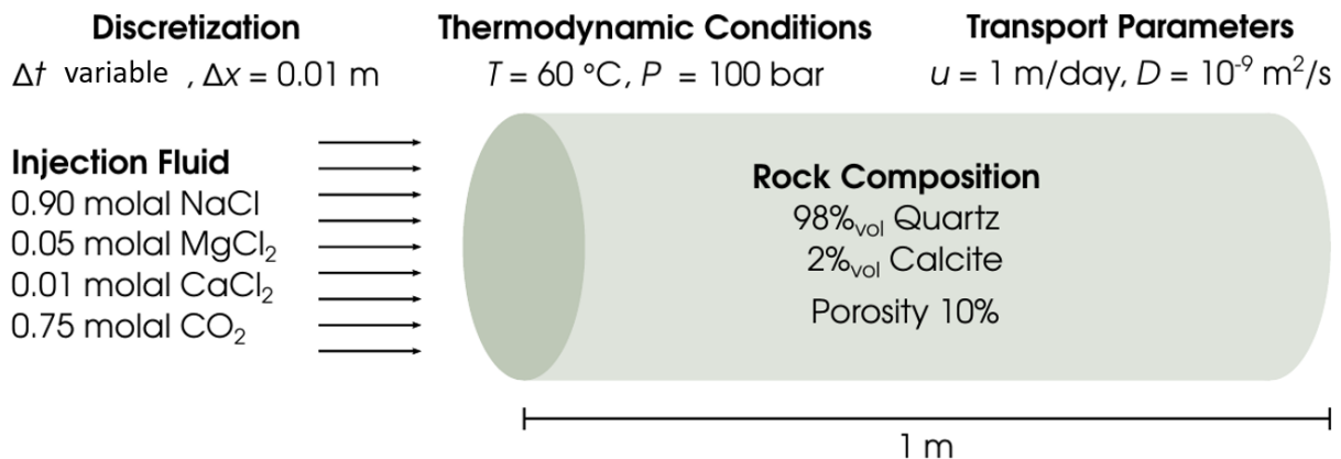
FIGURE 10.1 – Premier modèle de transport réactif utilisé pour développer un méta-modèle. Le modèle est présenté dans les travaux de Leal et al. [2017] pour développer un modèle de substitution au solveur de la chimie
