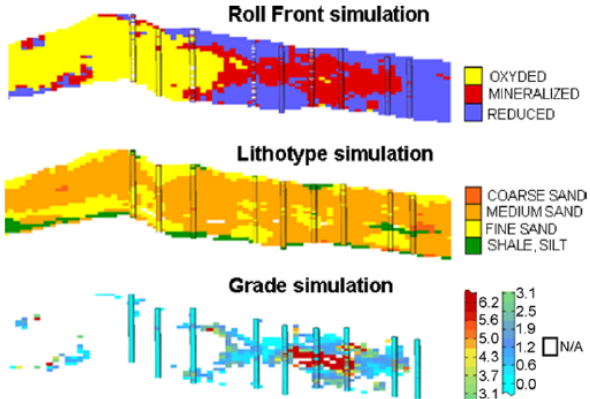
FIGURE 2.10 – Exemple d'une réalisation du gisement, constituée d'un triplet de simulations des propriétés lithotype, faciès OMR et teneur en uranium, d'après [Petit et al., 2012]
