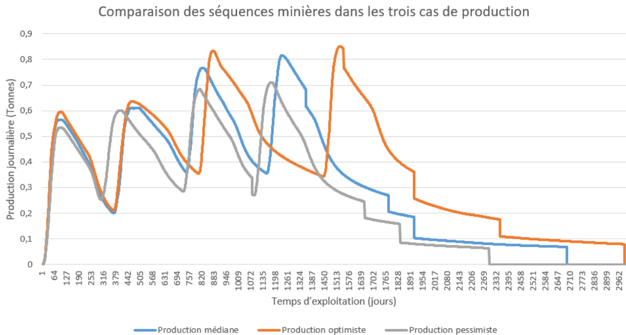
FIGURE 9.3 – Courbes de production journalière de l'exploitation des plans miniers calculés avec dates libres
