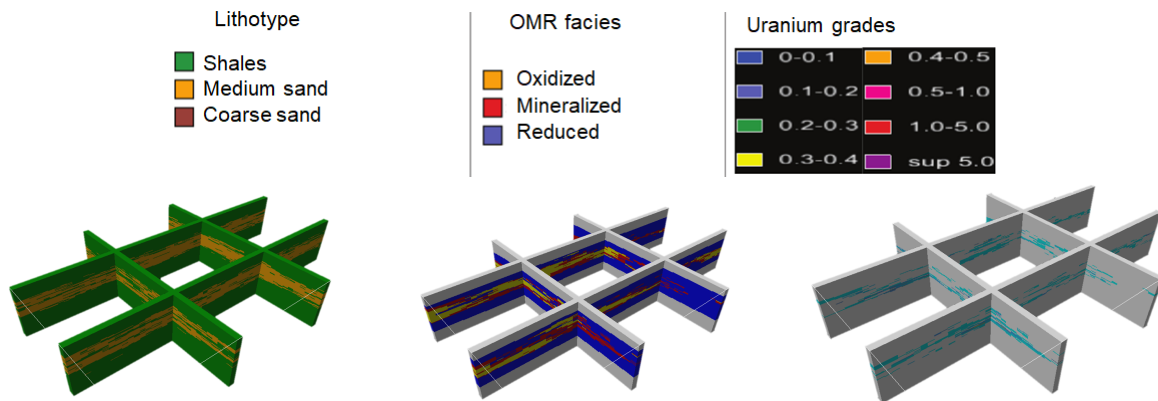
FIGURE 5.6 – Coupes verticales d'une réalisation du bloc de production PB02. La répartition spatiale des propriétés est différente pour chacune des réalisations
