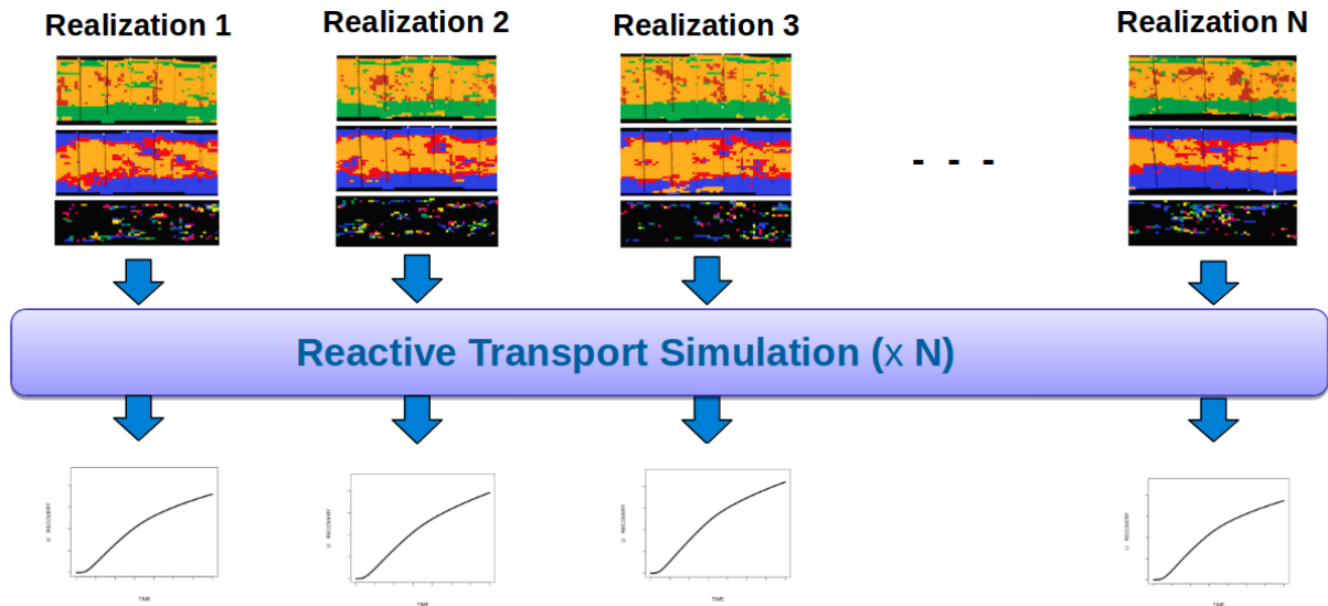
FIGURE 4.1 – Schéma de propagation directe de l'incertitude géologique en incertitude dynamique. L'exploitation de l'uranium par ISR est simulée dans chacune des N réalisations géostatistiques
