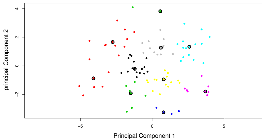
FIGURE 6.3 – Partitionnement en 10 clusters des réalisations en fonction de PB01 avec les descripteurs statiques. On n'observe aucune structure particulière dans le nuage de réalisations affiché
