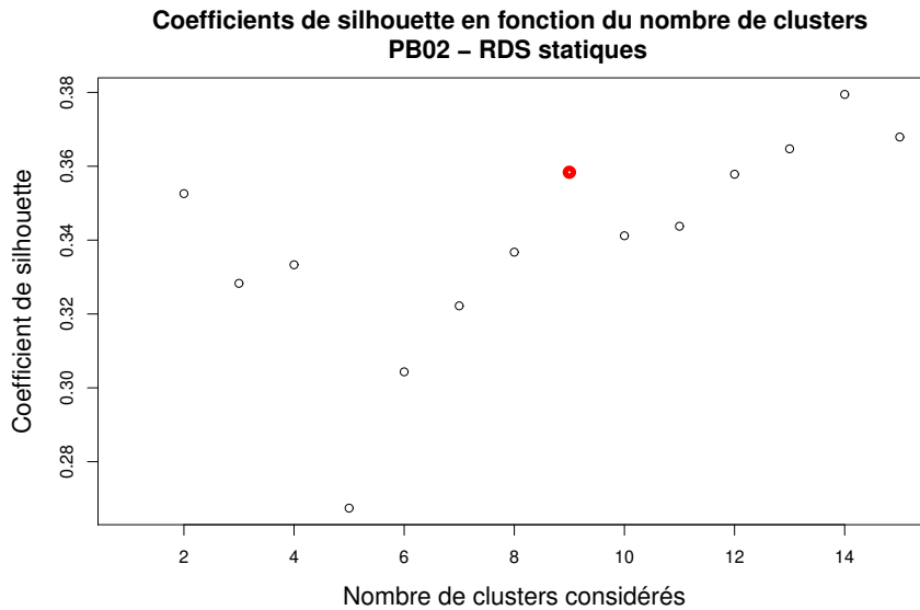
FIGURE 6.7 – Silhouettes moyennes des réalisations en fonction du nombre de clusters après le partitionnement des réalisations de PB02 avec les descripteurs statiques. Dans ce cas ci, on choisira de sélectionner 9 réalisations représentatives
