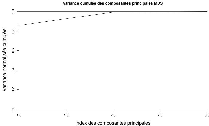
FIGURE 8.3 – Variance cumulée associée aux composantes principales du MDS effectué sur les trois descripteurs retenus. Plus de 99% de la variance est expliquée par les deux premières composantes principales
