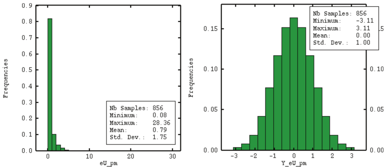
FIGURE 2.9 – Transformation des mesures de teneurs (à gauche) en données gaussiennes (à droite) par anamorphose par polynômes d'Hermite
