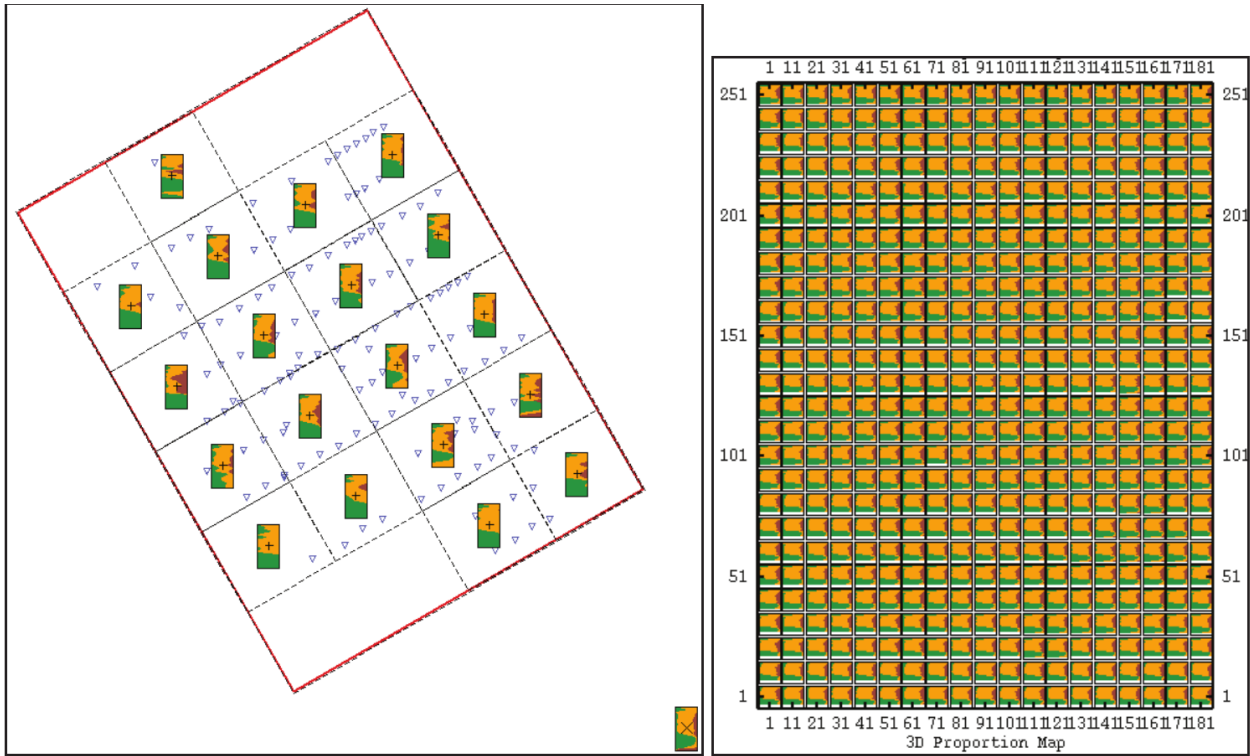
FIGURE 2.8 – Passage des courbes de proportions verticales à la matrice de proportions 3D, d'après [Garnier, 2014]. Les courbes de proportions verticales dans les mailles étant globalement stationnaires horizontalement, les proportions de la matrice de proportions sont la moyenne de toutes les courbes de proportions verticales
