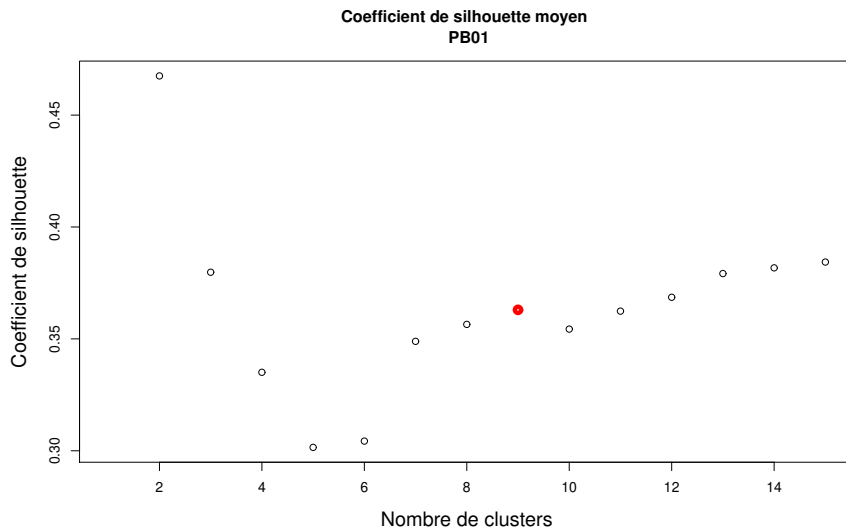
FIGURE 8.4 – Silhouettes moyennes des réalisations en fonction du nombre de clusters après le partitionnement des réalisations de PB01 avec les descripteurs du minéral traceur cinétique. Le meilleur compromis est de 9 clusters
