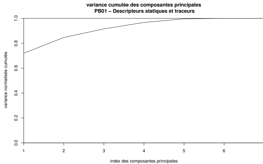
FIGURE 7.2 – Variance cumulée portée par les composantes principales du MDS sur la combinaison de descripteurs statiques et de récupération de traceurs des réalisations du bloc PB01. Les deux premières composantes expliquent 84.6% de la variance des réalisations
