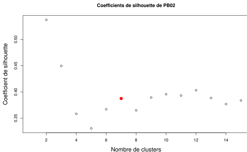
FIGURE 8.7 – Silhouettes moyennes des réalisations en fonction du nombre de clusters après le partitionnement des réalisations de PB02 avec les descripteurs obtenues sur la récupération du minéral traceur cinétique. Dans ce cas ci, on choisira de sélectionner 7 réalisations représentatives
