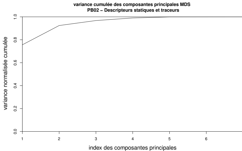
FIGURE 7.5 – Variance cumulée portée par les composantes principales du MDS sur les descripteurs statiques des réalisations du bloc PB02. Les deux premières composantes expliquent 92.4% de la variance des réalisations
