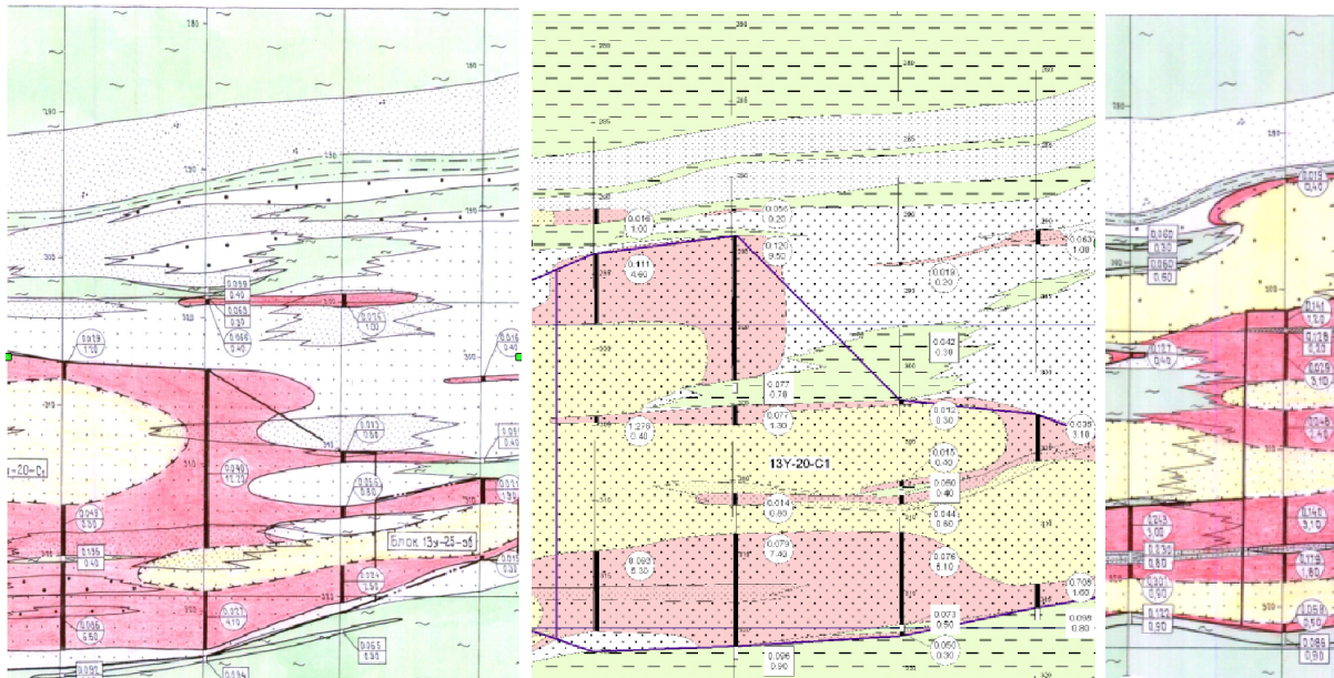
FIGURE 5.4 – Trois coupes verticales parallèles de PB02 montrant le lithotype et la minéralisation. Le vert correspond aux argiles imperméables, Le jaune et le blanc aux sables perméables, et enfin le rouge au minerai riche en uranium. Coupes provenant de Katco. Les traits de coupes sont tracés sur la figure 5.5
