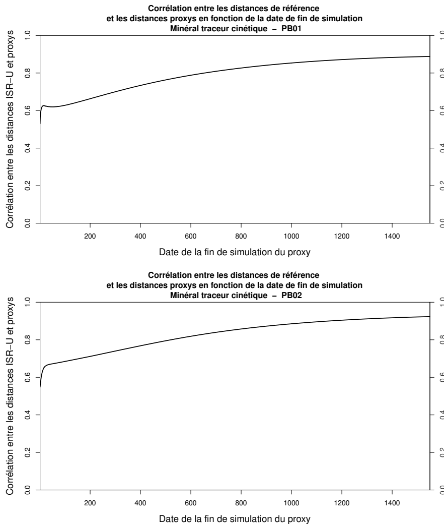
FIGURE 8.9 – Corrélation entre les distances de référence et les distances proxys en fonction de la date de fin de simulation des traceurs. On observe dans les deux cas que la corrélation ne s'améliore plus que très lentement à partir des 900 jours
