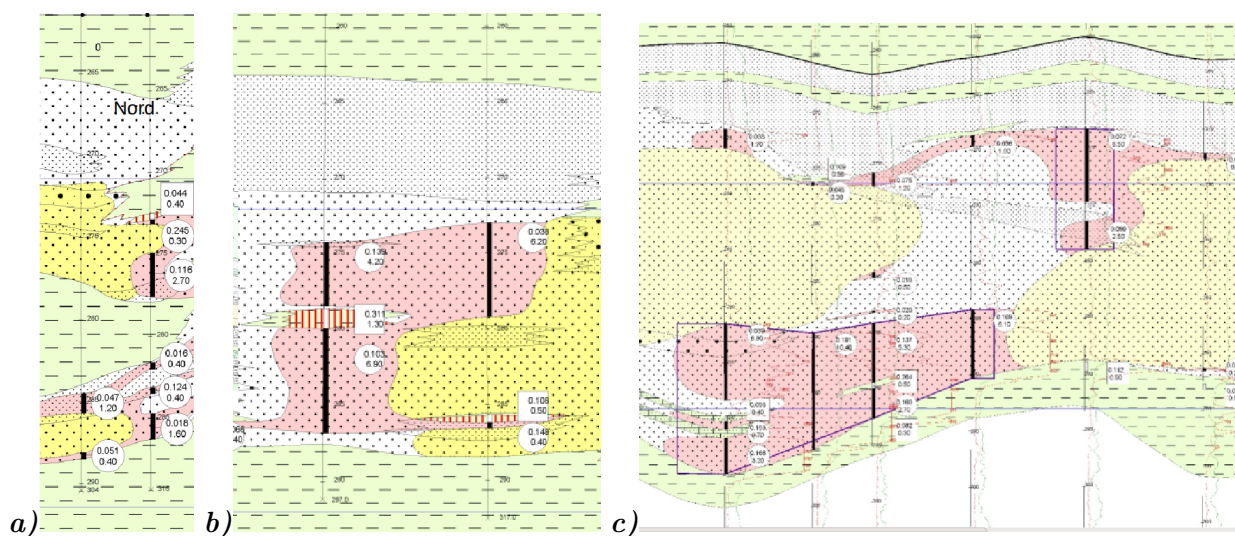
FIGURE 5.2 – Trois coupes géologiques verticales parallèles du bloc de production PB01 présentant la lithologie et la minéralisation. Le vert correspond aux argiles imperméables, Le jaune et le blanc aux sables perméables, et enfin le rouge au minerai riche en uranium. Coupes provenant de Katco.
