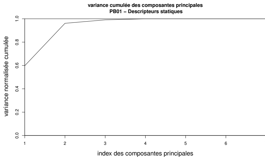
FIGURE 6.1 – Variance cumulée portée par les composantes principales du MDS sur les descripteurs statiques des réalisations du bloc PB01. Les deux premières composantes expliquent 96.1% de la variance des réalisations
