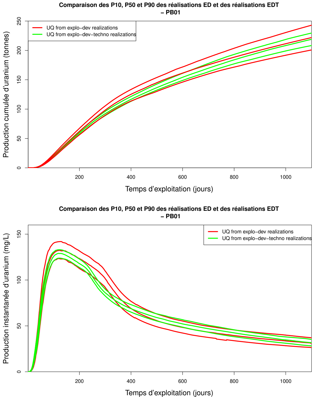
FIGURE 5.11 – Comparaison des quantifications d'incertitude des simulations ISR-U faites avec les réalisations conditionnées exploration développement et des quantification d'incertitude des simulations ISR-U calculées avec les réalisations conditionnées exploration développement et technologique sur PB01. Les courbes P_{50} tendent à se rejoindre vers la fin des simulations. Il s'agit d'un hasard, aucun facteur d'homogénéisation entre les deux ensembles de réalisations n'a été appliqué. Deuxièmement, On observe clairement une diminution de la taille de l'enveloppe d'incertitude entre les deux jeux de production d'uranium. L'enveloppe d'incertitude de production des réalisations mises à jour est à peu près incluse dans l'enveloppe initiale
