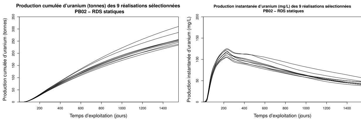
FIGURE 6.8 – Productions d'uranium cumulées et instantanées des neuf réalisations sélectionnées pour le bloc PB02 avec les descripteurs statiques. La sélection montre deux types de production : une forte et une faible. l'échantillonnage est hétérogène et ne reflète pas la production du jeu de réalisation de référence
