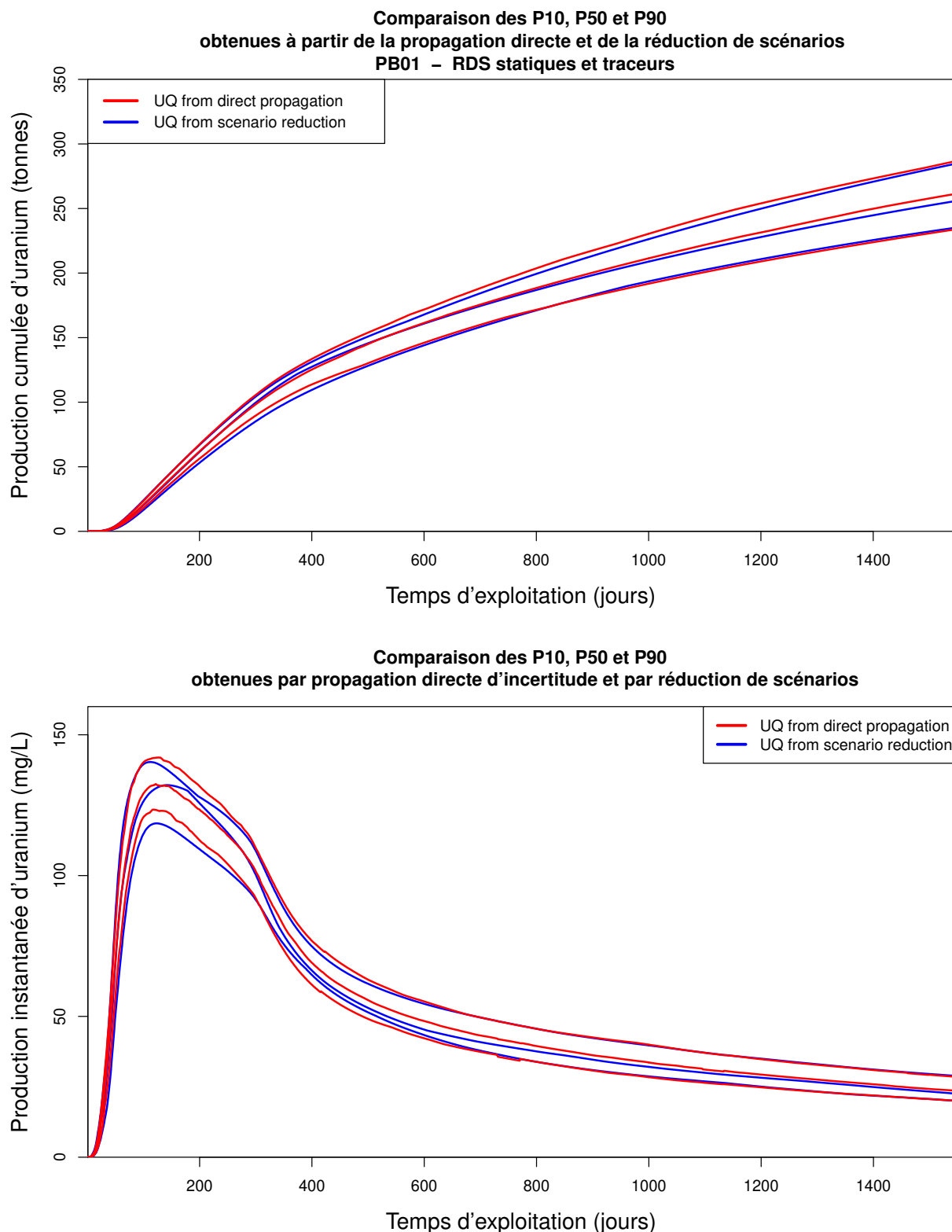
FIGURE 7.4 – Comparaison de la quantification d'incertitude de référence et celle approchée par la réduction de scénarios utilisant les descripteurs statiques et de récupération de traceurs sur PB01. Les courbes P_{10} , P_{50} et P_{90} de référence sont globalement bien approchées par celles obtenues par réduction de scénarios. On peut remarquer cependant deux écarts : un écart minime sur la masse d'uranium médiane produite en fin d'exploitation, et une sous-estimation de l'amplitude du pic de production au P_{10} .
