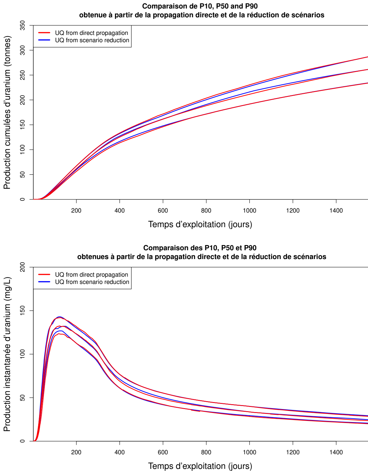
FIGURE 8.5 – Comparaison de la quantification d'incertitude de référence et celle approchée par la réduction de scénarios utilisant les descripteurs de la récupération du minéral traceur cinétique sur PB01. Les courbes P_{10} , p_{50} et P_{90} de la production cumulée et de la production instantanée de référence sont très bien approchées par celles obtenues à partir de la réduction de scénarios
