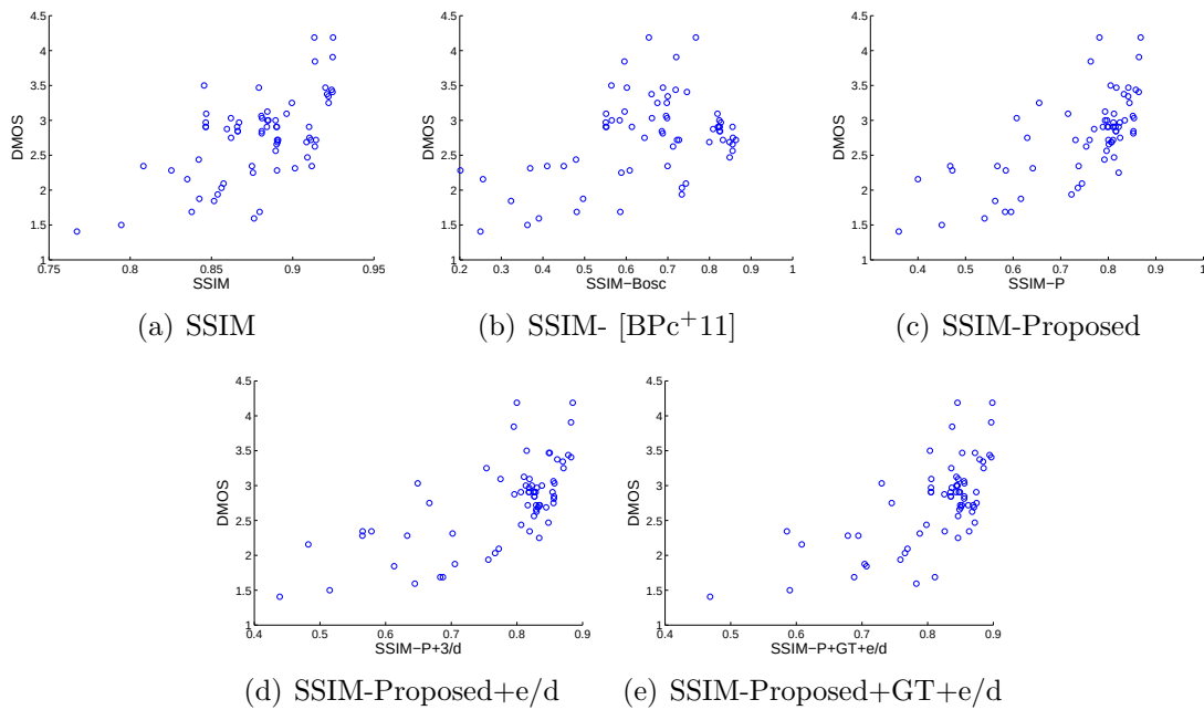
Figure 17 – Nuage de points des résultats objectifs pour le SSIM avec des ROI testés. Chaque point est le DMOS par rapport au score objectif moyen sur toutes les images pour une séquence, une synthèse et une méthode.
