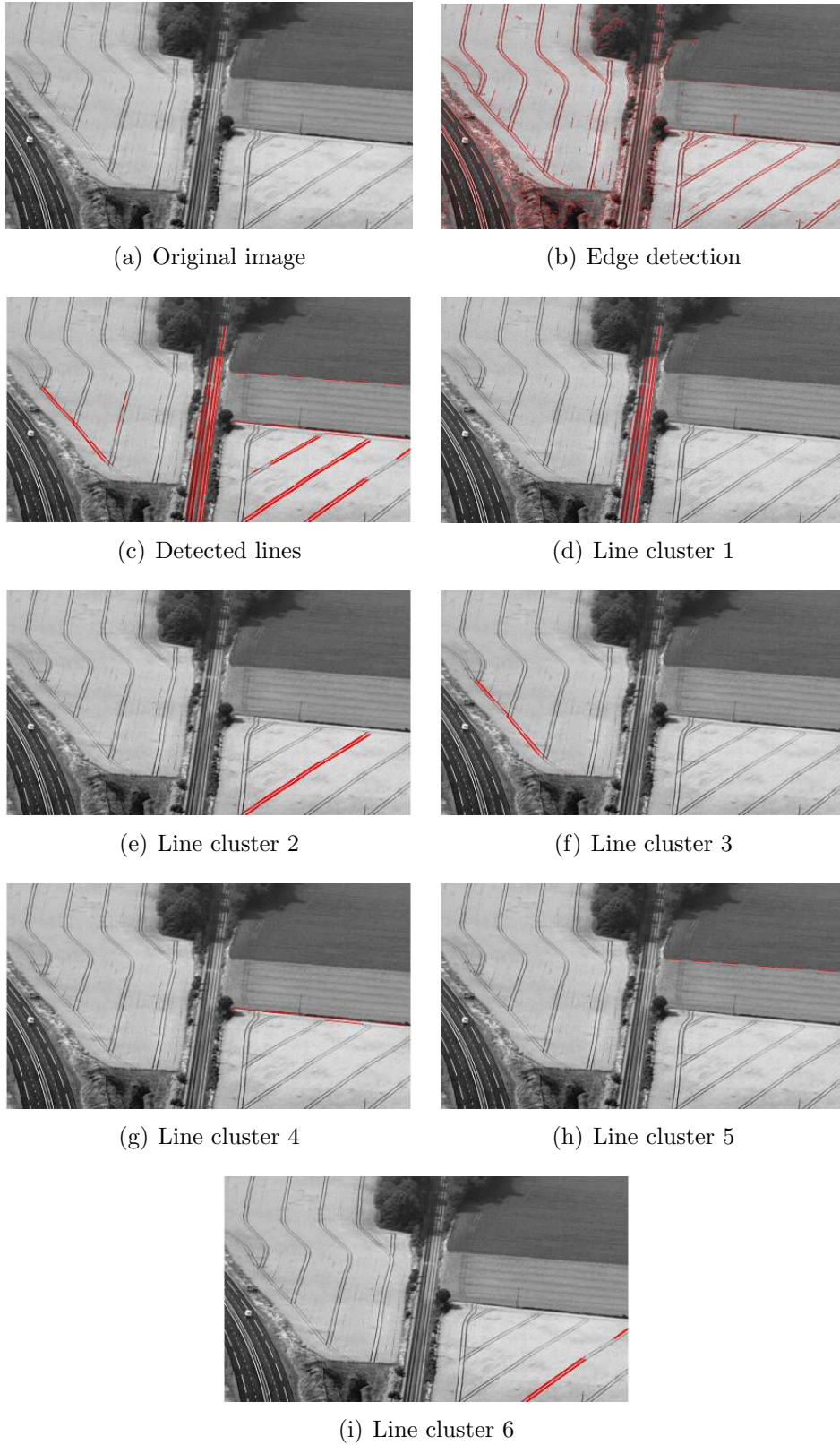
Figure 22 – Un exemple des lignes détectées et du processus de clustering pour l'image 40 de la Séquence 2.
