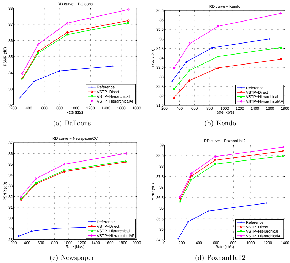
Figure 12 – Courbes RD de la référence et de la méthode proposée sur le scénario de test 3 vues pour les séquences Balloons, Kendo, NewspaperCC et PoznanHall2.
