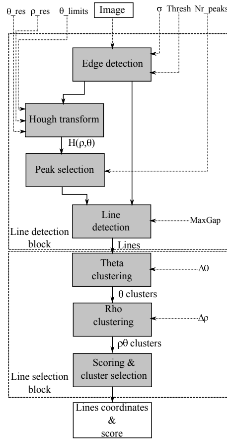
Figure 21 – Schéma général de l'algorithme.
