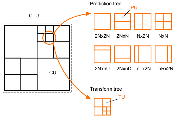
Figure 2 – Structure de partitionnement de trame dans HEVC.
