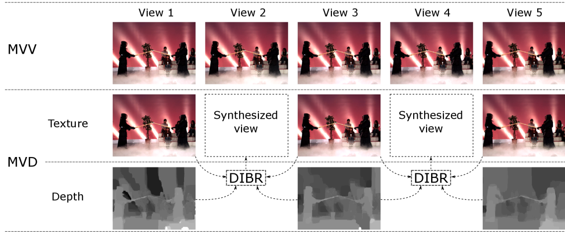
Figure 5 – Vidéo MultiView et MultiView-plus-depth.
