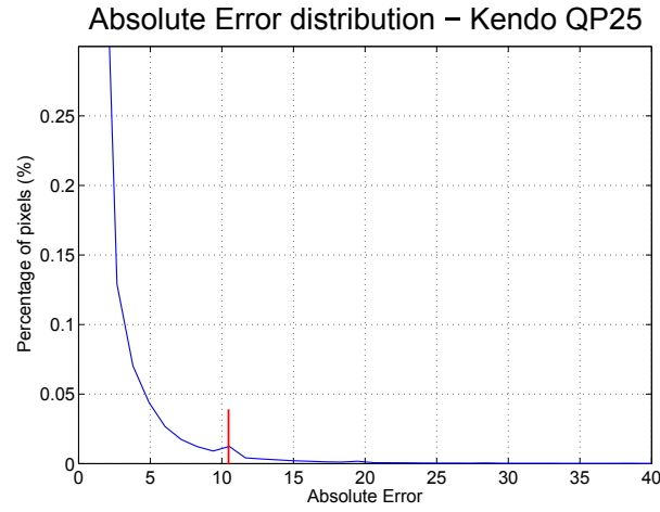
Figure 15 – Distribution d'erreur absolue pour une trame synthétisée dans une séquence de Kendo, à QP = 25.
