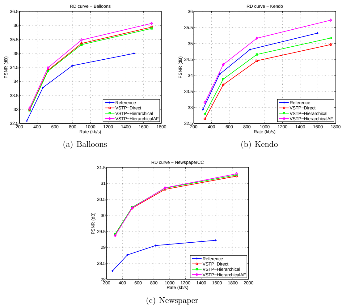
Figure 13 – Courbes RD de la référence et de la méthode proposée sur le scénario de test 5 vues pour les séquences Balloons, Kendo et NewspaperCC.
