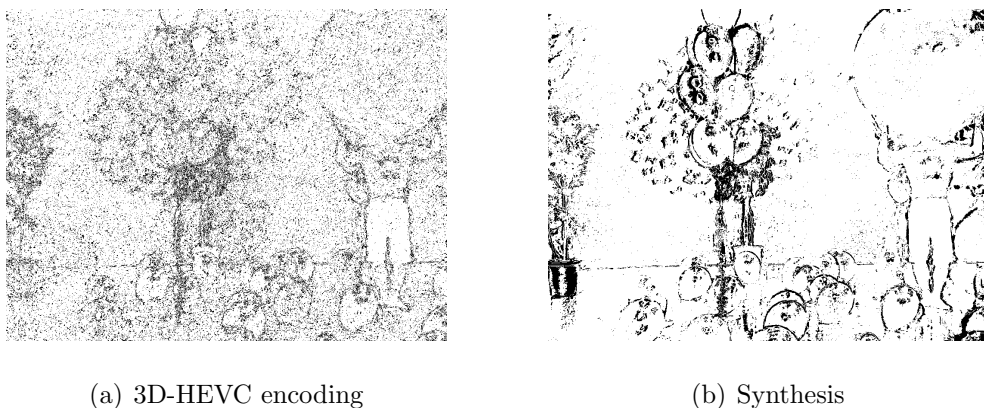
Figure 14 – Les masques binaires sur l'image 1 de la séquence Balloons, en noir, indiquent des pixels avec des erreurs absolues élevées.
