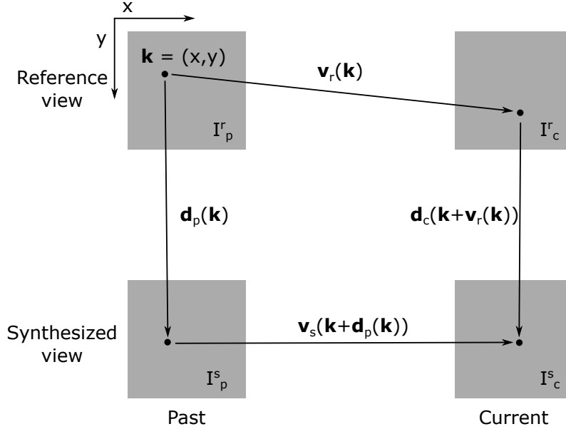
Figure 6 – Contrainte épipolaire, la relation entre les champs vectoriels de disparité (DVF) \mathbf{d}_p et \mathbf{d}_c à deux instants c et p respectivement, et les MVFs dans la vue synthétisée et de référence \mathbf{v}_s et \mathbf{v}_r respectivement pour une position \mathbf{k} dans le cadre de référence I_p^r .
