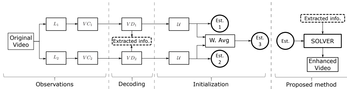
Figure 19 – Une vue schématique de la configuration expérimentale. Deux opérateurs de rééchantillonnage sont appliqués sur une séquence d’entrée. Chaque observation est compressée et décompressée, et des informations utiles sont extraites. Les observations décodées sont suréchantillonnées à leur résolution d’origine en utilisant l’inverse de l’opérateur de dégradation ou une méthode SOA SR. Ensuite, le cadre proposé est initialisé avec une estimation \tilde{A} haute résolution et les informations extraites pendant le décodage.
