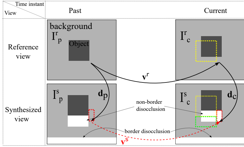
Figure 7 – Récupération temporelle de la zone non-occultées. Les carrés en pointillés jaunes marquent la position de l’objet dans le cadre précédent, le carré en pointillés vert montre les zone non-occultées dans le cadre précédent et les carrés en pointillés rouges indiquent la zone non-occultée qui était visible dans une trame précédente.
