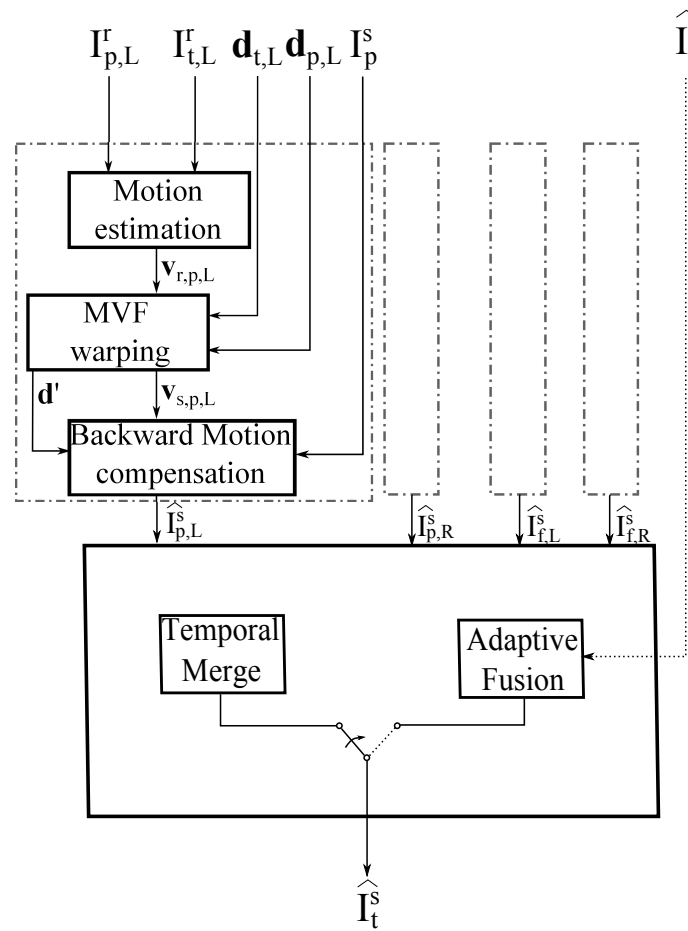
Figure 10 – Diagramme de flux pour la synthèse de vues exploitant la prédiction temporelle (VSTP).
