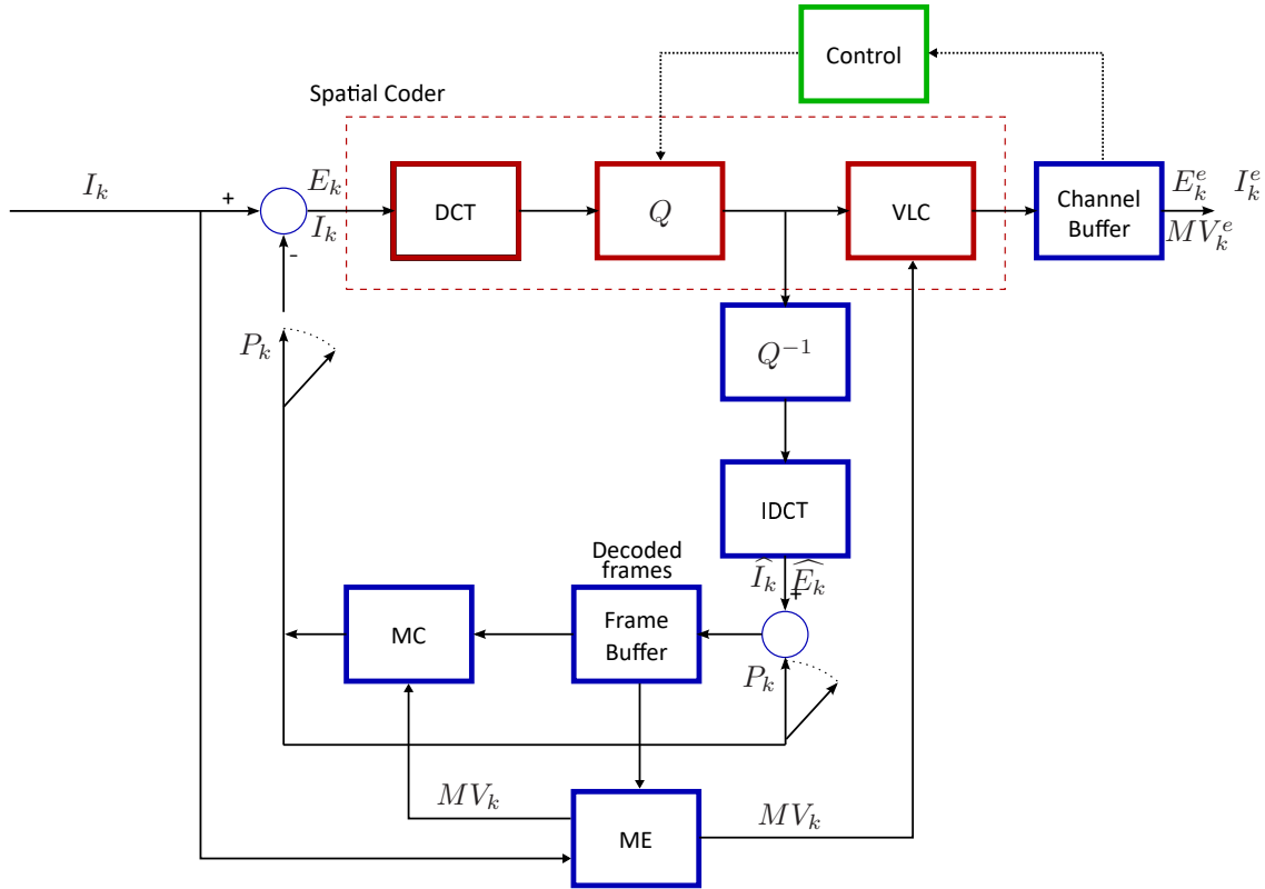
Figure 1 – Schéma générique du codeur hybride.
