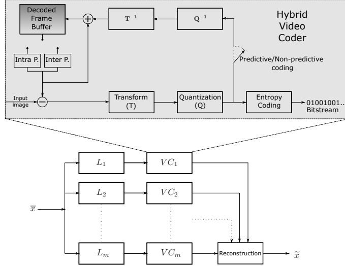
Figure 18 – Un modèle générique pour le sous-échantillonnage, la compression et la reconstruction de plusieurs sources vidéo.
