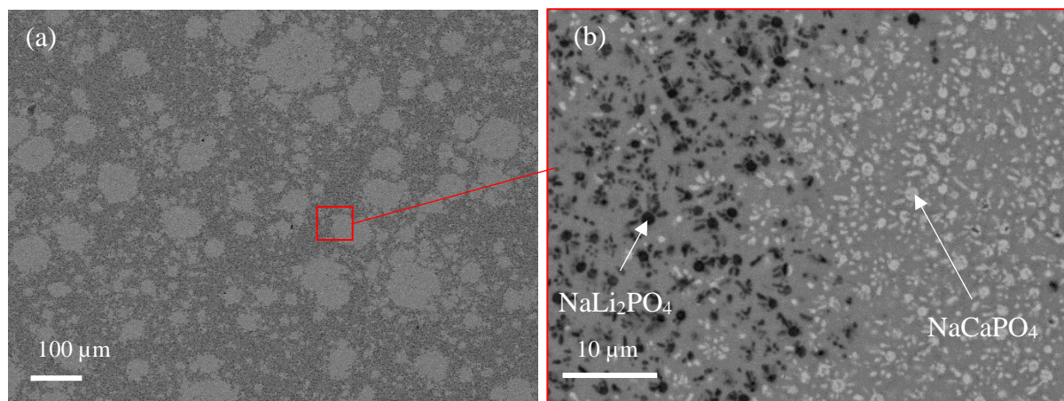
Figure 16 : Clichés MEB en électrons rétrodiffusés de l'échantillon 20.P50 RL refroidi lentement à 1 °C.min -1 .
