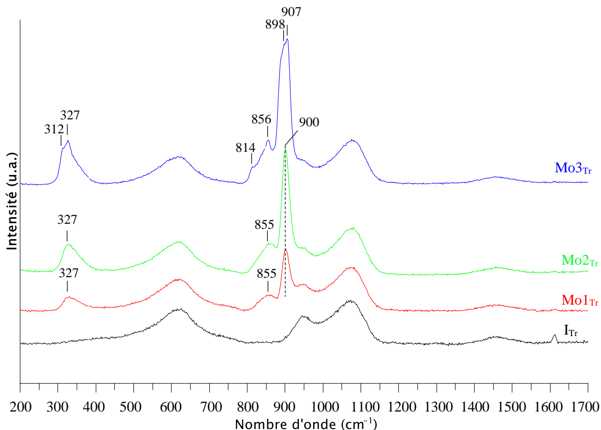
Figure 9 : Spectres Raman des échantillons trempés de la série \text{Mo}_x obtenus après trempe du liquide en fusion à 1100 °C.
