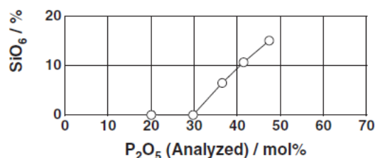
Figure 16 : Evolution de la proportion d'entités SiO_6 en fonction de la proportion d'oxyde de phosphore dans le binaire SiO_2 - P_2O_5 (fusion à 1500 °C et refroidissement à température ambiante) [59].
