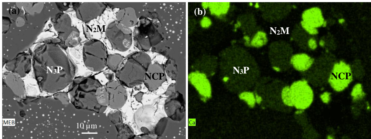
Figure 25 : (a) Cliché MEB de l'échantillon Mo3P4 RL refroidi lentement à 1 °C.min -1 , (b) cartographie EDX pour l'élément Ca du cliché (a). N3P = Na 3 PO 4 , NCP = NaCaPO 4 , N2M = Na 2 MoO 4 .
