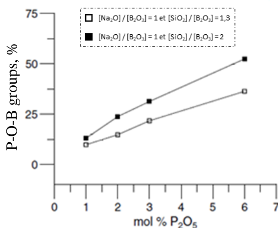
Figure 19 : Variation de la proportion de liaisons P – O – B dans des verres du système SiO_2 - Na_2O - B_2O_3 - P_2O_5 (□ : [Na_2O]/[B_2O_3] = 1 et [SiO_2]/[B_2O_3] = 1,3 , ■ : [Na_2O]/[B_2O_3] = 1 et [SiO_2]/[B_2O_3] = 2 ) en fonction de la teneur en P_2O_5 (%mol). Dans cette étude, les espèces phosphatées liées aux atomes de bore sont de type pyrophosphate P_2O_7^{4-} , cette figure présente donc les groupes P_2O_7^{3-} - B [79].
