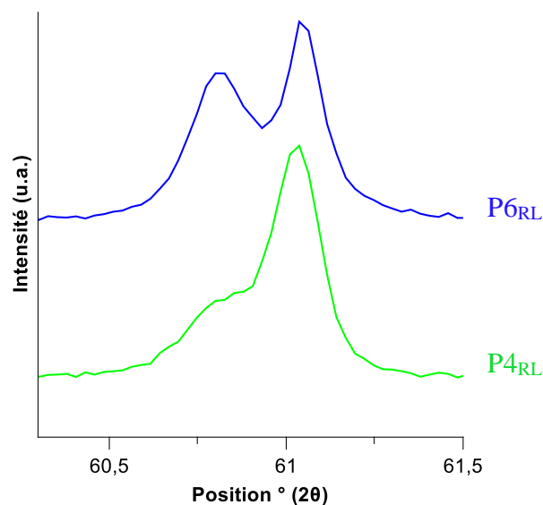
Figure 10 : Diagrammes de diffraction des rayons X sur l'intervalle [60,3 ; 61,5] des échantillons \text{P4}_{\text{RL}} et \text{P6}_{\text{RL}} refroidis lentement à 1^\circ\text{C}\cdot\text{min}^{-1} depuis 1100 °C.
