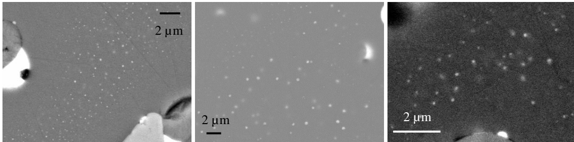
Figure 24 : Phases molybdates de taille nanométriques observées pour les échantillons refroidis lentement à 1 °C.min -1 depuis 1100 °C: (a) Mo 3 P 4 RL, (b) Mo 3 P 6 RL, (c) Mo 3 P 8 RL.
