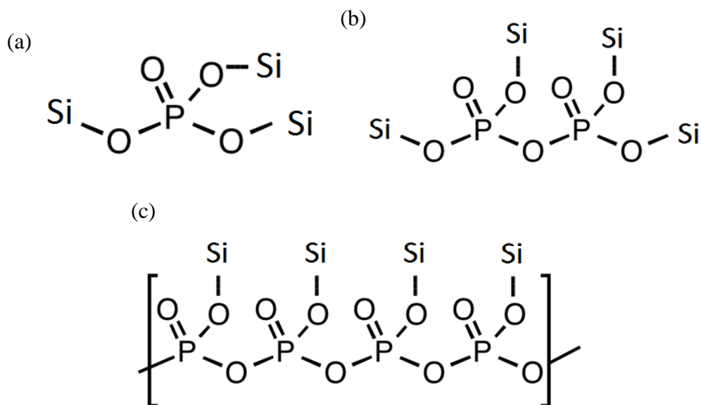
Figure 15: Représentations (a) d'un groupement orthophosphate PO_4 dilué dans le réseau silicaté, (b) d'un groupement pyrophosphate P_2O_7 relié au réseau silicaté, (c) d'une chaîne métaphosphate reliée au réseau silicaté.
