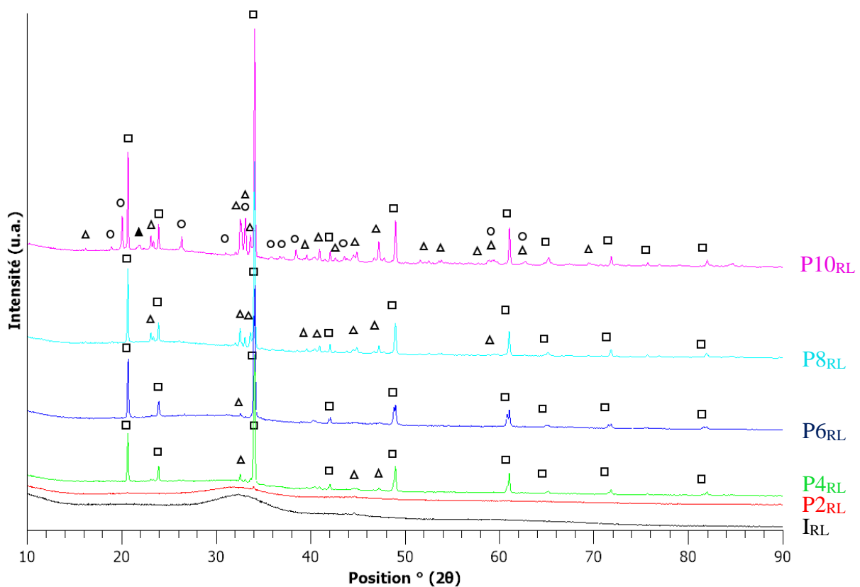
Figure 7 : Diagrammes de diffraction des rayons X des échantillons P_{xRL} refroidis lentement à 1 \text{ } ^\circ\text{C}\cdot\text{min}^{-1} depuis 1100 \text{ } ^\circ\text{C} . \square : \gamma\text{-Na}_3\text{PO}_4 (00-031-1318), \circ : \text{Na}_4\text{P}_2\text{O}_7 (04-018-4331), \triangle : \text{NaCaPO}_4 (04-0016-6900), \blacktriangle : \text{SiO}_2 cristobalite (04-013-9484).
