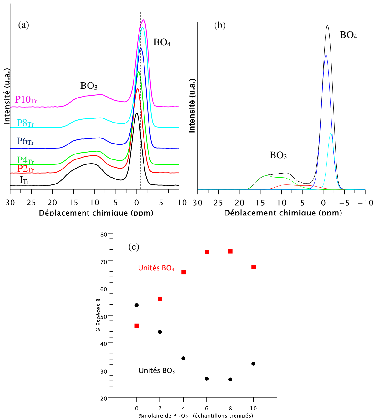
Figure 25 : (a) Spectres RMN ^{11}\text{B} des échantillons de la série \text{P}_x obtenus après trempé du liquide en fusion à 1100^\circ\text{C} . (b) Exemple de simulation du spectre RMN ^{11}\text{B} de \text{P6}_{\text{Tr}} avec 4 compositions : deux pour les unités \text{BO}_3 et deux pour les \text{BO}_4 . (c) Evolution des proportions d'unités \text{BO}_3 et \text{BO}_4 correspondantes dans ces échantillons en fonction de la teneur en \text{P}_2\text{O}_5 , obtenues par simulation des spectres (l'erreur sur la mesure est estimée à \pm 1\% ).
