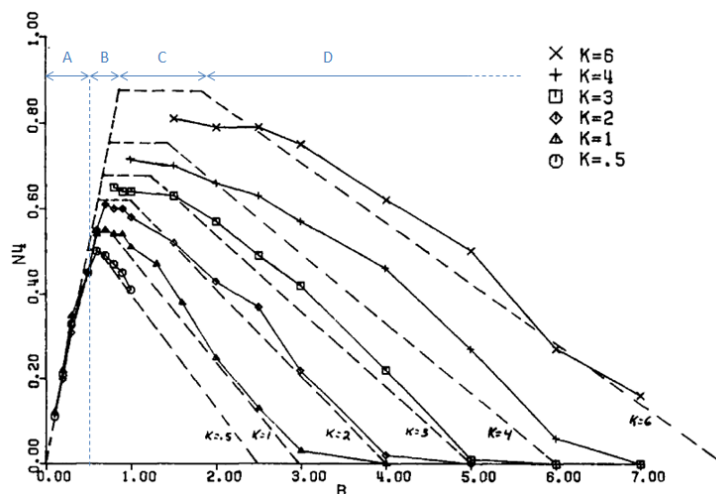
Figure 7 : Evolution de N_4 en fonction de R et K dans le système ternaire \text{SiO}_2 - \text{B}_2\text{O}_3 - \text{Na}_2\text{O} adapté de [32]. Les lignes pointillées représentent les prédictions du Modèle de Bray et les traits pleins représentent les points expérimentaux obtenus par Bray et al. par RMN du bore [30] [32]. Les lettres indiquées en haut de la figure désignent les différents domaines de R (pour K = 6 ).
