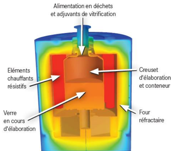
Figure 3 : Schéma du four du procédé IN CAN MELTER montrant, au sein du four, le creuset métallique (en orange) contenant le mélange des déchets et de la fritte de verre [14]. Le conteneur représenté ici est deux fois moins haut qu'un conteneur CSD-V.
