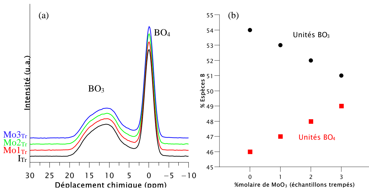
Figure 10 : (a) Spectres RMN 11 B des échantillons trempés de la série Mox obtenus après trempé du liquide en fusion à 1100 °C, (b) proportion d'unités BO 3 et BO 4 correspondantes (l'erreur sur la mesure est estimée à ± 1 %).
