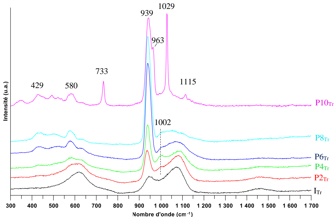
Figure 23 : Spectres Raman des échantillons de la série Px obtenus après trempe du liquide en fusion à 1100\text{ °C} .
