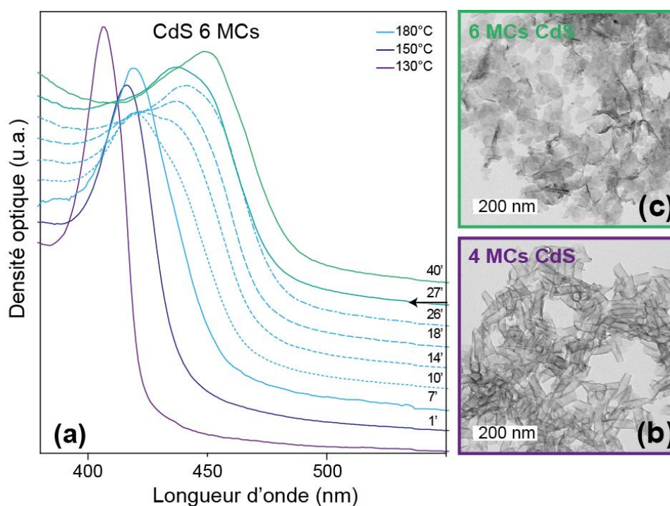
Figure 49 : D/R sur les NPLs de CdS de 4 MCs. (a) Suivi cinétique en absorption de la croissance de 4 MCs à 6 MCs des NPLs de CdS. (b) Image de microscopie électronique à transmission des NPLs de CdS initiales de 4 MCs et (c) des NPLs finales de 6 MCs.
