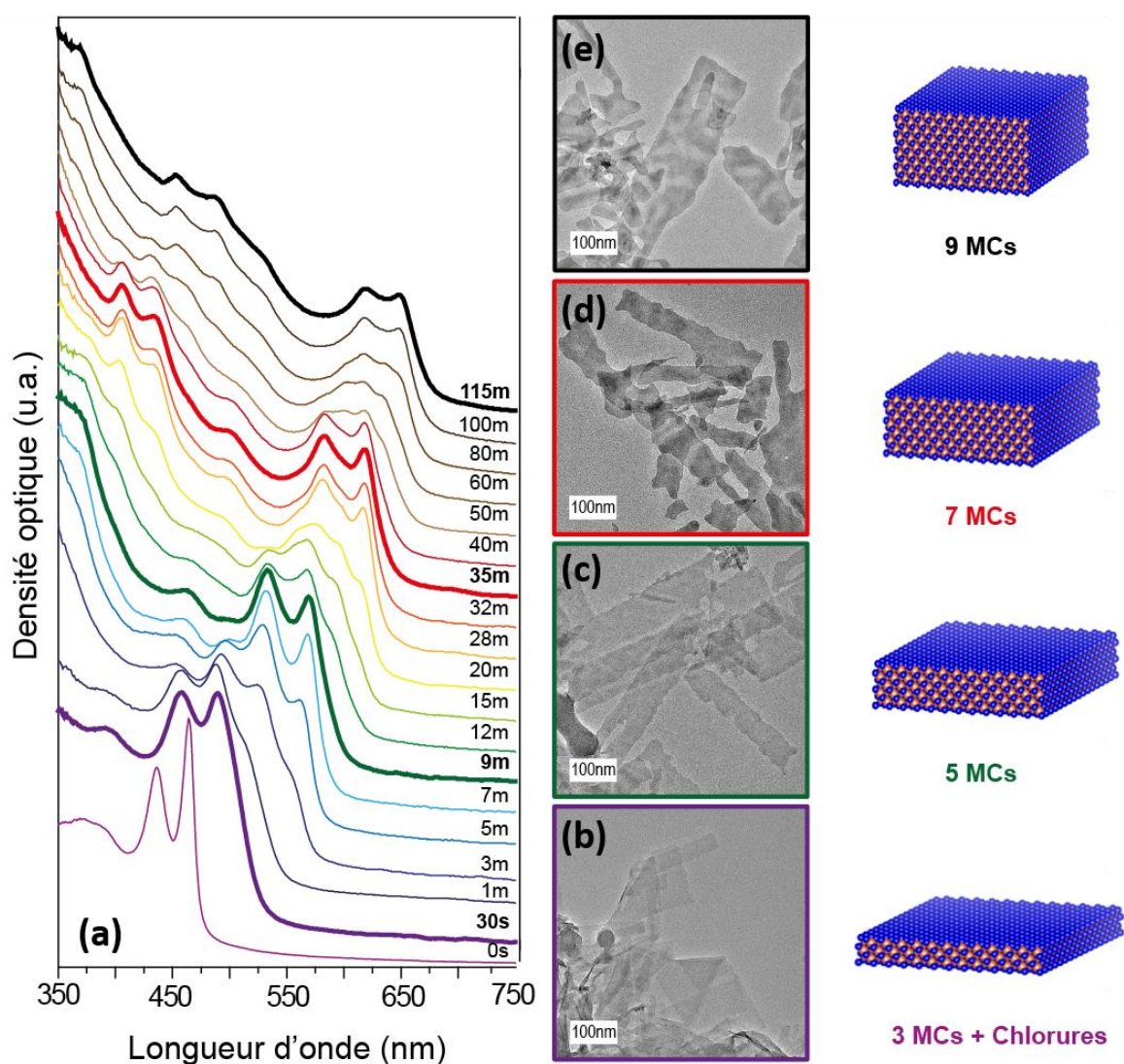
Figure 27 : Croissance des NPLs de CdSe 3 MCs de grandes dimensions latérales. (a) Suivi de la cinétique de réaction par absorption. (b) Image de MET des CdSe 3 MCs après 30 secondes, avec les chlorures en surface. (c) Image de MET des CdSe 5 MCs après 9 minutes. (d) Image de MET des 7 MCs après 35 minutes. (e) Image de MET des 9 MCs après quasiment 2 heures.
