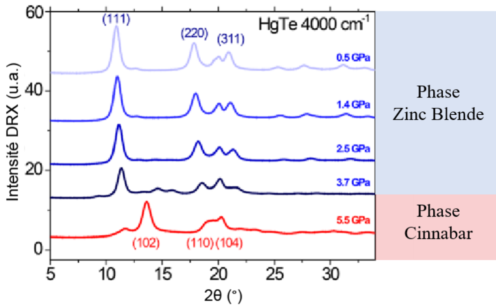
Figure 65: Diffractogrammes de NCs de HgTe sous pression de 0 GPa à 5,5 GPa. Issue de Livache et al. 140
