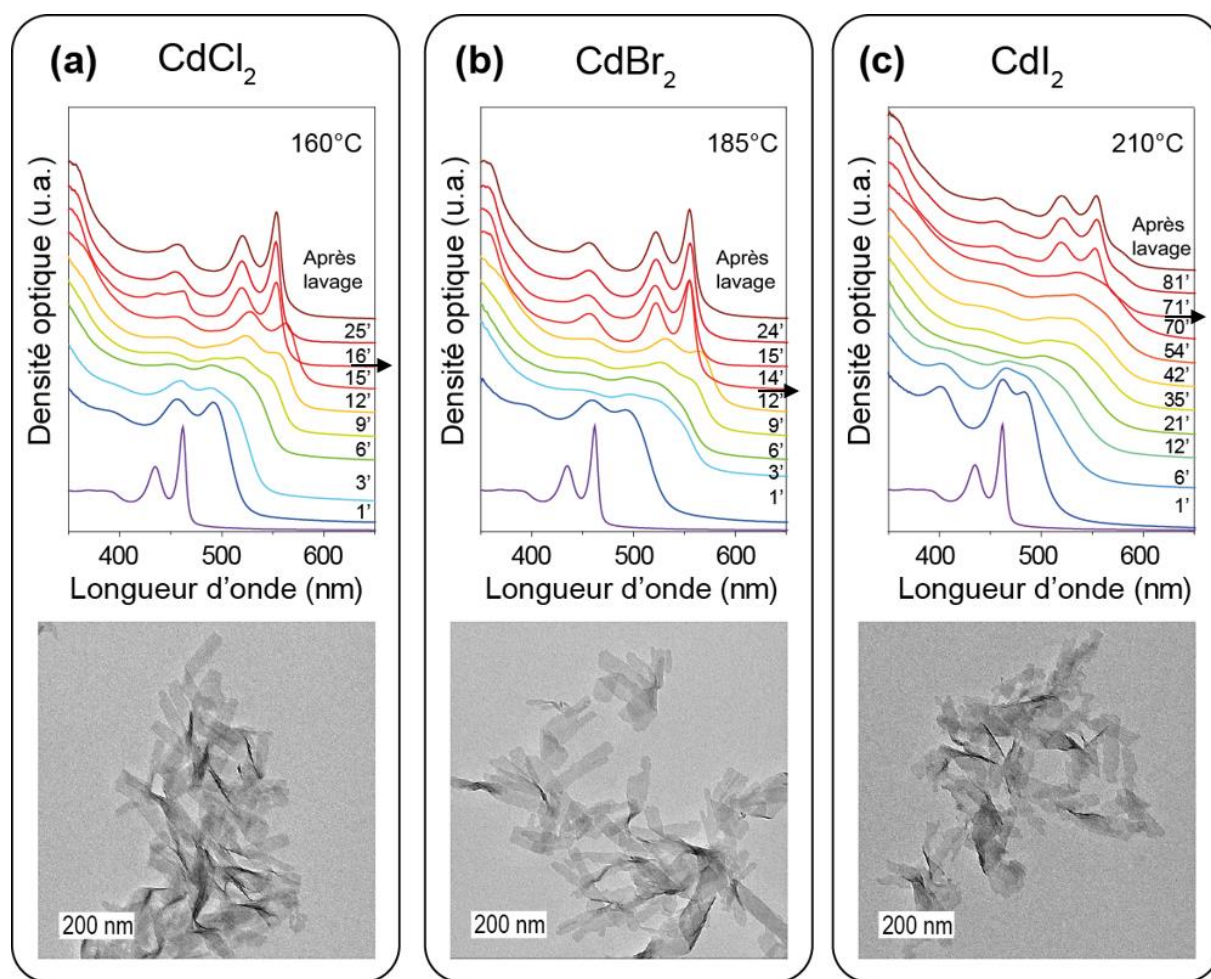
Figure 34 : Croissance de NPLs de CdSe 5 MCs à partir de CdSe 3 MCs avec différents halogénures. Suivi en absorption de la cinétique de réaction et image MET des NPLs 5 MCs finales avec respectivement l'utilisation du (a) chlorure de cadmium, (b) bromure de cadmium, (c) iodure de cadmium. Les flèches noires représentent le moment où l'acétate de cadmium en poudre (30 à 40 mg) a été ajouté à la solution.
