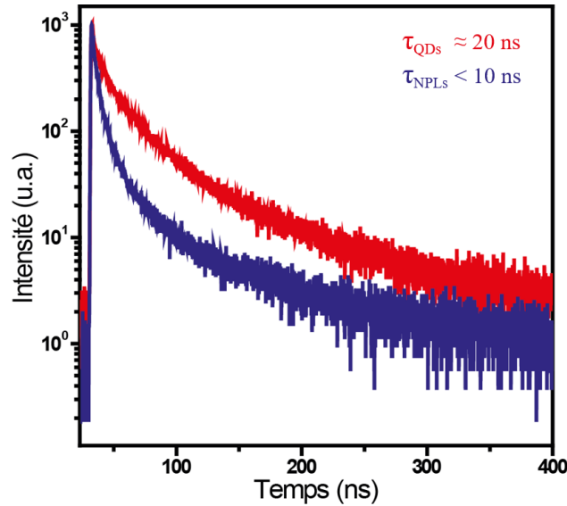
Figure 11: Comparaison du temps de vie de fluorescence entre des NPLs de CdSe et QDs de CdSe de largeur de bande interdite équivalente.
