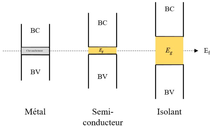
Figure 1 : Représentation des différents types de matériaux. De gauche à droite. Un semi-métal, où les deux bandes se touchent. Les semi-métaux sont caractérisés par un gap négatif. Un semi-conducteur, où la bande de valence et de conduction sont séparées par une largeur de bande interdite. Il n'y a passage de courant que par apport d'énergie permettant de traverser ce potentiel. Enfin, les isolants, où la largeur de bande interdite est trop importante pour permettre un passage du courant.
