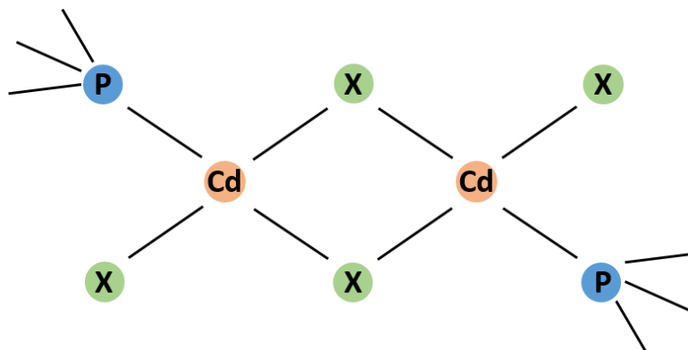
Figure 31 : Schéma représentatif du complexe de TBP:CdX 2 .
