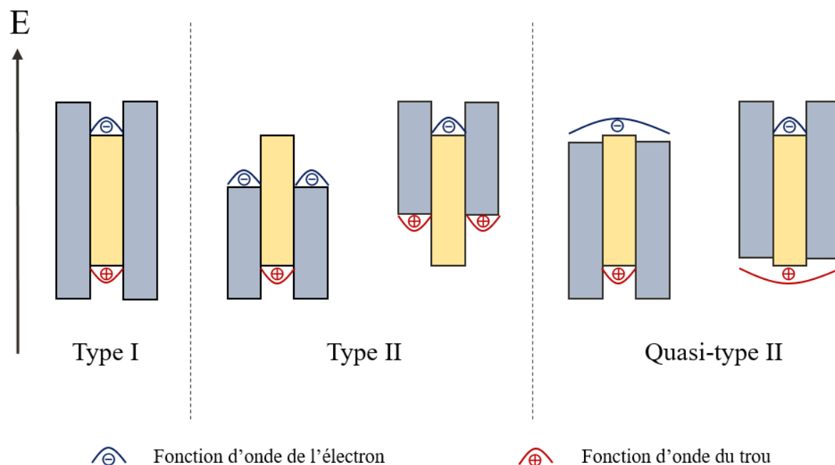
Figure 19 : Représentation des différents alignements de bande des hétérostructures de type cœur/coque. De gauche à droite. Type I, les fonctions d'onde des deux porteurs de charge sont confinées dans le matériau de cœur. Comme CdSe/ZnS. Type II, les fonctions d'onde des porteurs de charge sont confinées dans un matériau différent. Comme CdTe/CdSe ou CdSe/CdTe. Quasi-type II, la fonction d'onde d'un des porteurs de charge est délocalisée dans les deux matériaux alors que l'autre reste confinée dans le cœur. Comme CdSe/CdS.
