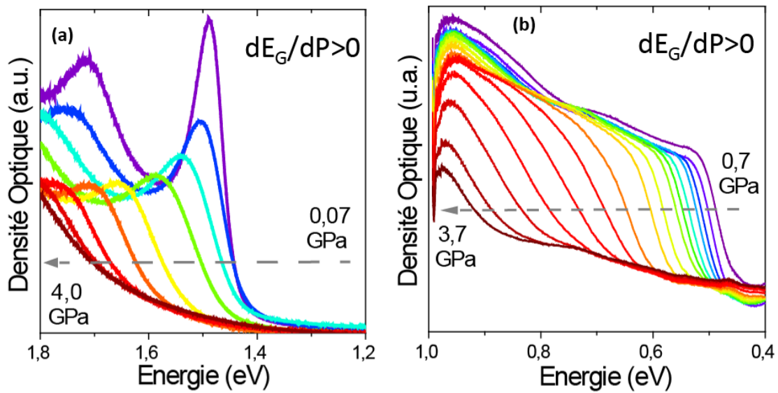
Figure 68: Evolution du premier pic excitonique des (a.) NPLs de HgTe à 200 K et (b.) NCs de HgTe à 300 K en énergie, en fonction de la pression de 0 à 4 GPa. Issue de Livache et al. 140 .
