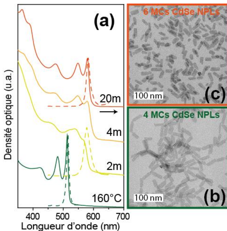
Figure 47: (a) Suivi cinétique en absorption du passage de CdSe 4 MCs à 6 MCs. (b) Image de microscopie électronique à transmission des NPLs initiales de 4 MCs et (c) NPLs finales de 6 MCs.
