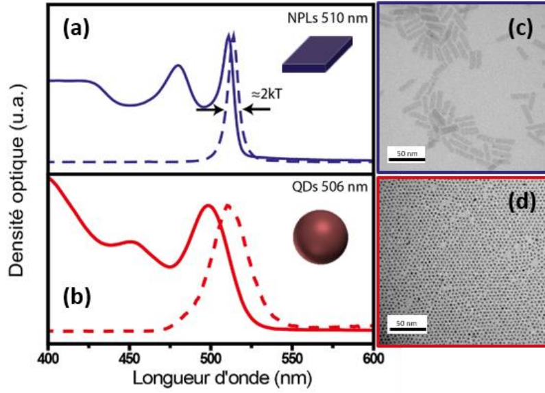
Figure 10: (a) En bleu, le spectre d'absorption (trait plein) et d'émission (tirets) de NPLs de CdSe 4 MCs. (b) En rouge, le spectre d'absorption (trait plein) et d'émission (tirets) de QDs de largeur de bande interdite équivalente aux NPLs. (c) et (d) images au microscope électronique à transmission de NPLs de CdSe 4 MCs et de QDs de CdSe.
