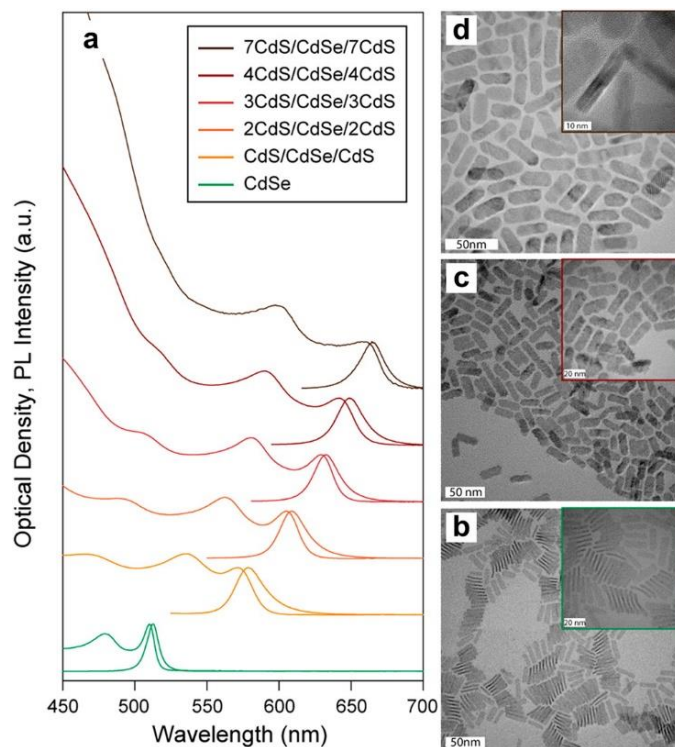
Figure 21 : A gauche spectre d'absorption et d'émission des NPLs de CdSe de cœur et de chaque cœur/coque avec n couche de CdS ( n de 1 à 7). La coque étant de plus en plus épaisse, le confinement est de plus en plus faible et donc les propriétés optiques sont décalées vers le rouge. A droite, images au MET des (b) CdSe 4 MCs, (c) n = 4 MCs de CdS (d) n = 7 MCs de CdS. La bidimensionnalité est maintenue tout au long de la c-ALD. Reproduit de Ithurria et al. 54 .
