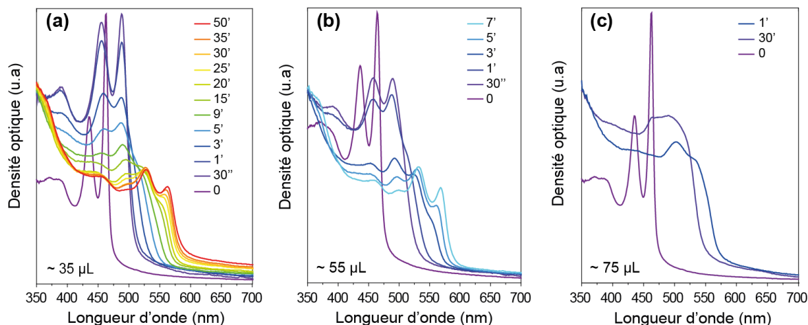
Figure 32 : Suivi cinétique en absorption sur plusieurs minutes de la croissance en épaisseur de NPLs de CdSe larges de 3 MCs à 160 °C avec (a) 35 µL, (b) 55 µL et (c) 75 µL d'une solution de TBP:CdCl 2 à 0,5 M.
