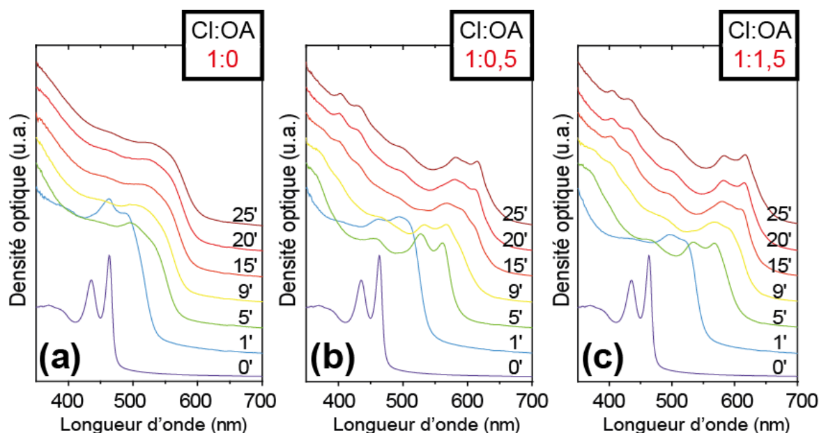
Figure 35 : Croissances des NPLs de CdSe 7 MCs à partir de CdSe 3 MCs avec différents ratios de chlorures/acide oléique. Suivi en absorption de la réaction avec les ratios Cl:AO respectivement de (a) 1:0, (b) 1:0,5, (c) 1:1,5.
