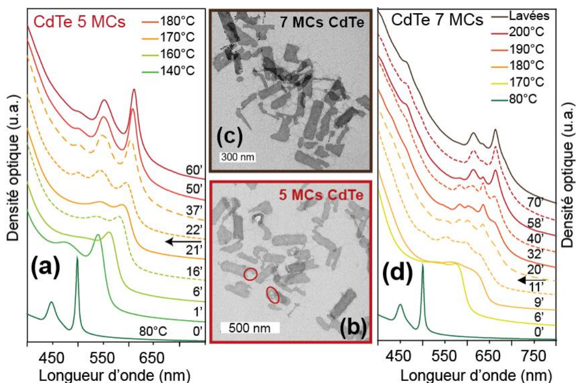
Figure 50 : D/R sur les NPLs de CdTe de 3 MCs. (a) Suivi cinétique en absorption de la croissance de 3 à 5 MCs des NPLs de CdTe. (b) image de microscopie électronique à transmission des NPLs de CdTe finales de 5 MCs. (d) Suivi cinétique en absorption de 3 à 7 MCs des NPLs de CdTe. (c) image de microscopie électronique à transmission des NPLs de CdTe finales de 7 MCs.
