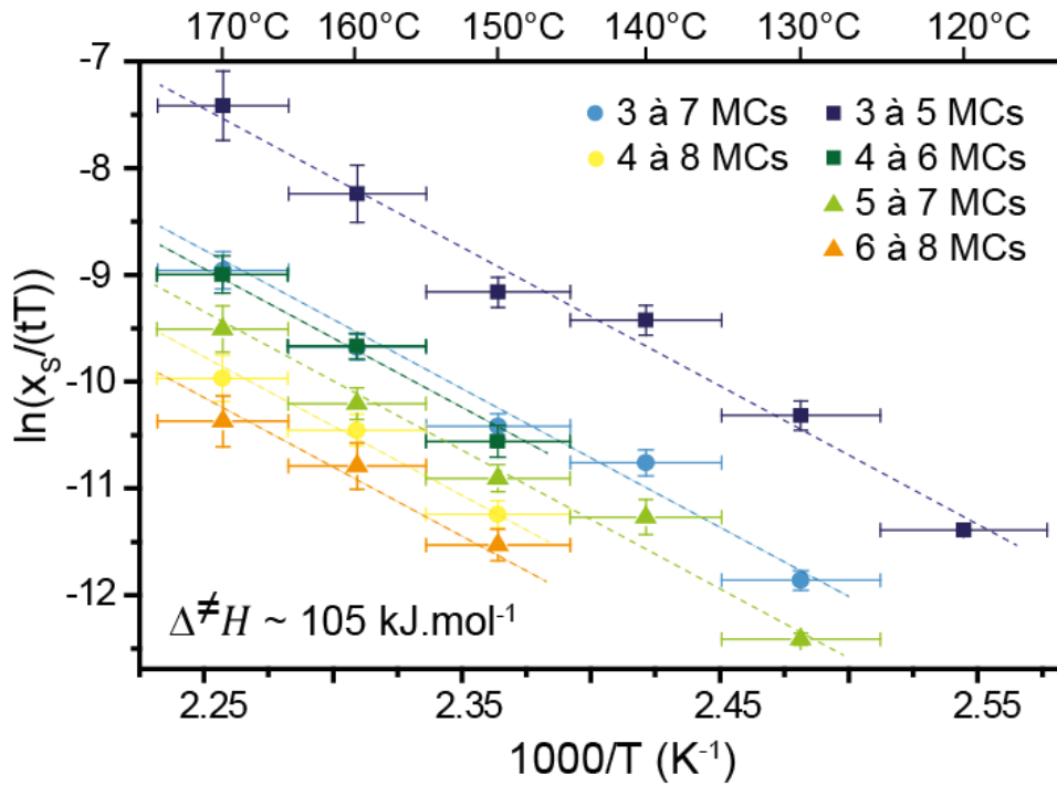
Figure 45 : Inverse du temps de passage de N à N+2 MCs en fonction de l'inverse de la température de croissance selon la loi d'Eyring.
