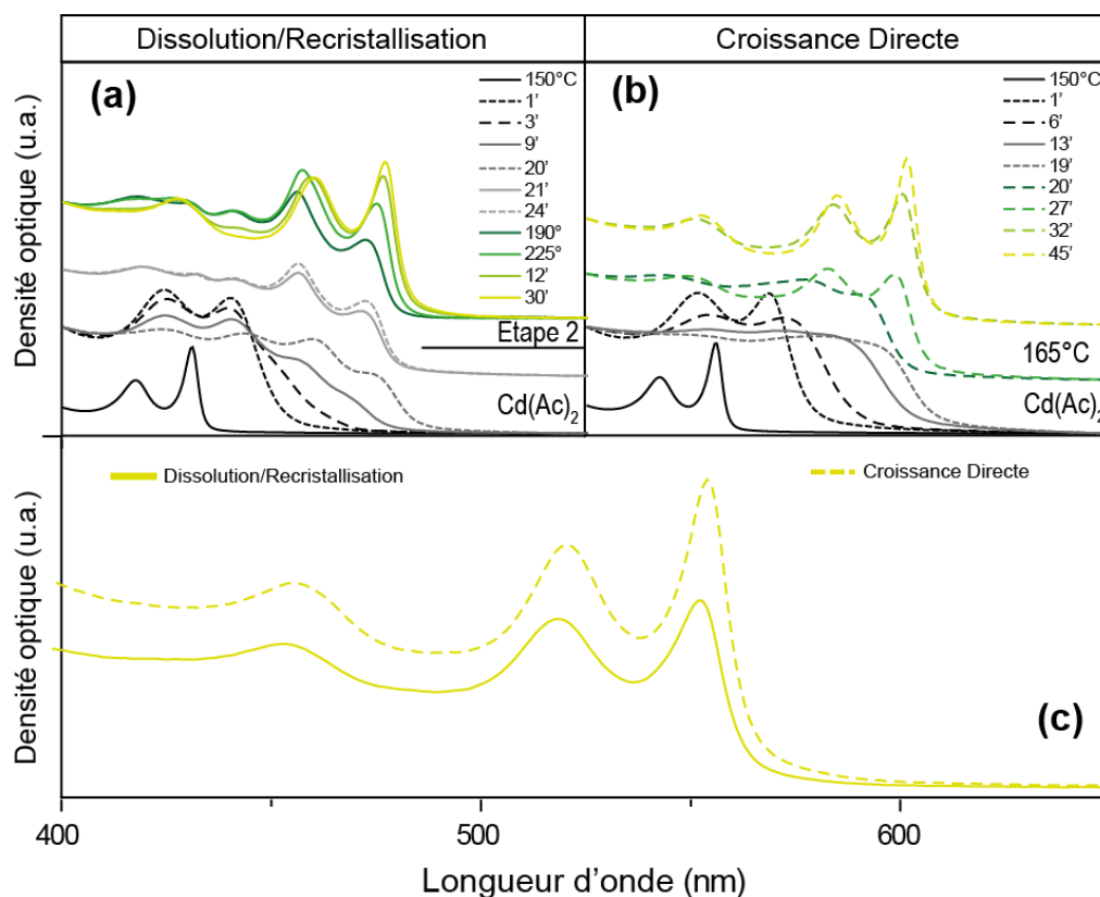
Figure 53: (a) Obtention en 2 étapes de CdSe 5 MCs. La dissolution/recrystallisation permet de synthétiser des CdSe 5 MCs. La seconde étape est un recuit sur les NPLs synthétisées et lavées. Ceci permet d'obtenir des NPLs de 5 MCs d'une meilleure cristallinité. (b) Obtention de CdSe 5 MCs à partir de 3 MCs, via une croissance directe. (c) Comparaison des 2 spectres d'absorption des CdSe 5 MCs obtenus en fin de réaction via les 2 méthodes. En trait plein méthode de D/R et pointillé méthode de croissance directe.
