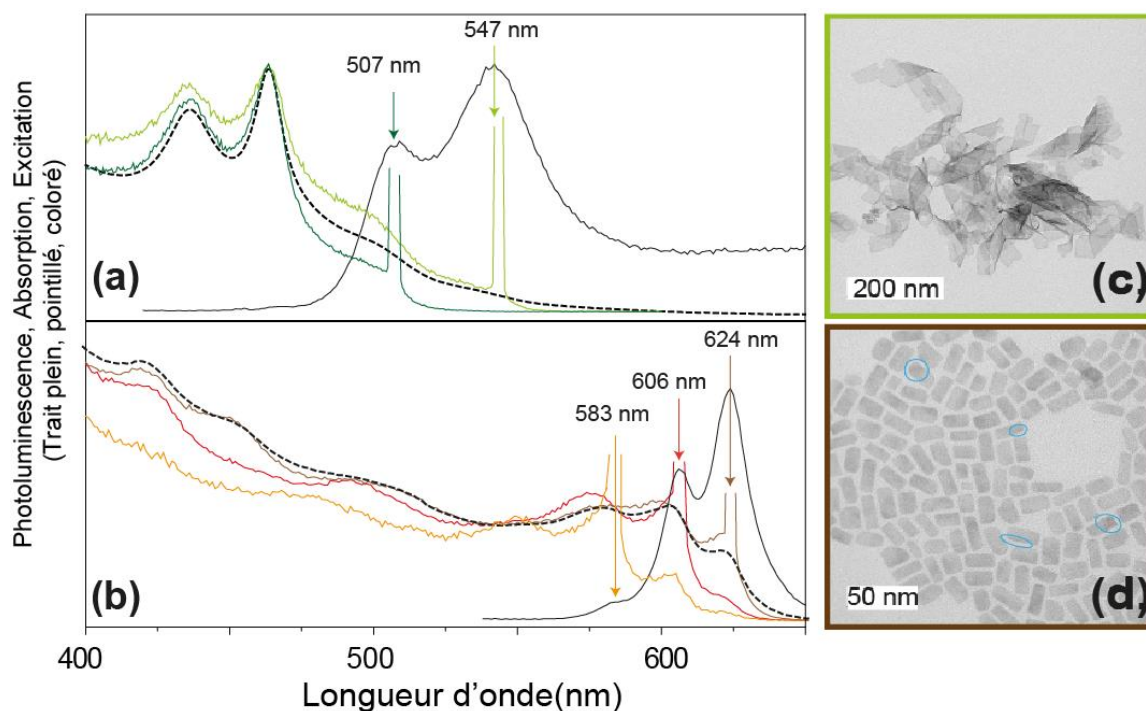
Figure 55 : Absorption, émission et excitation des NPLs de CdSe (a) 3 MCs avec marches de 4 MCs et 5 MCs et (b) 6 MCs avec marches de 7 MCs et 8 MCs. (c) et (d) images TEM respectives, après ajout de l'acétate de Cadmium et lavage.
