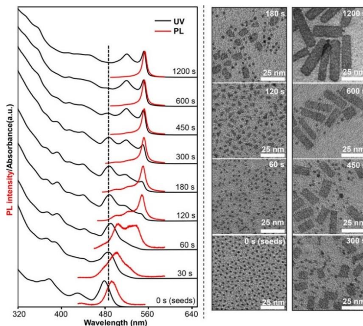
Figure 15 : A gauche, suivi cinétique en absorption (noir) et en émission (rouge) du passage des QDs de CdSe en NPLs de CdSe. Le spectre d'absorption des QDs diminue d'intensité au cours du temps, et celui des NPLs de 5 MCs à 555 nm apparaît petit à petit. A droite, suivi par imagerie au microscope électronique à transmission du passage des QDs aux NPLs. Reproduit de Chen et al. 48 .
