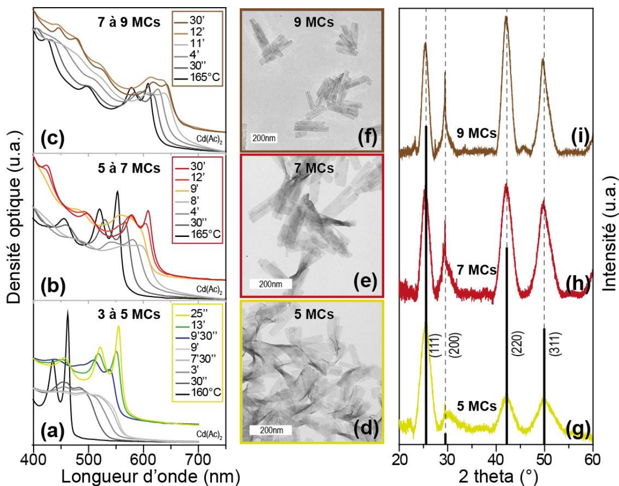
Figure 51 : Croissance directe des NPLs de CdSe de 3 MCs à 7 MCs. Suivi en absorption du passage de (a) 3 à 5 MCs, (b) 5 à 7 MCs et (c) 7 à 9 MCs. Les images MET des NPLs finales de (d) 5 MCs, (e) 7 MCs, (f) 9 MCs. Les NPLs montrent des bords bien définies et pas de trous en surface. Les diffractogrammes confirment aussi la conservation de la phase zinc-blende pour toutes épaisseurs (g) 5 MCs, (h) 7 MCs, (i) 9 MCs. L'intensité peut varier avec la modification de l'orientation des NPLs en fonction de l'épaisseur.
