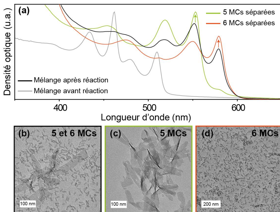
Figure 40 : Suivi de la cinétique de réaction en absorption pour un mélange d'épaisseurs 3 MCs et 4 MCs. (a) Spectre d'absorption du mélange avant et après croissance ainsi que les spectres après lavage des NPLs de CdSe de 4 MCs et 6 MCs. Images MET du mélange (b) avant séparation, (c) des 5 MCs après séparation et (d) des 6 MCs après séparation.
