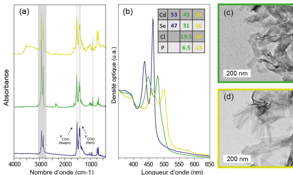
Figure 33 : (a) Spectroscopie infrarouge des NPLs de CdSe 3 MCs passivées par des carboxylates en bleu, des chlorures (1:1) en vert et chlorures (2:1) en jaune. (b) Les spectres d'absorption respectifs des échantillons précédents. (c) et (d) images MET des CdSe passivées par les chlorures avec les 2 différents ratios.
