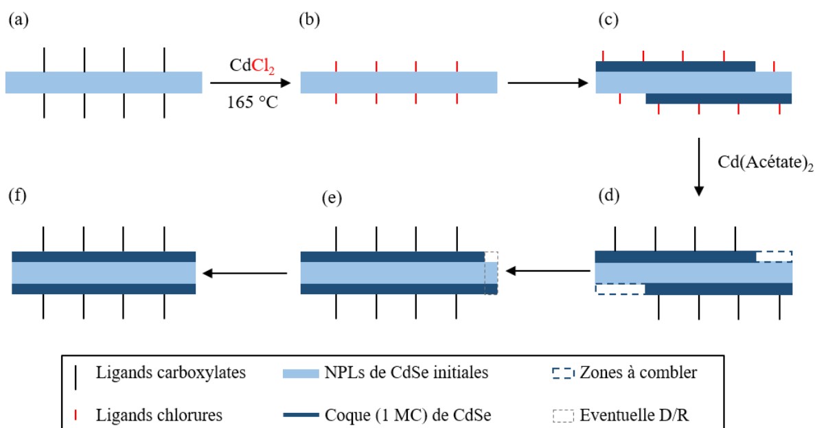
Figure 52: Proposition de mécanisme pour la croissance directe sur des NPLs de CdSe 3 MCs. (a) NPLs initiales passivées par des carboxylates. (b) Injection du chlorure de cadmium à 165 °C, rapidement suivi par un échange de ligands entre carboxylates et chlorures. La surface est dite activée. L'acide oléique n'est pas représenté ici mais il costabilise l'halogénure. (c) 1 MC de CdSe cristallise de part et d'autre du cœur de CdSe. La coque recouvre ici plus de 50 % des surfaces larges. (d) Quenching de la réaction par l'acétate de cadmium. Les halogénures sont remplacés par les carboxylates. La croissance des coques n'est pas complète mais la présence de monomères de CdSe en solution permet d'achever les coques. Les NPLs présentent ici des marches (e) Il peut encore subsister des zones partiellement complétées. C'est à ce stade qu'il peut se produire de la D/R. Cela ne reste qu'une hypothèse. (f) NPLs finales de CdSe 5 MCs.
