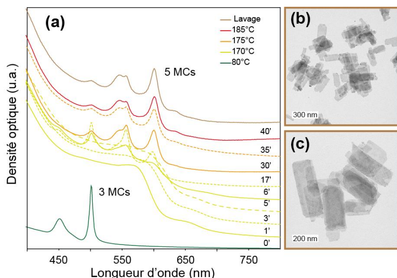
Figure 57: (a) Suivi cinétique par absorption de la croissance directe d'une monocouche de CdTe de part et d'autre de NPLs de CdTe 3 MCs. Après 40 minutes, la population principale est celle des 5 MCs mais son isolation n'est pas parfaite. (b) et (c) images MET des NPLs finales. Elles sont très peu dégradées avec des bords bien définis. La dissolution est inhibée.
