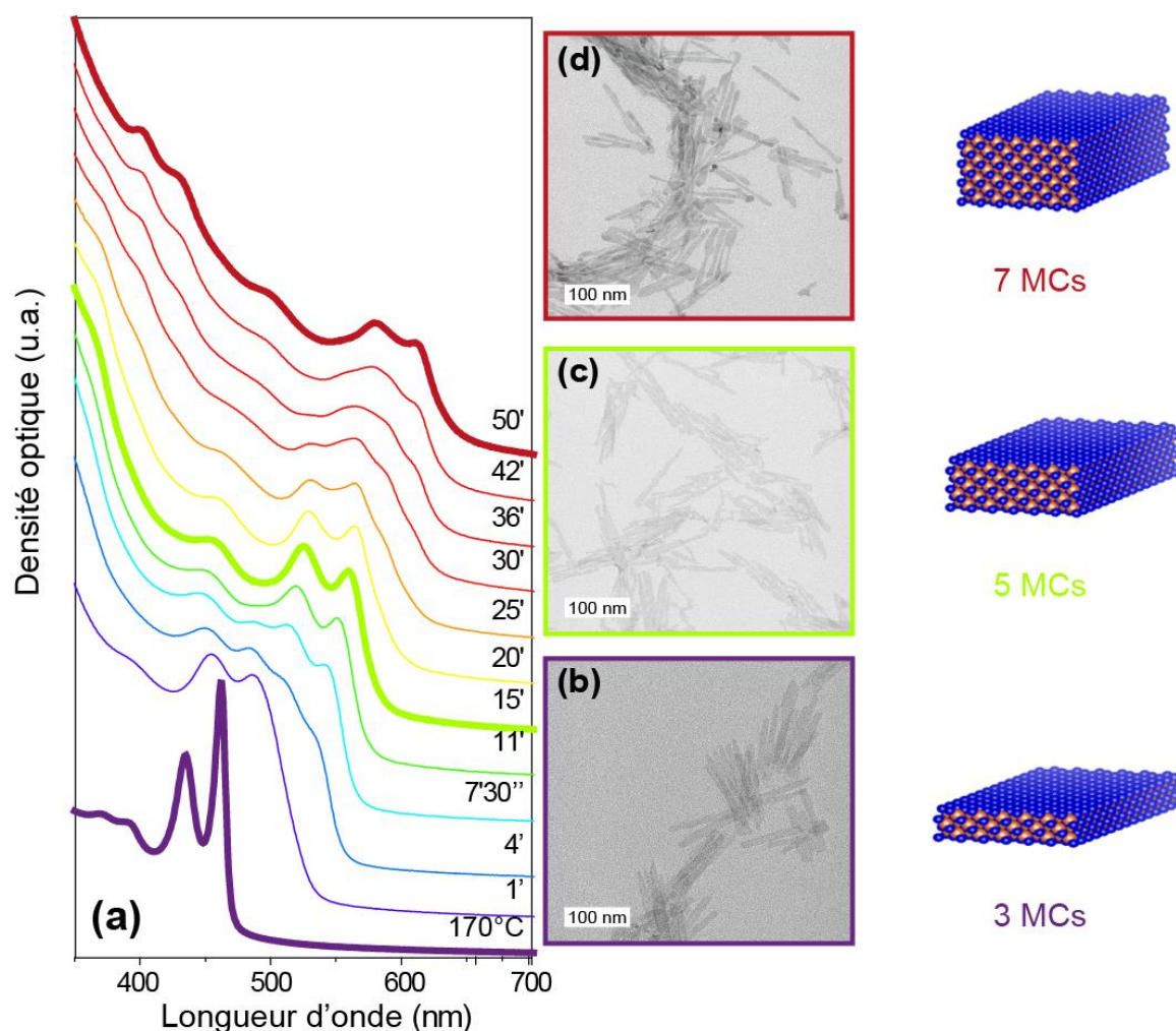
Figure 28 : Croissance des NPLs de CdSe 3 MCs de petites dimensions latérales. (a) Suivi de la cinétique de réaction par absorption. (b) image MET des CdSe 3 MCs initiales. (c) Image MET des 5 MCs après 15 minutes. (d) Image MET des 7 MCs après 50 minutes.
