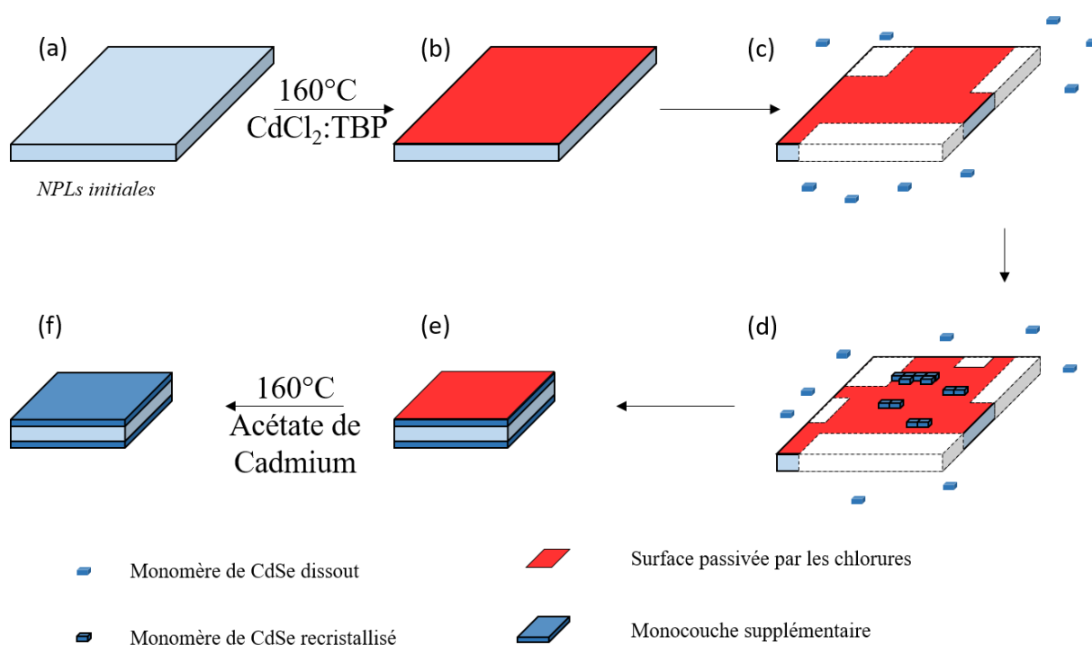
Figure 39 : Schéma représentatif du mécanisme de D/R permettant l'obtention de NPLs de N+2 MCs à partir de N MCs. (a) NPLs initiales de N MCs (avec N = 3 par exemple). (b) NPLs initiales de 3 MCs passivées par les chlorures.
