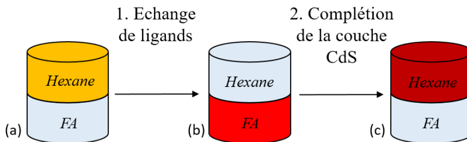
Figure 20 : Différentes étapes de la c-ALD. (a) Les NPLs sont dans la phase apolaire (hexane). (b) Après échange de ligands au soufre, la surface est chargée négativement et passe donc en phase polaire dans le formamide. (c) L'ajout d'un précurseur d'acétate conjointement avec un ligand oléate permet de compléter la couche de CdS et d'apporter la neutralité en surface. Une solution stable colloïdalement se reforme en phase apolaire hexane. Les NPLs étant de plus en plus épaisses, la coloration de la solution passe de jaune à rouge puis à rouge foncé.
