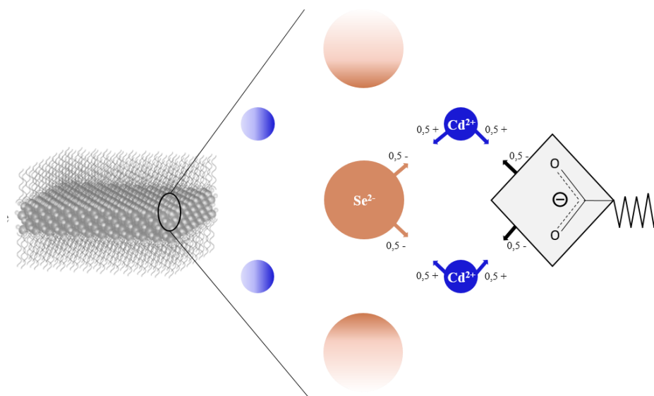
Figure 8 : Focus sur la liaison d'un ligand carboxylate avec la surface d'une NPL de CdSe. La tête polaire est pontant entre deux Cd de surface.
