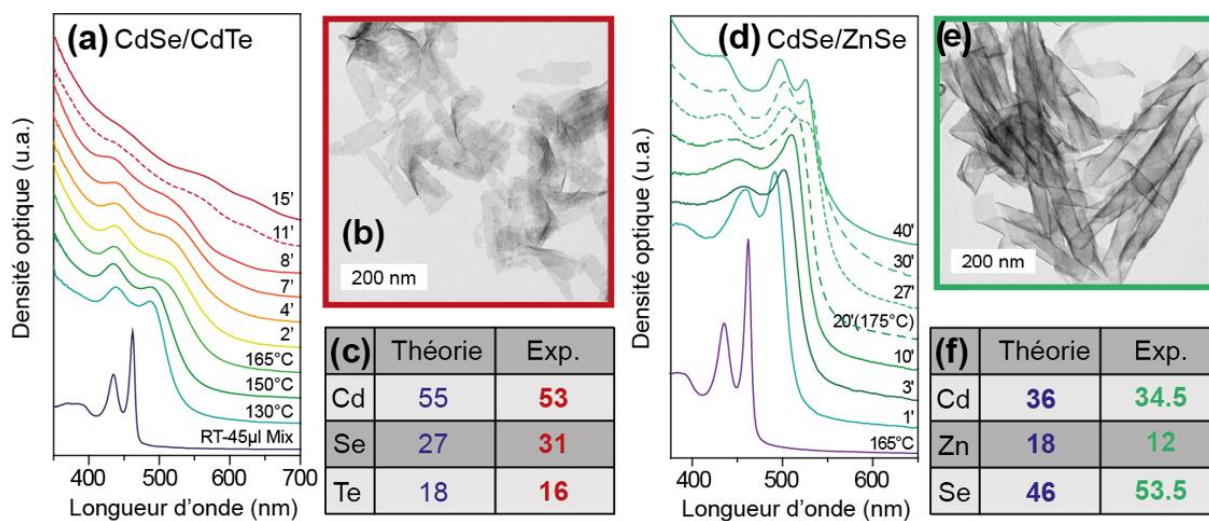
Figure 58 : Suivi cinétique de la réaction par absorption de la croissance de (a) CdTe et (d) ZnSe, sur des NPLs de cœur de CdSe. (b) et (d) représentent les images MET des hétérostructures obtenues. La dimension 2D est conservée dans les 2 cas. Les contraintes apportées par les ligands carboxylates sur la couche de Zinc tendent à enrrouler les NPLs de CdSe/ZnSe. (c) et (f) récapitulent les ratios atomiques théoriques et mesurés des cœurs de CdSe 3 MCs, avec une couche de part et d'autre de CdTe et ZnSe respectivement.
