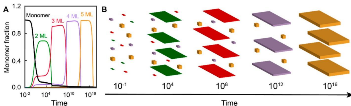
Figure 18 : (A) Evolution de la fraction molaire de CdSe en fonction du temps. Le modèle prédit la croissance des NPLs les plus fines d'abord. Puis leur dissolution en faveur des NPLs plus épaisses d'une monocouche. (B) représentation du phénomène de mûrissement. La réaction est cinétiquement en faveur de l'extension latérale des NPLs les plus fines. A temps long les NPLs les plus épaisses sont favorisées et atteintes par mûrissement. Reproduit de Knüsel et al. 52 .
