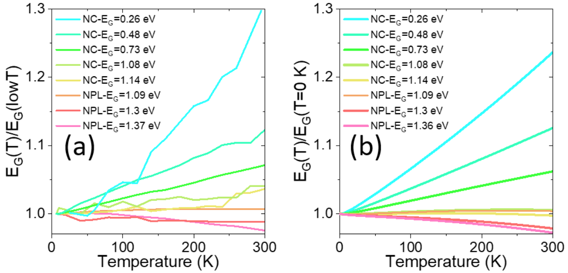
Figure 72 : (a) Mesures expérimentales du décalage du gap en fonction de la température pour des NCs de tailles différentes et NPLs de chimie de surface différentes. (b) Simulation de (a).
