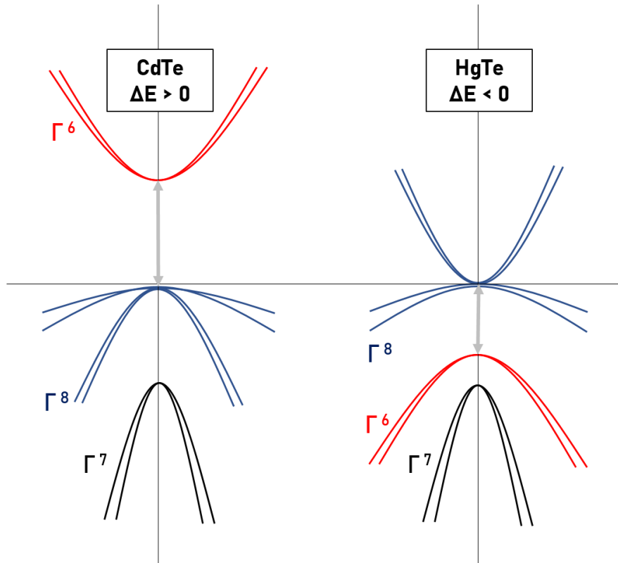
Figure 69: Structure de bande de CdTe (a) et HgTe (b).
