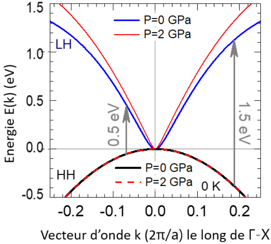
Figure 74 : Evolution de la LH et de la HH pour les QDs (faible énergie) et NPLs (haute énergie) de 0 et 2 GPa. Simulations issues du modèle à 3+1 bandes.
