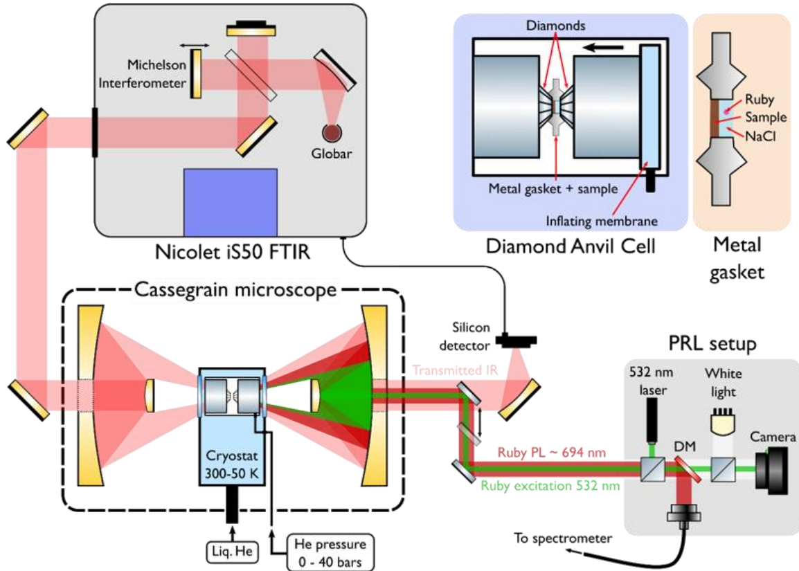
Figure 67: Schéma représentatif du montage expérimental au synchrotron SOLEIL pour la mesure des spectres d'absorption en pression à différentes températures.
