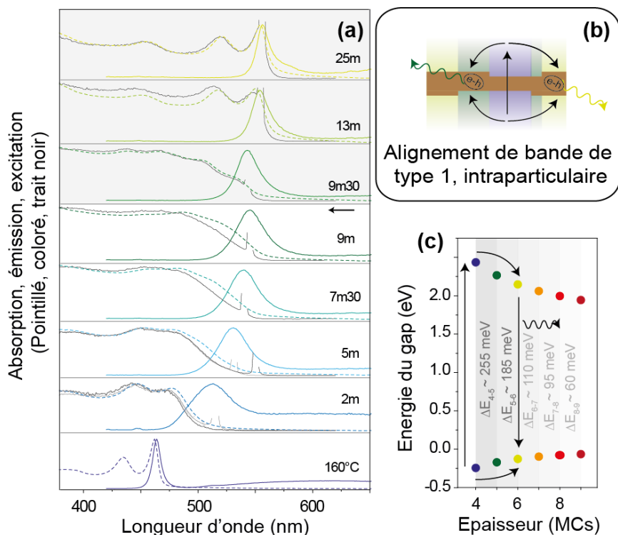
Figure 54: (a) Absorption, émission et excitation d'échantillons de NPLs de CdSe 3 MCs durant une croissance à 5 MCs. (b) Représentation d'une NPL à marches, avec un alignement de type induit par le confinement. L'exciton se recombine favorablement dans les zones les plus épaisses. (c) Énergie de gap des NPLs de CdSe d'épaisseurs variables. Valeurs issues de Dufour et al. 61 .
