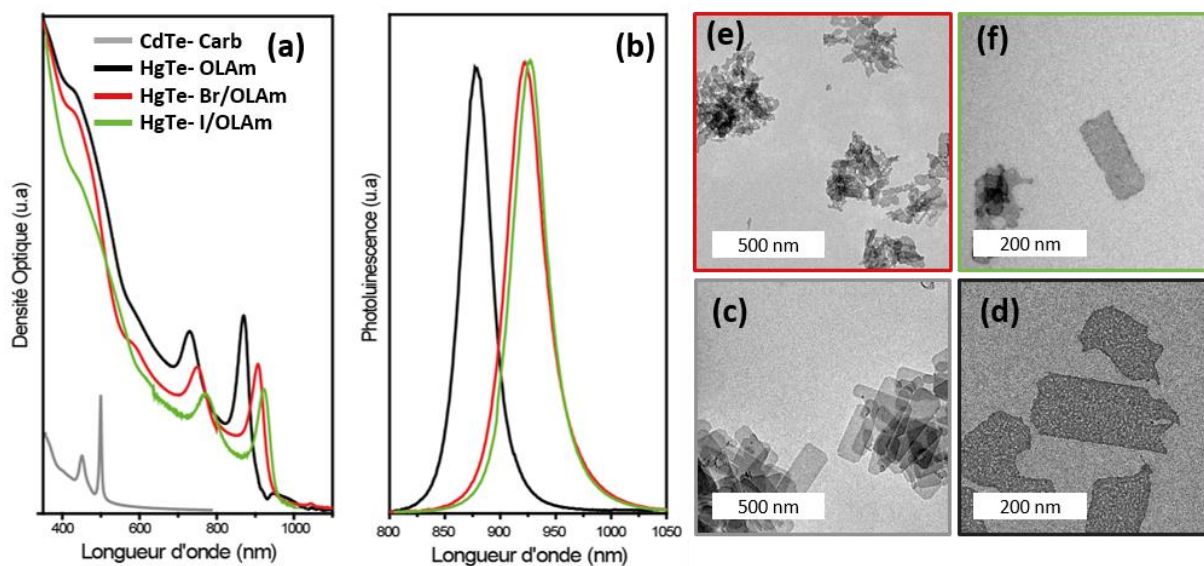
Figure 60 : (a) : Spectres d'absorption des NPLs de CdTe 3 MCs (gris) passivées par des carboxylates, de HgTe 3 MCs après échange cationique (noir) passivées par de l'oleylamine, de HgTe 3 MCs après échange de ligands par Br/OLAm (rouge) et de HgTe 3 MCs après échange de ligands par I/OLAm. (b) Spectres d'émission des NPLs de HgTe-OLAm (noir), HgTe-Br/OLAm (rouge) et HgTe-I/OLAm (vert). Images au MET des NPLs de (c) CdTe 3 MCs, (d) HgTe 3 MCs (e) HgTe 3 MCs après échange de ligands au bromure et (f) HgTe 3 MCs après échange de ligands à l'iode.
