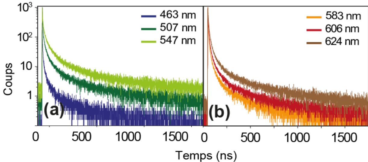
Figure 56 : Mesure de temps de vie de fluorescence à différentes longueurs sur les NPLs de CdSe (a) 3 MCs avec marches et (b) 6 MCs avec marches. Pour (a) les longueurs d'onde d'intérêt sont celles du premier pic excitonique des 3 MCs, 4 MCs et 5 MCs. Pour (b) des 6 MCs, 7 MCs et 8 MCs.
