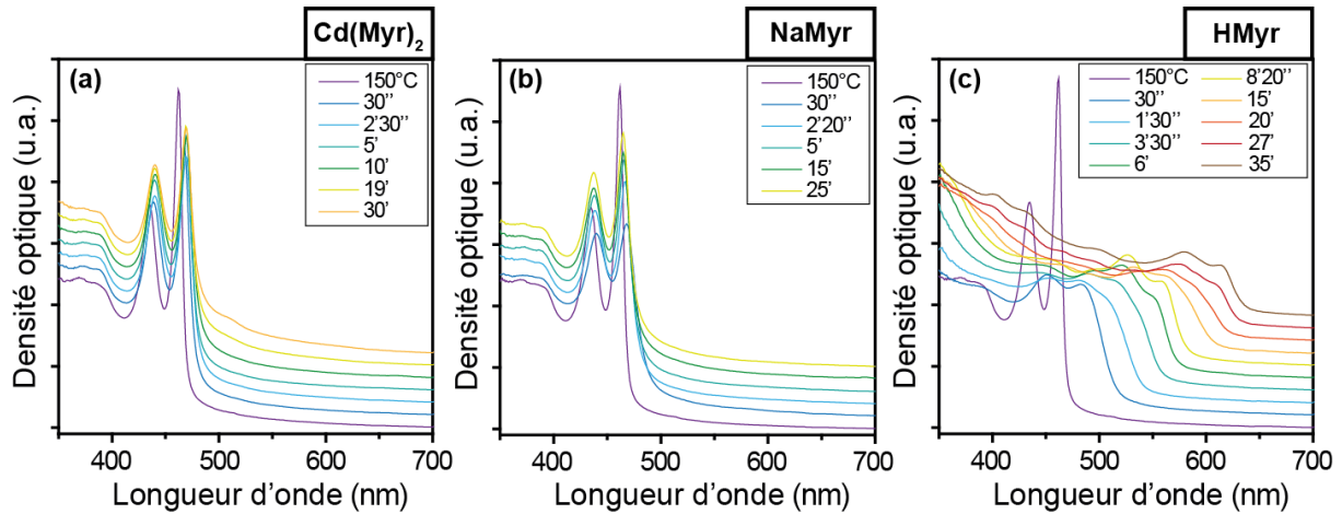
Figure 36 : Croissance de CdSe 3 MCs en fonction de la nature du ligand ajouté. (a) Myristate de Cadmium, (b) Myristate de Sodium, (c) Acide Myristique.
