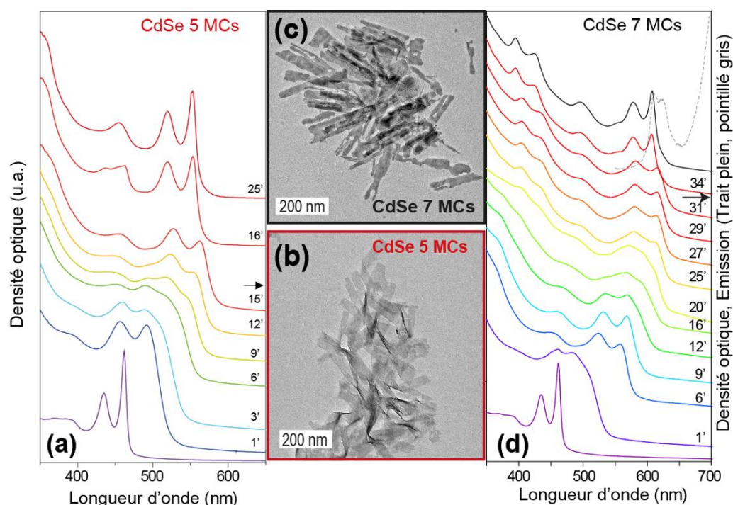
Figure 46: (a) Suivi cinétique en absorption du passage des NPLs de CdSe 3 MCs à 5 MCs. L'ajout de l'acétate de cadmium à 15 minutes est représenté par une flèche noire (b) Image de microscopie électronique à transmission des NPLs finales de 5 MCs. (c) Image de microscopie électronique à transmission des NPLs finales de 7 MCs. (d) Suivi cinétique en absorption du passage de 3 MCs à 7 MCs. L'ajout de l'acétate de cadmium à 31 minutes est représenté par une flèche noire. Emission en pointillé.
