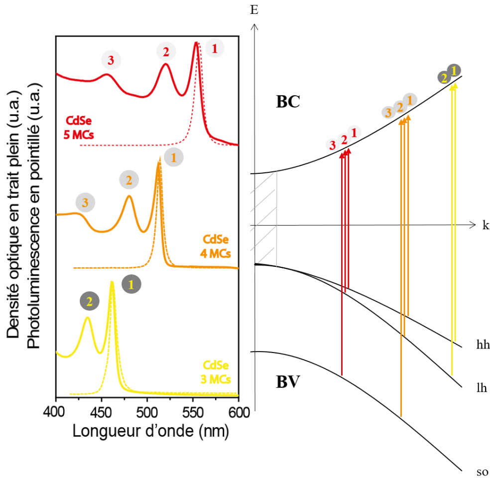
Figure 9 : A gauche, spectres d'absorption (trait plein) et d'émission (tirets) des NPLs de CdSe 3 MCs, 4 MCs et 5 MCs. Les différentes transitions (trou lourd-électron, trou léger-électron, spin orbite-électron) sont notées respectivement 1, 2 et 3. Pour les NPLs de CdSe 3 MCs la transition électron spin orbite n'est pas représentée (inférieure à 400 nm). Les mêmes transitions sont représentées à droite sur la structure de bande simplifiée d'une nanoplaquette de CdSe.
