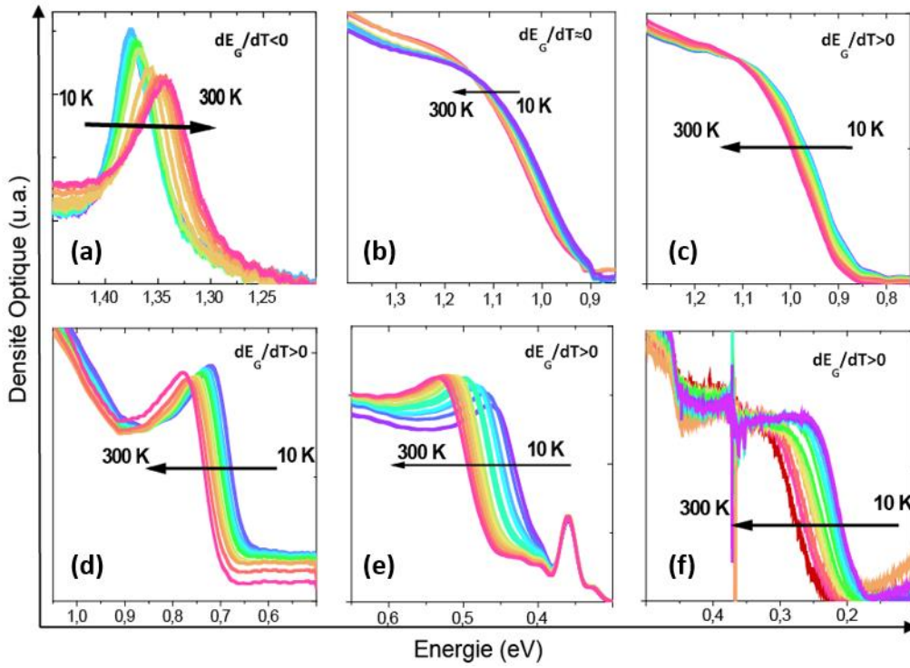
Figure 64: Influence de la température sur le premier pic excitonique de 300 K à 10 k. (a) NPLs de HgTe 3 MCs. (b) QDs de HgTe 9k. (c) QDs de HgTe 8k. (d) QDs de HgTe 6k. (e) QDs de HgTe 4k. (f) QDs de HgTe 2k.
