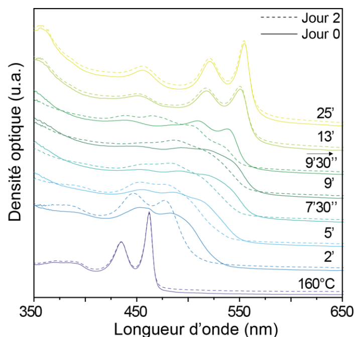
Figure 38 : Suivi cinétique par absorption sur plusieurs minutes de la croissance de NPLs de CdSe de 3 à 5 MCs. Spectres d'absorption en trait plein à j_0 et en pointillé à j+2 . Les mesures en absorption sont faites le jour même et à j+2 .
