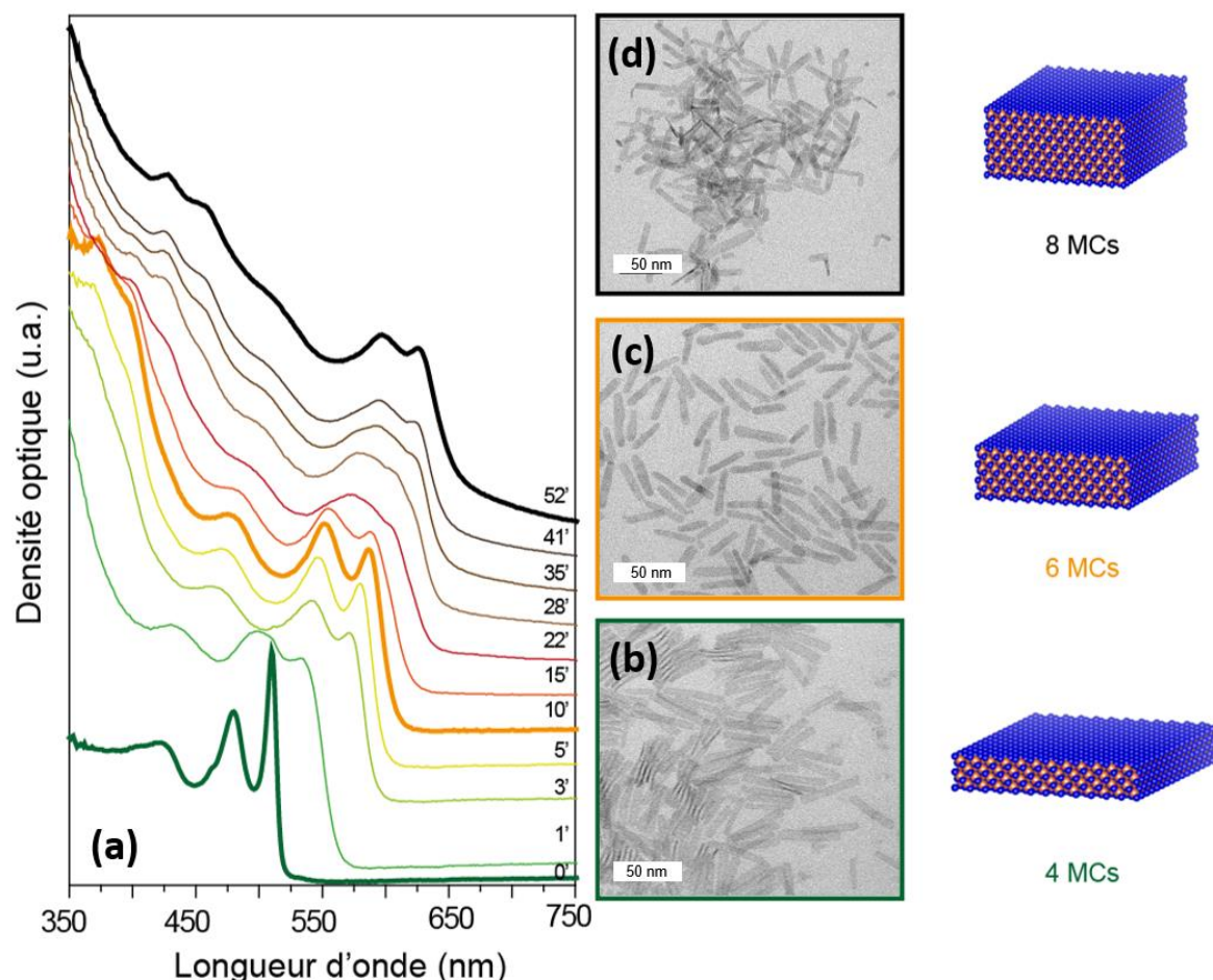
Figure 29 : Croissance des NPLs de CdSe 4 MCs de petites dimensions latérales. (a) Suivi de la cinétique de réaction par absorption. (b) Image MET des CdSe 4 MCs initiales. (c) Image MET des 6 MCs après 10 minutes. (d) Image MET des 8 MCs après 52 minutes.
