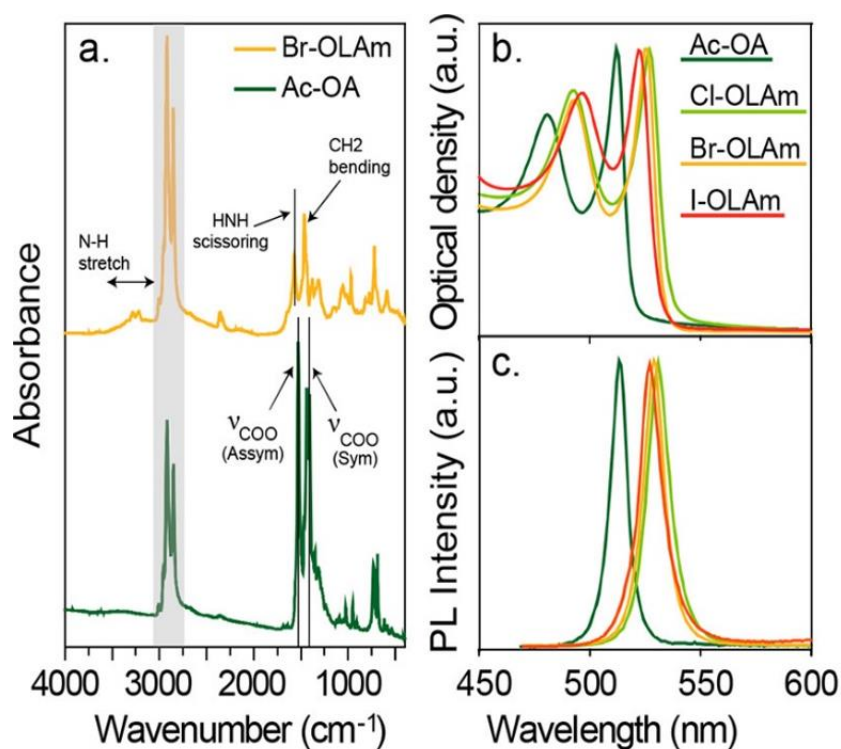
Figure 23 : Spectroscopie infrarouge des NPLs de CdSe 4 MCs passivées par des carboxylates en vert et le mélange Bromure-Oleylamine en jaune permettant de mettre en évidence la liaison hydrogène. (b) Spectres d'absorption des NPLs de CdSe 4 MCs passivées par des carboxylates et les différents halogénures. Les transitions sont décalées vers le rouge pour chaque halogénure. (c) Spectres d'émission correspondants. Le même décalage est observé. Reproduit de Dufour et al. 61 .
