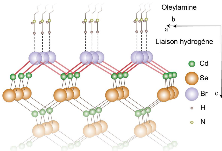
Figure 24 : Schéma représentatif de la passivation de la surface par des bromures costabilisé par la liaison hydrogène de l'amine. Ici, le bromure est en position pontant entre les Cd. Reproduit de Dufour et al. 61 .
