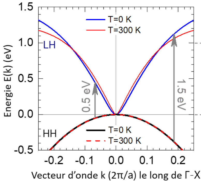
Figure 71: Evolution de la LH et de la HH pour les QDs (faible énergie) et NPLs (haute énergie) à 0 et 300 K. Simulations issues du modèle à 3+1 bandes.
