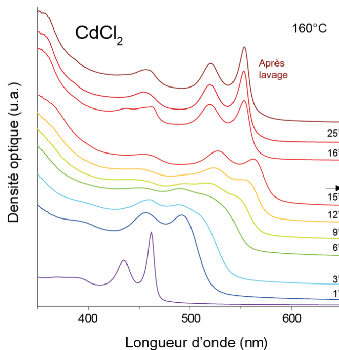
Figure 37 : Suivi cinétique en absorption de la croissance de NPLs de CdSe 5 MCs à partir de NPLs de CdSe 3 MCs. La réaction est arrêtée après 15 minutes par ajout d'acétate de cadmium (symbolisé par la flèche noire) et les NPLs de CdSe 5 MCs sont obtenues au bout de 25 minutes.
