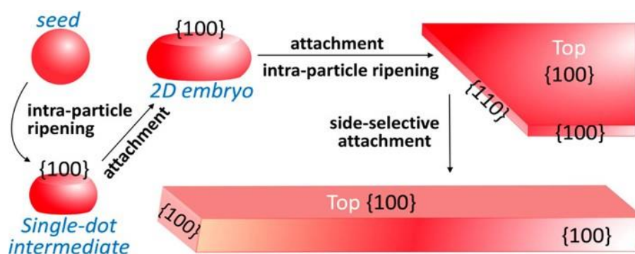
Figure 16 : Mécanisme de formation des NPLs de CdSe par attachement orienté des ligands en surface. Reproduit de Chen et al. 48 .
