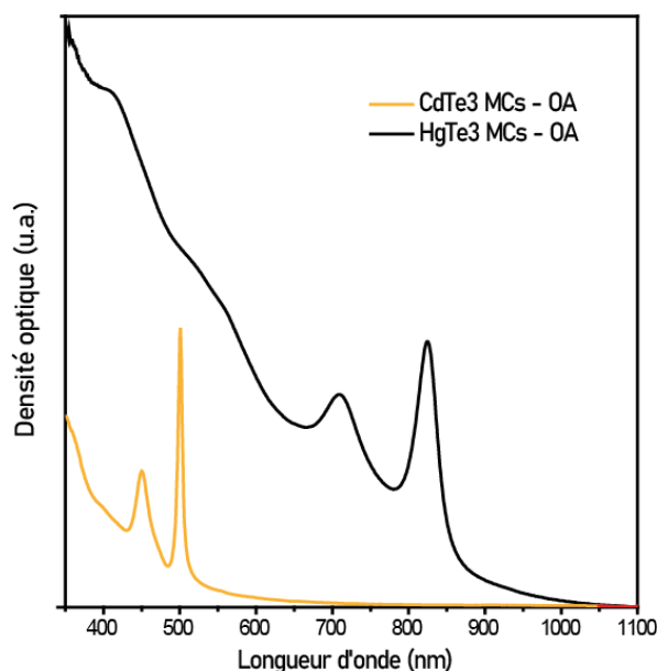
Figure 59 : Spectres d'absorption des NPLs de CdTe 3 MCs (orange) et de HgTe 3 MCs (noir) après échange cationique entre le cadmium et le mercure. Les NPLs sont ici passivées par de l'acide oléique.
