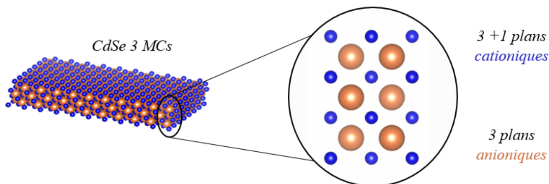
Figure 7 : Focus sur l'empilement de NPLs de CdSe 3 MCs. Avec une alternance de 3 plans anioniques et 3+1 plans cationiques.
