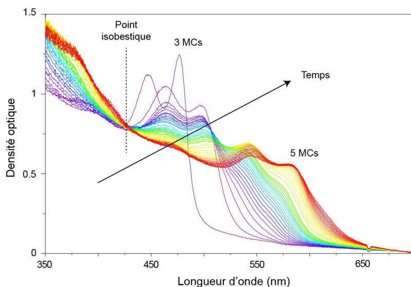
Figure 42 : Suivi d'une D/R de NPLs de CdSe 3 MCs en absorption via une sonde in situ dans le ballon. Les spectres ne sont pas normalisés et un point isobestique apparaît à 425 nm. Il y a donc conservation de matière.
