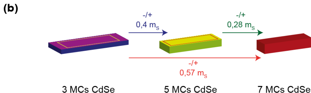
Figure 43: (a) La dissolution/Recristallisation se fait en 2 étapes. Dissolution des NPLs principalement par les bords (1) et recristallisation des monomères libre sur les faces larges (2). N représente le nombre de MCs dans une NPL, m_s la quantité molaire de surface et x_s le ratio de dissolution. L'étape (1) est l'étape limitante. (b) Schéma représentatif de la dissolution et de la réduction des dimensions latérales en faveur de l'épaississement.
