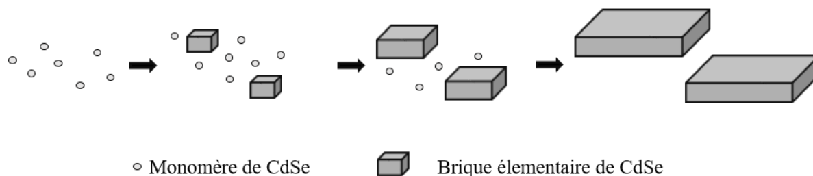
Figure 14 : Mécanisme de formation des NPLs de CdSe, proposé par Ithurria et al. 47 en 2011.
