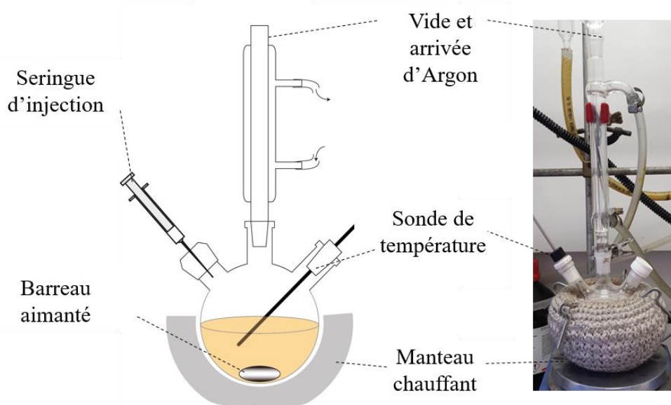
Figure 13 : A gauche, schéma d'un ballon tricol monté sur un chauffe ballon et relié à un réfrigérant permettant de faire le vide et de travailler sous atmosphère inerte avec l'entrée de l'argon. A droite photo du montage utilisé en laboratoire au LPEM.
