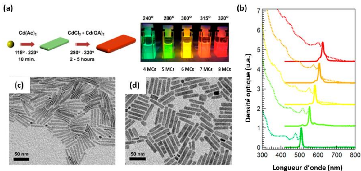
Figure 25 : Utilisation du chlorure de cadmium pour des synthèses de CdSe de différentes épaisseurs. (a) Passage des QDs de CdSe aux NPLs de CdSe 4 MCs par ajout d'acétate de cadmium. L'injection du chlorure à plus haute température et pour plusieurs heures de réaction permet d'atteindre 8 MCs. Les NPLs sont aussi étendues latéralement. (b) Absorption et émission des NPLs de CdSe de 4 MCs, 5 MCs, 6 MCs, 7 MCs et 8 MCs. (c) et (d) images au microscope électronique à transmission des NPLs de 4 MCs et 7 MCs. Issue de Christodoulou et al. 24 .
