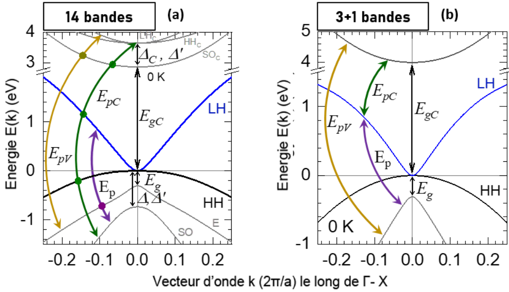
Figure 70: Représentation de la structure de bande de HgTe dans le modèle à (a) 14 bandes et (b) 3+1 bandes.
