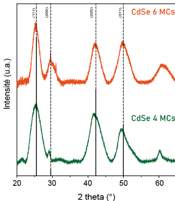
Figure 30 : Diffractogrammes des NPLs de CdSe 4 MCs (en vert) et NPLs de CdSe 6 MCs (en orange) après croissance. L'ajout de 2 MCs ne change pas la structure cristalline ZB initiale des NPLs de CdSe 4 MCs.
