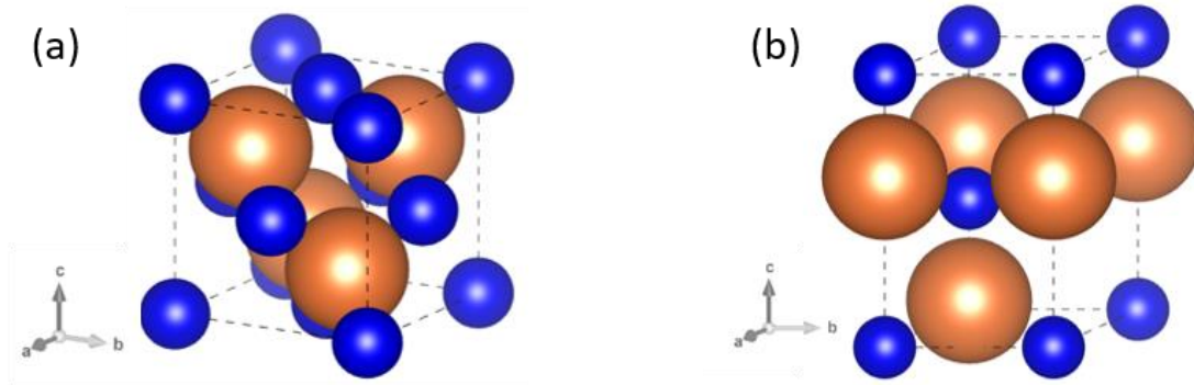
Figure 6 : Maille élémentaire de CdSe cristallisé sous forme (a) Zinc blende et (b) Wurtzite.
