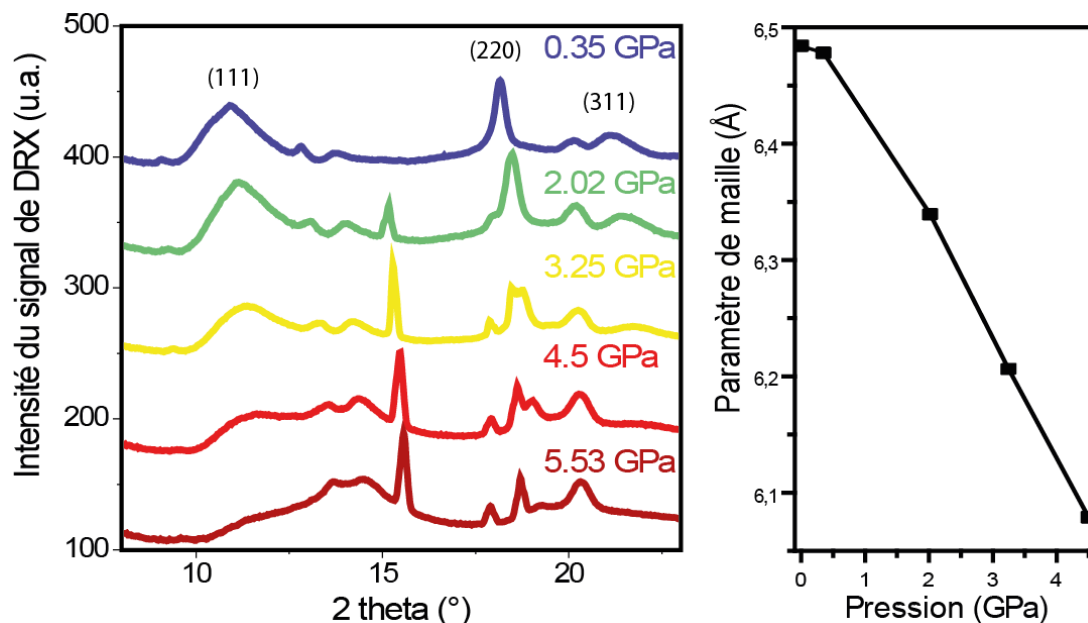
Figure 66: (a) Diffractogrammes des NPLs de HgTe sous pression de 0 GPa à 5,53 GPa. (b) Paramètre de maille des NPLs en fonction de la pression.
