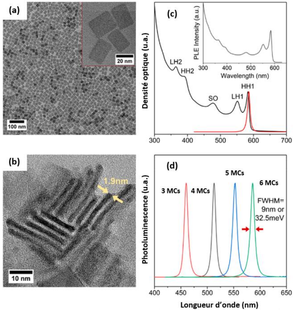
Figure 26: (a) Images de microscopie électronique à transmission des CdSe 6 MCs et (b) à haute résolution. (c) Absorption en noir et émission en rouge des NPLs de CdSe 6 MCs. L'encart représente la spectroscopie en excitation centrée à 585 \text{ nm} . Issue de Cho et al. 23 .
