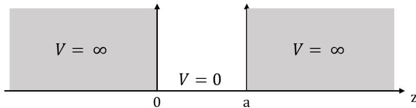
Figure 5 : Représentation d'un puit de potentiel quantique avec les porteurs de charge confinés selon une seule direction. Ici z, entre 0 et a.
