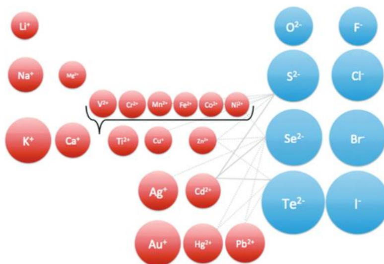
Figure 22 : Tableau périodique des éléments représentés par leurs rayons ioniques. Les tirets lient les couples d'échanges cationiques possibles avec l'anion. Reporté par la littérature jusqu'en 2012. Reproduit de Rivest et al. 87 .
