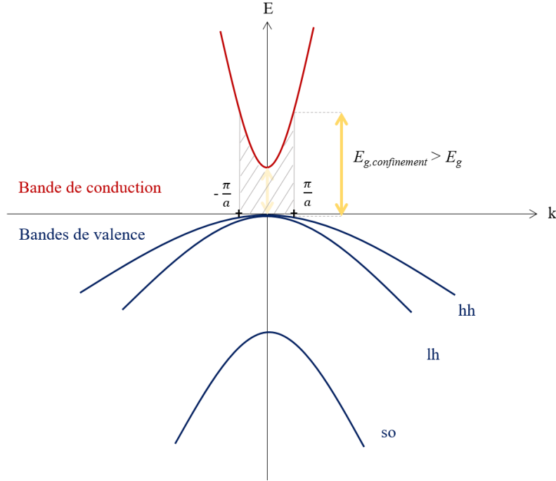
Figure 2: Structure de bande du matériau massif de CdSe. La bande de conduction et de valence sont séparées par une largeur de bande interdite E_g . À k \neq 0 , la bande de valence est dégénérée en 3 sous bandes : trou lourd, trou léger, spin orbite. Sous régime de confinement, les niveaux d'énergies sont discrets et atteignables par impulsions de \pi/a .
