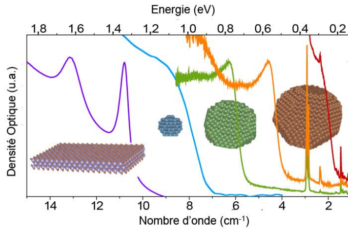
Figure 62: Spectres d'absorption des NPLs aux QDs de HgTe les plus gros en fonction du nombre d'onde et de l'énergie de confinement
