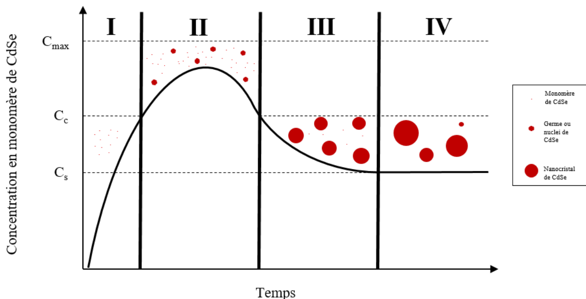
Figure 12 : Représentation qualitative du diagramme de Lamer 39 . Avec C_s , le seuil de solubilité, C_c le seuil critique de supersaturation. Le mécanisme est scindé en 4 parties. I, formation des monomères de CdSe. II, début de nucléation des germes de CdSe. III, Croissance des germes de CdSe. Il n'y a plus de nucléation à partir de cette étape. IV, mûrissement d'Ostwald à temps très long.
