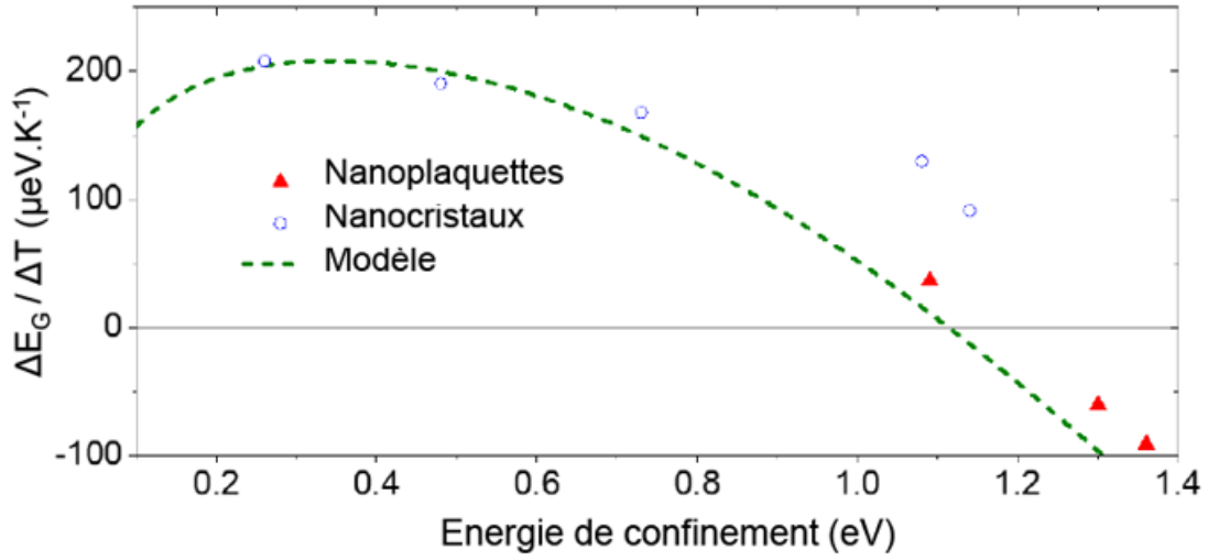
Figure 73 : Influence de la température sur les NCs de HgTe en fonction de l'énergie de confinement à T = 10 K. En pointillé vert, la tendance issue du modèle k.p à 3+1 bandes.
