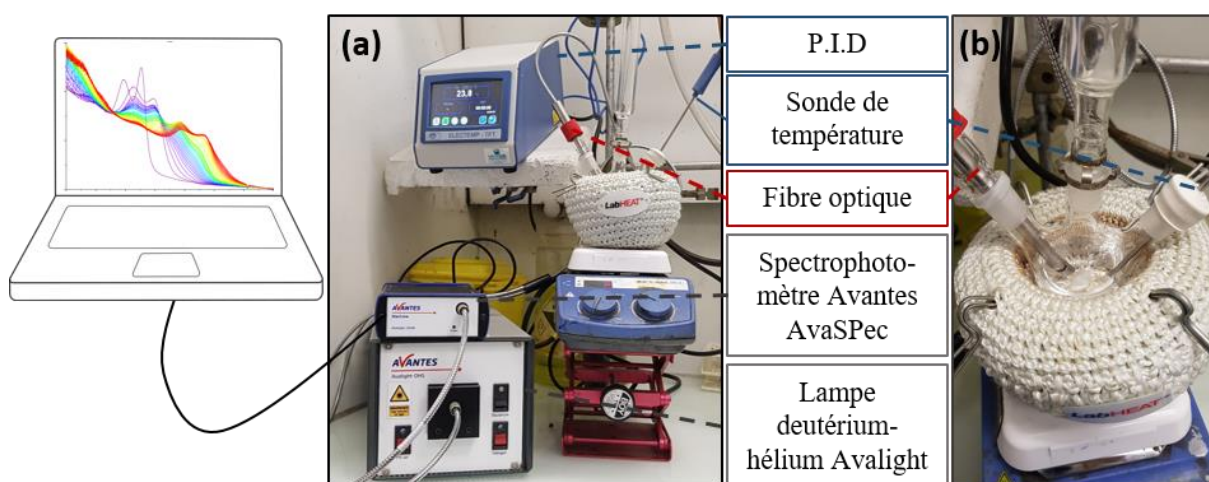
Figure 41 : (a) Photo du montage expérimental de sonde d'absorption in situ . La sonde est introduite à l'intérieur du milieu réactionnel et permet un suivi en direct de l'absorption en solution lors de la D/R. Le suivi en absorption se fait grâce au logiciel Avasoft (b) Photo du tricol contenant la sonde de température, la fibre optique pour la mesure des spectres d'absorption et la solution de croissance. Le spectrophotomètre est connecté à un ordinateur.
