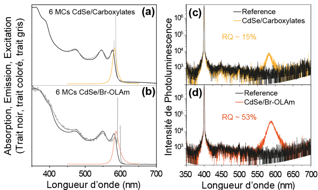
Figure 48 : Absorption, émission et excitation des NPLs de 6 MCs avec (a) des carboxylates en surface et (b) Bromure/Oleylamine en surface. (c) et (d) spectres de référence de la mesure du rendement quantique pour respectivement les NPLs de CdSe 6 MCs avec les carboxylates et Bromure/Oleylamine en surface.
