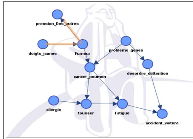
FIGURE 5.14 – Structure de réseau Bayésien apprise en utilisant l’algorithme Taboo de BayesiaLab, en omettant la variable "anxiété".
