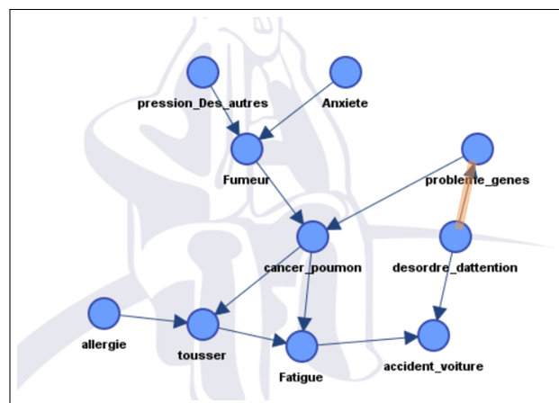
FIGURE 5.19 – Structure de réseau Bayésien apprise en utilisant l’algorithme EQTaboo ou celui des classe d’équivalence de BayesiaLab, en omettant la variable "doigts jaunes".
