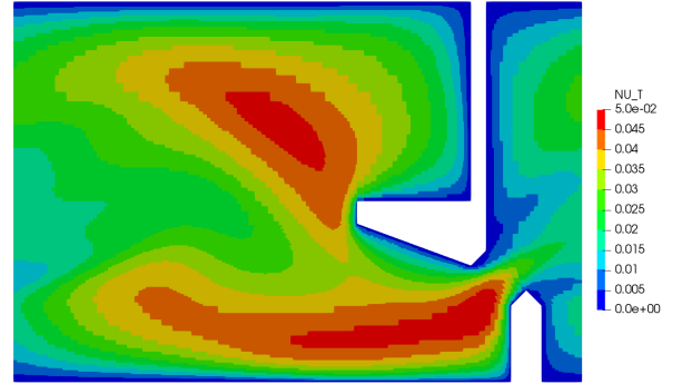
(d) Turbulent viscosity \nu_T field with code_saturne .
