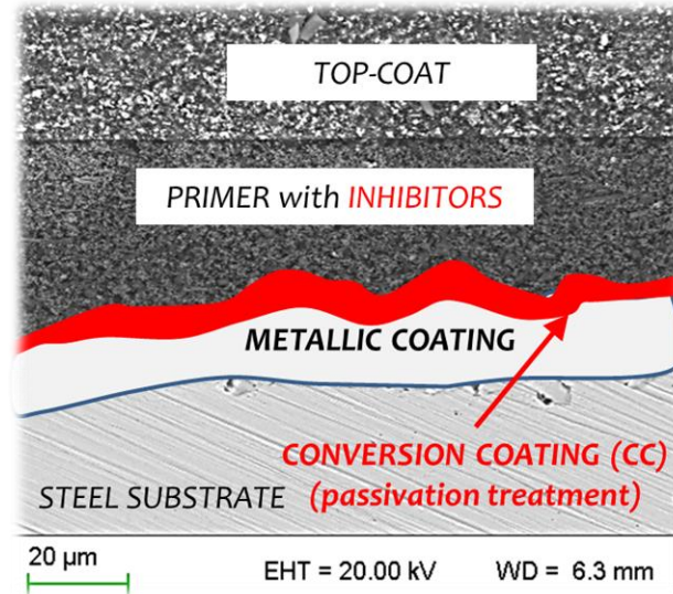
Figure 1.2: Schéma typique d'un système de protection contre la corrosion (échelle non respectée)
