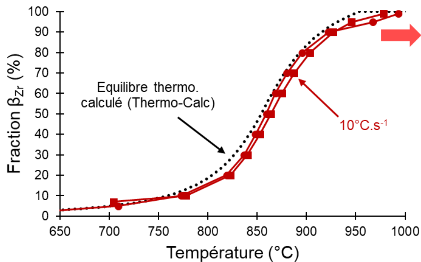
Figure V.3. Cinétiques de transformation au chauffage à 10^{\circ}\text{C}\cdot\text{s}^{-1} , après un passage dans le domaine \beta_{\text{Zr}} . Les données de dilatométrie et de DRXS sont respectivement représentées par des marqueurs rectangulaires et ronds.
