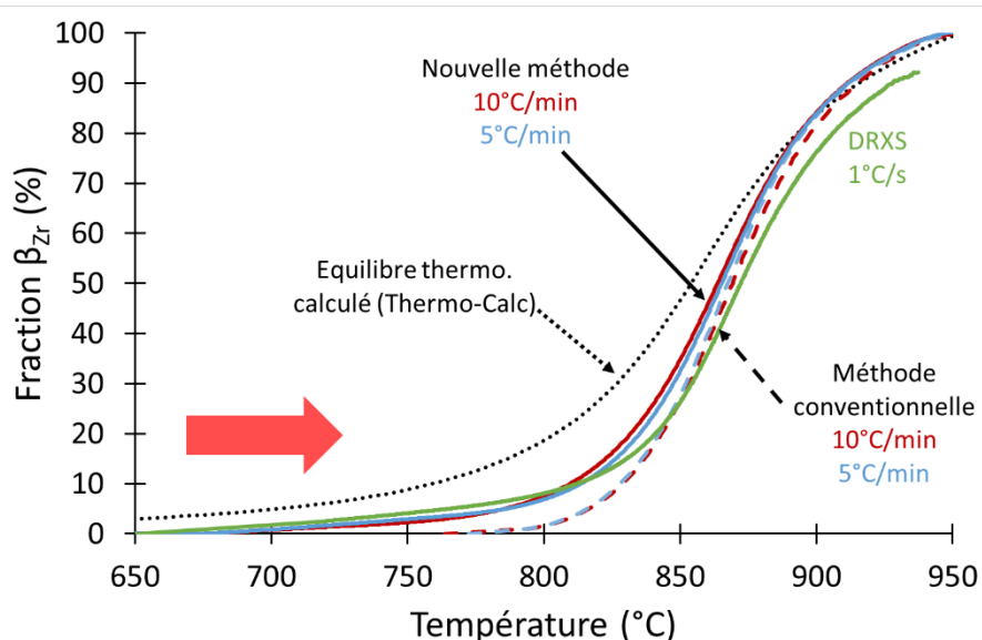
Figure IV.25. Comparaison des cinétiques obtenues en calorimétrie entre la méthode conventionnelle et la nouvelle méthode. La courbe obtenue en DRXS à 1°C.s -1 est aussi tracée comme référence.
